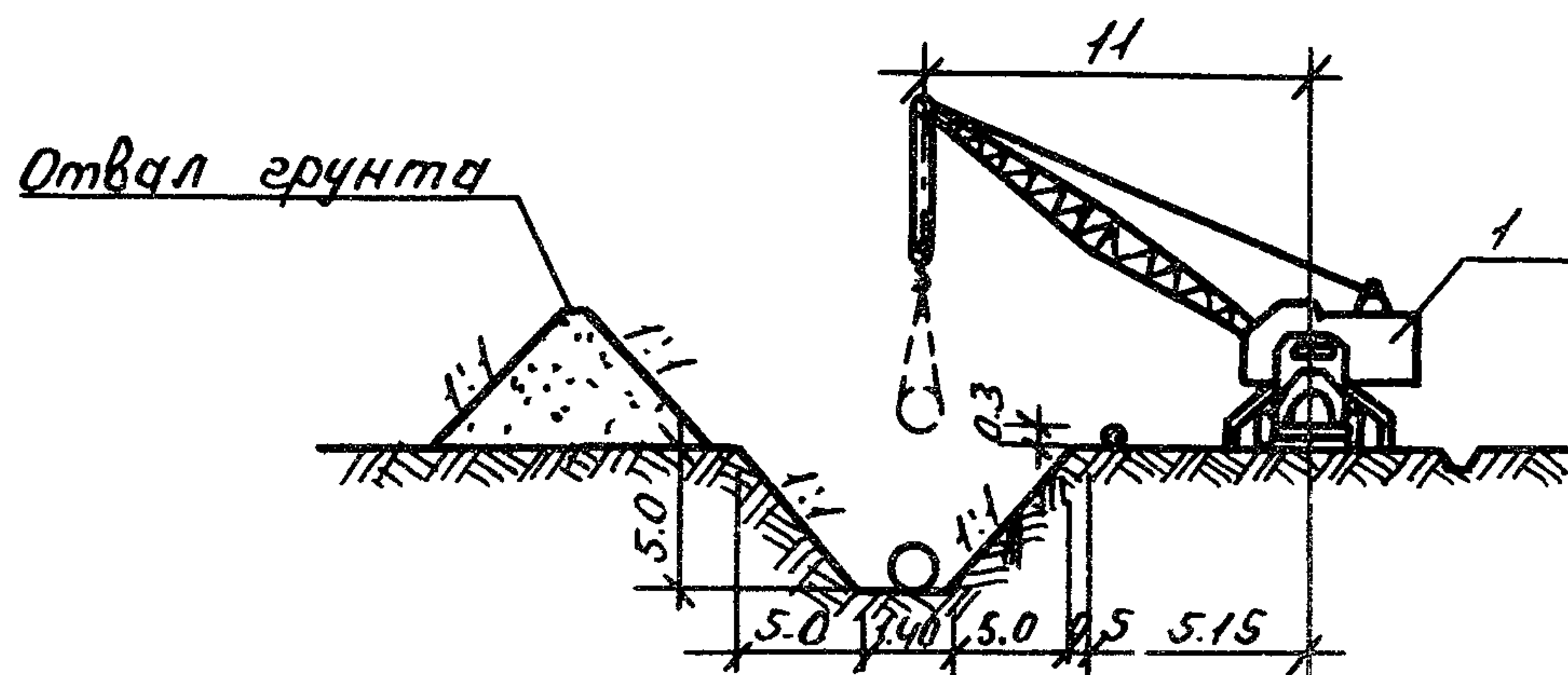
Разрез по А-А РИС. 1. Схема производства работ
