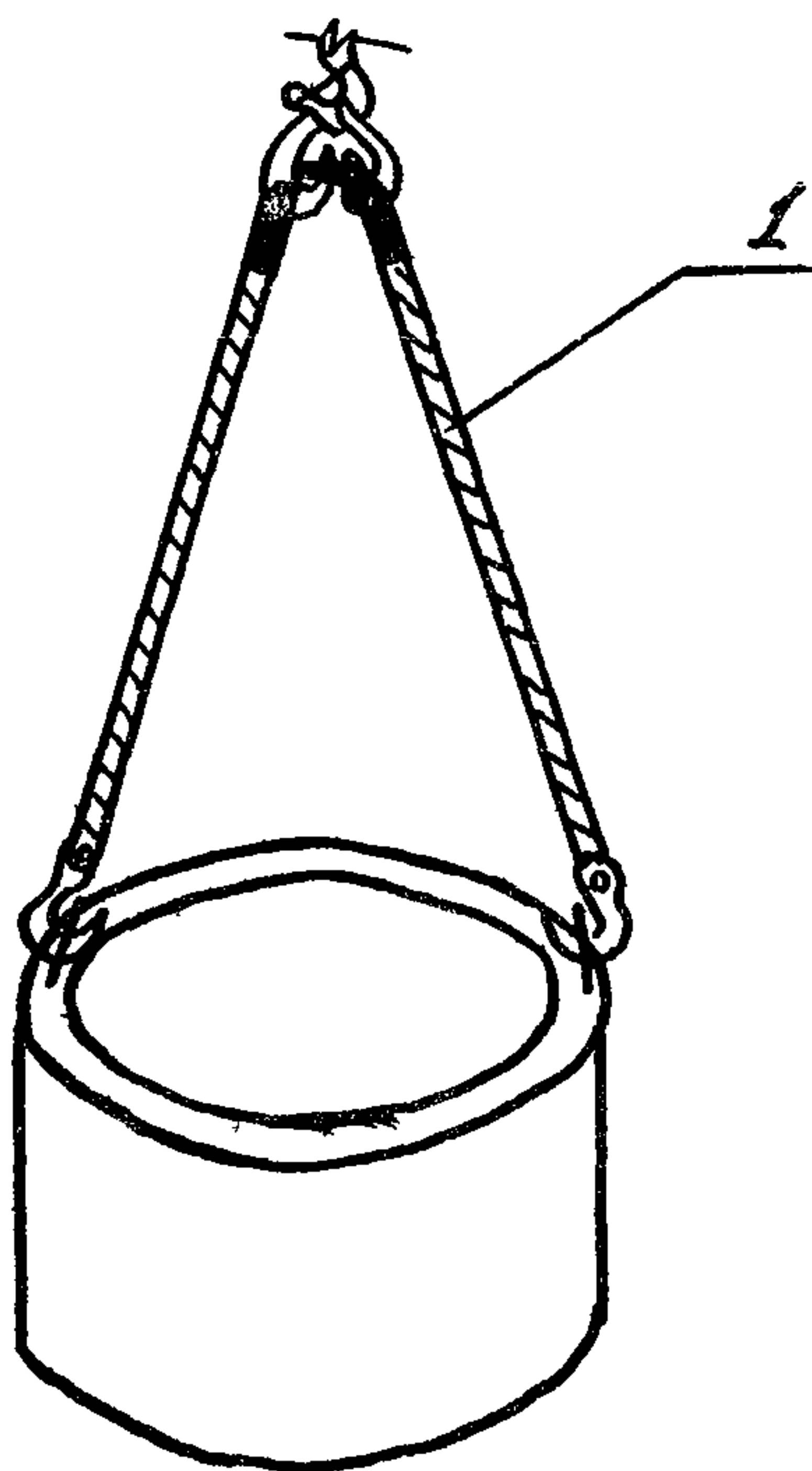
Рис. 8. Строповка блоков колодца 1 - двухветвевой строп
