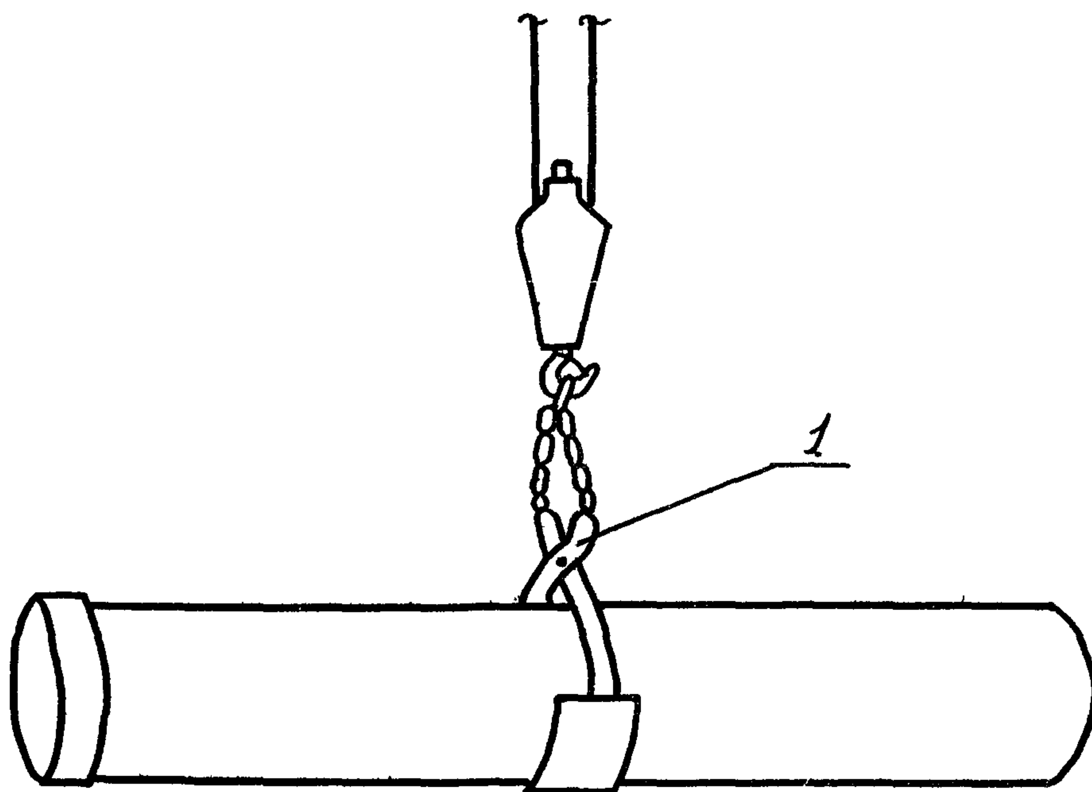
Рис. 7. Строповка труб 1 - клещевой захват
