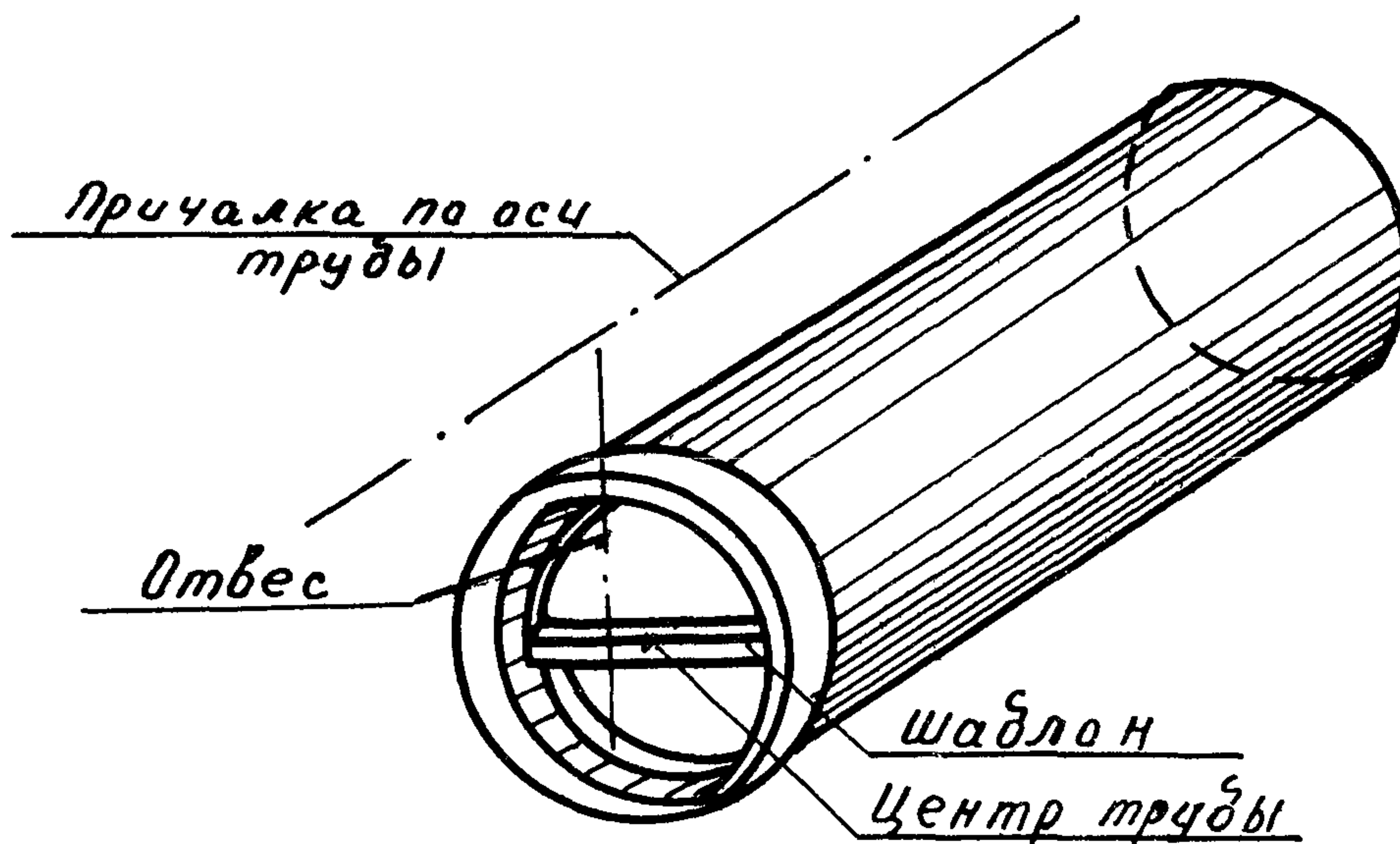
Рис. 2. Центровка труб со стороны раструба
