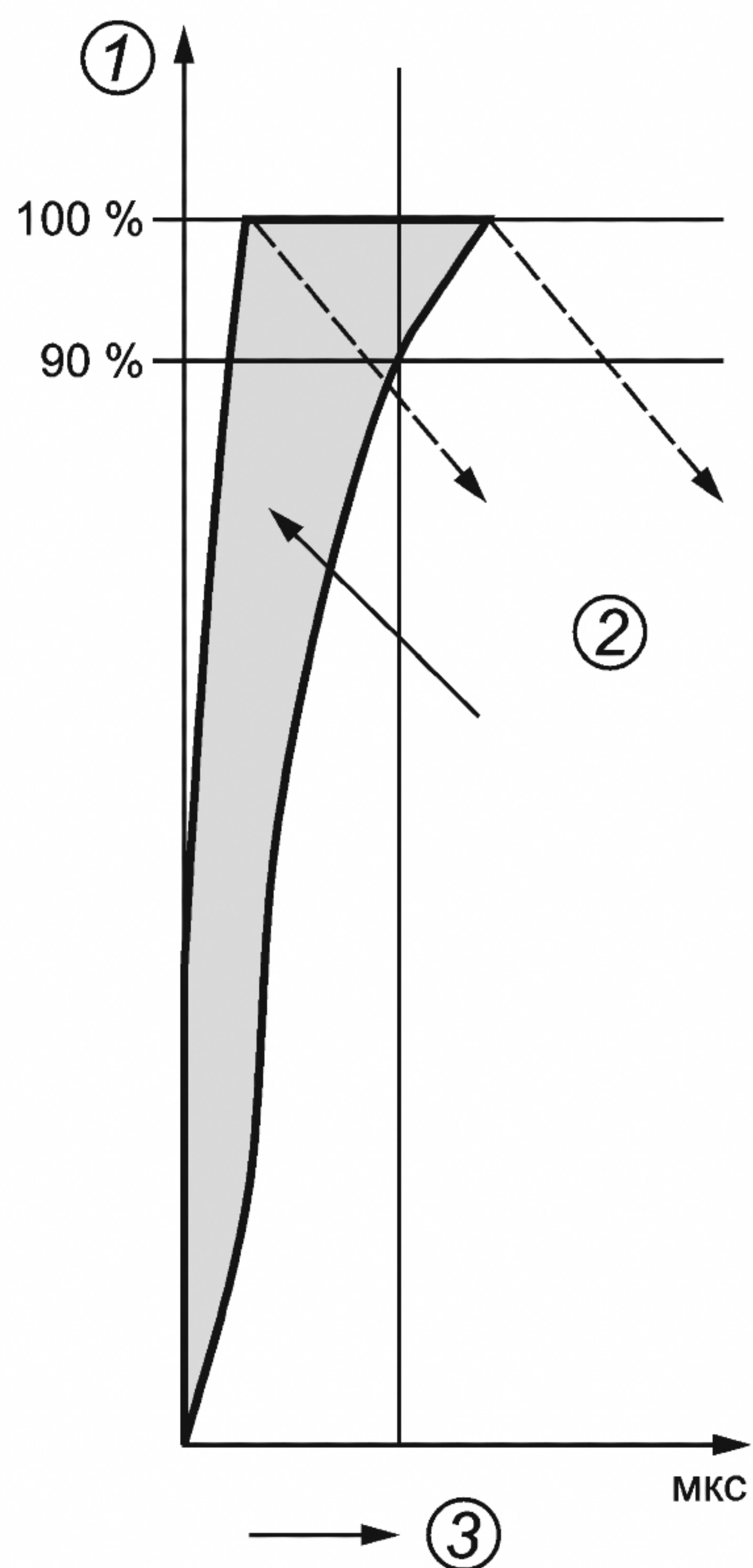
1 — действующее напряжение; 2 — диапазон времени подъема фронта волны; 3 — не более 75 мкс
