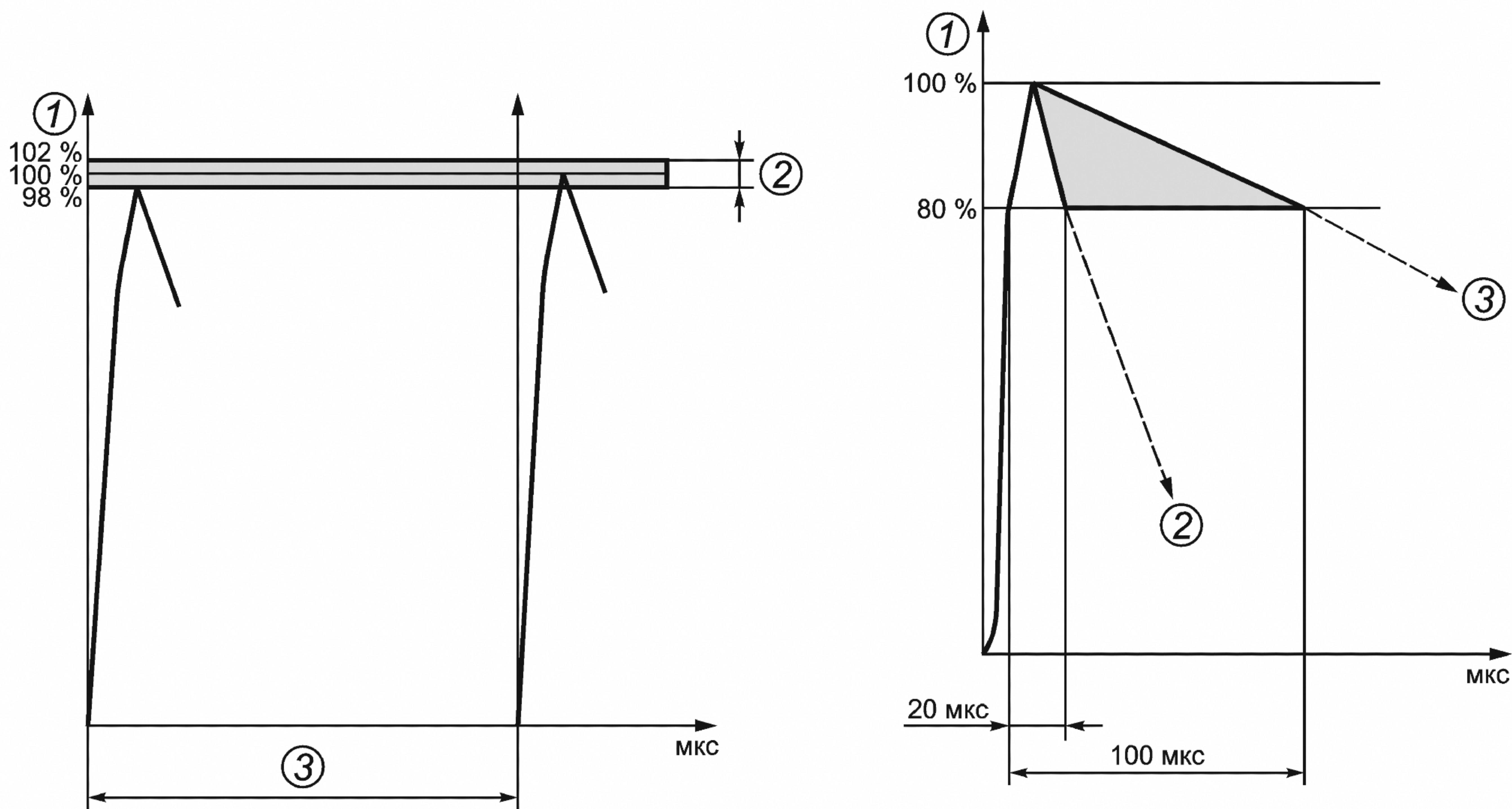
1 — действующее напряжение; 2 — минимальная продолжительность импульса; 3 — максимальная продолжительность импульса
