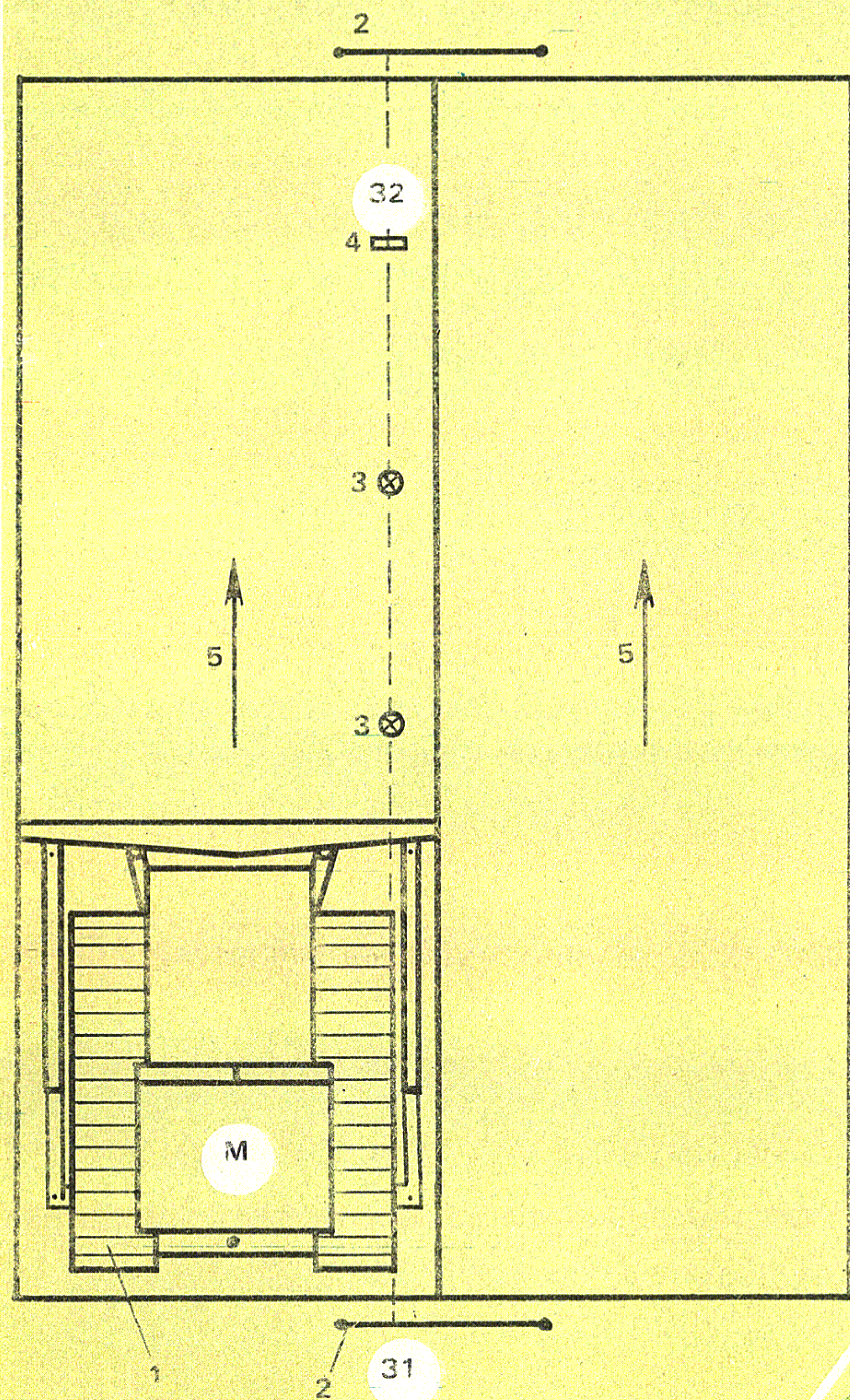
СХЕМА ОРГАНИЗАЦИИ РАБОЧЕГО МЕСТА 1 — бульдозер; 2 — обноски; 3 — маяки-указатели; 4 — визирка; 5 — направление движения; М — машинист; 31, 32 — землекопы
