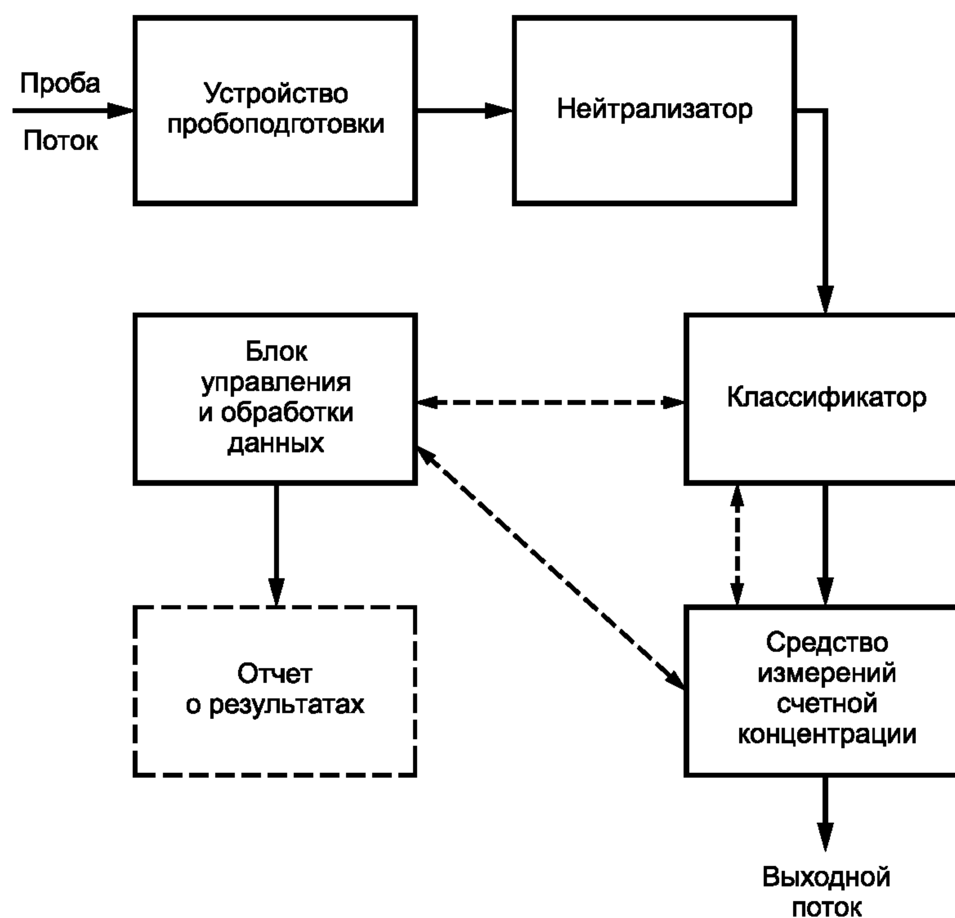
Рисунок 1 — Типичная блок-схема САДЭП
