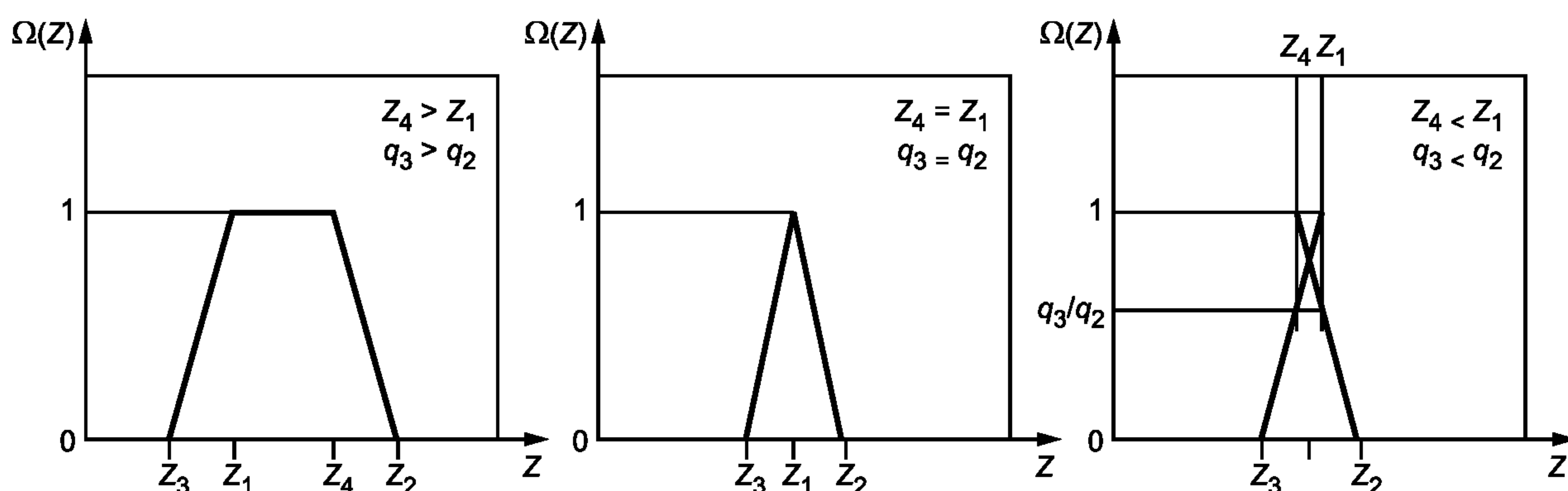
Рисунок Б.2 — Передаточные функции цилиндрического классификатора
