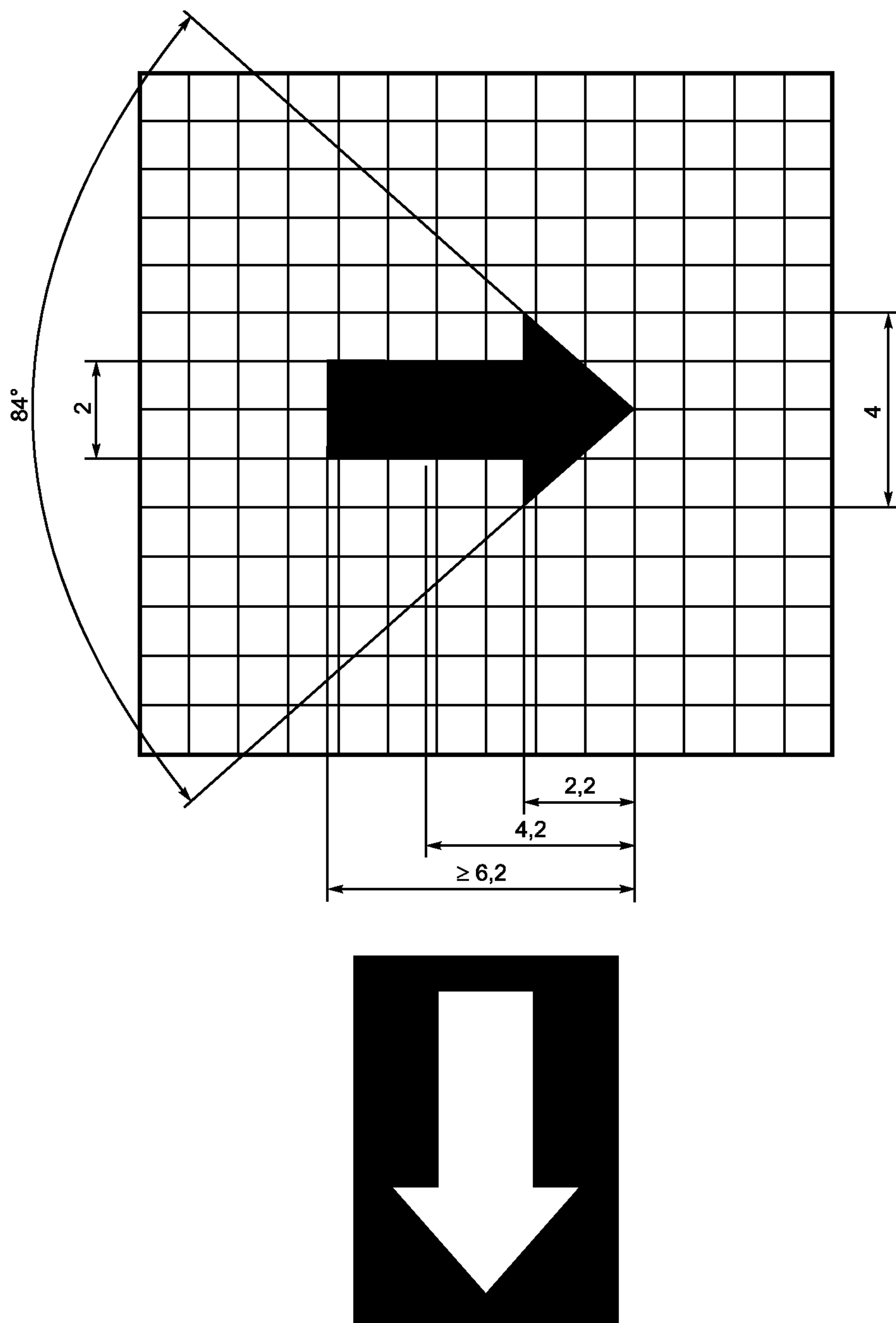
Рисунок D.22 — Стрелка, обозначающая давление или силу
