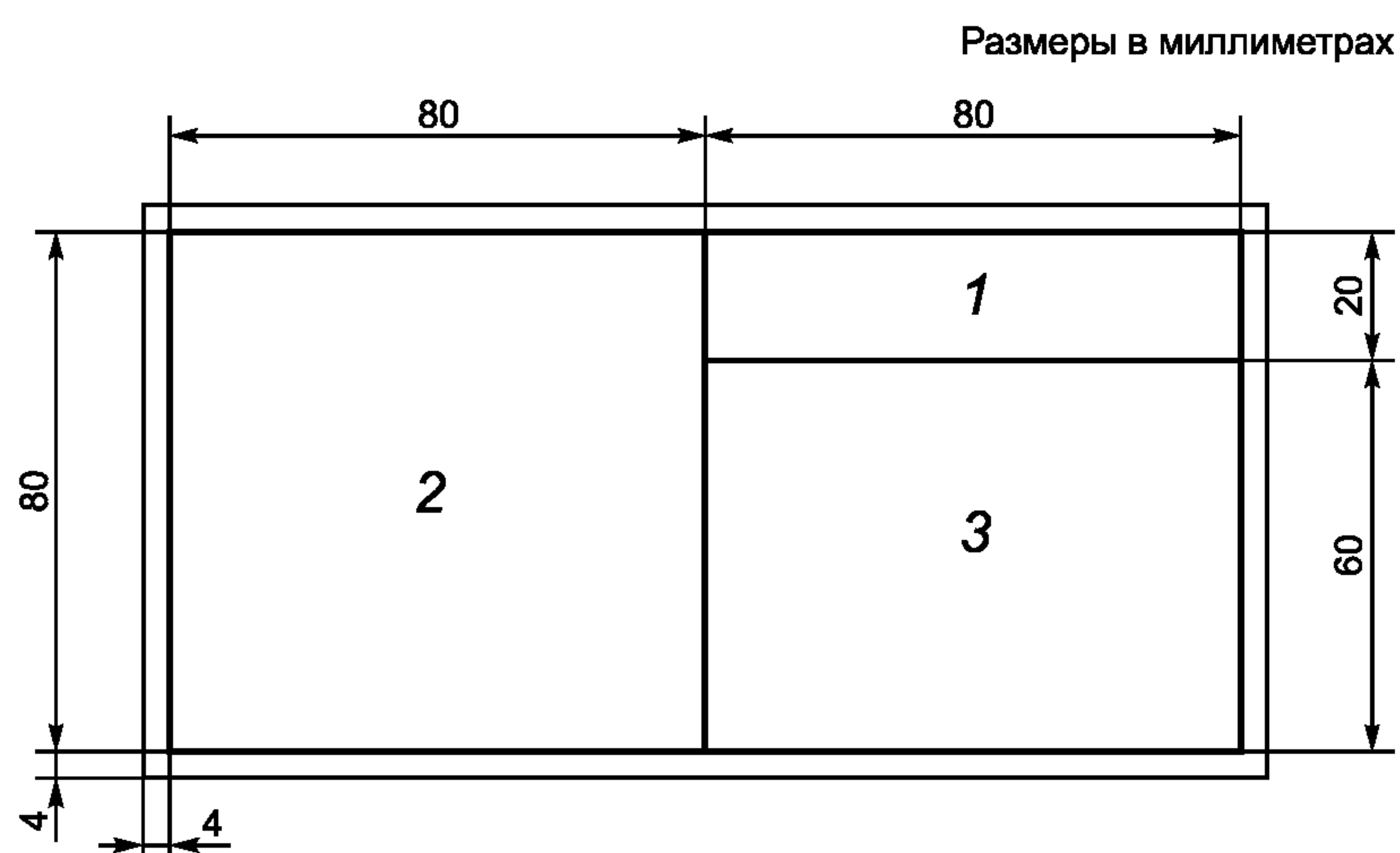
а) Горизонтальная конфигурация
