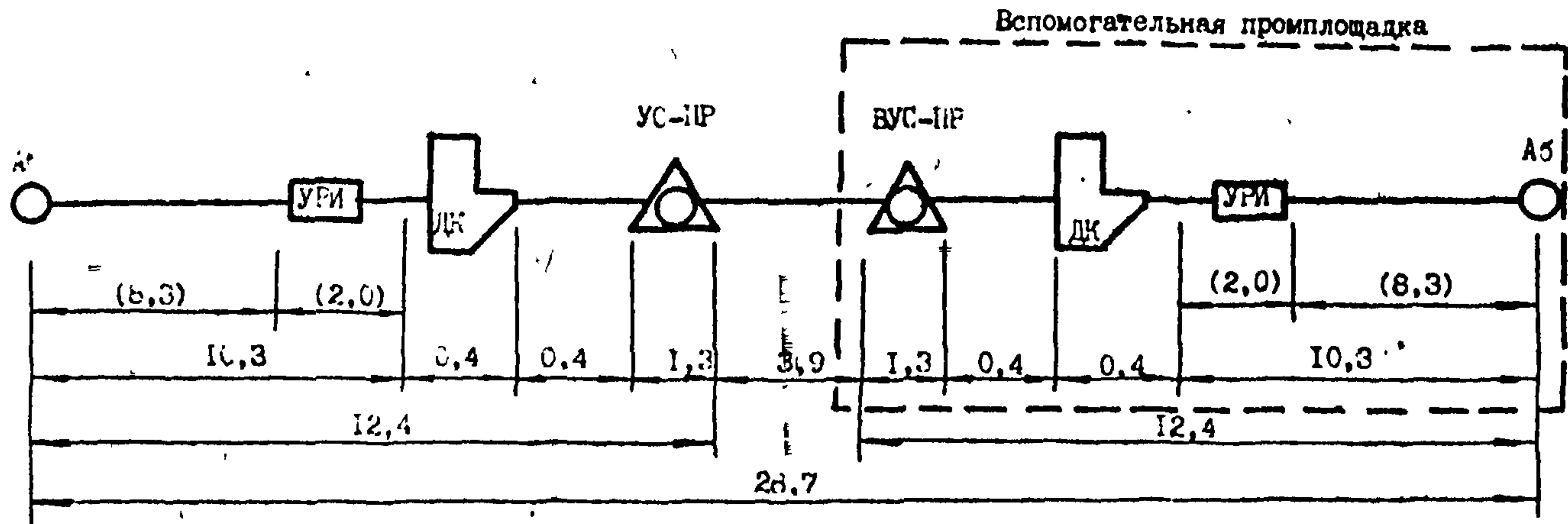
Рис. 6.5. Распределение затухания, дБ, на телефонной сети предприятия.
