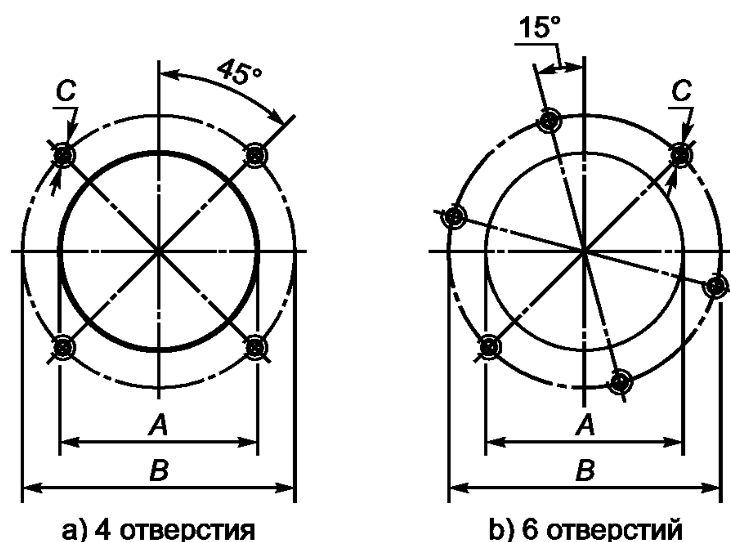
Рисунок 1 — Присоединительные размеры горелок
