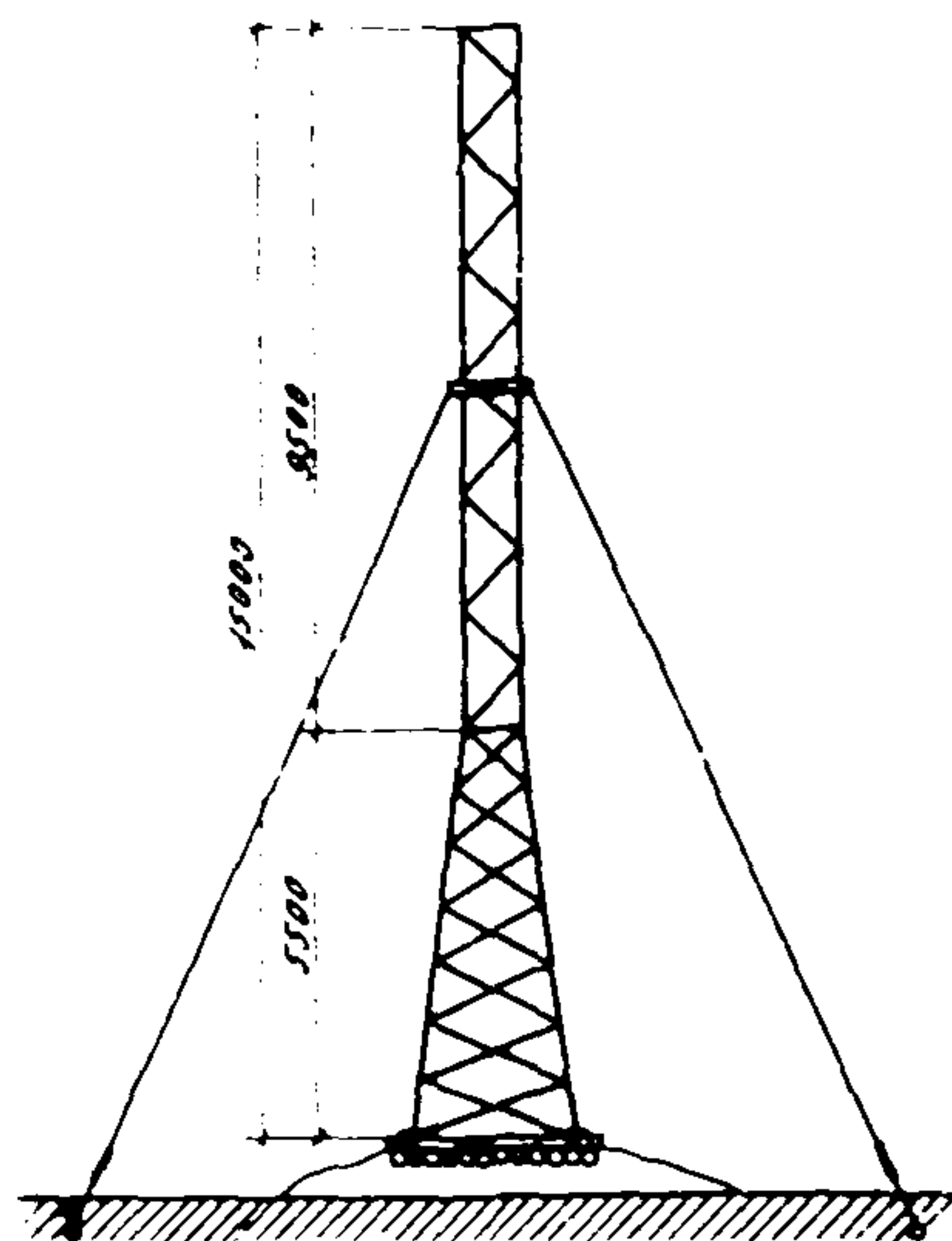
Рис.5. Общий вид мачты УКВ радиостанции (15 м)
