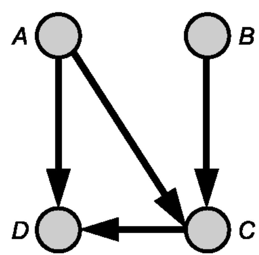
Рисунок В.11 — Пример сети Байеса
