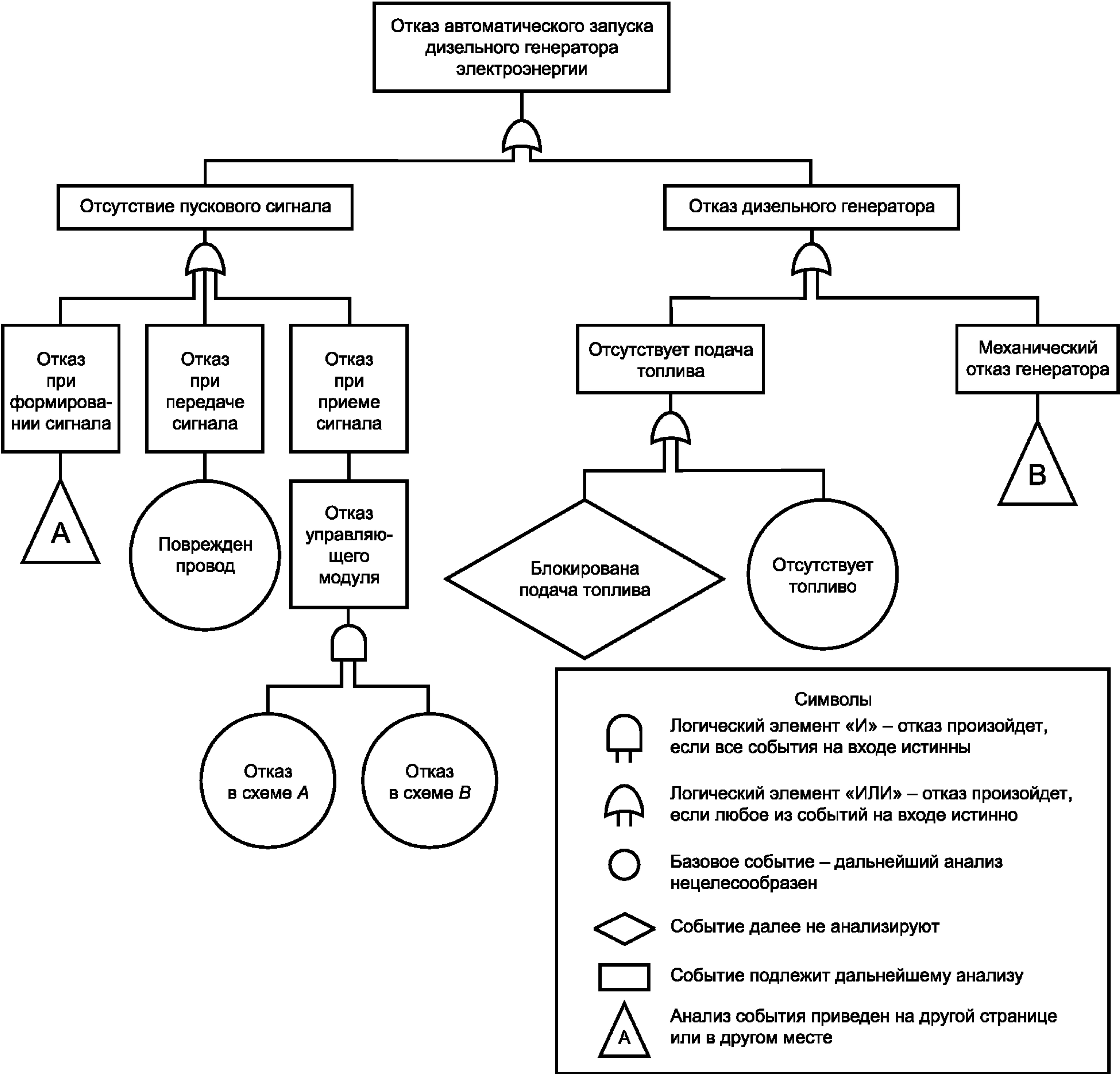
Рисунок В.2 — Пример метода FTA
