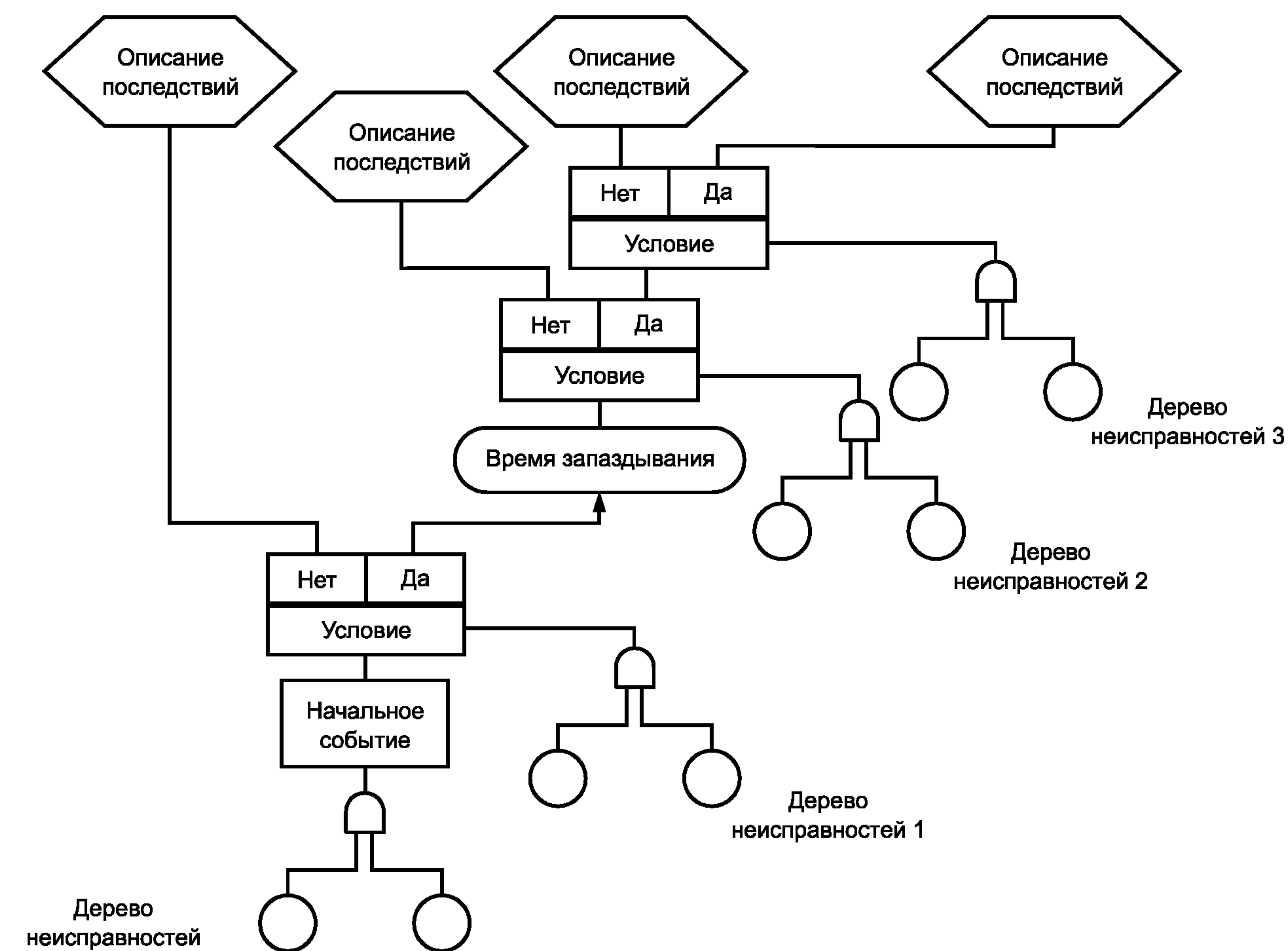
Рисунок В.4 — Пример анализа причин и последствий
