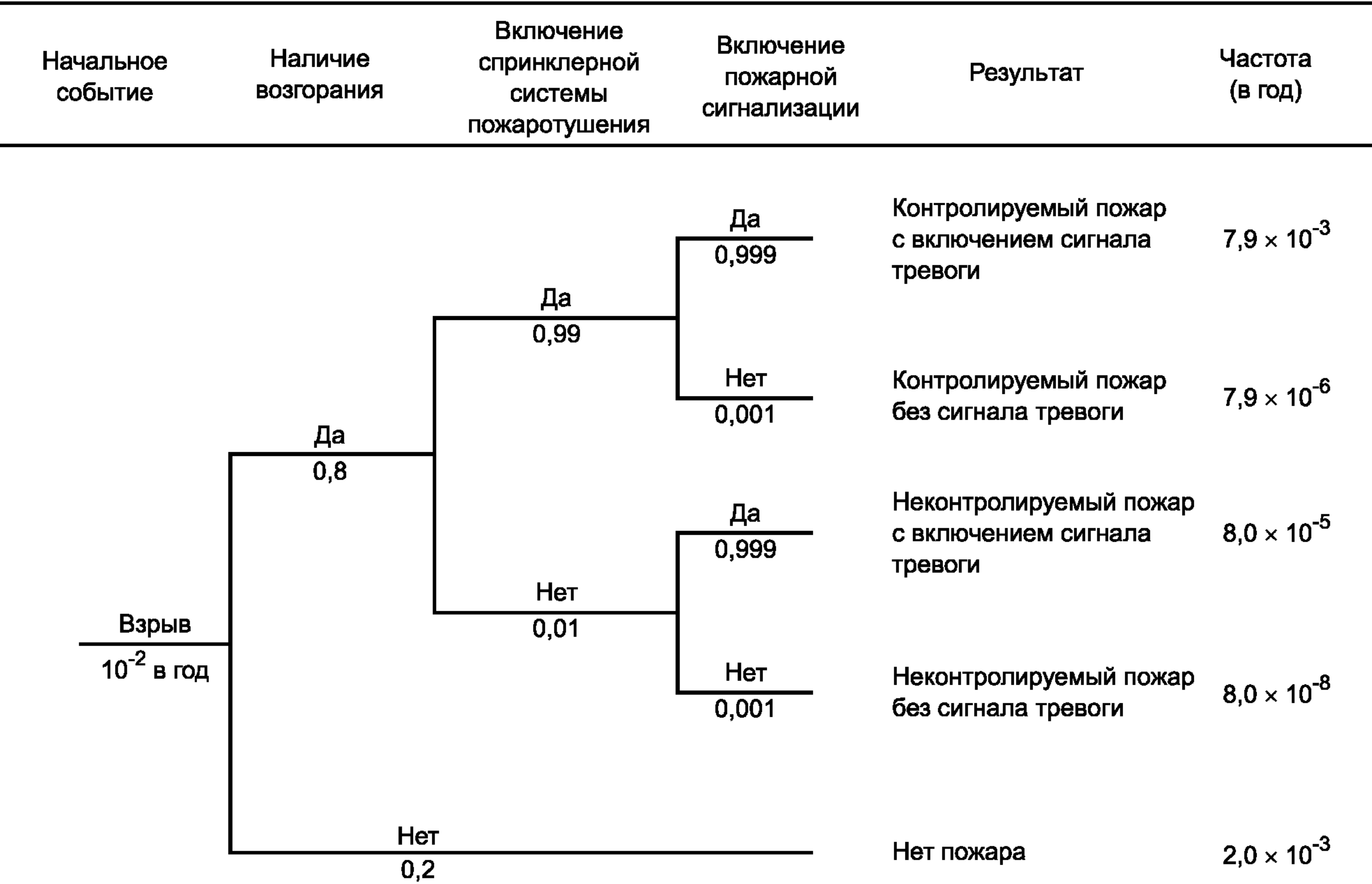
Рисунок В.3 — Пример дерева событий
