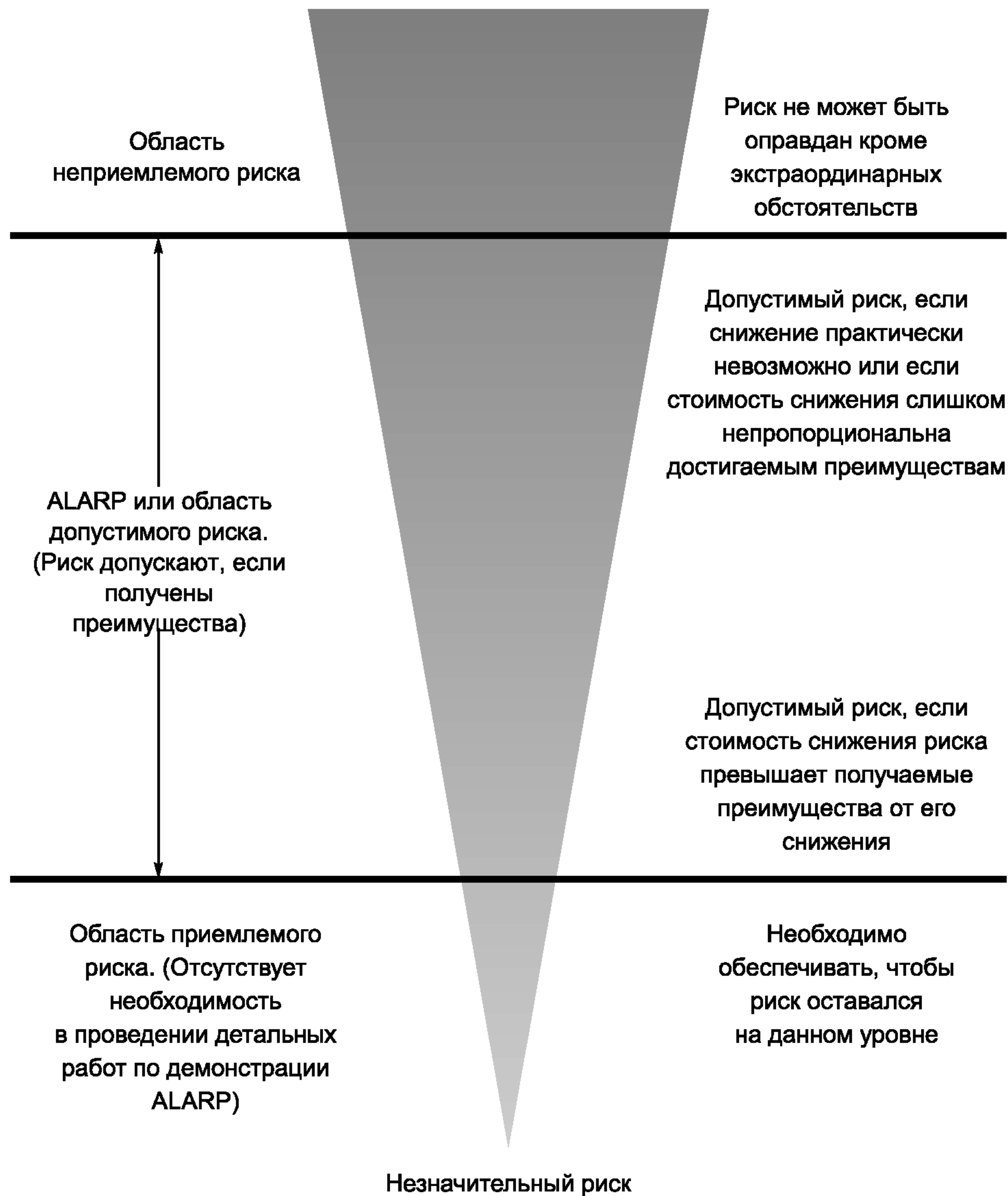
Рисунок В.15 — Концепция ALARP
