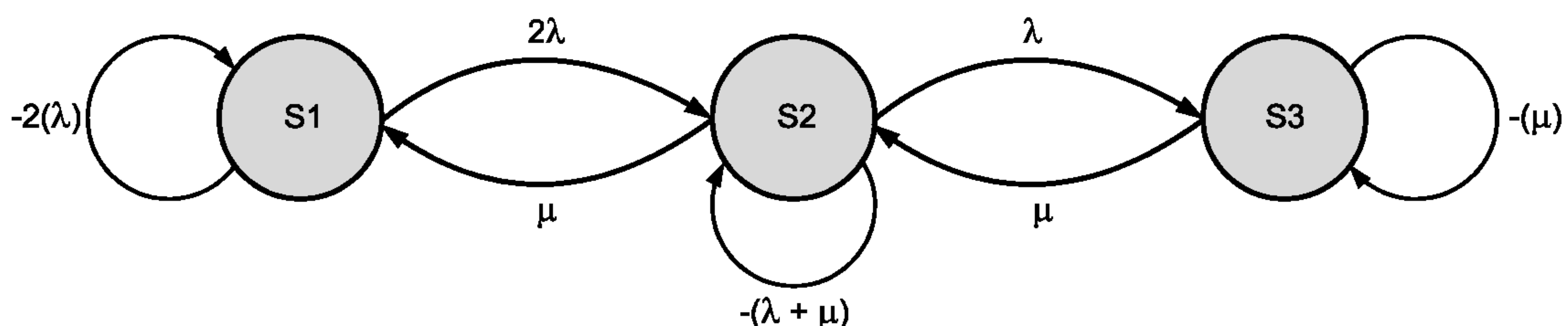
Рисунок В.10 — Пример диаграммы состояний перехода
