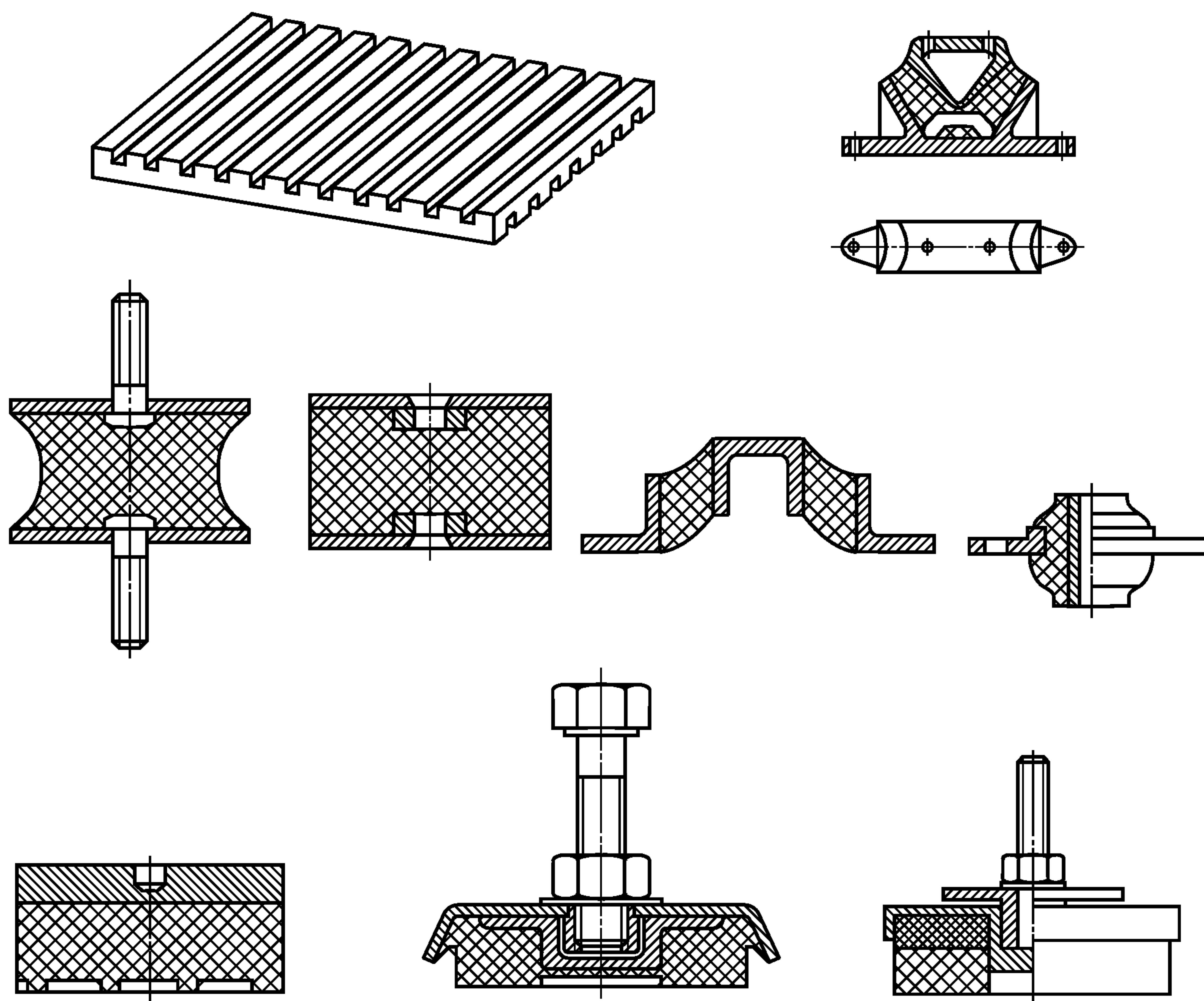
Рисунок А.1 — Примеры пружин из эластомерных материалов
