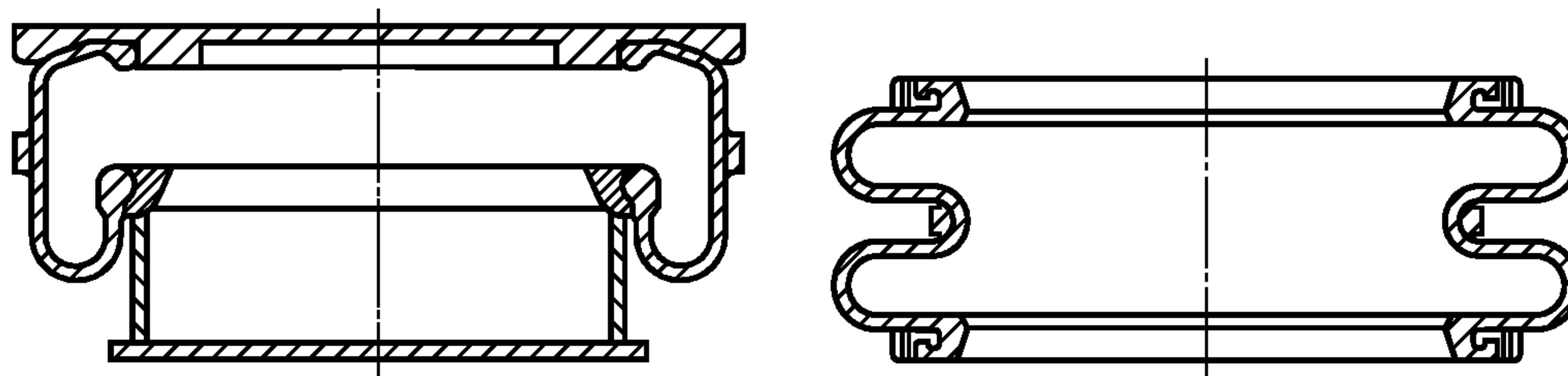
Рисунок А.4 — Примеры пневматических пружин
