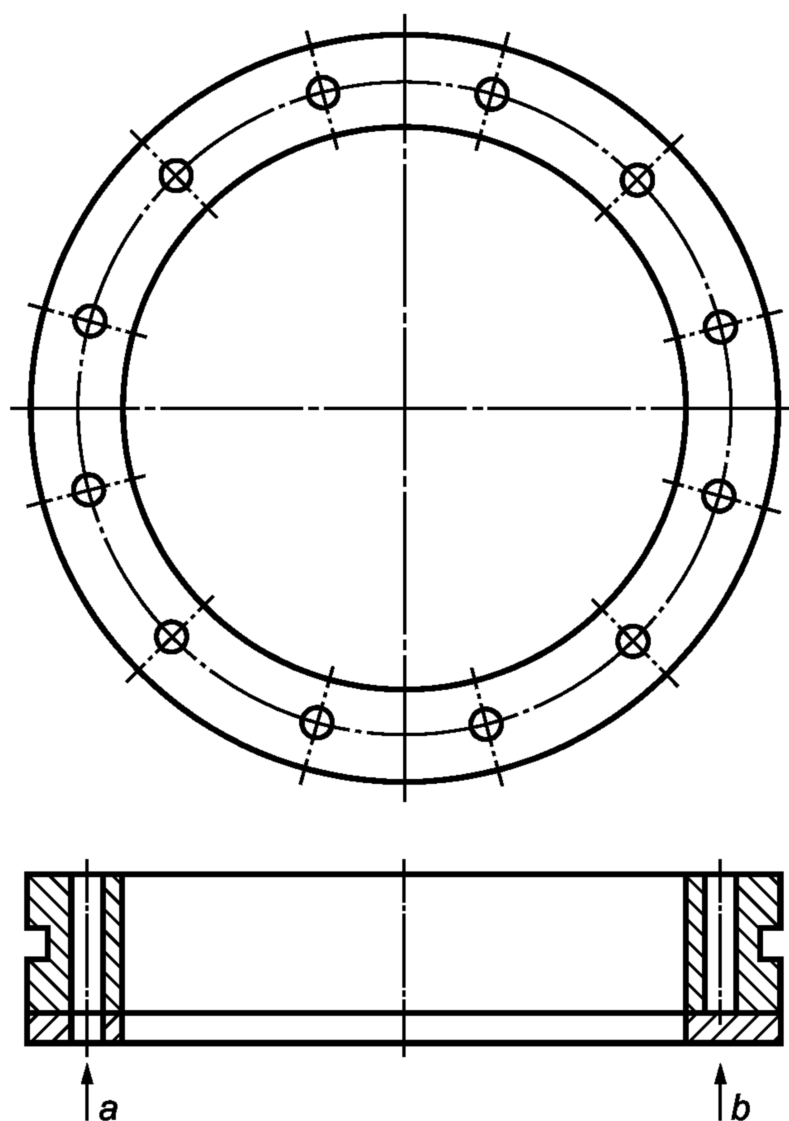
Половина секции с нижним кольцом
