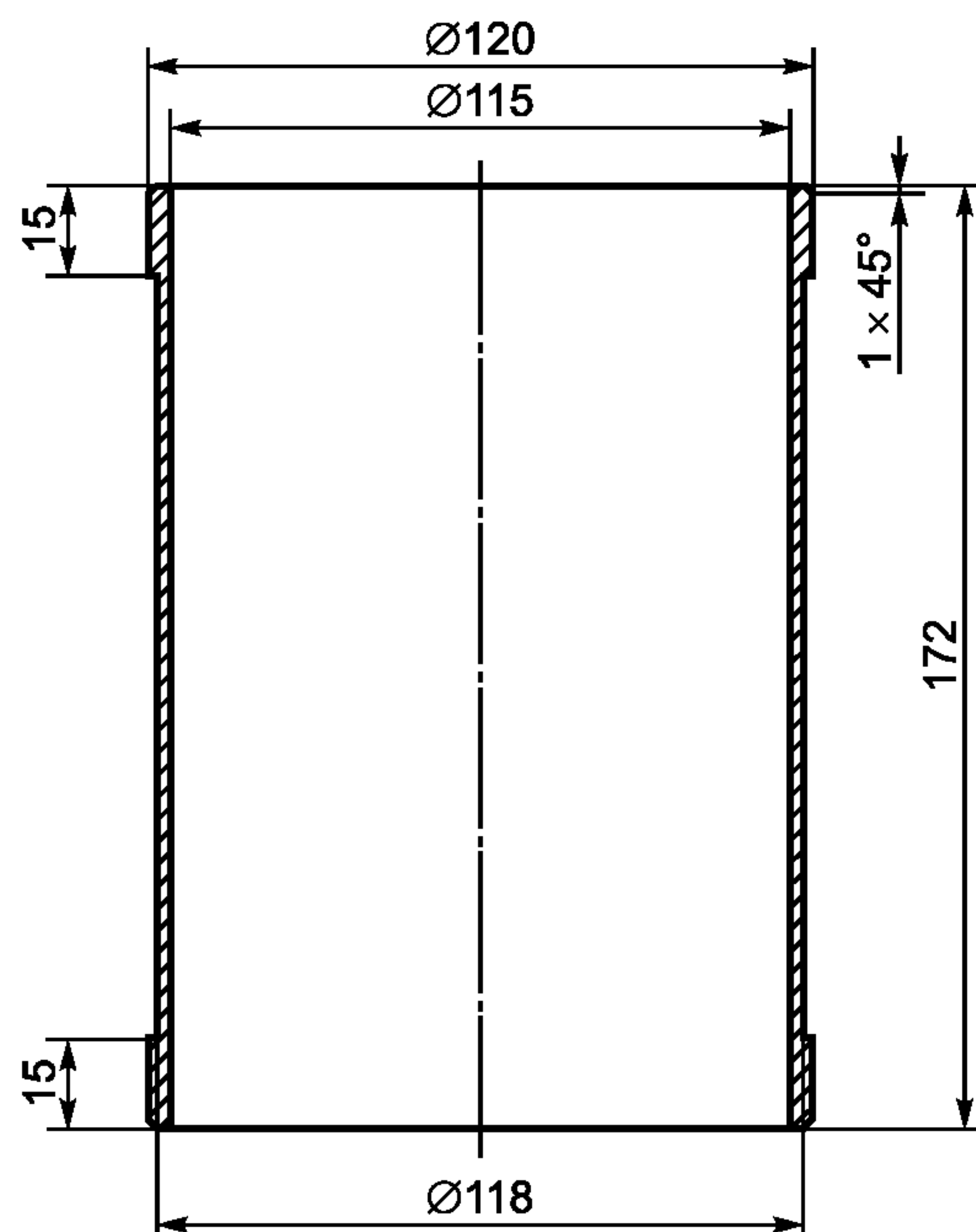
Рисунок 4 — Корпус цилиндра
