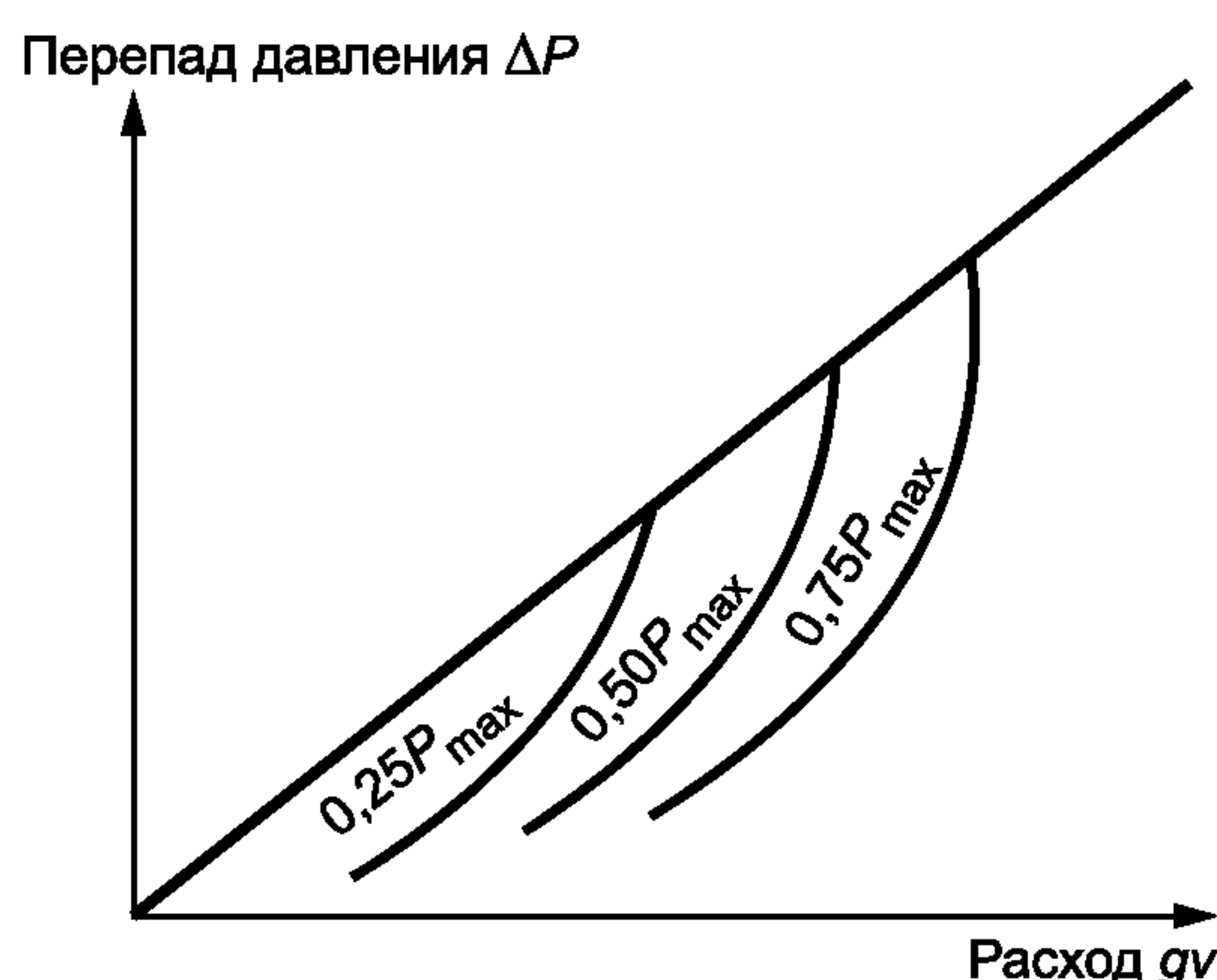
Рисунок 8 — Пример расходных характеристик
