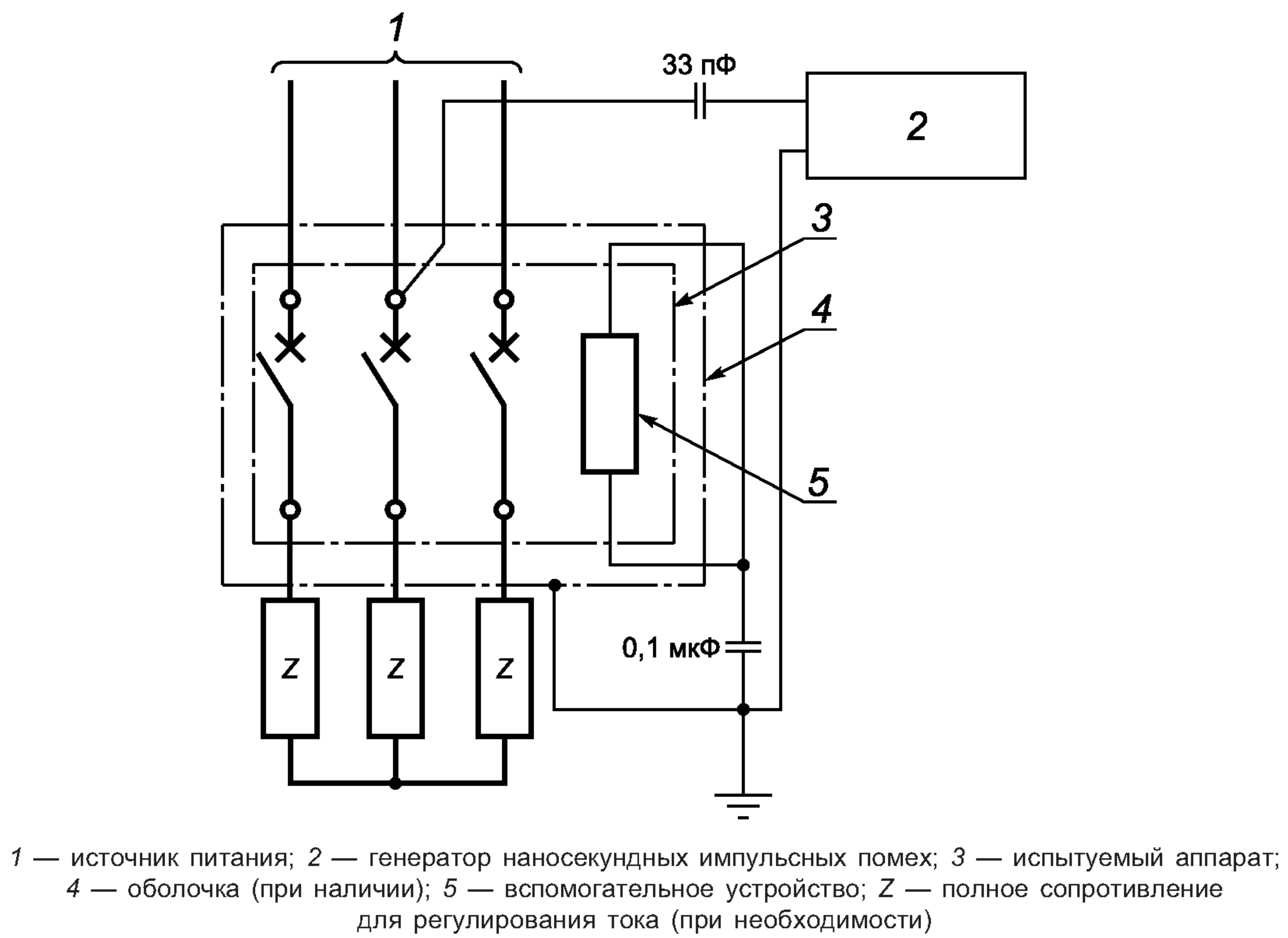
Рисунок 15 — Испытательная цепь для проверки устойчивости к наносекундным импульсным помехам. Трехфазная конфигурация цепи
