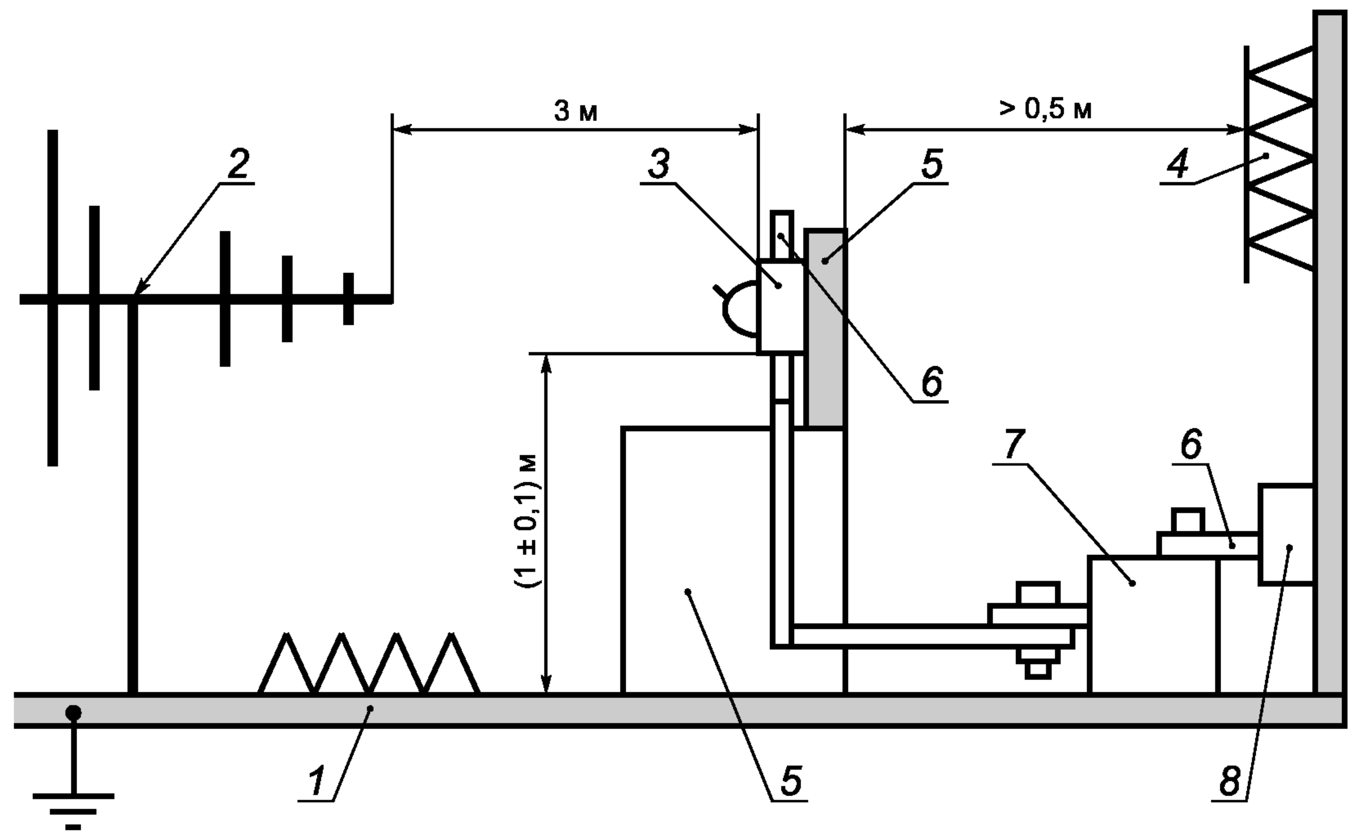
1 — заземляющая пластина; 2 — антенна; 3 — испытуемый аппарат; 4 — поглотители эха; 5 — изолирующий материал; 6 — соединения, удерживаемые на минимуме; 7 — трансформатор; 8 — главный фильтр
