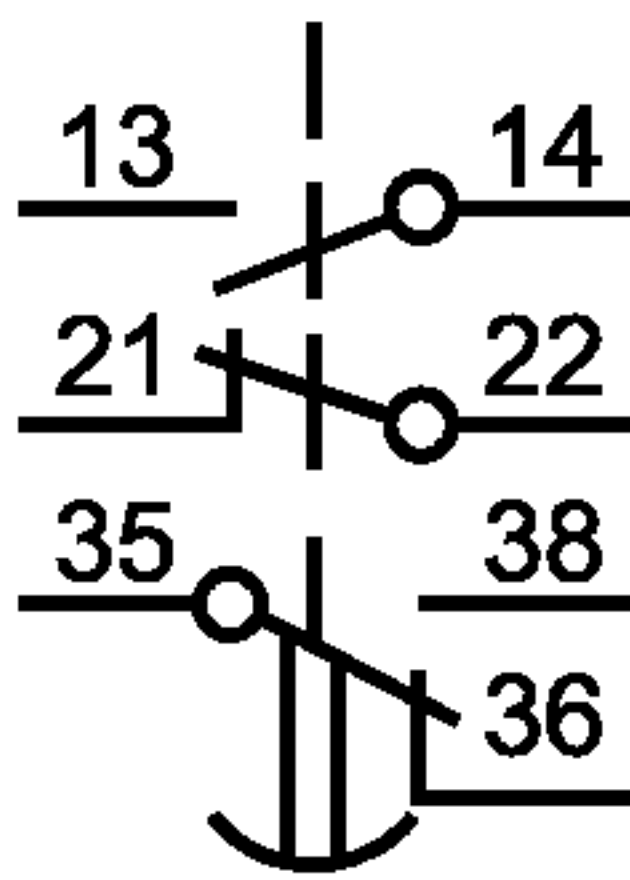
Три контактных элемента
