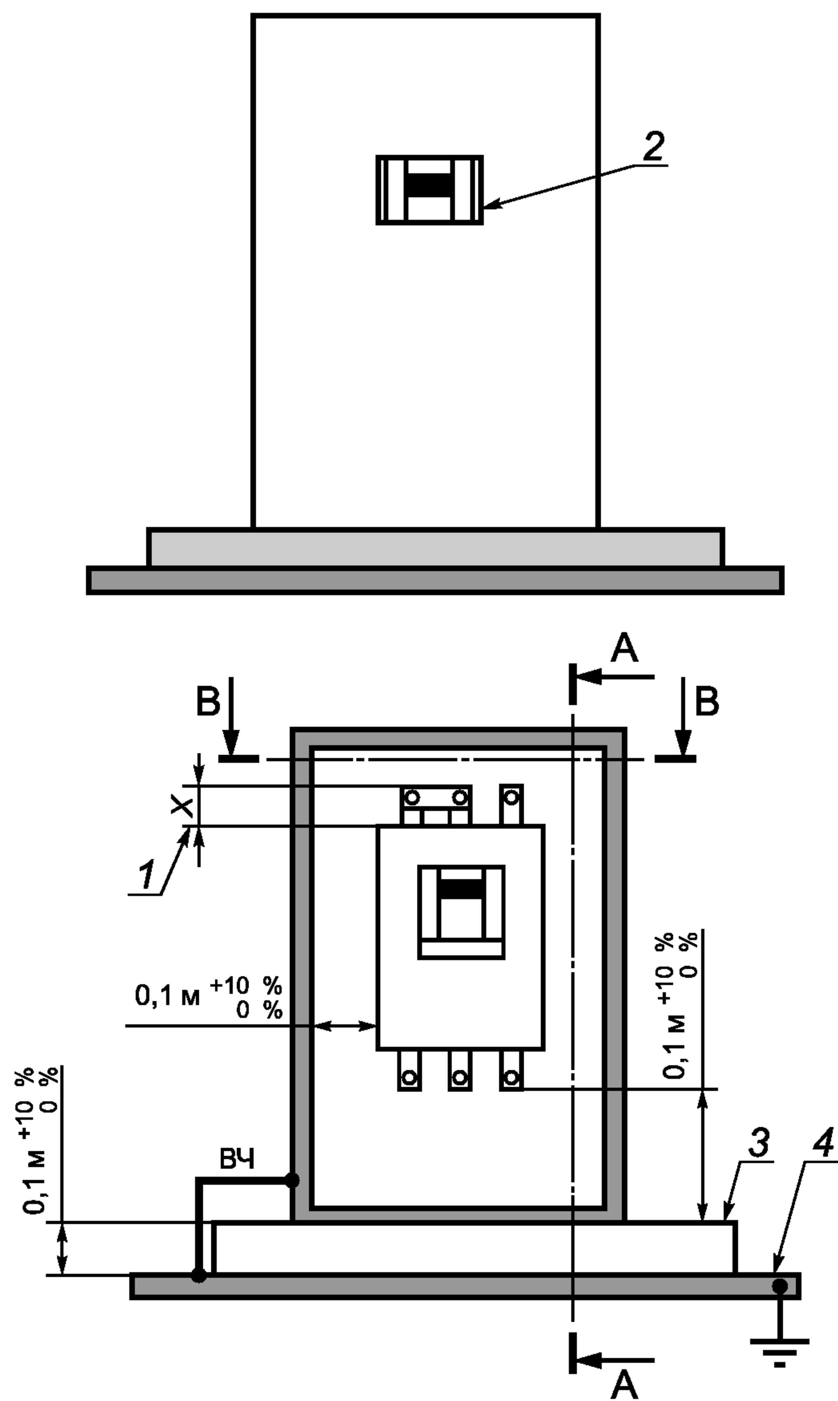
1 — минимальный размер X; 2 — минимальное отверстие дверцы согласно инструкции изготовителя; 3 — изолирующее основание; 4 — заземляющая пластина
