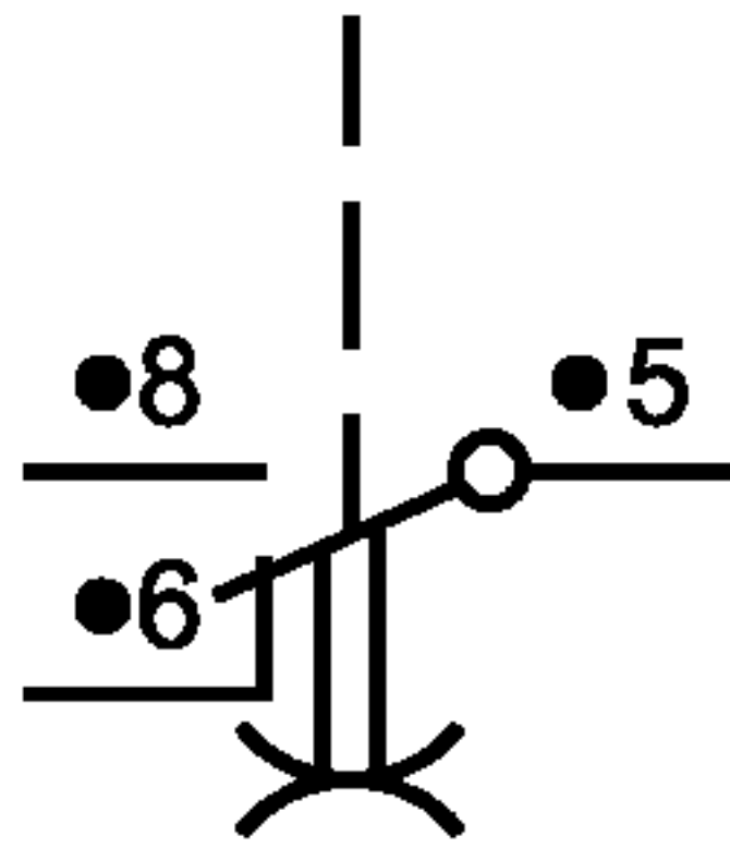
Переключающий контакт с замедлением в обоих направлениях
