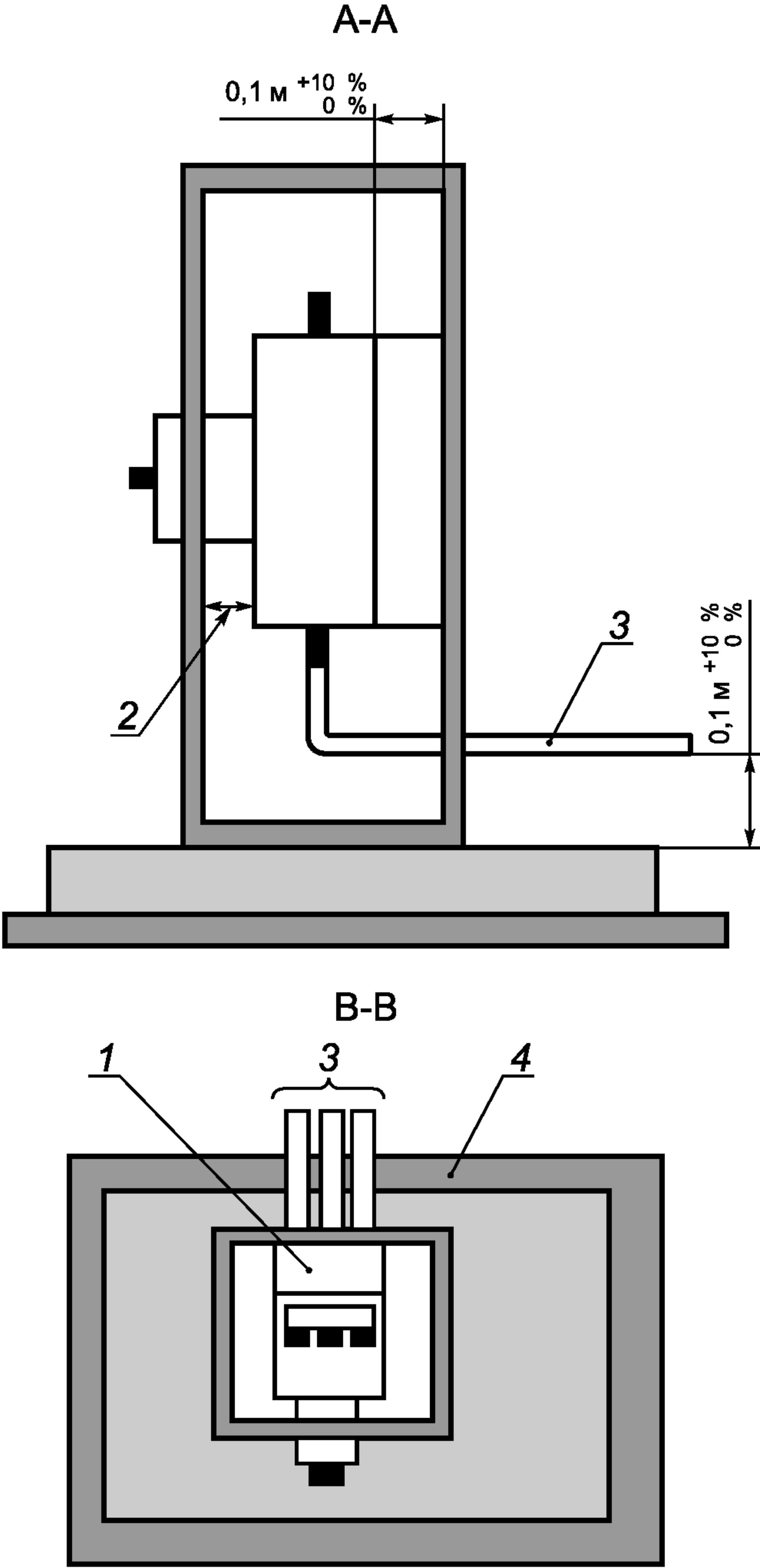
1 — изолирующее основание; 2 — минимальное расстояние в соответствии с инструкцией изготовителя; 3 — источник питания; 4 — заземляющая пластина
