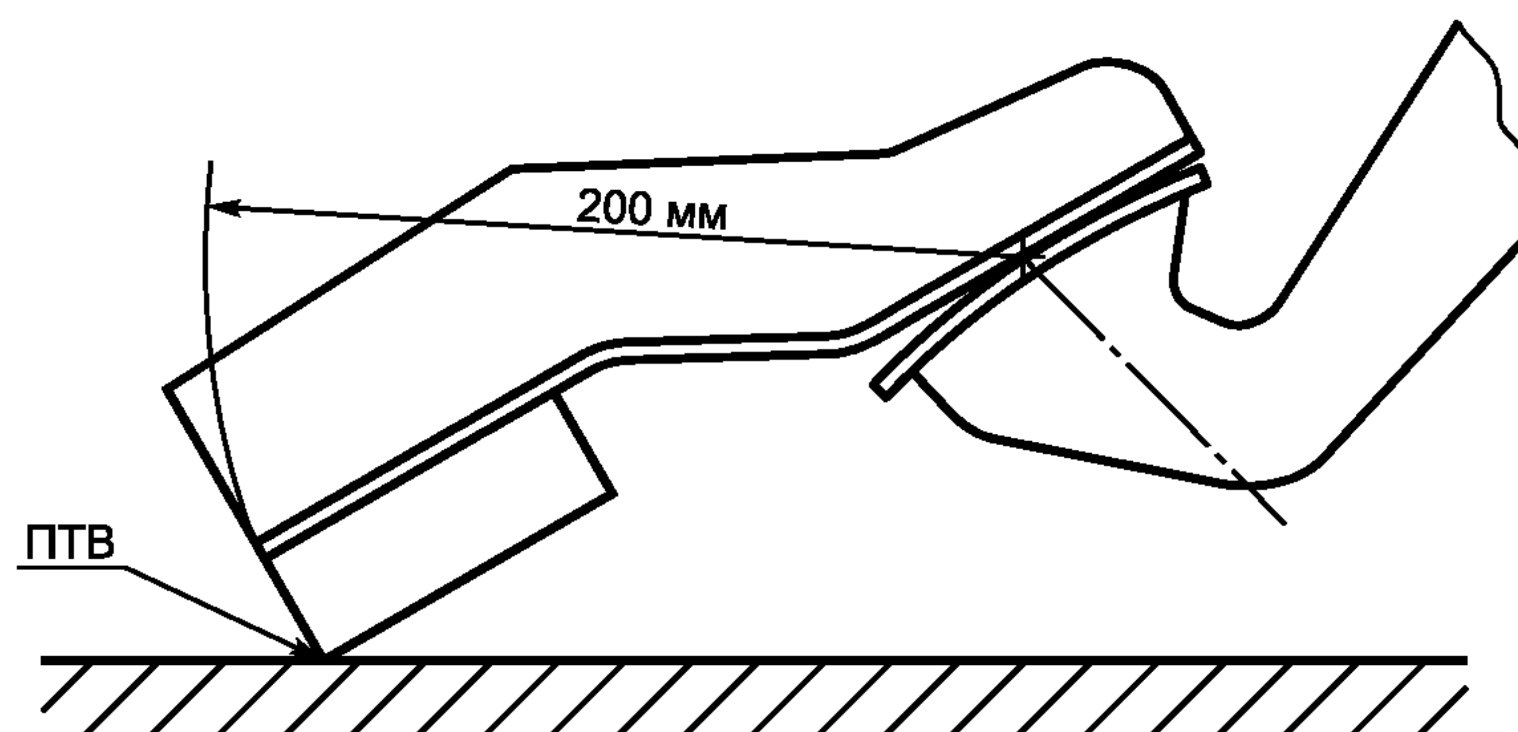
б) педаль подвесного (маятникового) типа
