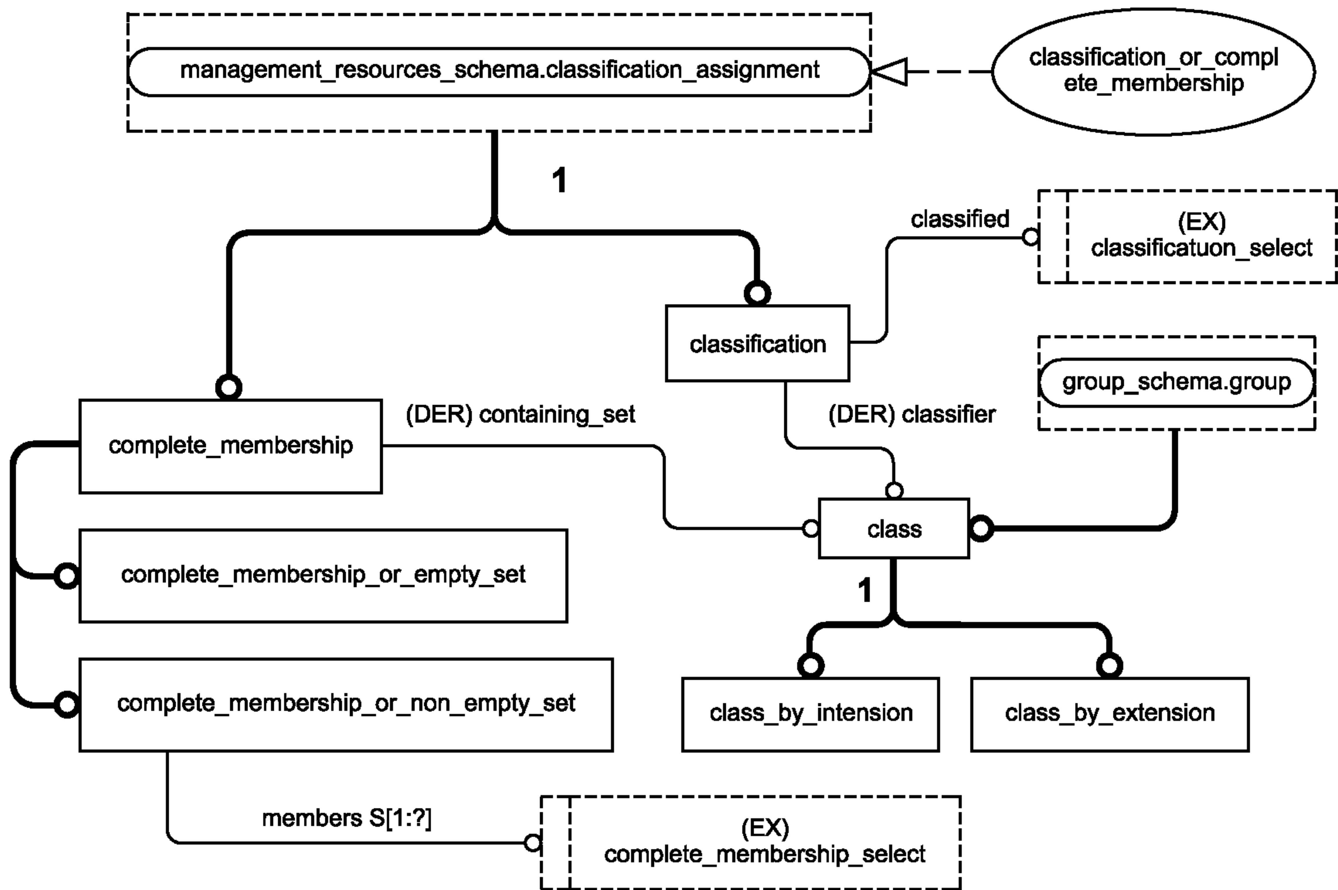
Рисунок D.1 — EXPRESS-G диаграмма схемы classification_schema
