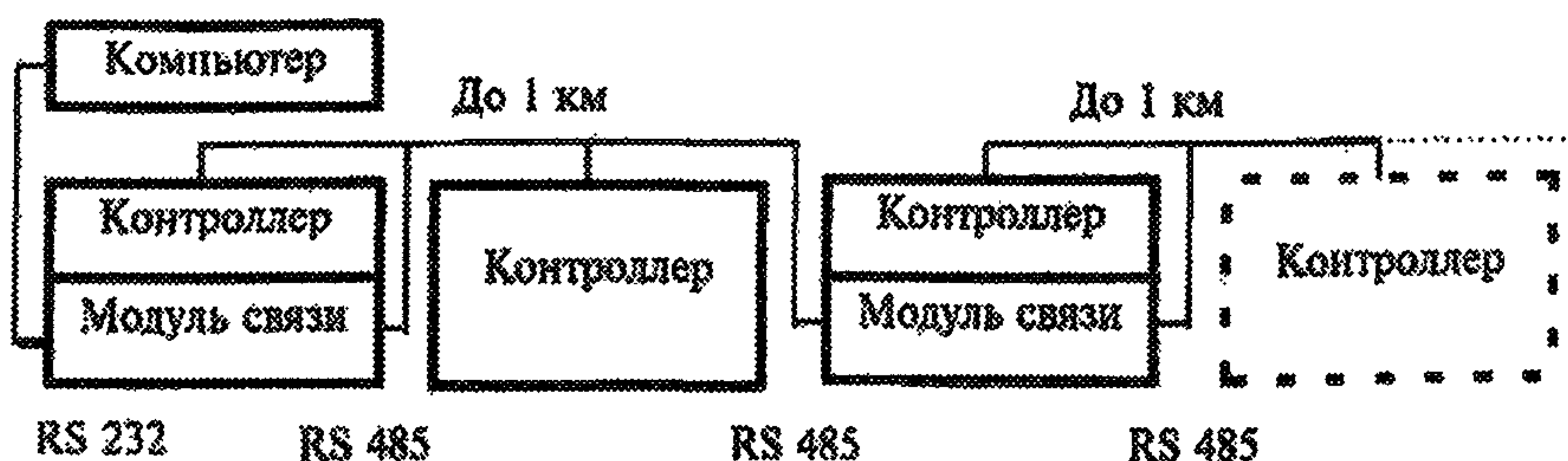
Рисунок 6 - Увеличение длины ветви при использовании двух модулей связи
