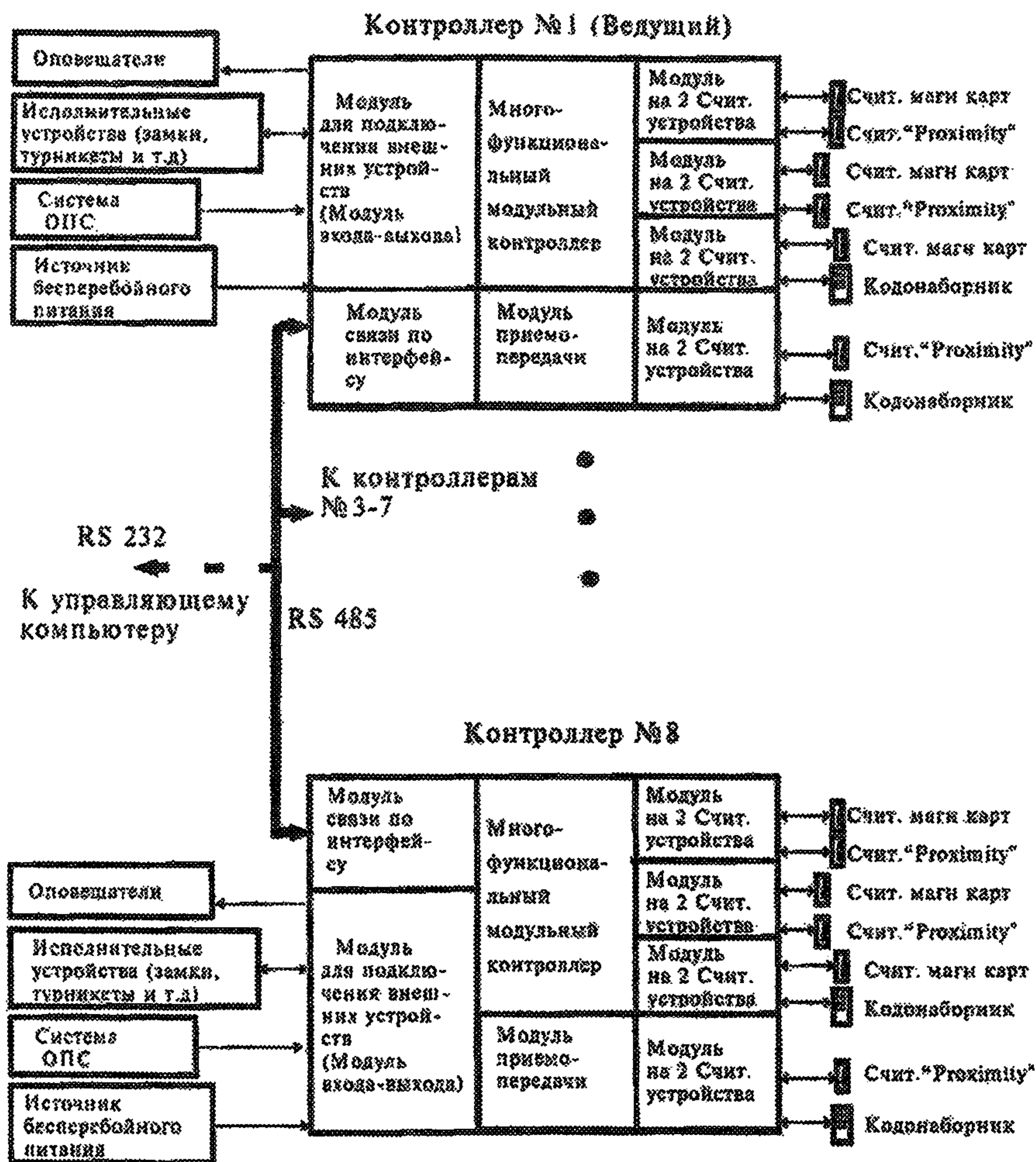
Рисунок 3 - Примерная структурная схема построения сетевой СКУД
