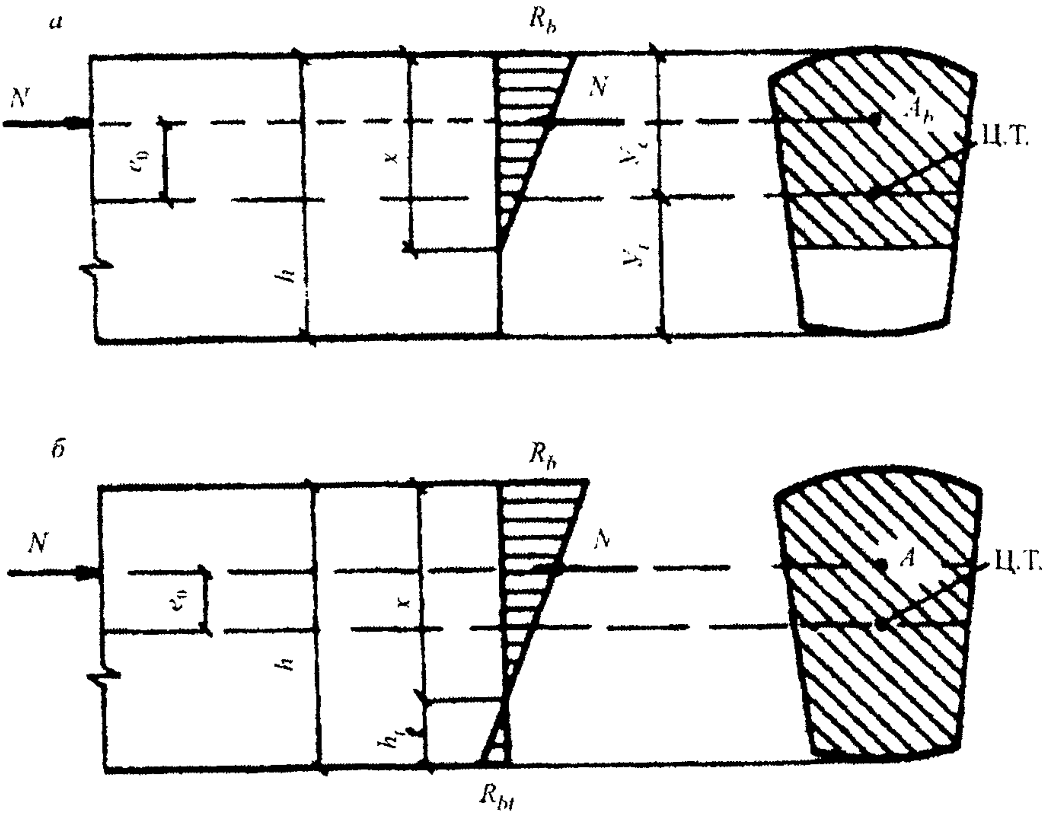
а – без учета сопротивления бетона растянутой зоны; б – с учетом сопротивления бетона растянутой зоны
