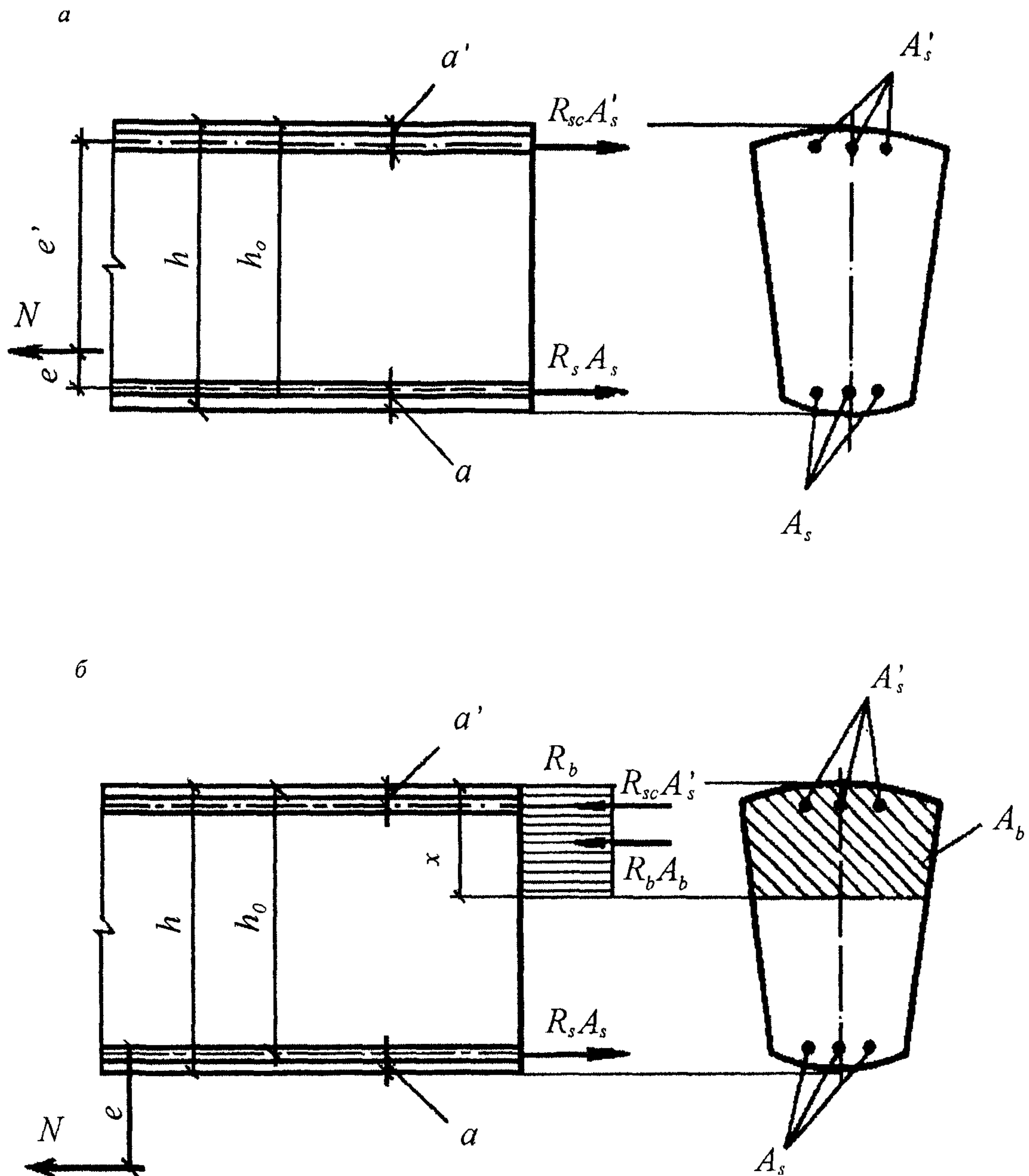
а – продольная сила N приложена между равнодействующими усилий в арматуре A_s и A_{s'} ; б – продольная сила N приложена за пределами расстояния между равнодействующими усилий в арматуре A'_s и A_{si}
