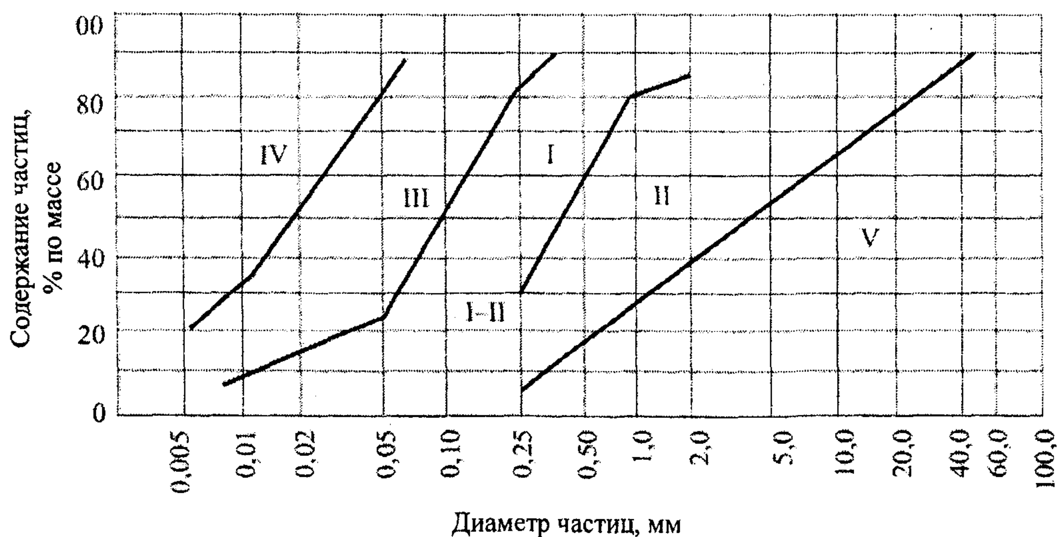
Рисунок 6 – Группы грунтов, используемых для намыва плотин
