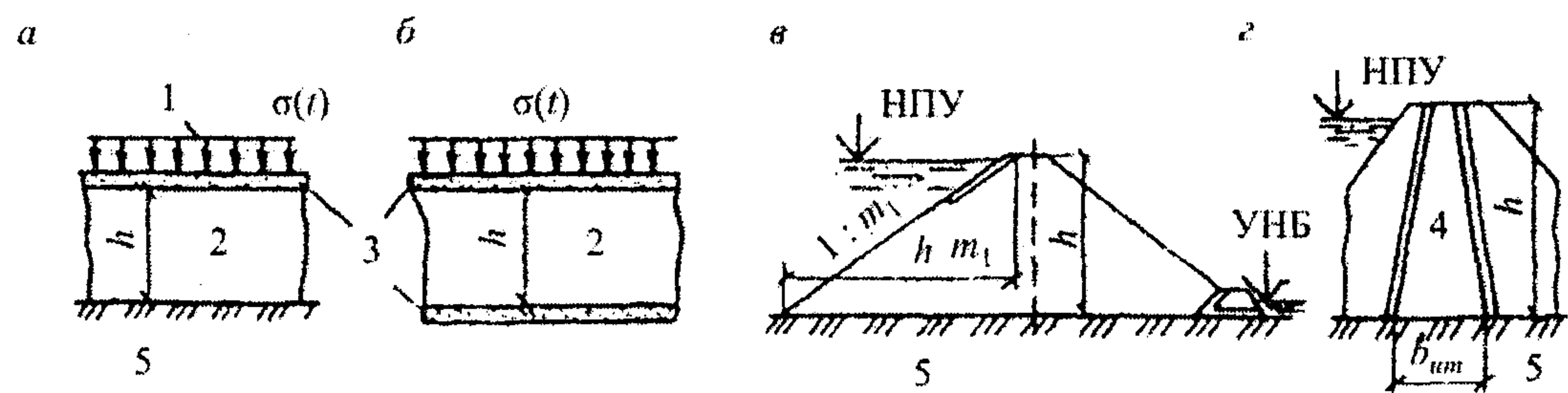
а – слой на водоупоре; б – слой на дренаже; в – однородная плотина; г – ядро каменно-земляной плотины
