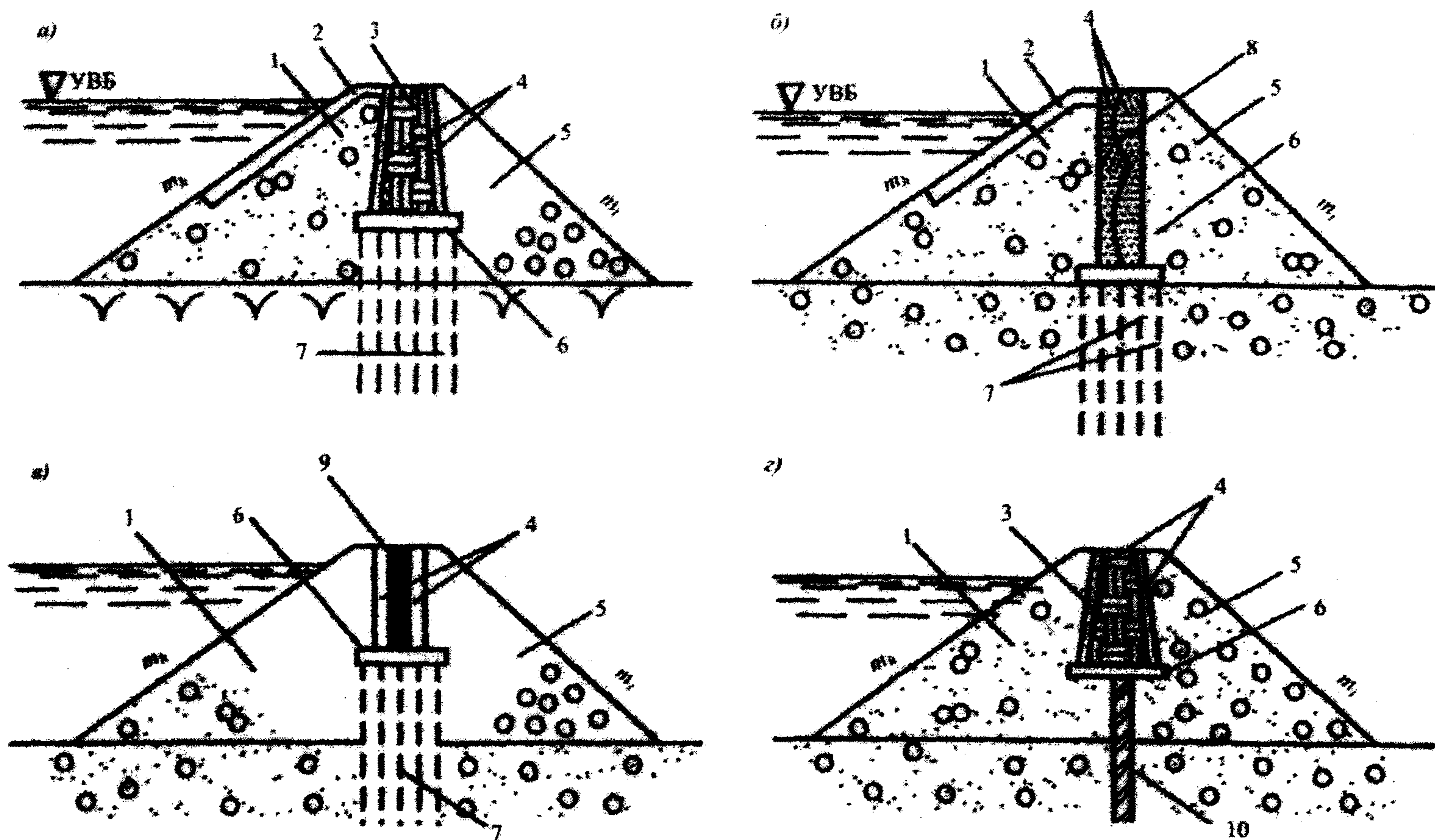
1 - верховая призма; 2 - крепление верхового откоса; 3 - грунтовое ядро; 4 - переходные слои (обратные фильтры); 5 - низовая призма; 6 - сопрягающий элемент; 7 - инъекционная завеса; 8 - пленочная диафрагма; 9 - асфальтобетонная диафрагма («стена в грунте»); 10 - «стена в грунте» m_h — коэффициент верхового откоса; m_n — коэффициент низового откоса.
