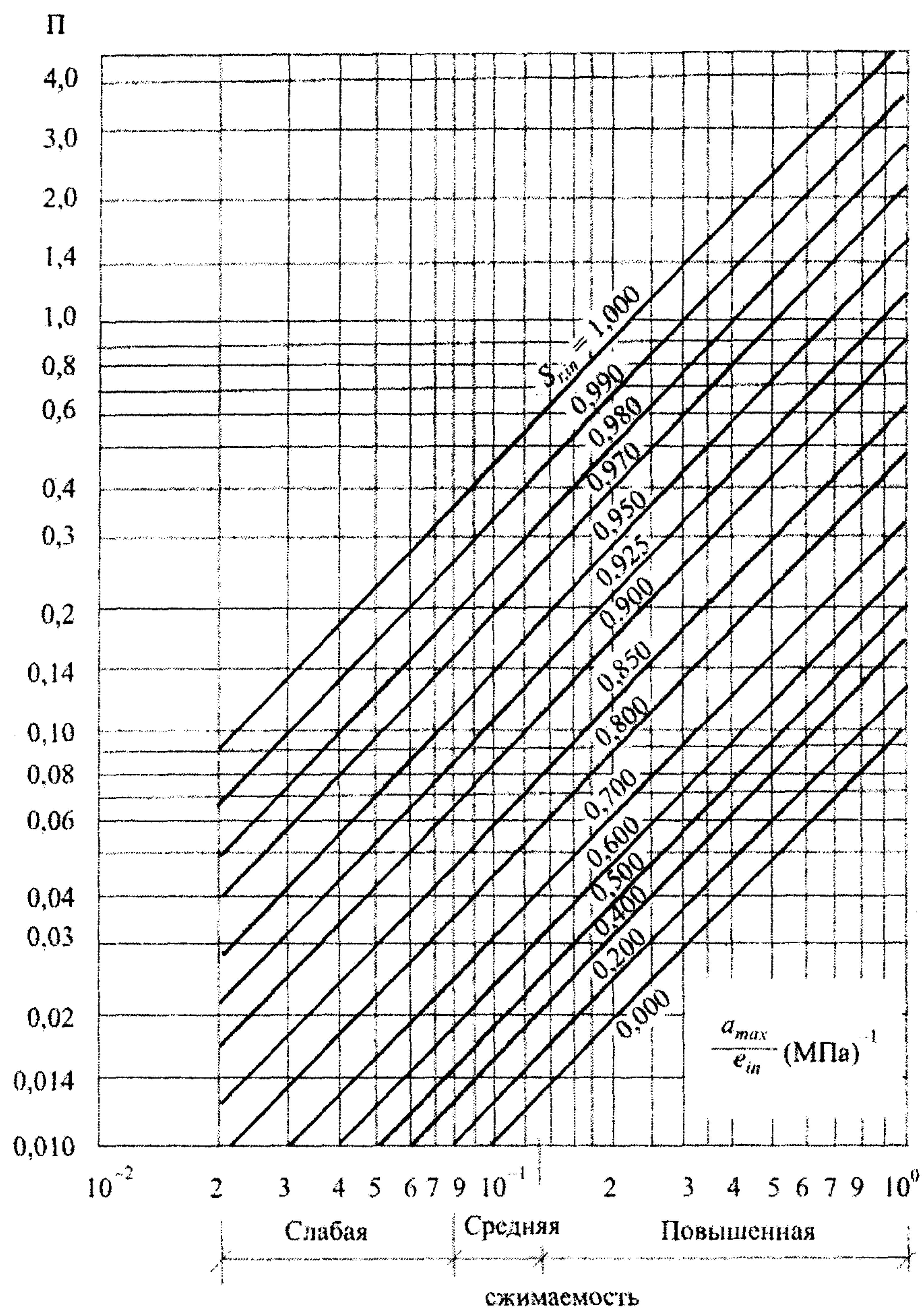
Рисунок А.2 – Номограмма для определения параметра \Pi
