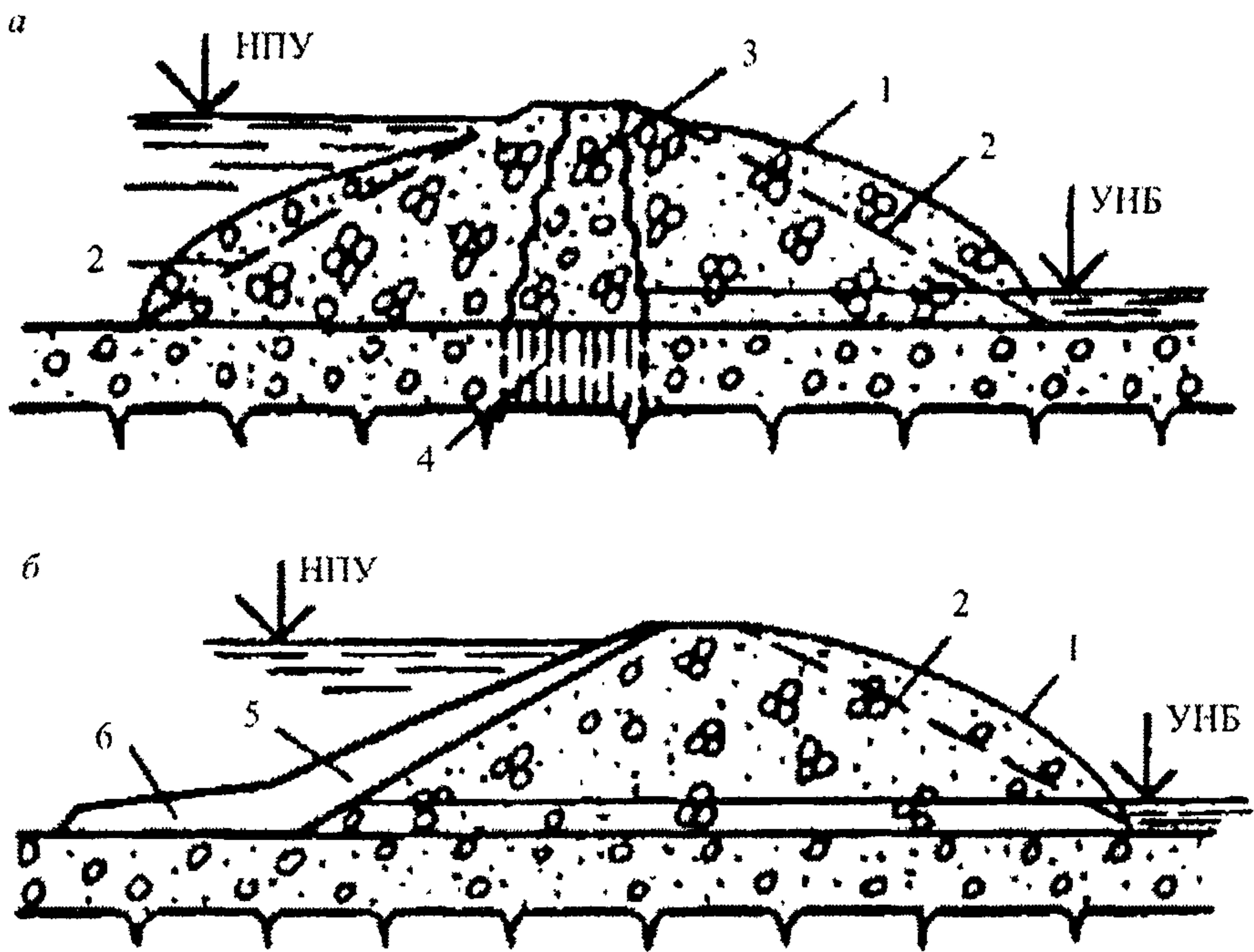
а, б – см. таблицу 7; 1 – контур навала; 2 – контур расчетного профиля; 3 – инъекционное ядро; 4 – инъекционная завеса; 5 – экран; 6 – понур
