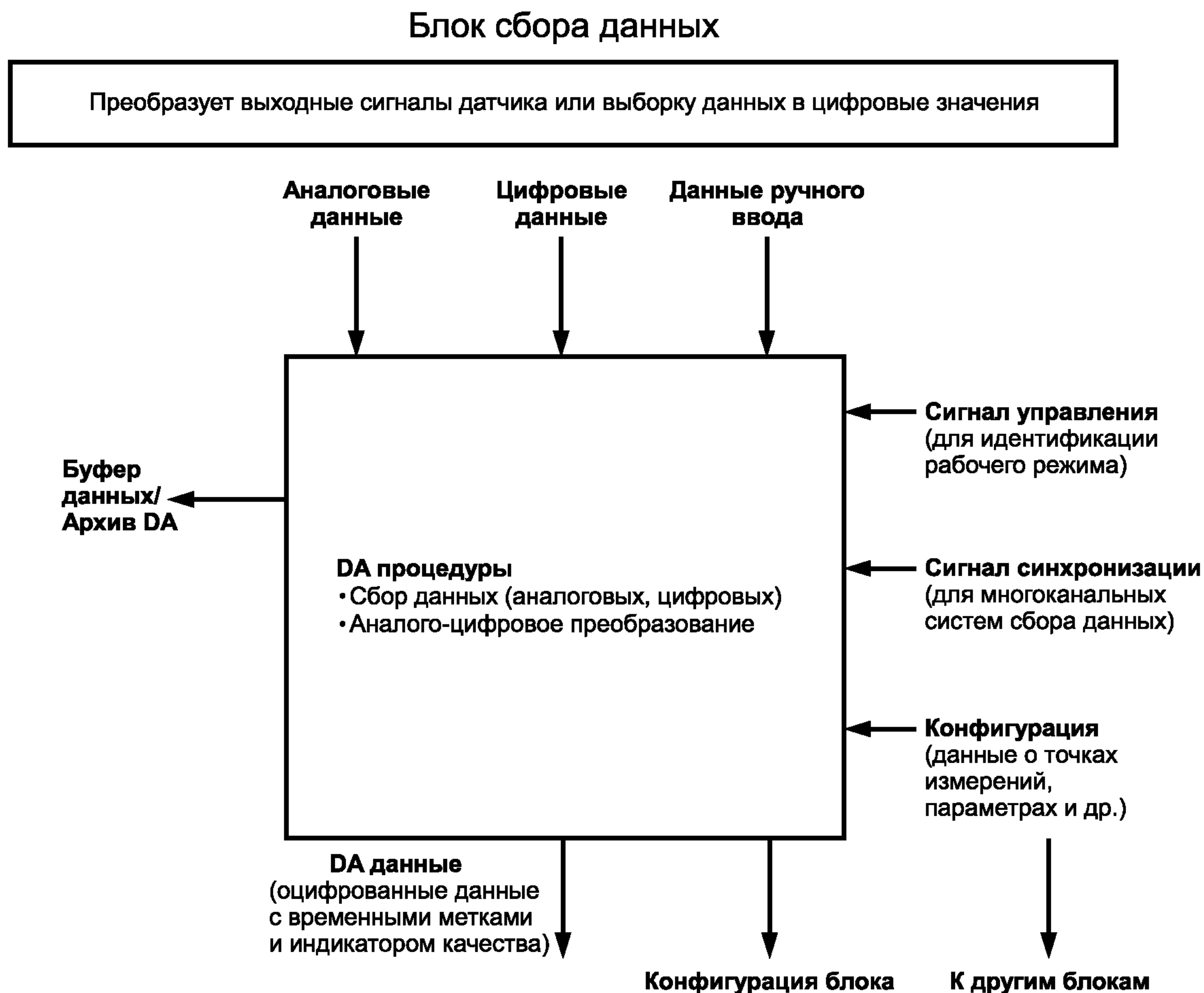
Рисунок 3 — Блок сбора данных
