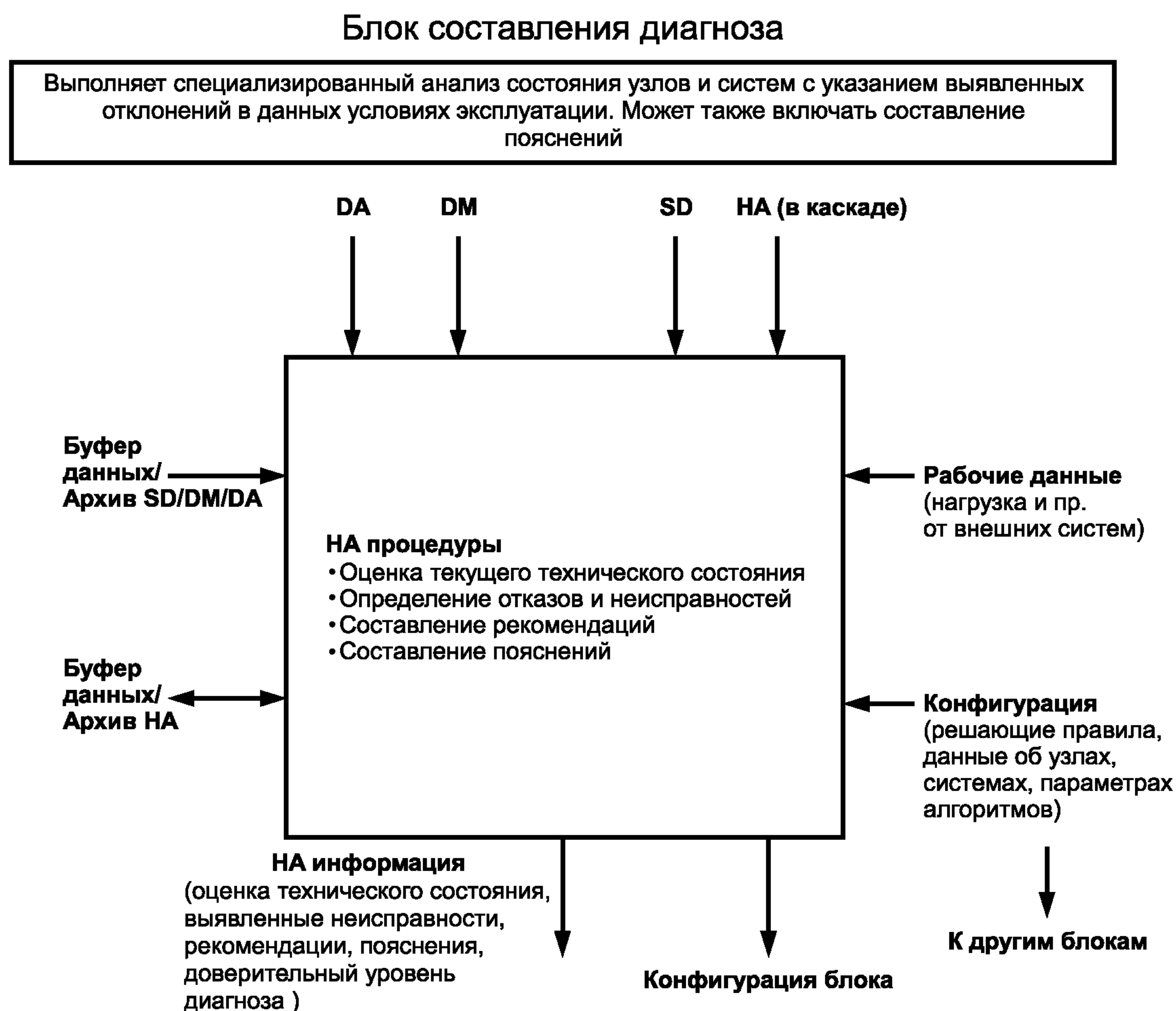
Рисунок 6 — Блок составления диагноза
