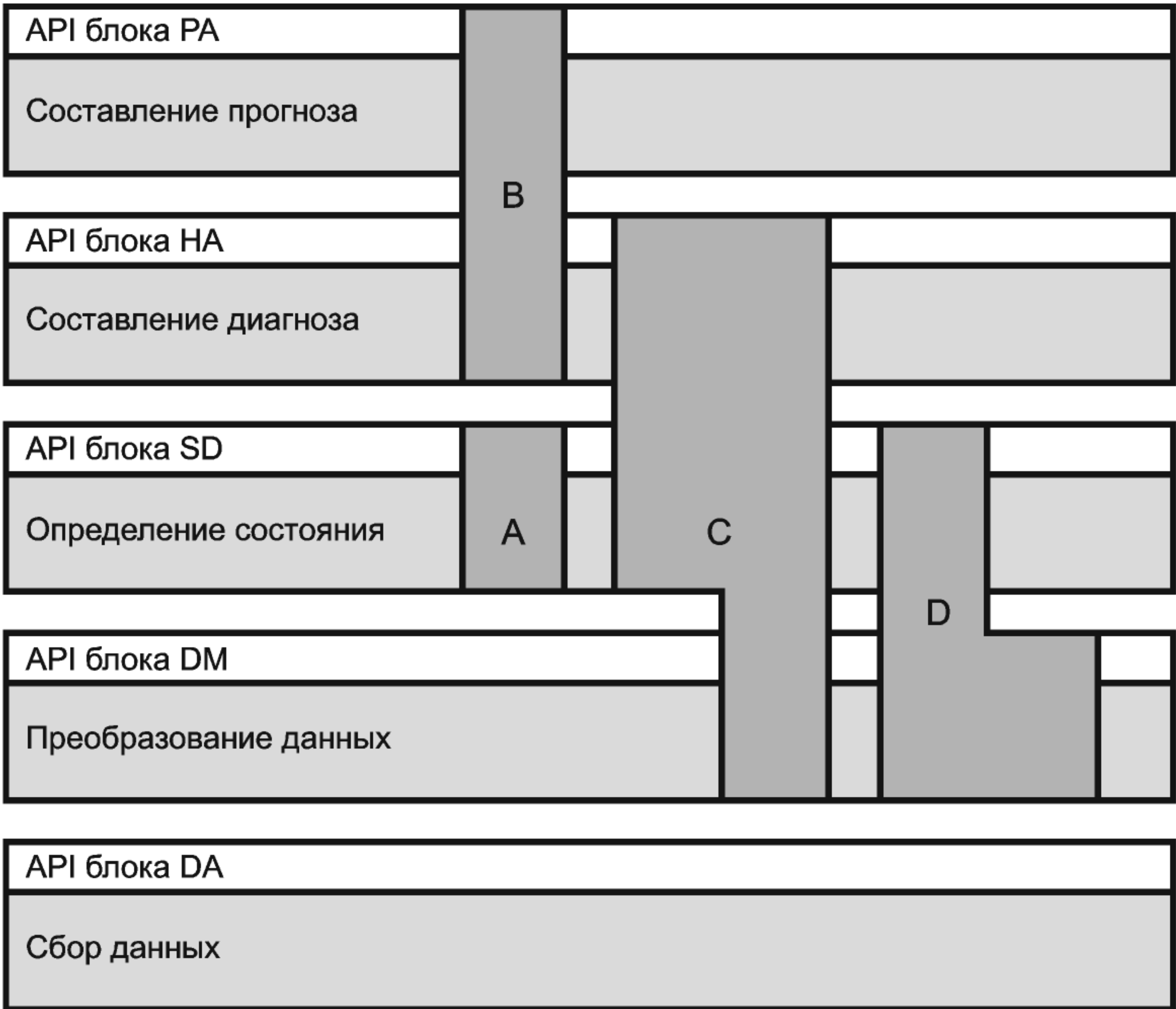
Рисунок 10 — Пример объединения в модуле функций нескольких блоков
