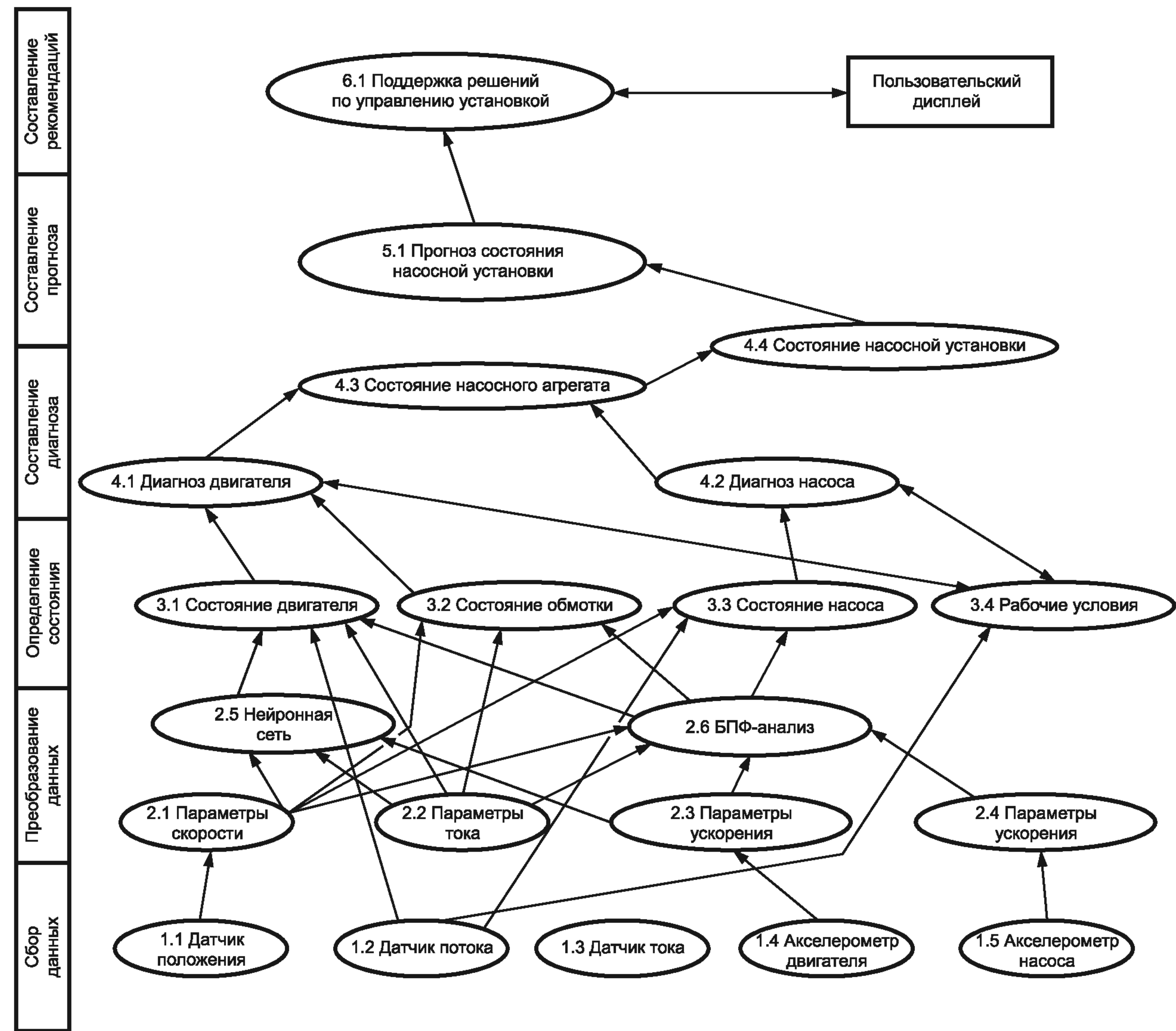
Рисунок 11 — Пример совместимой модульной системы
