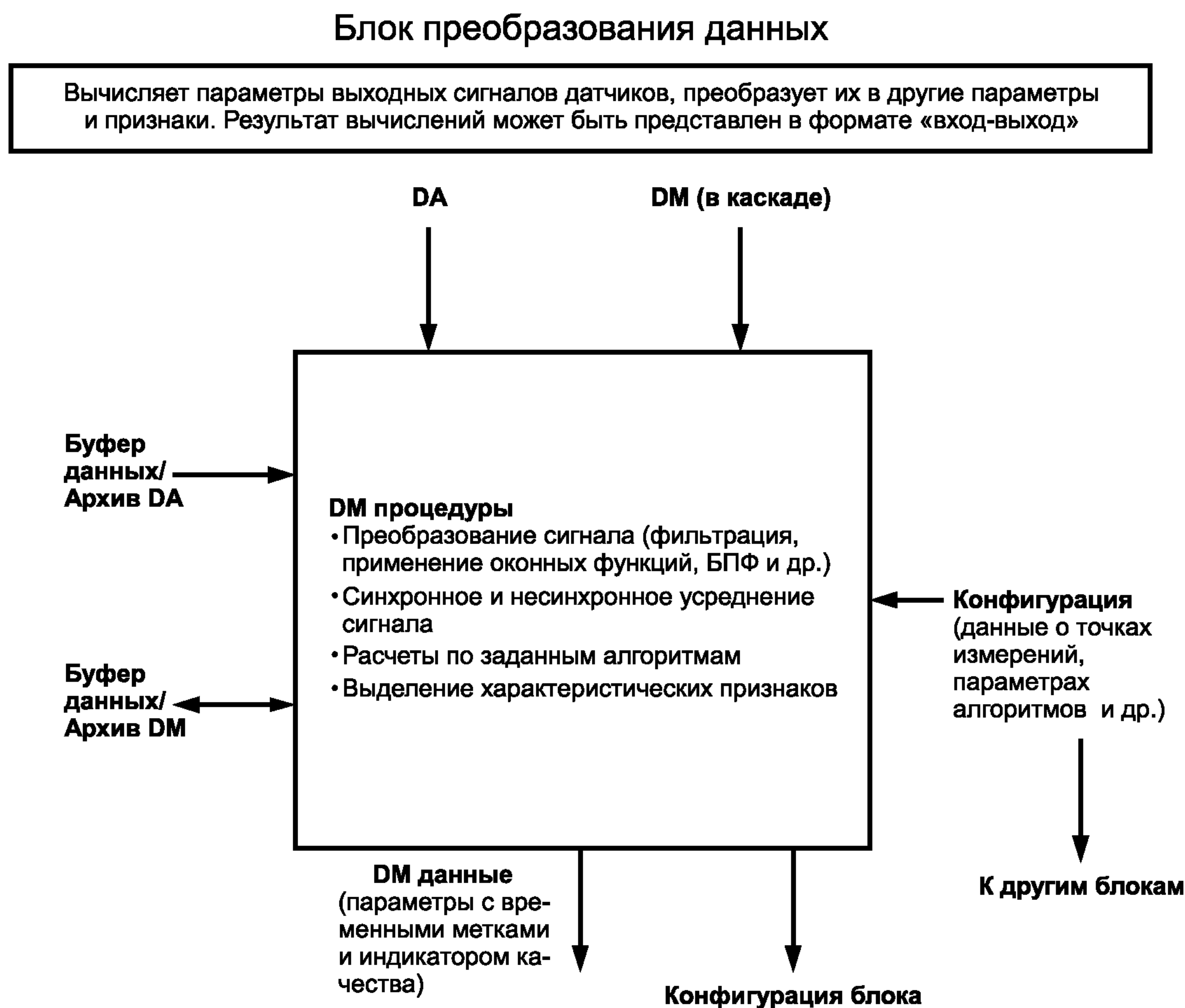
Рисунок 4 — Блок преобразования данных
