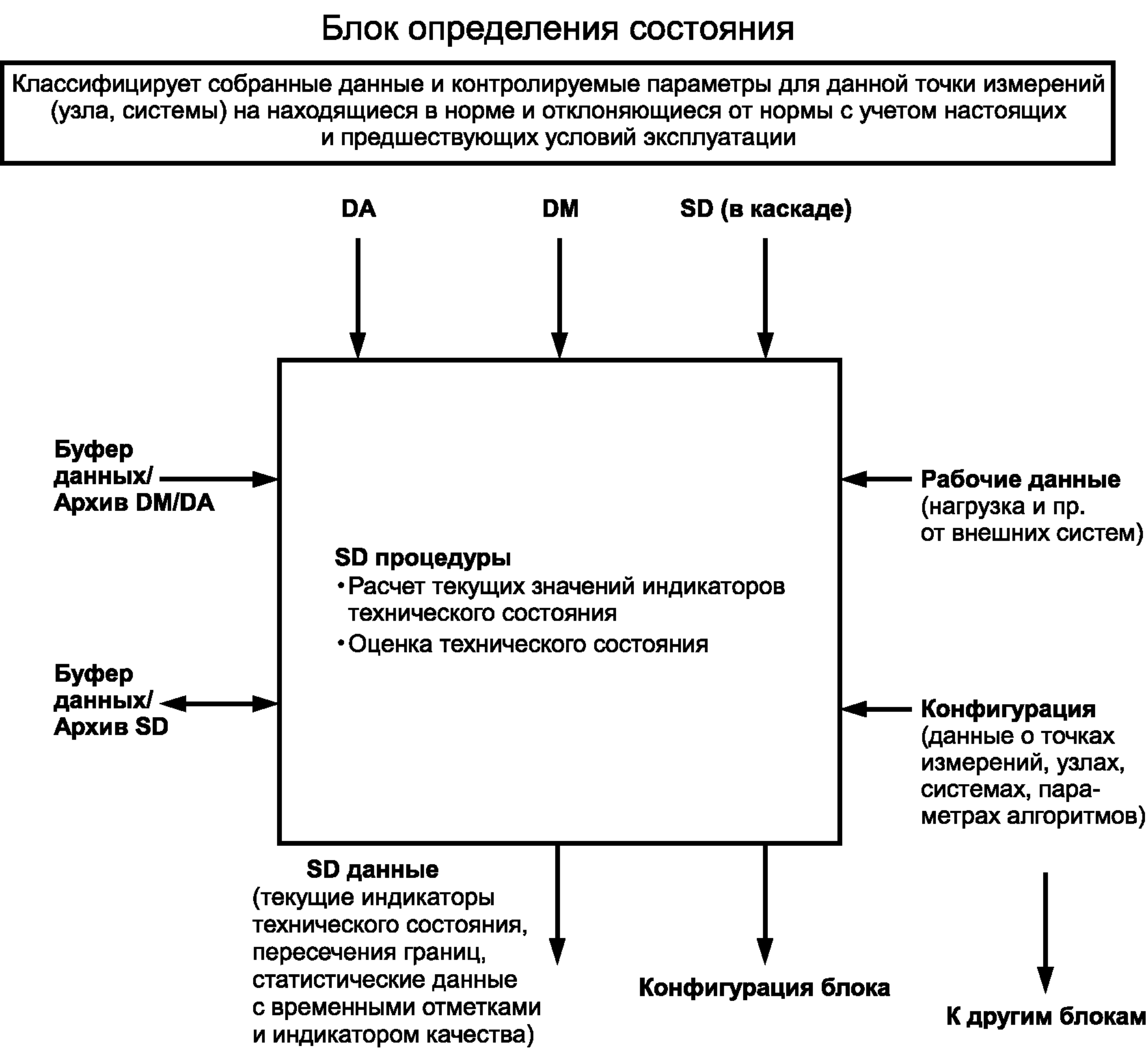
Рисунок 5 — Блок определения состояния
