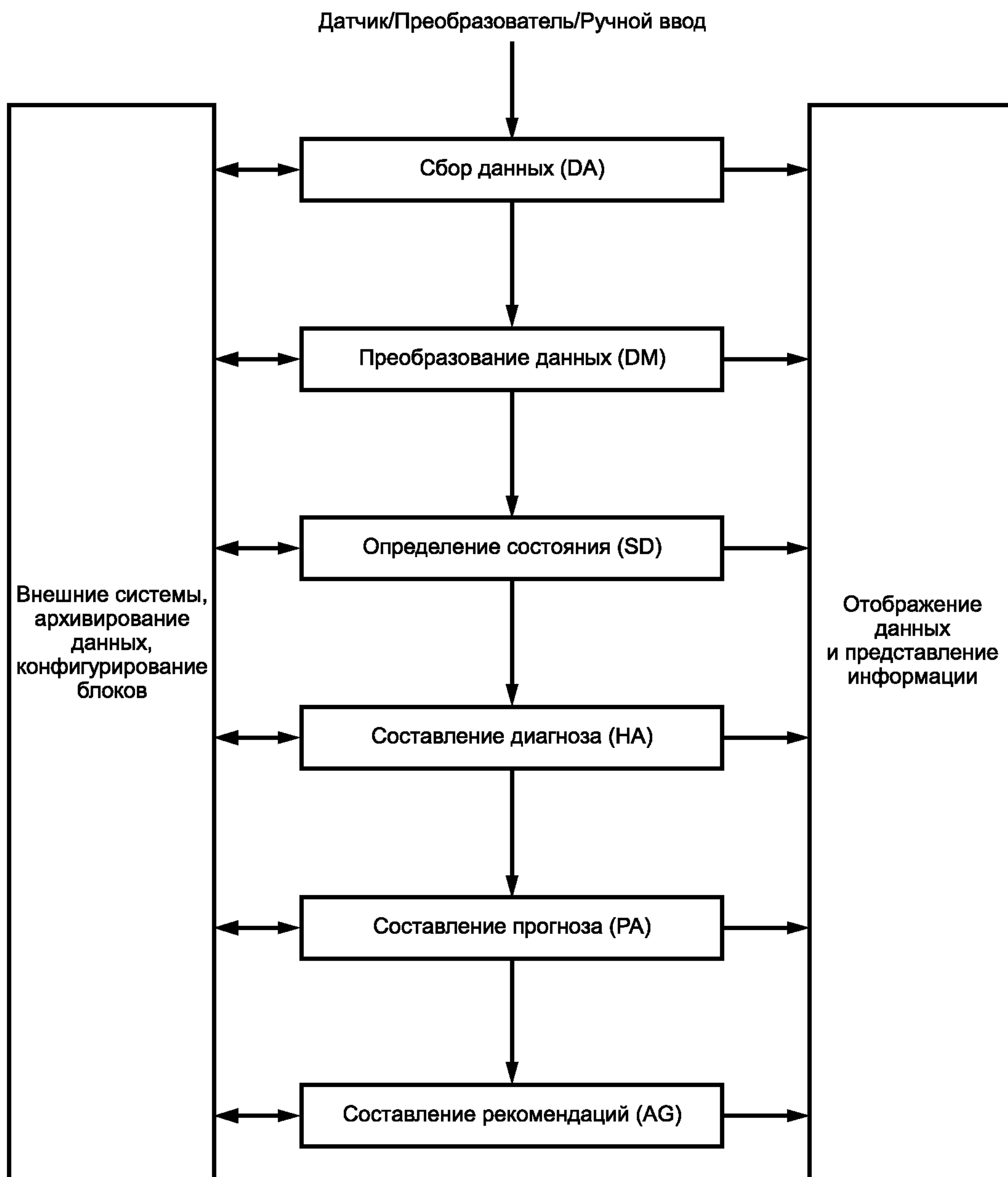
Рисунок 2 — Блок-схема этапов обработки данных
