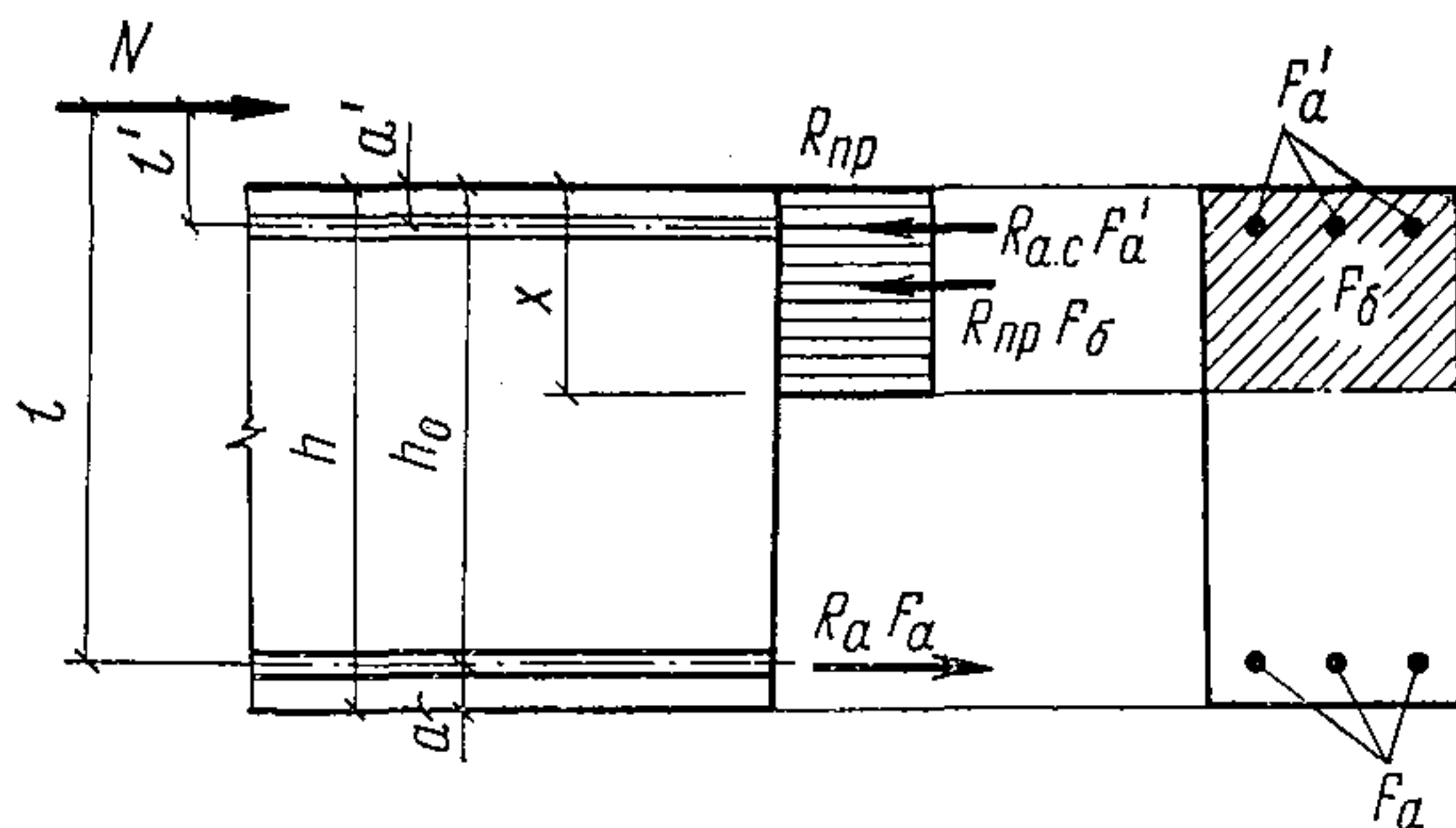
Рис. 5. Схема усилий и эпюра напряжений в сечении, нормальном к продольной оси внецентренно сжатого элемента, при расчете его по прочности.
