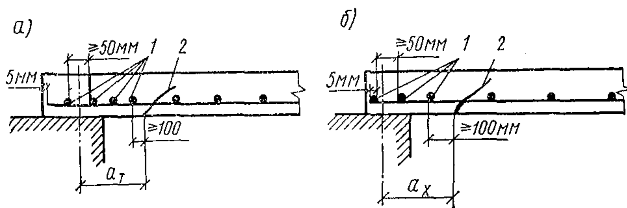
Рис. 13. Примеры анкеровки растянутых стержней арматуры на опорах плит из ячеистого бетона
