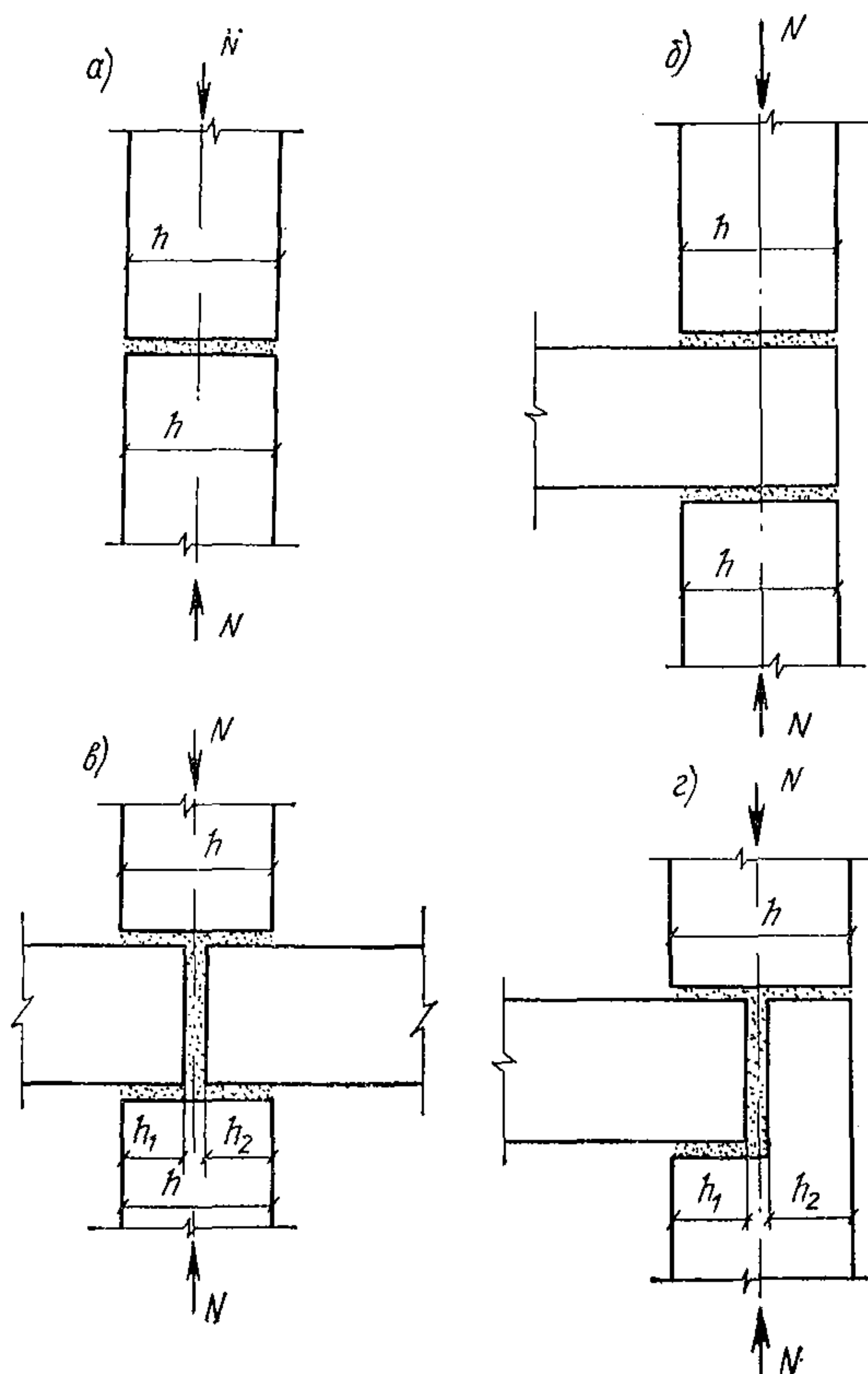
Рис. 14. Опорные сечения стен из панелей (блоков)
