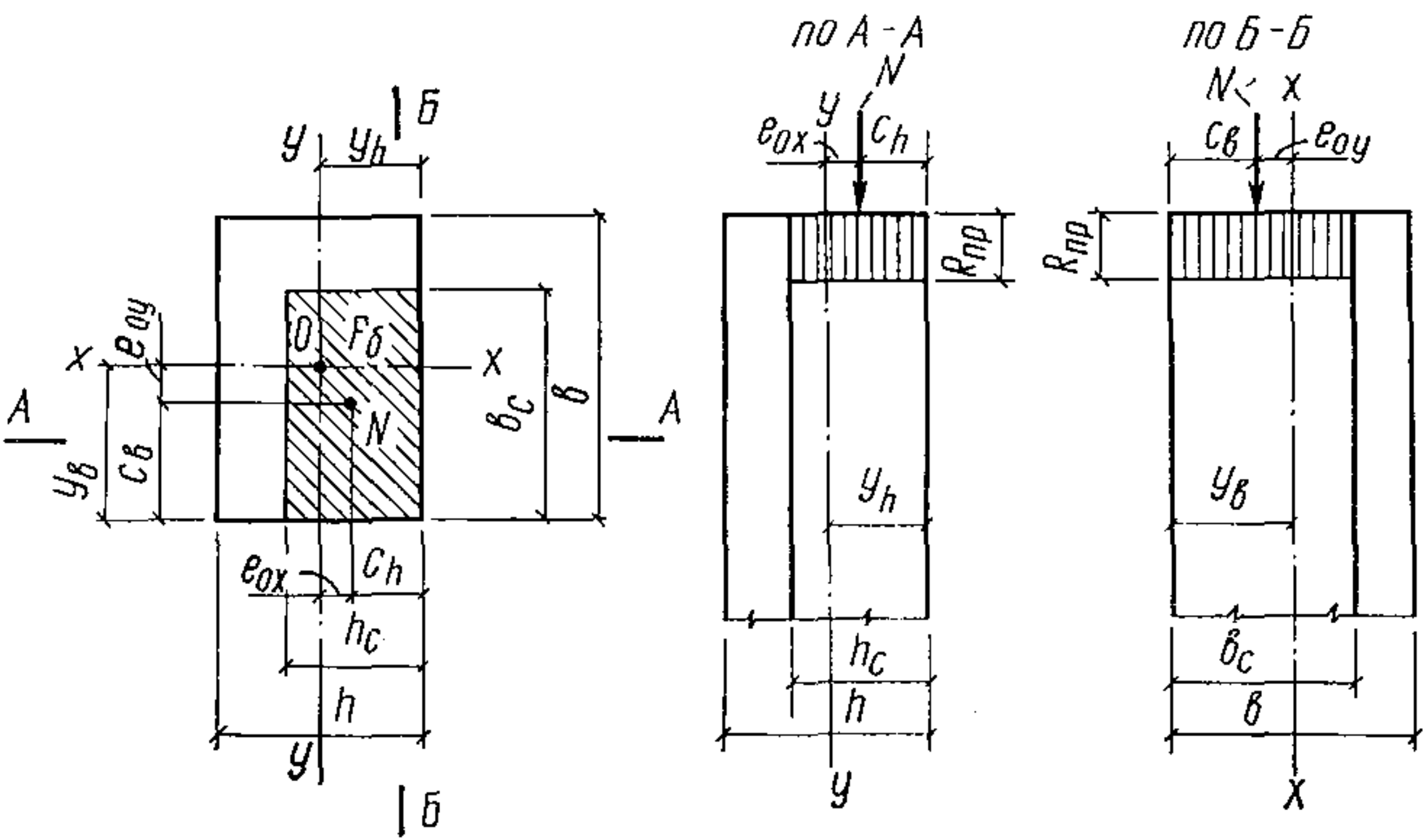
Рис. 2. Схема расположения усилий и эпюра напряжений в поперечном сечении бетонного элемента при косом внецентренном сжатии.
