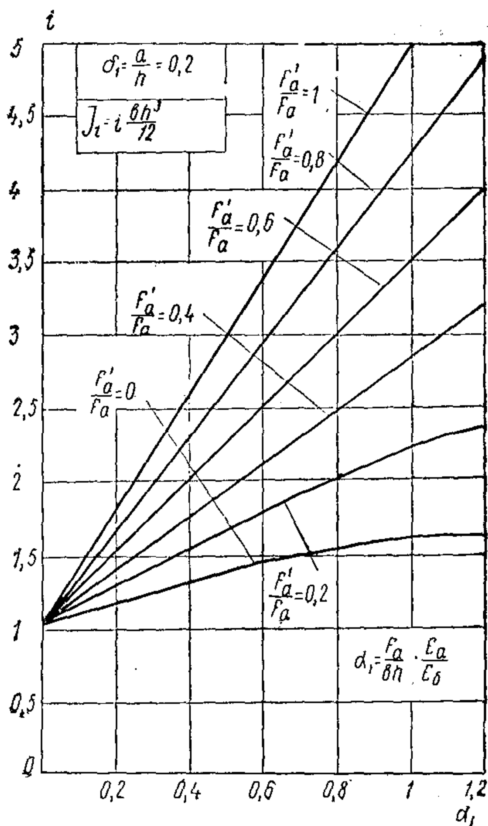
Рис. 18. График значений коэффициента i для вычисления приведенного момента инерции J_{пр} и расчета жесткости изгибаемых элементов прямоугольного сечения при \delta_1 = 0,2
