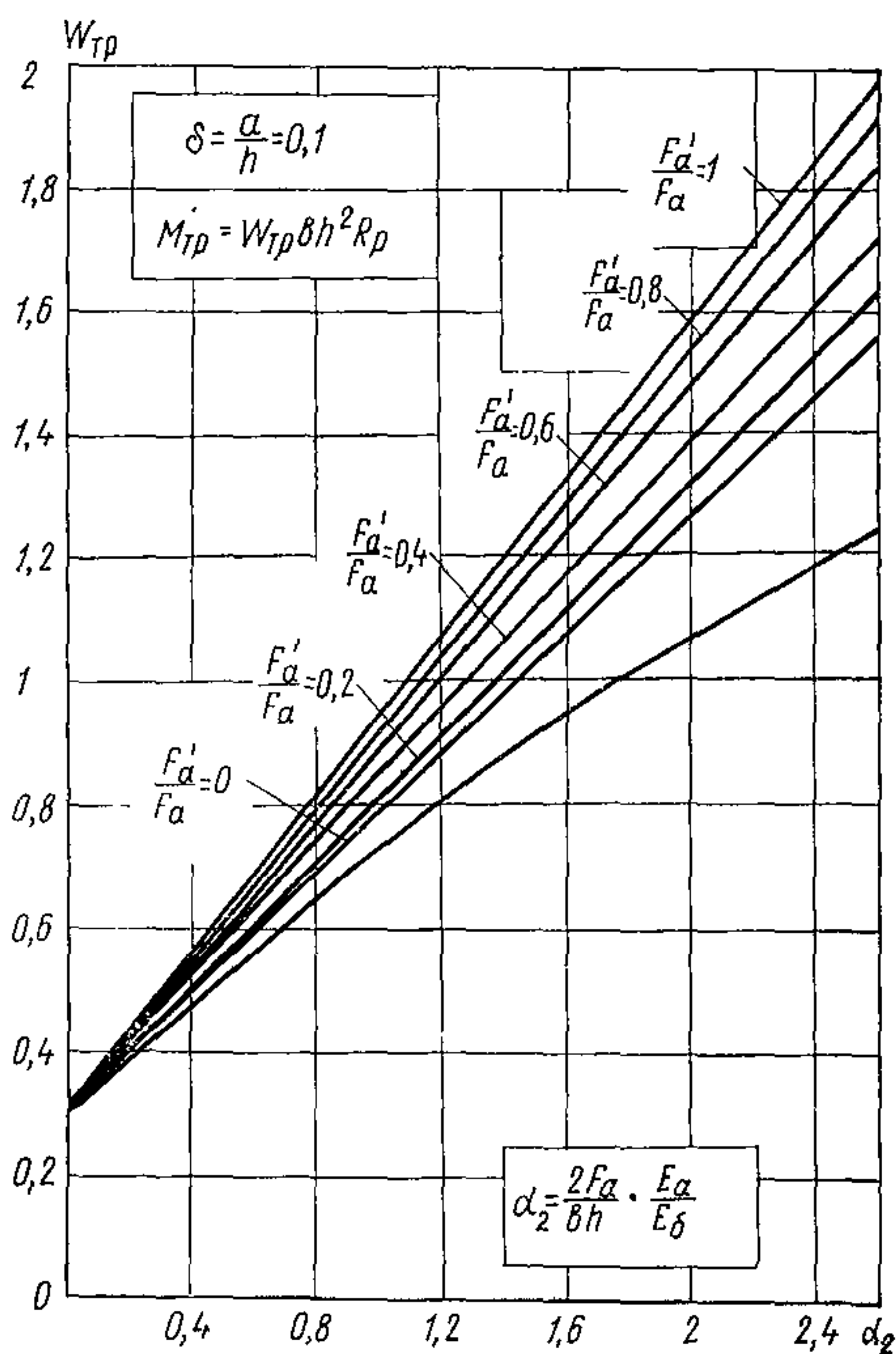
Рис. 15. График значений коэффициента W_{тр} для определения момента появления трещин в изгибаемых элементах прямоугольного сечения при \delta_1=0,1
