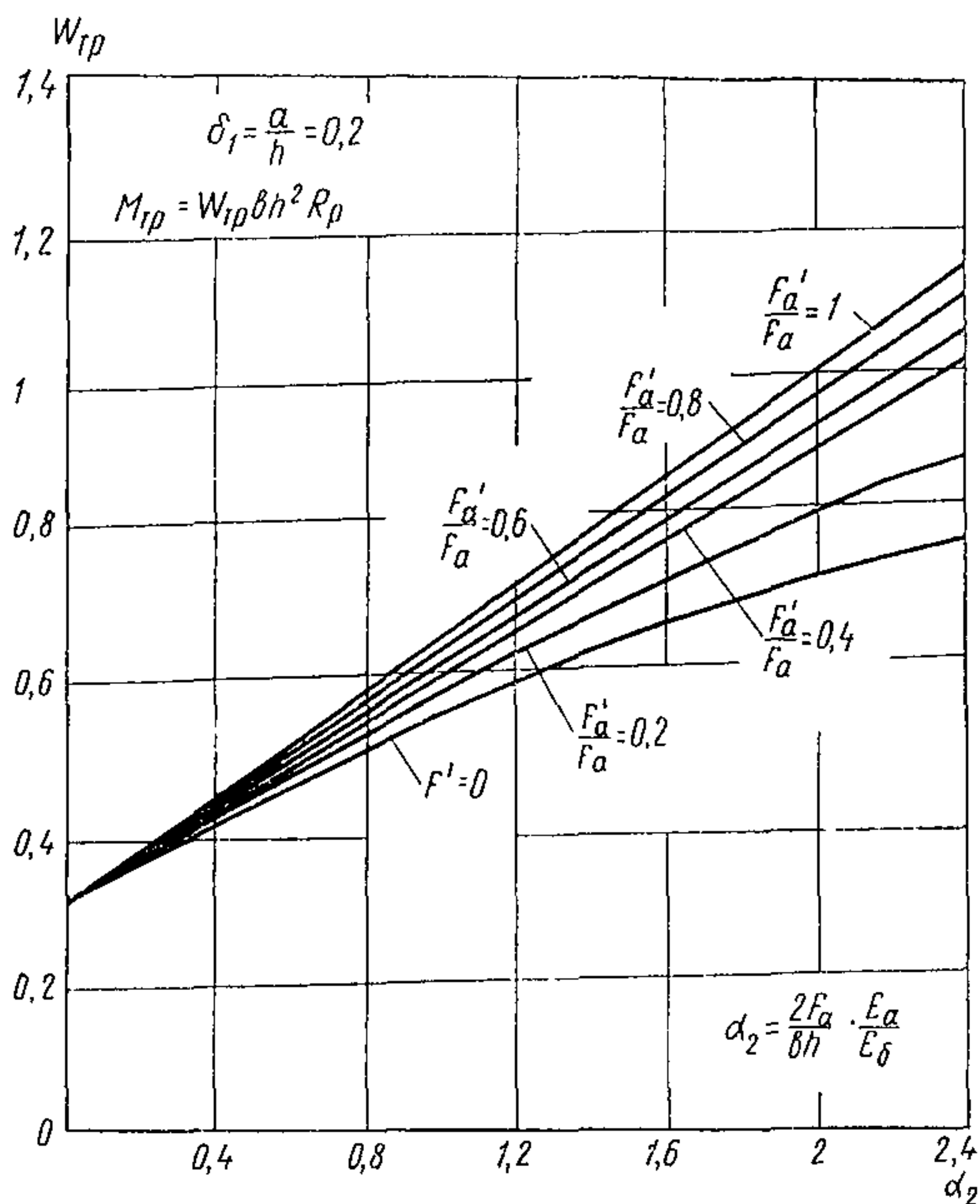
Рис. 16. График значений коэффициента W_{тр} для определения момента появления трещин в изгибаемых элементах прямоугольного сечения при \delta_1 = 0,2
