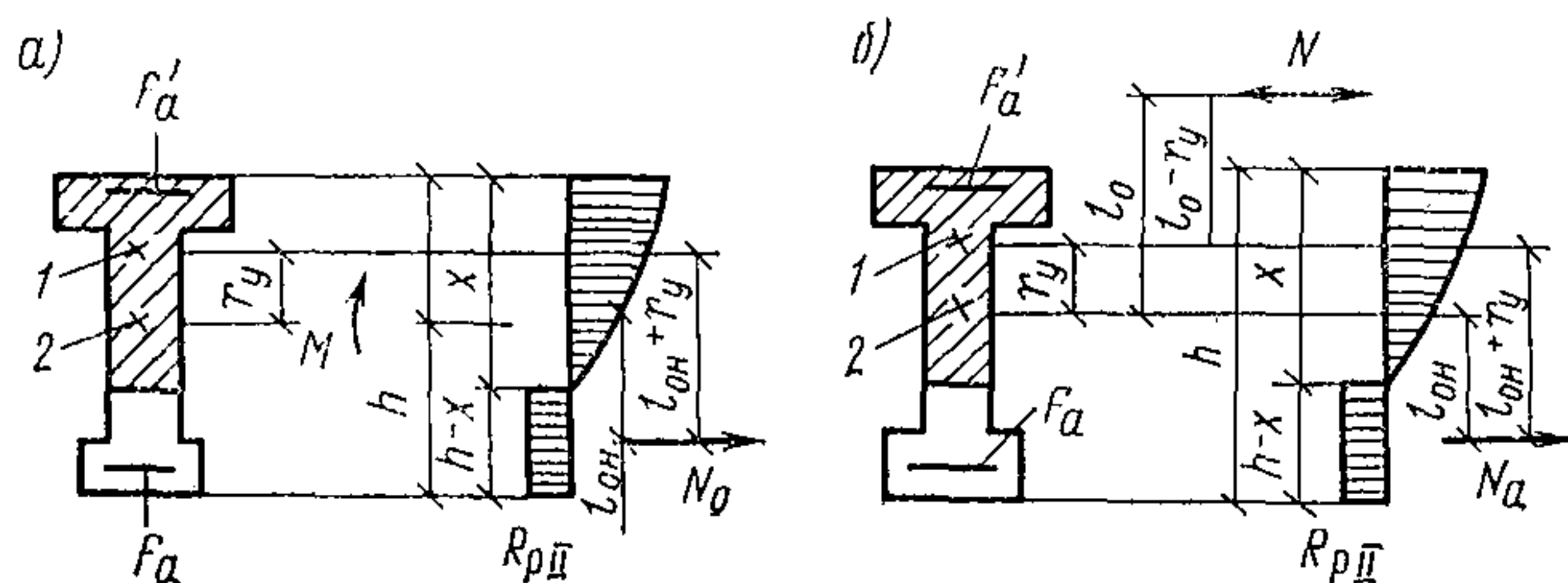
Рис. 11. Схемы усилий и эпюра напряжений в поперечном сечении элемента при расчете его по образованию трещин, нормальных к продольной оси элемента, в зоне сечения, растянутой от действия внешних нагрузок
