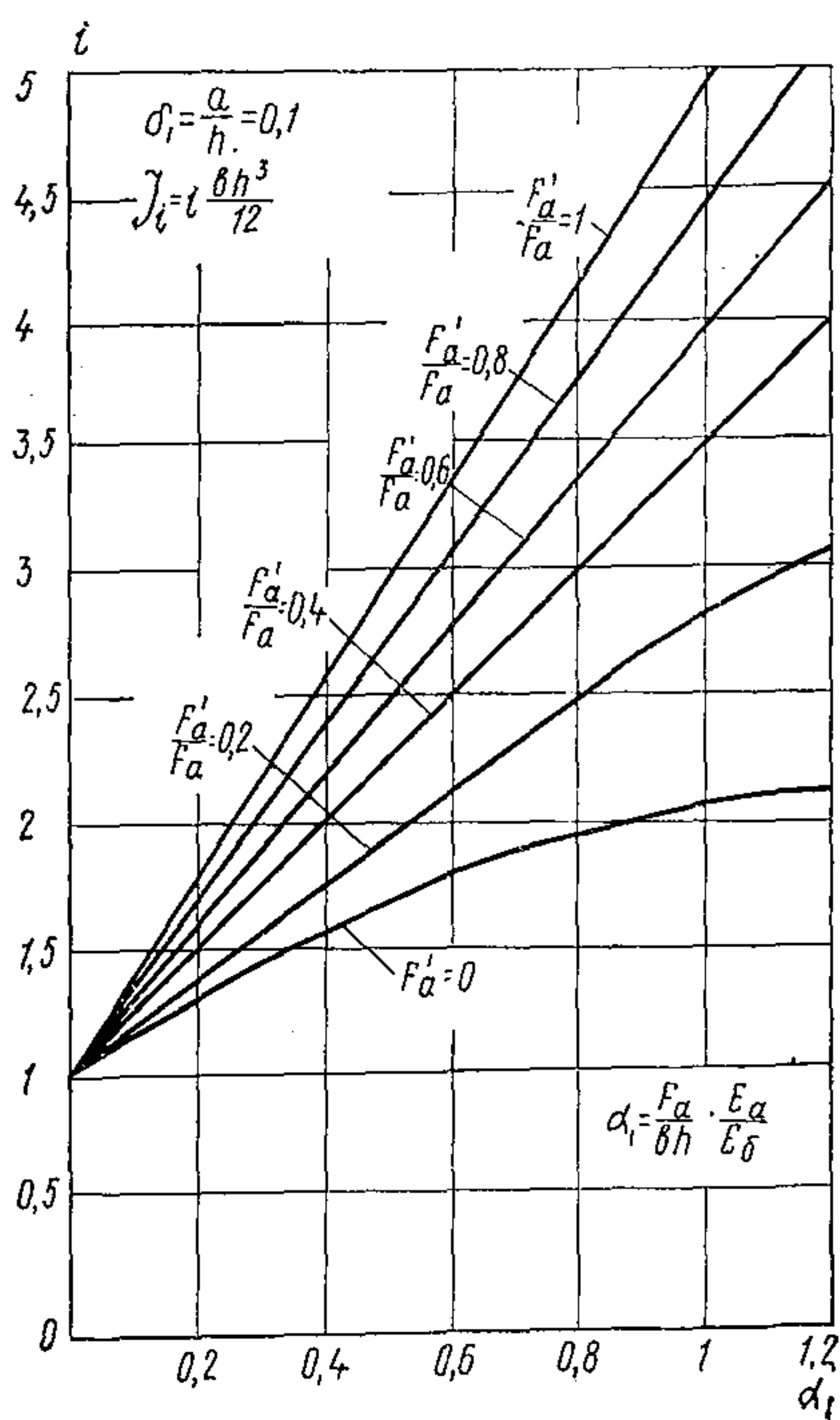
Рис. 17. График значений коэффициента i для вычисления приведенного момента инерции J_{\text{пр}} и расчета жесткости изгибаемых элементов прямоугольного сечения при \delta_1 = 0,1
