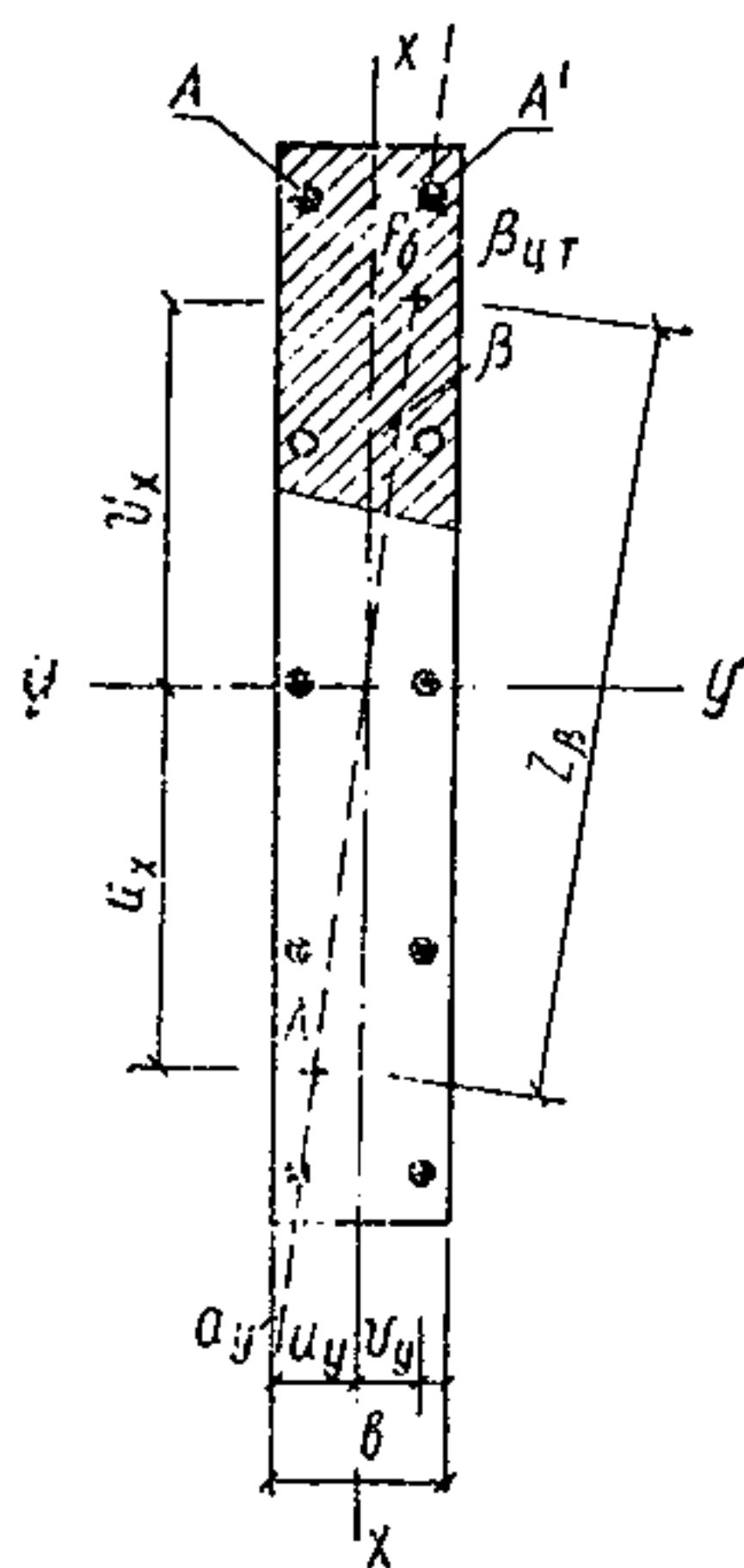
Рис. 9. Поперечное сечение железобетонного элемента, работающего на кривой изгиб
