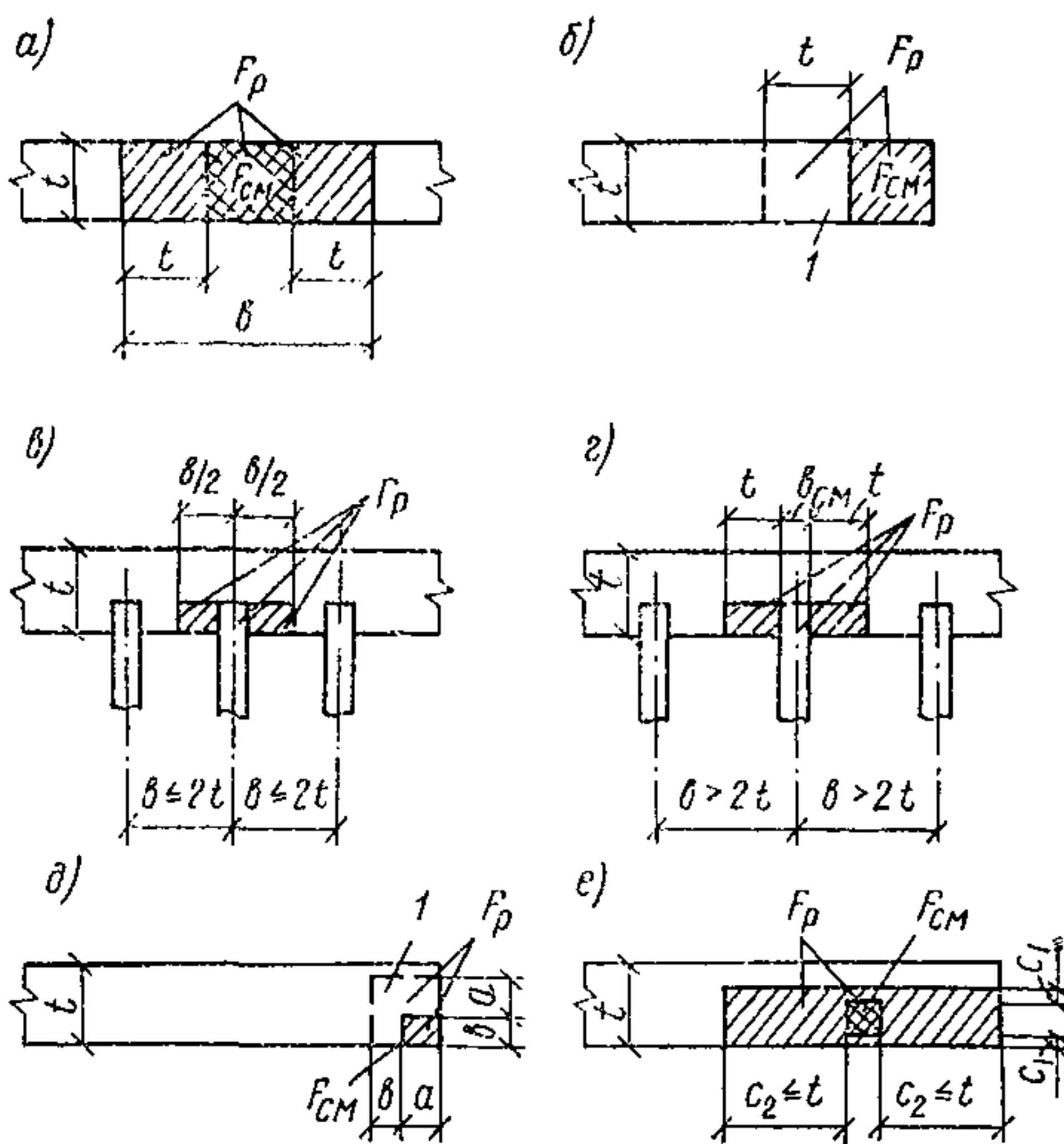
Рис. 10. Определение расчетной площади F_p при расчете на местное сжатие
