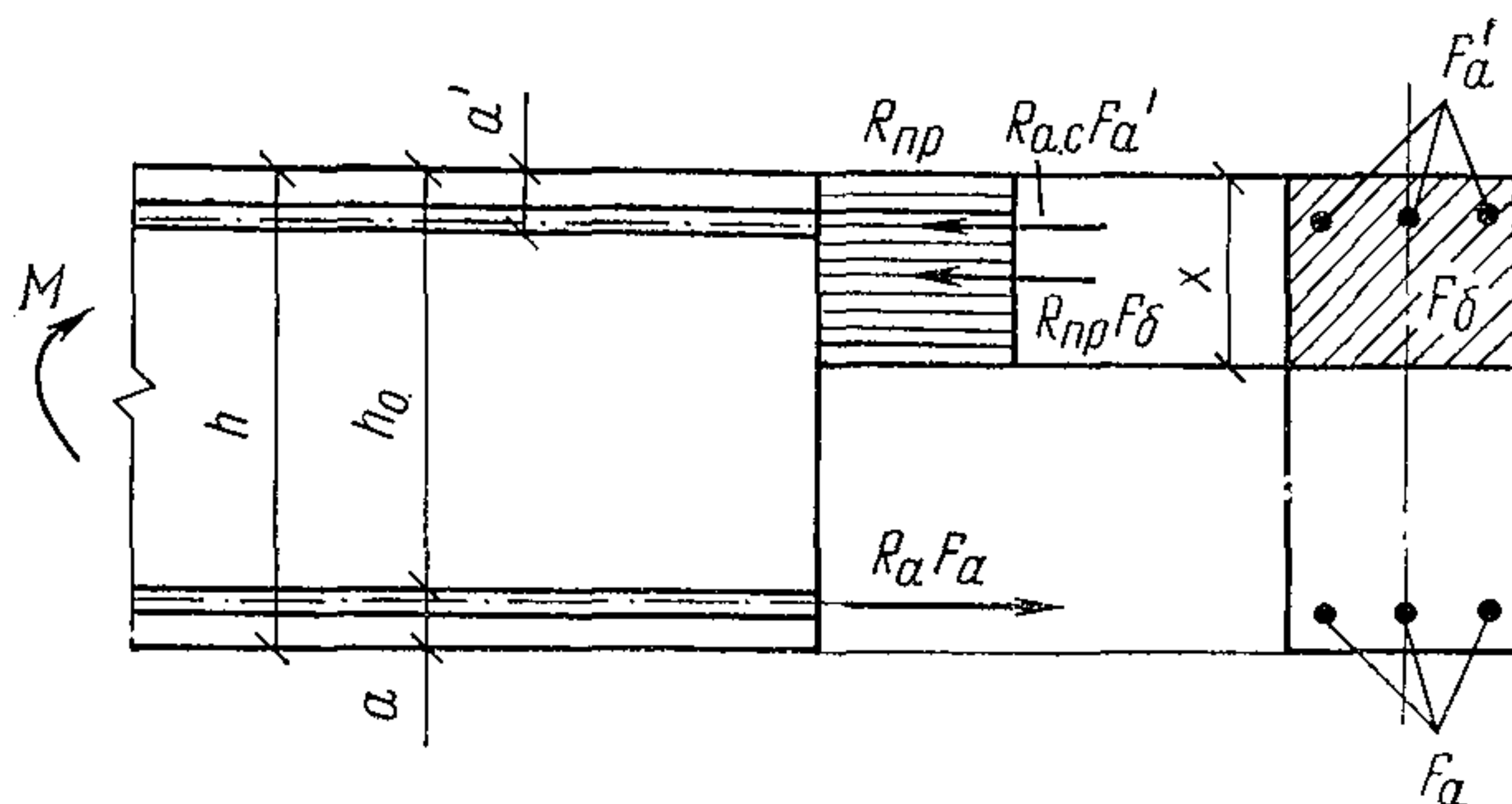
Рис. 3. Схема усилий и эпюра напряжений в сечении, нормальном к продольной оси изгибаемого железобетонного элемента, при расчете его по прочности
