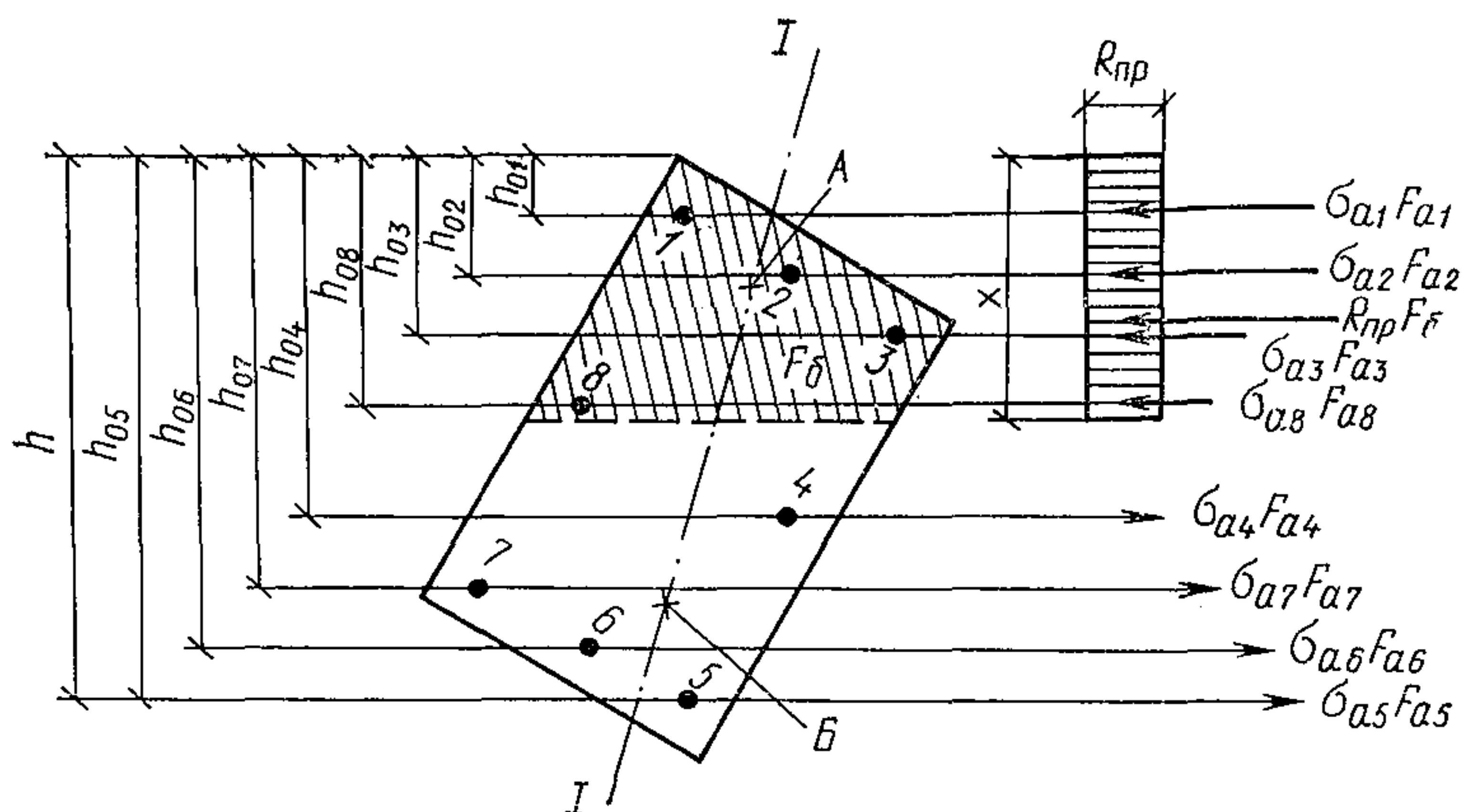
Рис. 6. Схема усилий и эпюра напряжений в сечении, нормальном к продольной оси железобетонного элемента, в общем случае расчета по прочности
