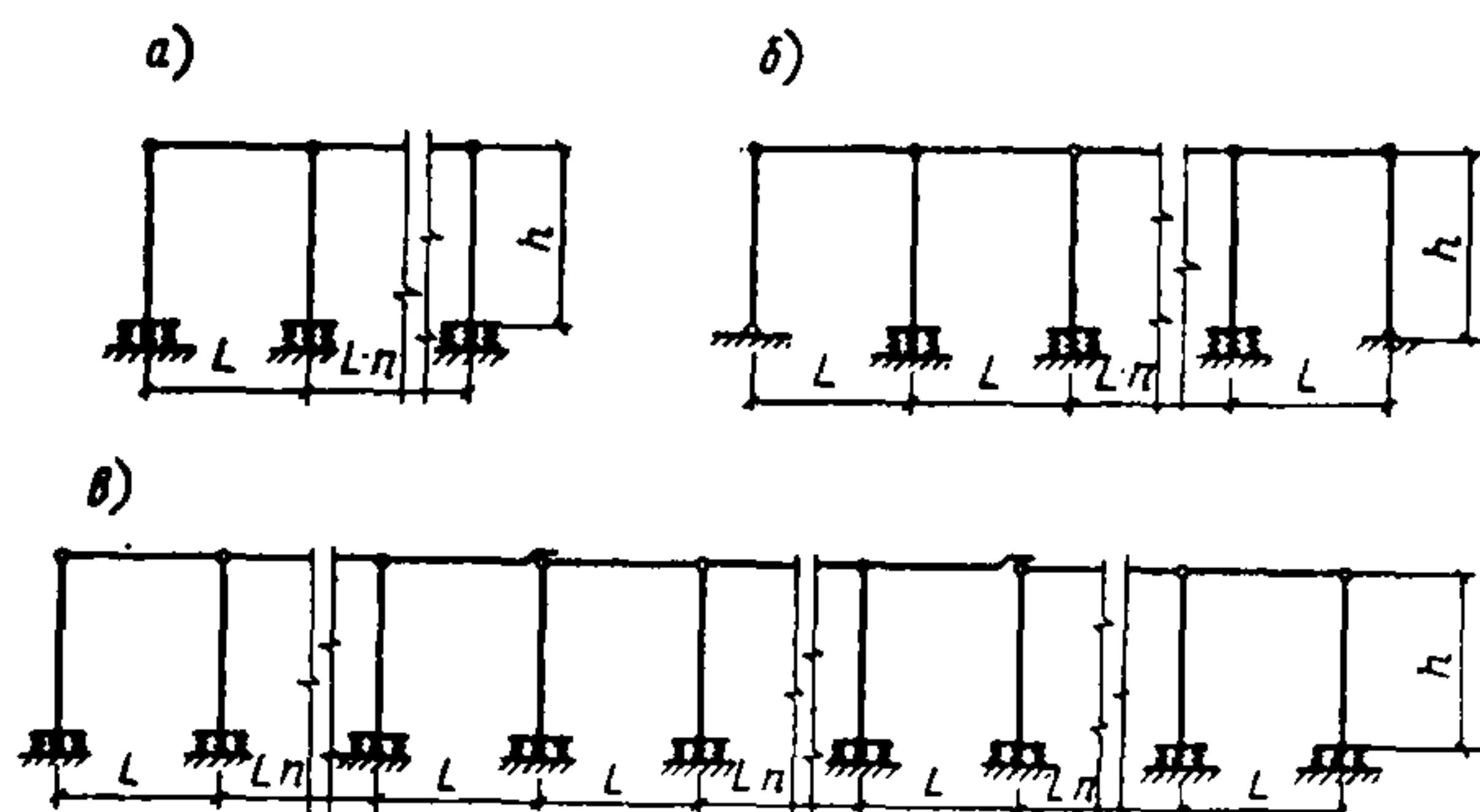
Рис. 5. Схемы поперечных рам одноэтажных каркасных зданий
