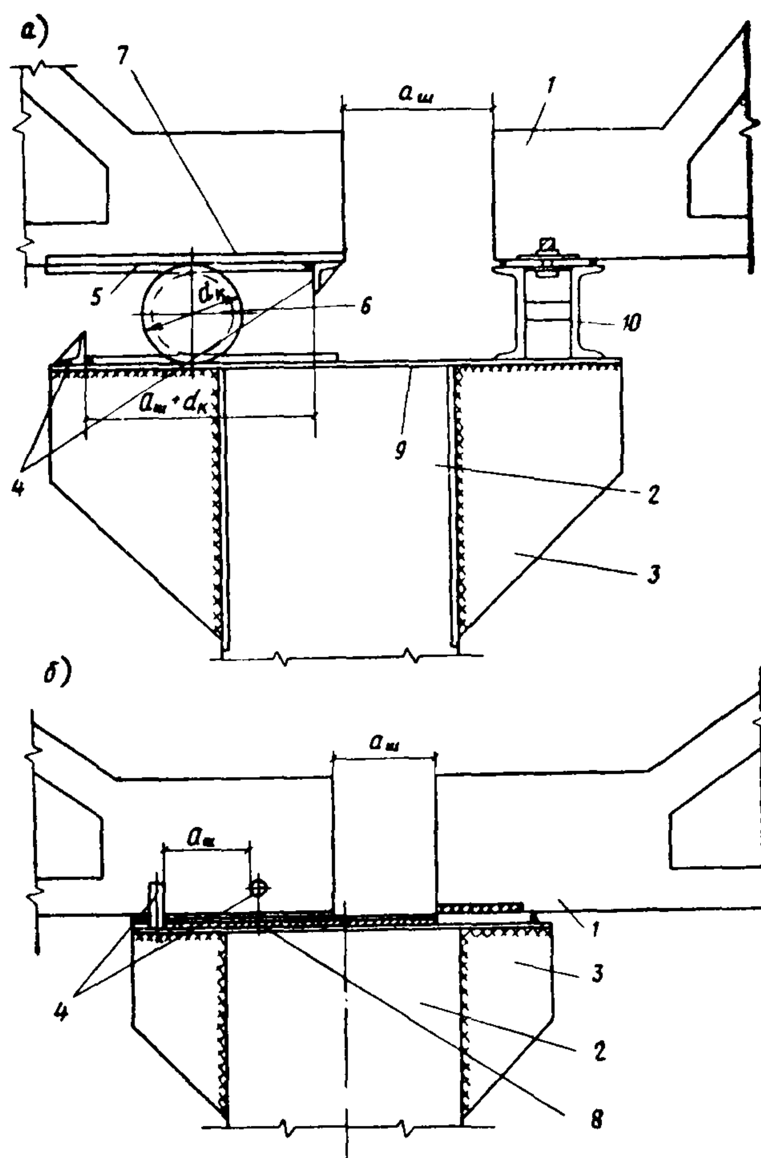
Рис. 6. Шарнирно-подвижные сопряжения
