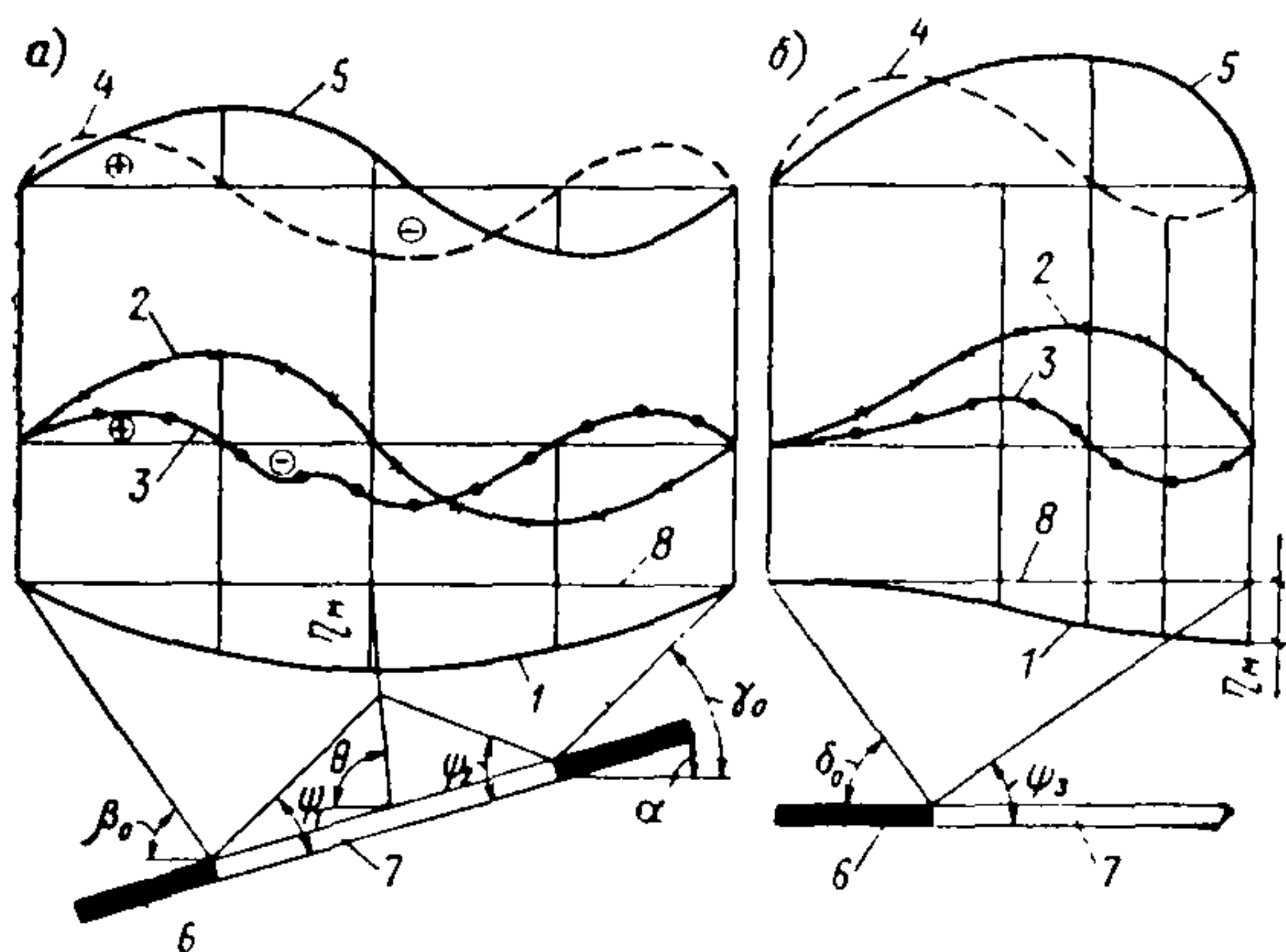
Рис. 1. Мульти сдвигения и эпюры деформаций земной поверхности
