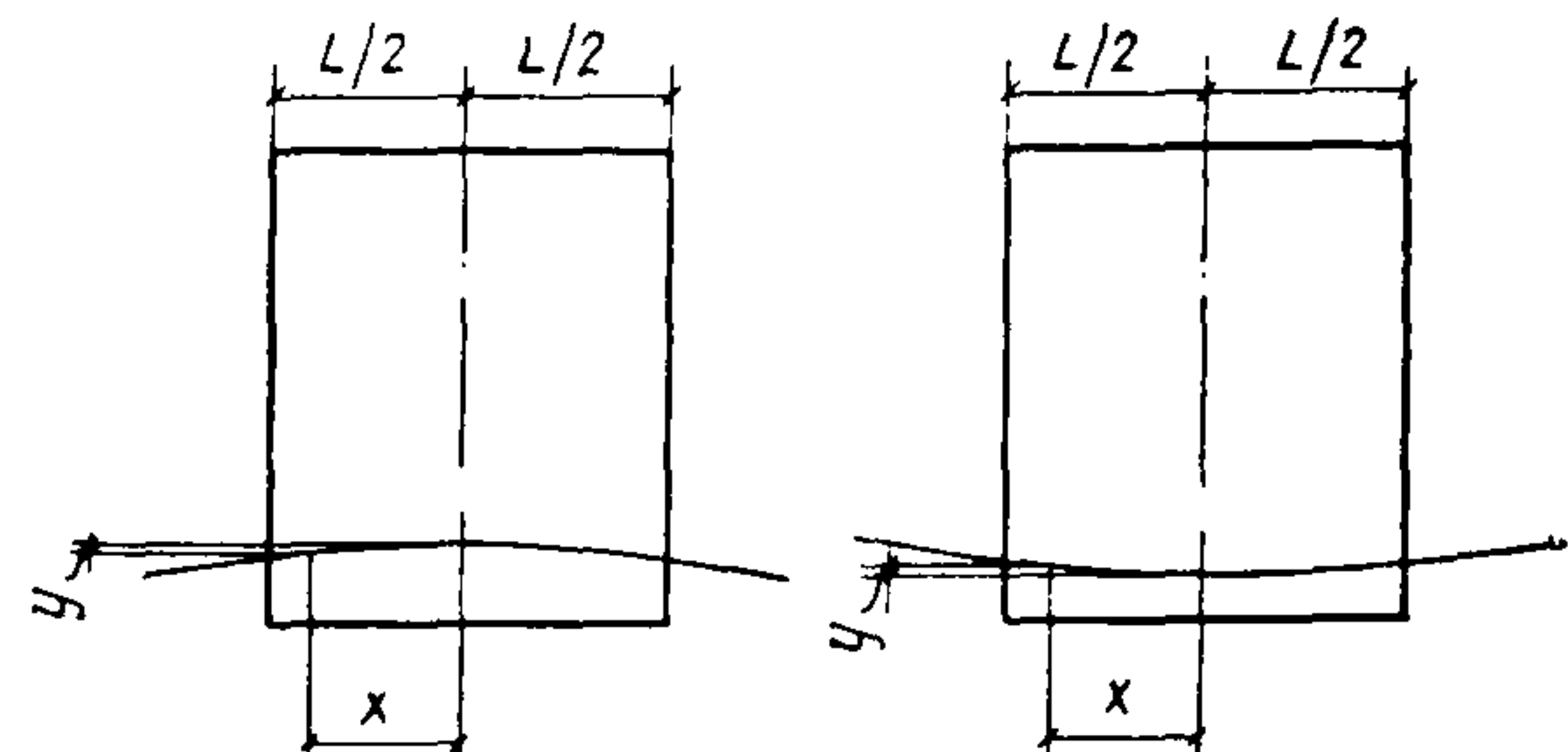
Рис. 2. Схема к расчету неравномерных оседаний из-за кривизны земной поверхности
