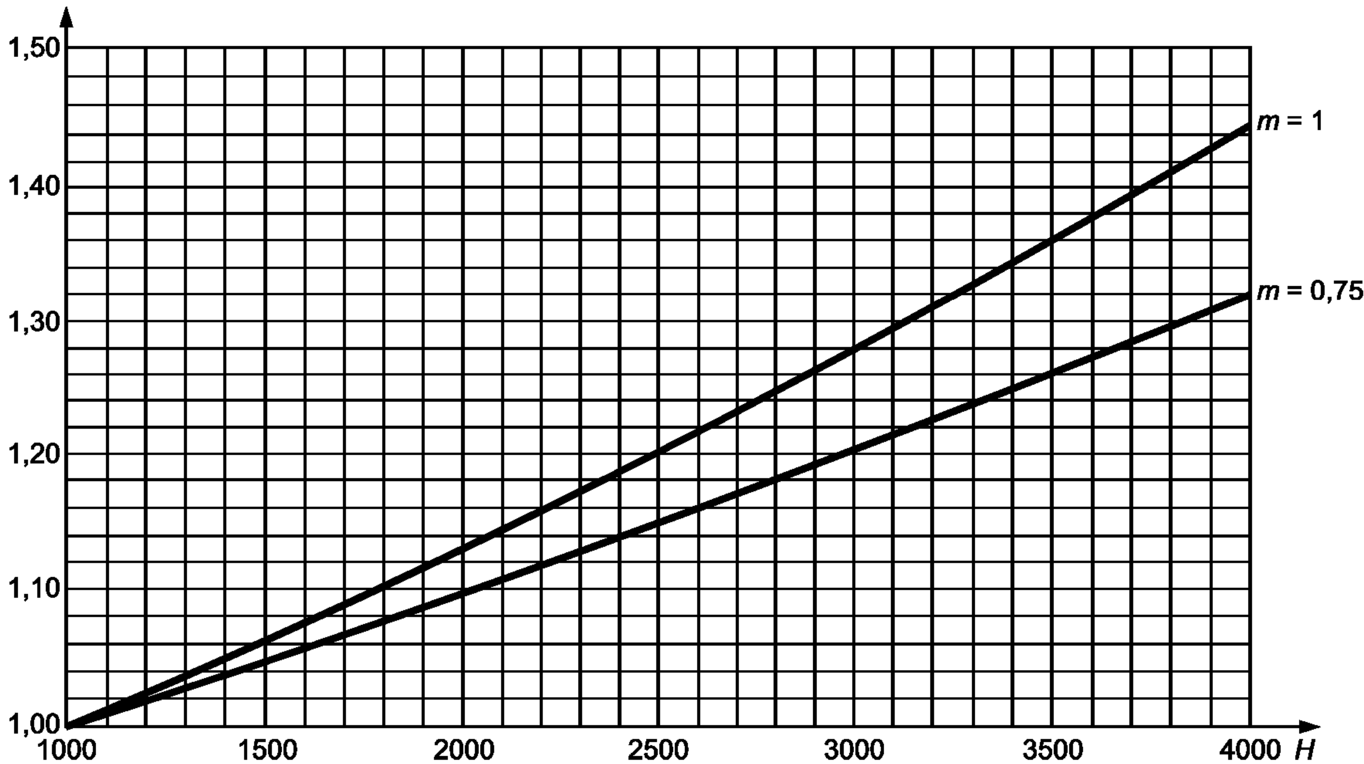
Рисунок 3 — Корректирующий высотный коэффициент
