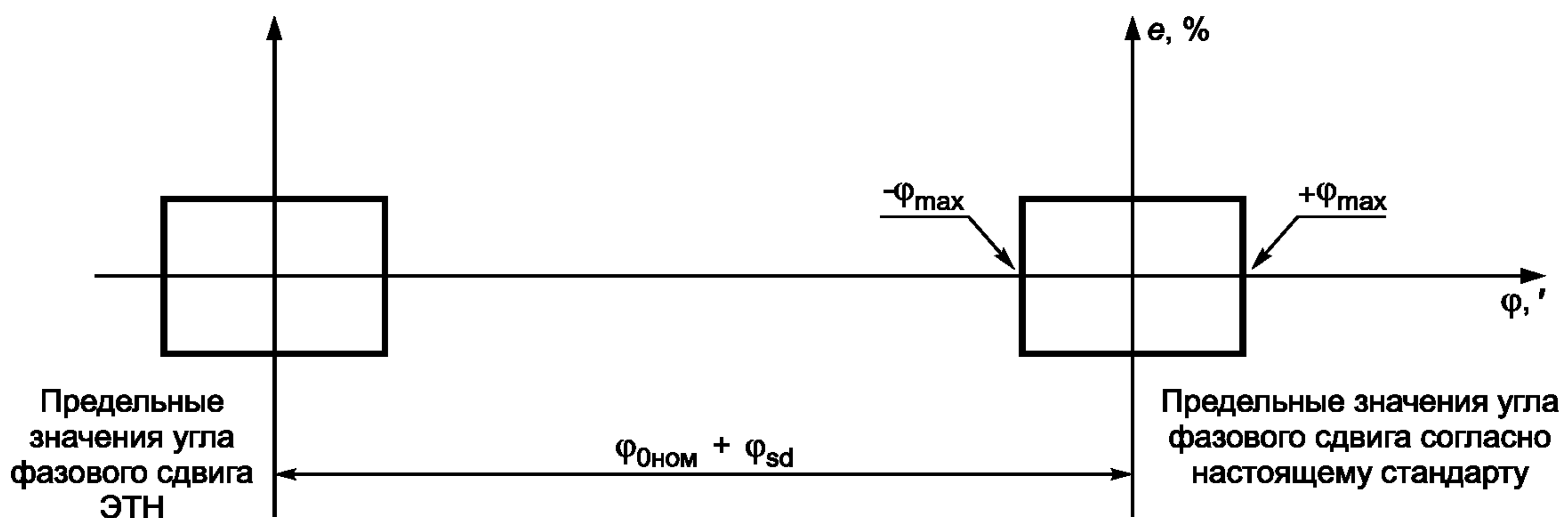
Рисунок В.7 — Требования к углу фазового сдвига
