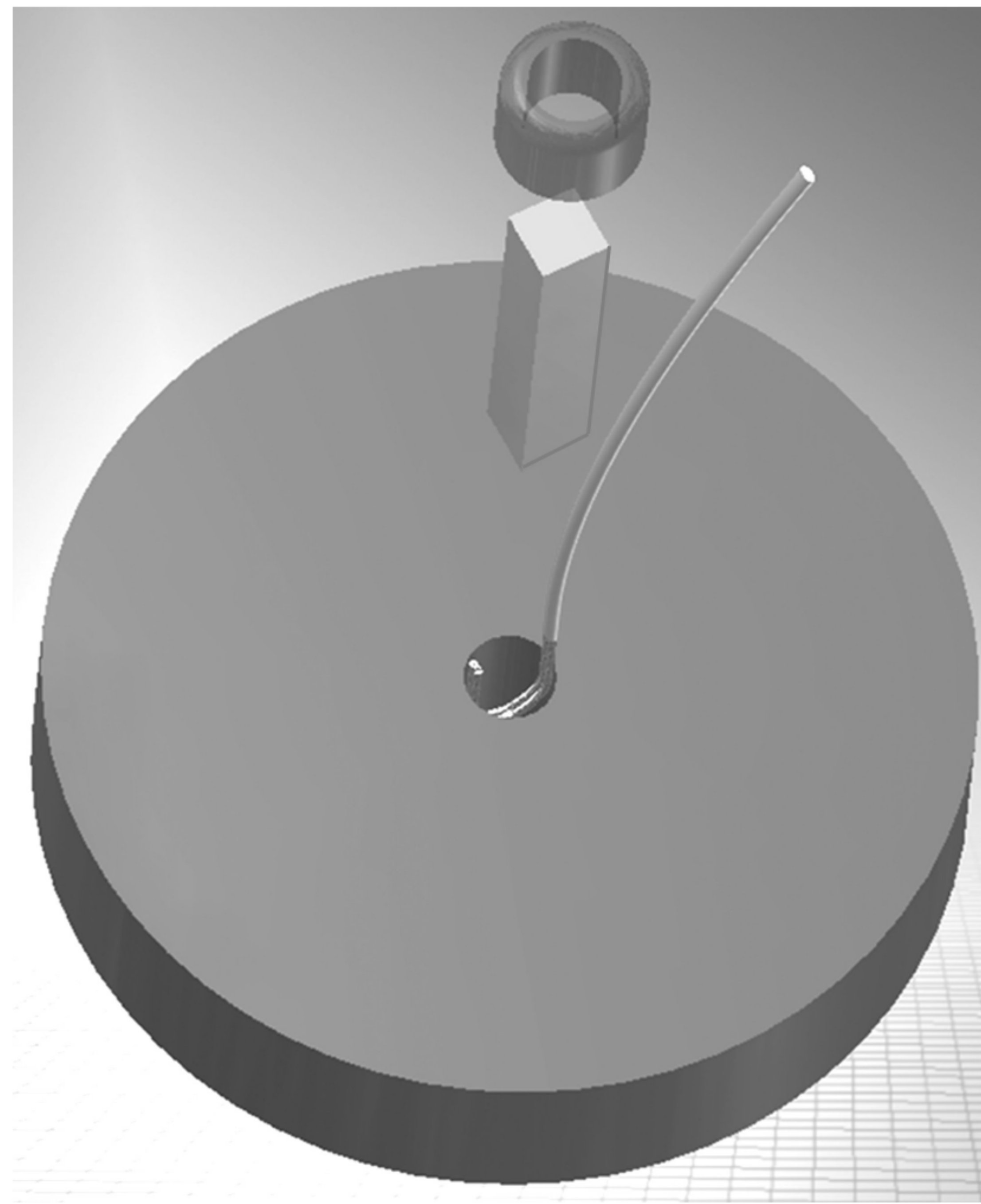
Рисунок 6 — Установка термopары на медный диск калориметра
