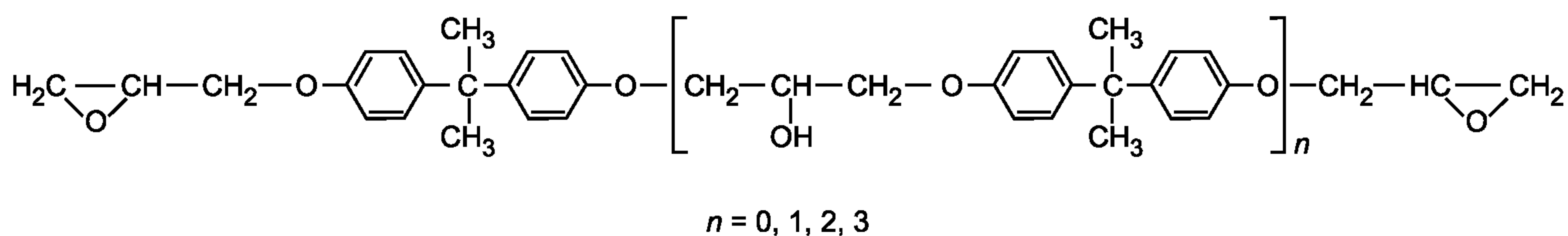
Рисунок А.1 — Молекулярная структура эпоксидной смолы
