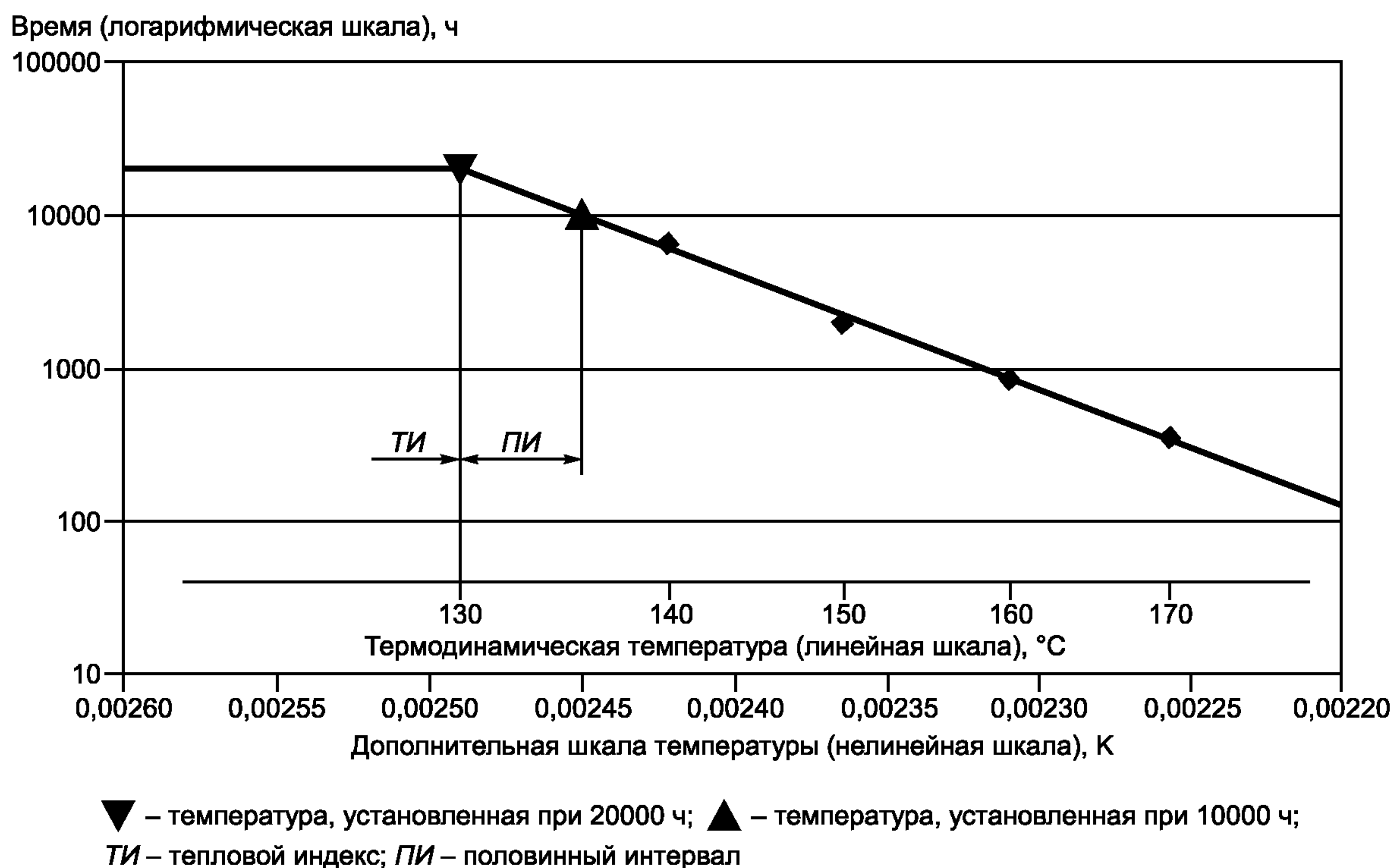
Рисунок А.2 — График теплостойкости
