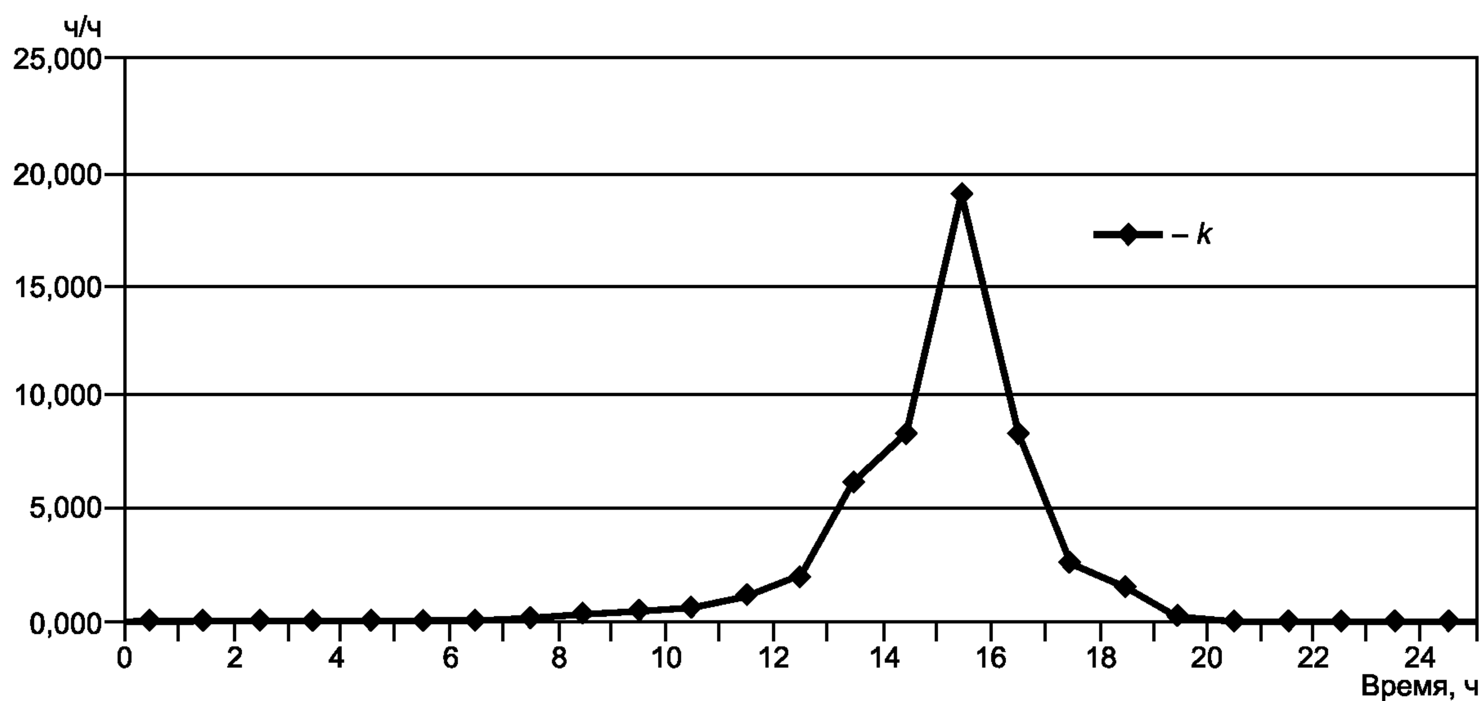
Рисунок Б.4 — Скорость теплового старения в зависимости от времени
