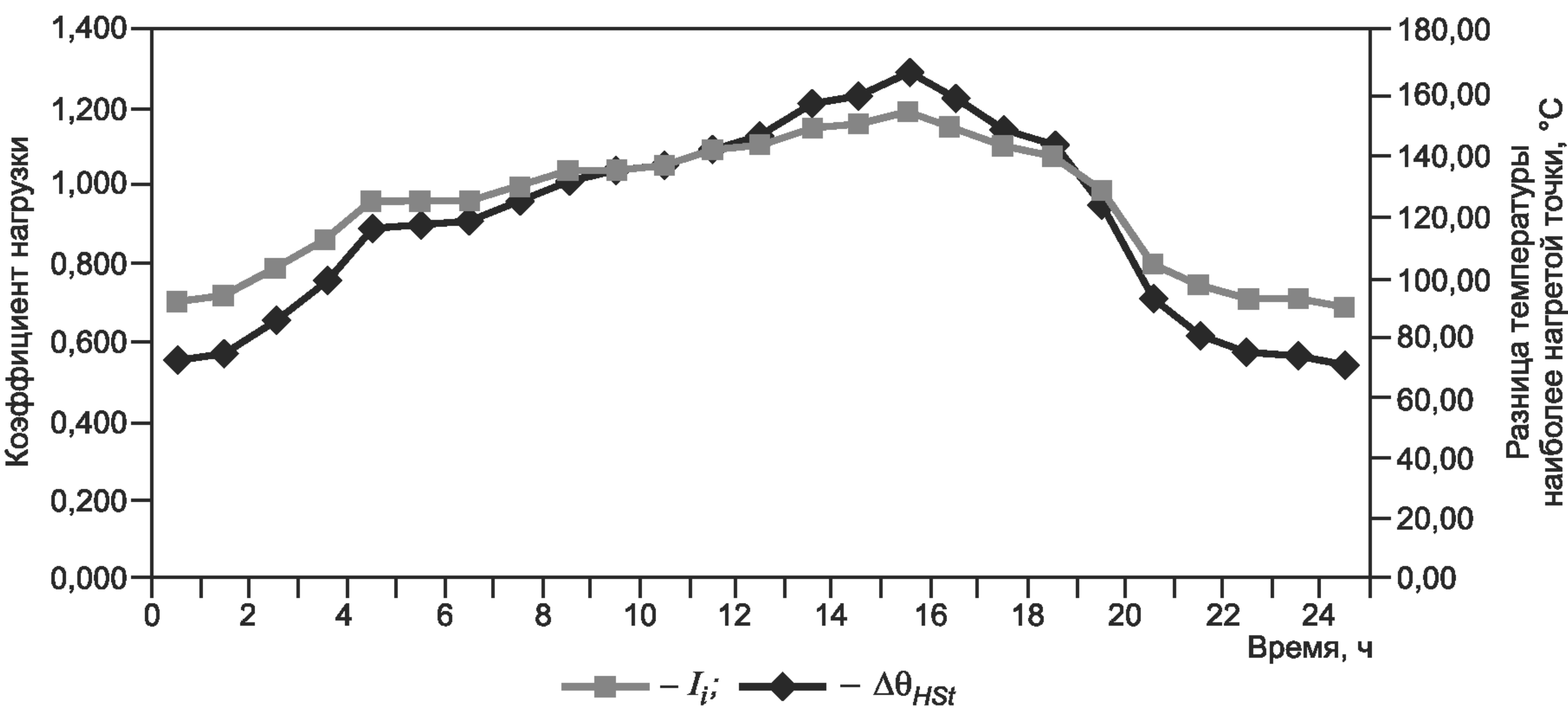
Рисунок Б.3 — Ток нагрузки и рост температуры наиболее нагретой точки обмотки
