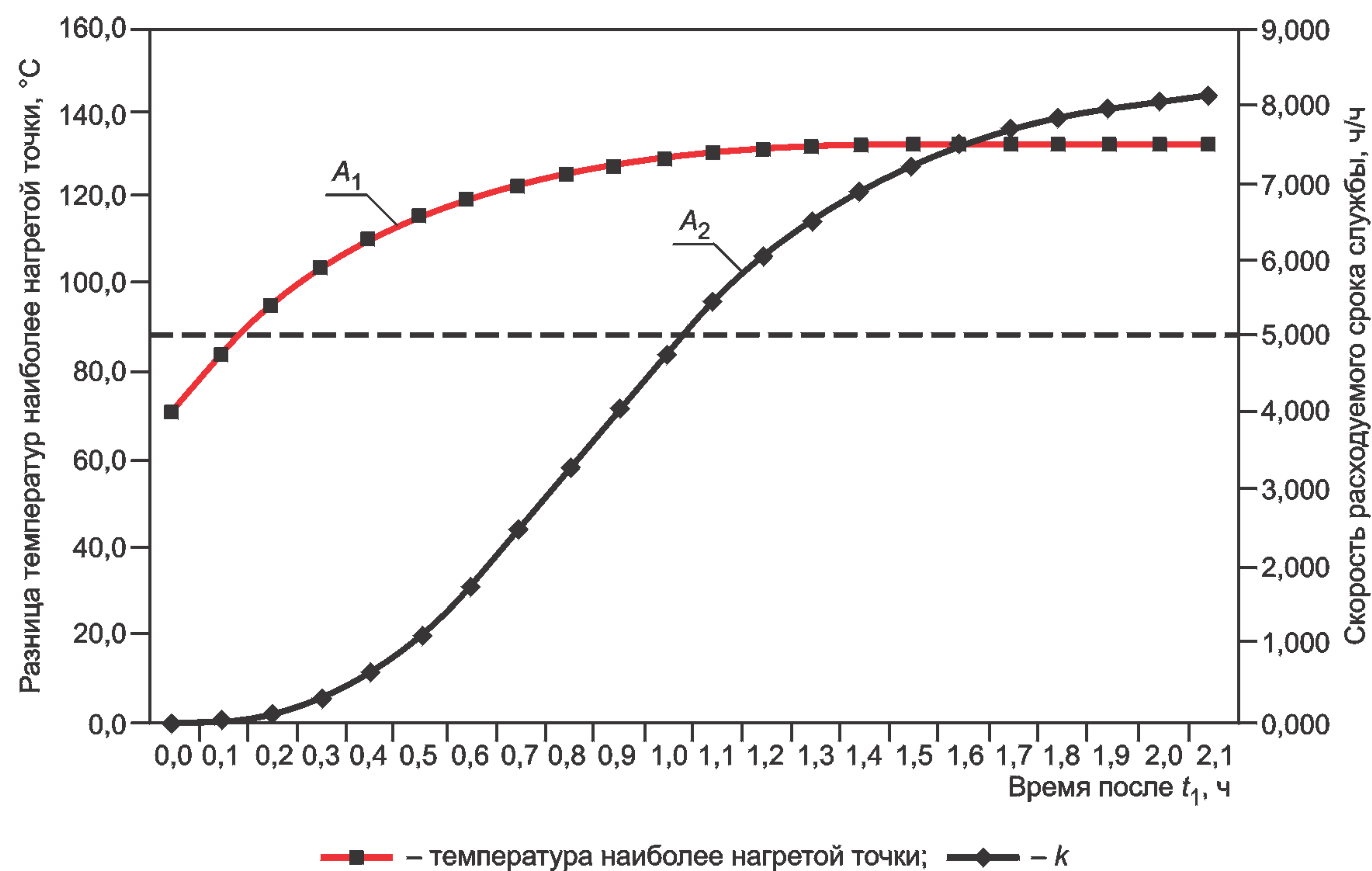
Верхняя кривая — рост разницы температуры наиболее нагретой точки, °С. Нижняя кривая: скорость расходуемого срока от всего срока службы трансформатора, соответствующая росту температуры наиболее нагретой точки
