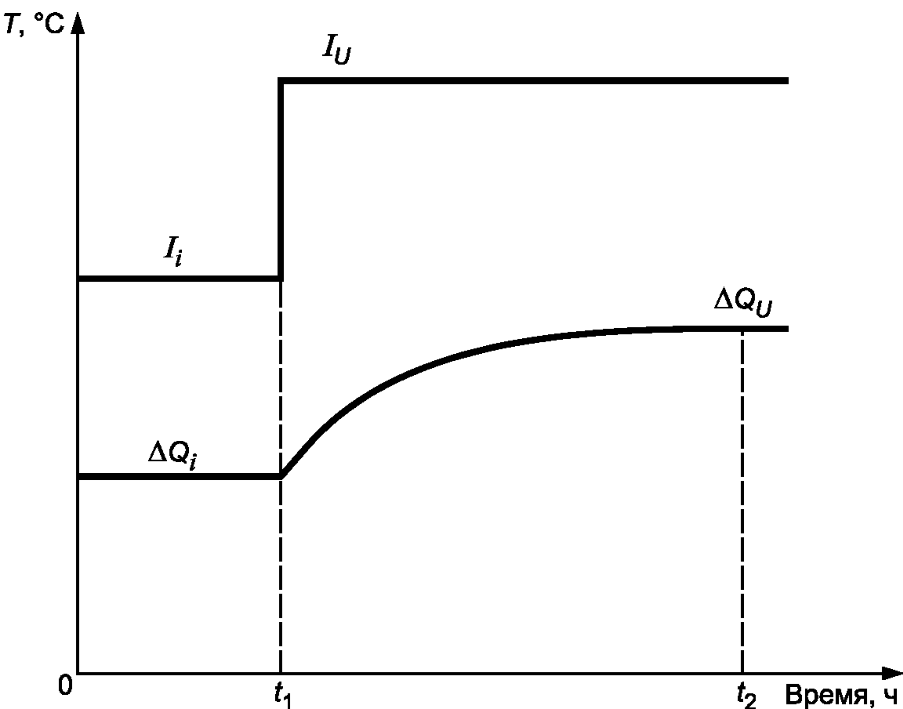
Верхняя кривая: начальная и максимальная нагрузки. Нижняя кривая: рост температуры выше температуры окружающей среды
