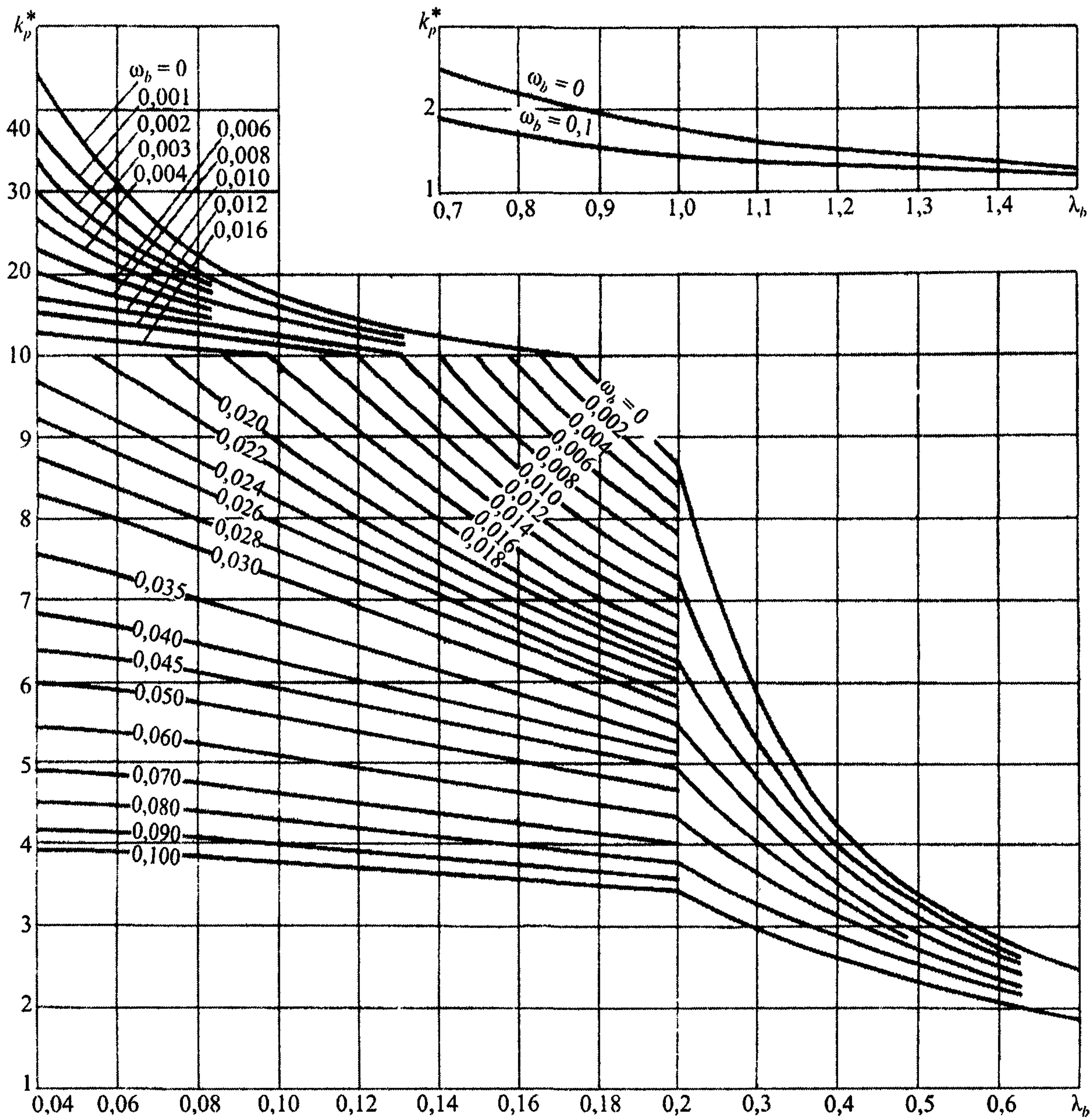
Рисунок 1 – График для определения значений коэффициента k_p^*
