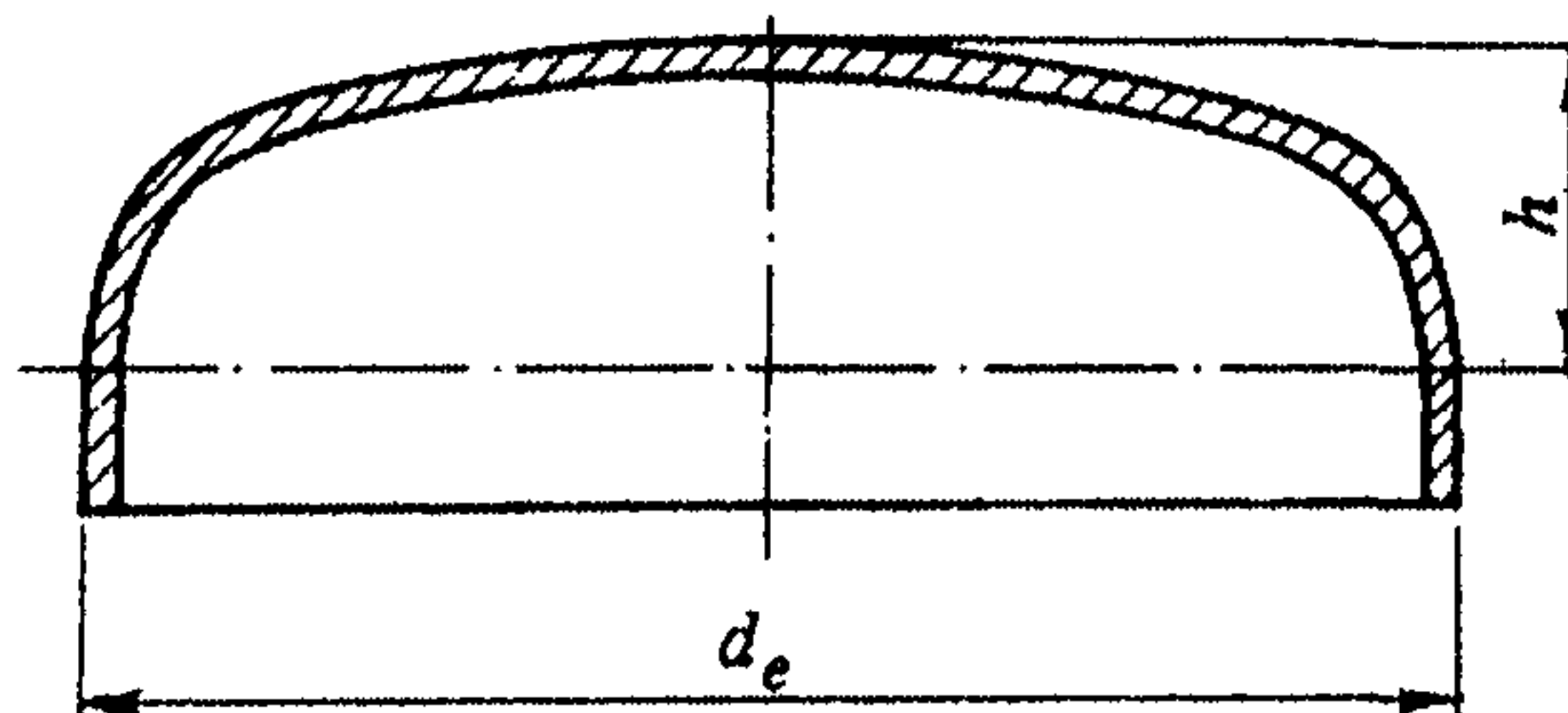
Рисунок А.3 – Заглушка эллиптическая
