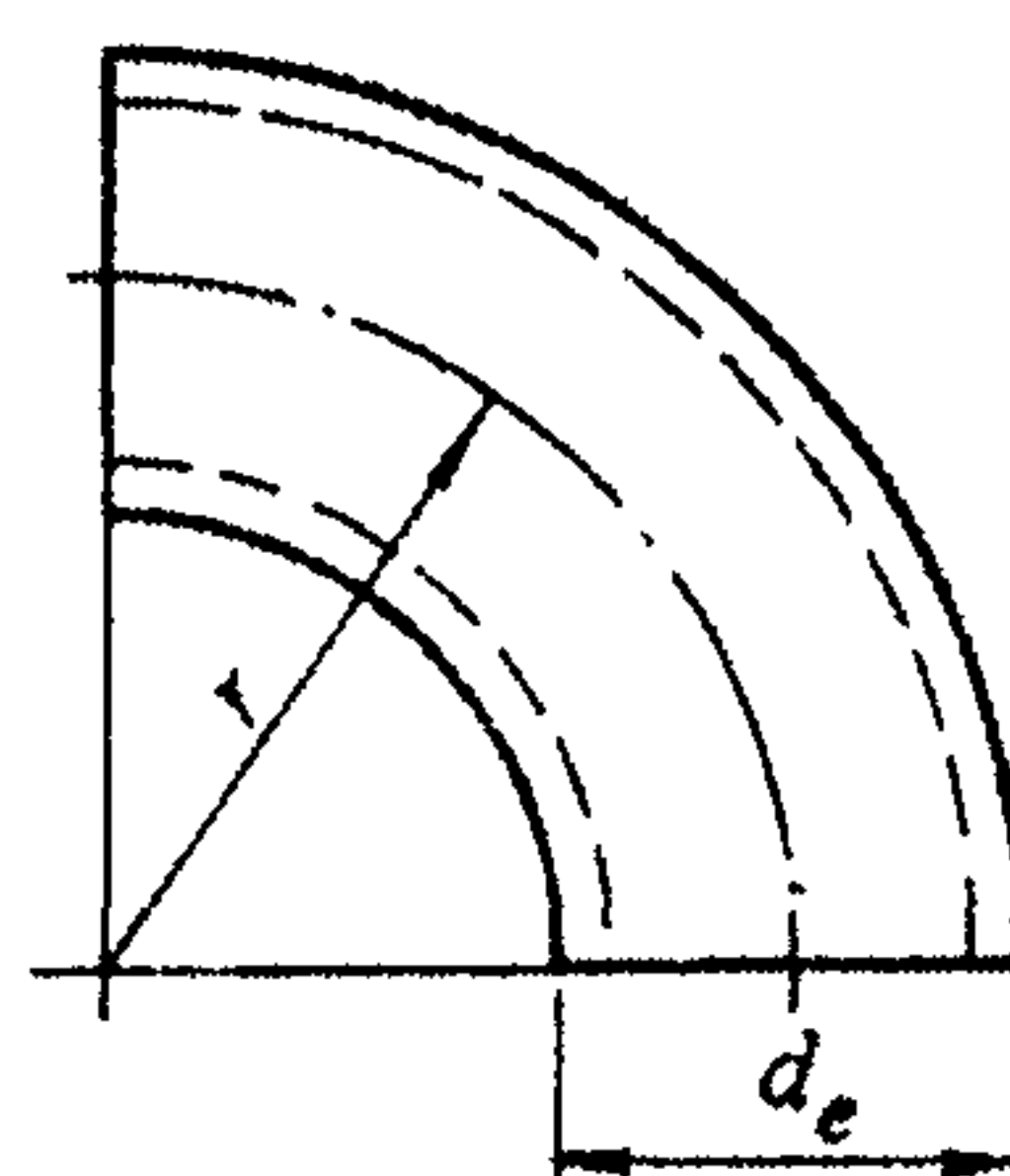
Рисунок А.4 – Отвод бесшовный и штамповарный
