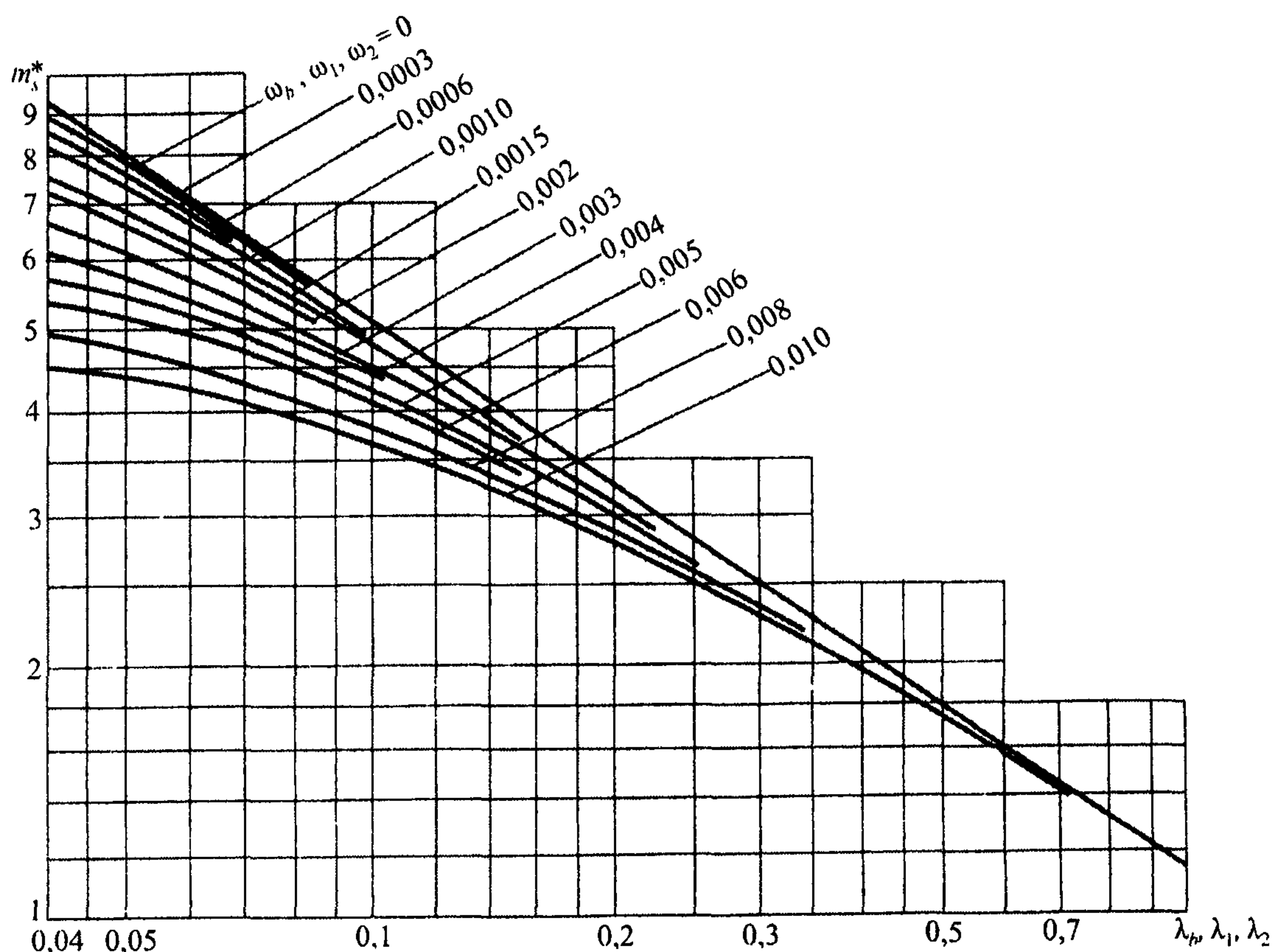
Рисунок 2 – График для определения значений коэффициента m_s^*
