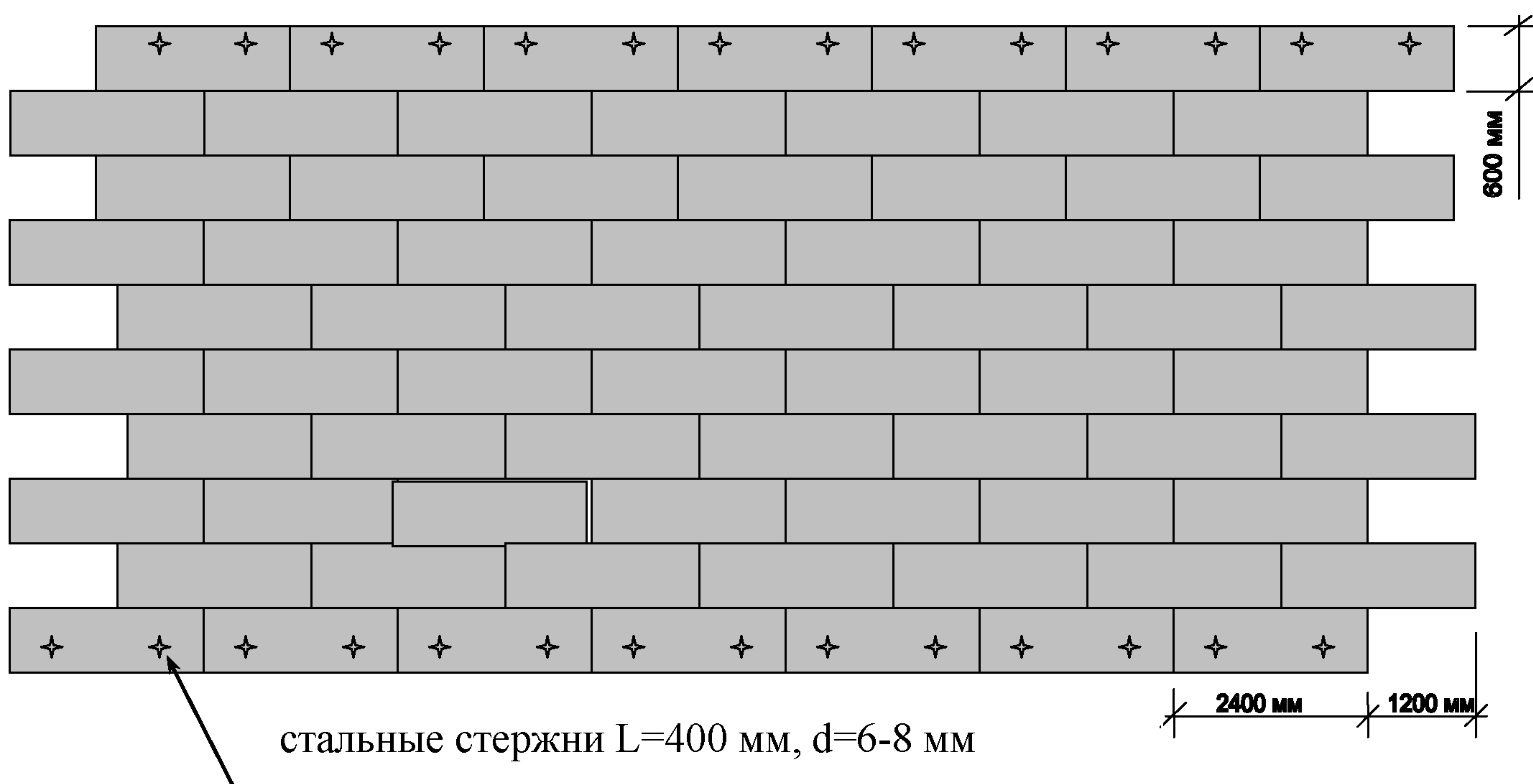
Рисунок 5 - Раскладка вспененных геоплит в теплоизоляционном слое
