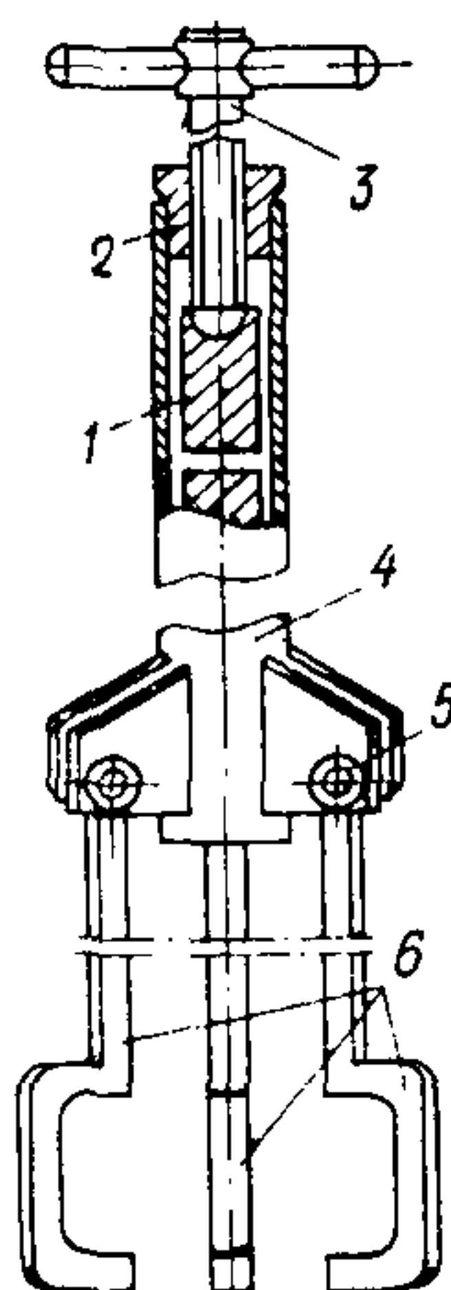
Рис. 2. Приспособление для снятия рабочего колеса с вала центробежных насосов типа НДиД
