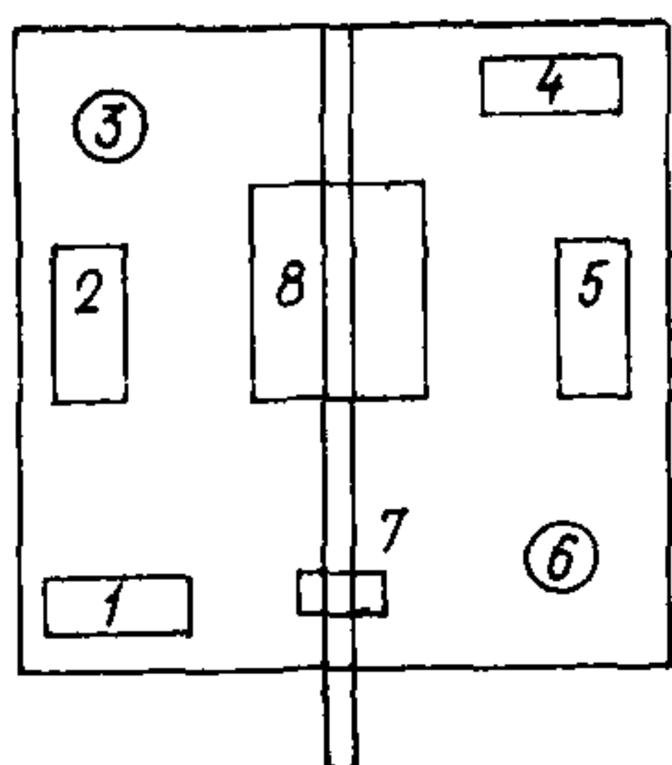
Рис. 8. Типовая схема организации рабочего места слесаря-ремонтника при ремонте насосов
