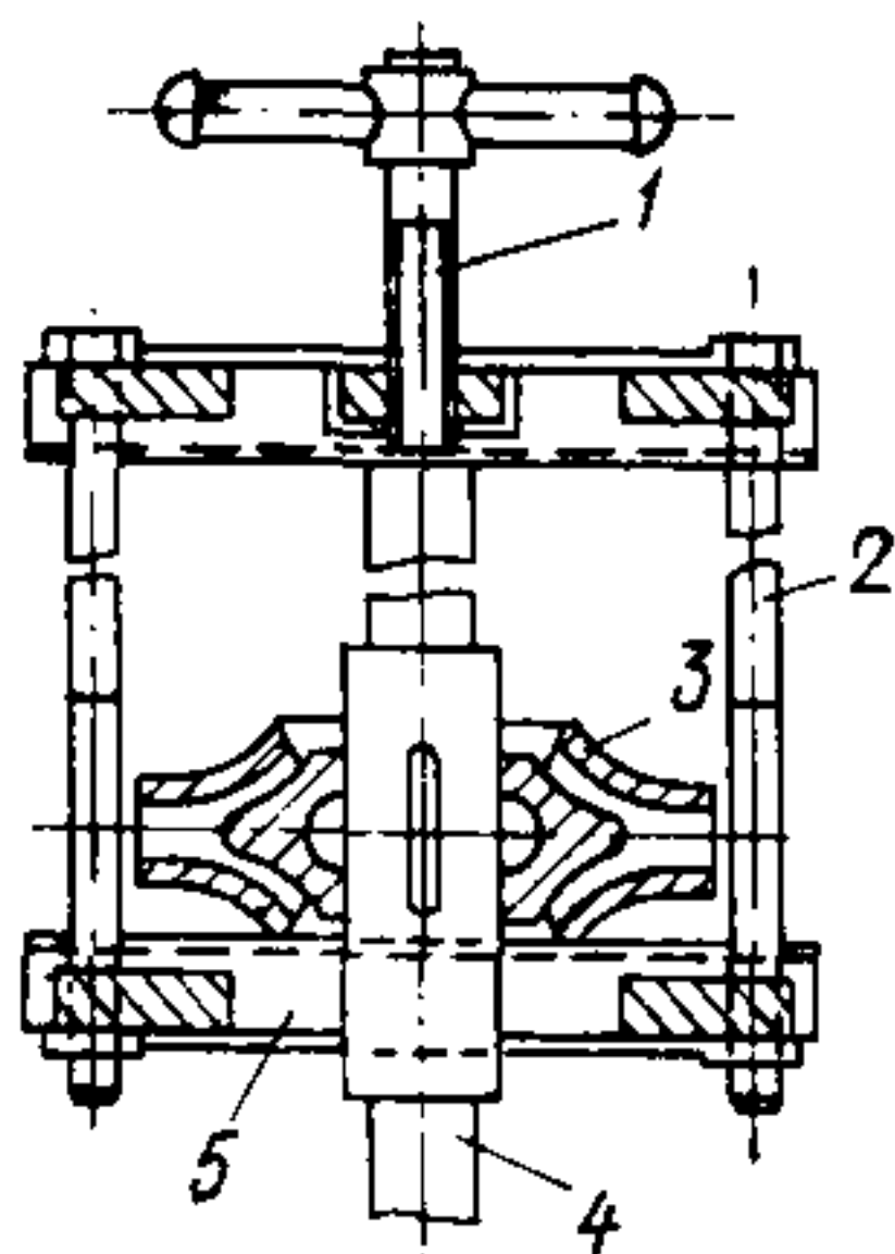
Рис. 3. Приспособление для спрессовки рабочих колес
