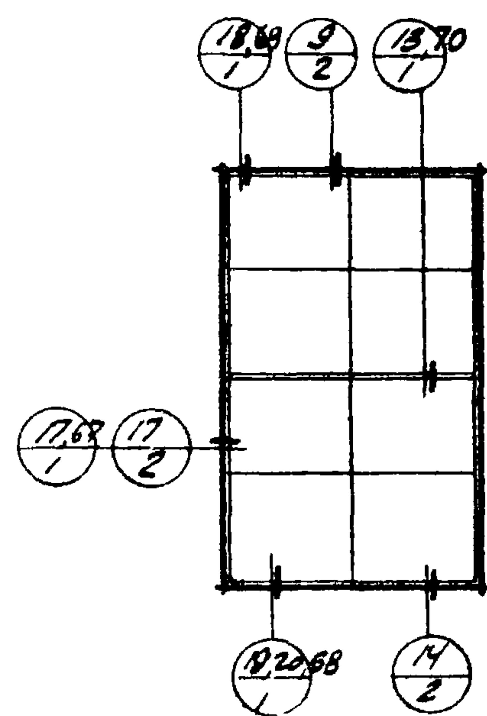
ОДИНАРНЫЕ ПЕРЕПЛЕТЫ СПАРЕННЫЕ ПЕРЕПЛЕТЫ В КИРПИЧНЫХ СТЕНАХ
