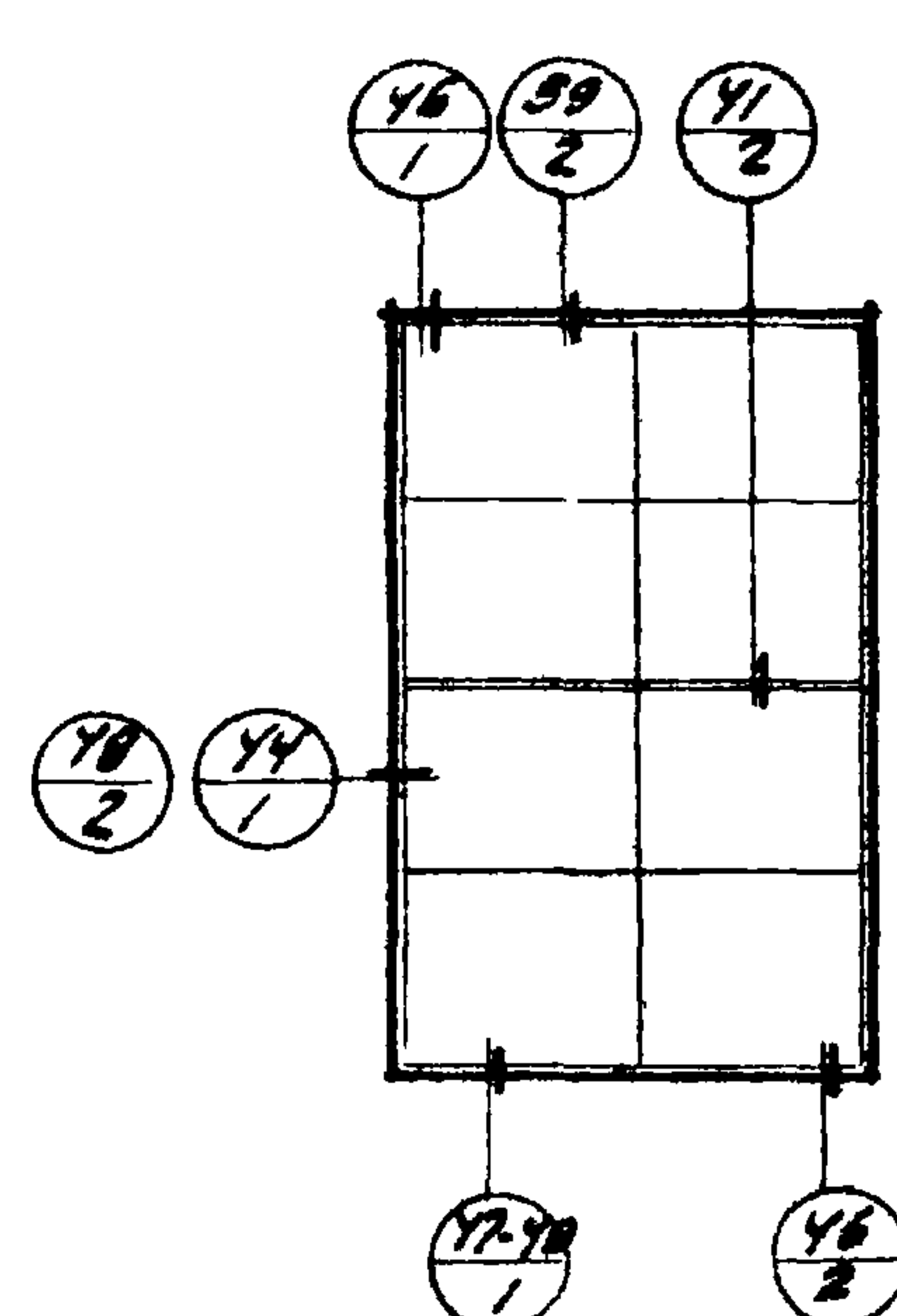
ДВОЙНЫЕ РАЗДЕЛЬНЫЕ ПЕРЕПЛЕТЫ В КИРПИЧНЫХ СТЕНАХ
