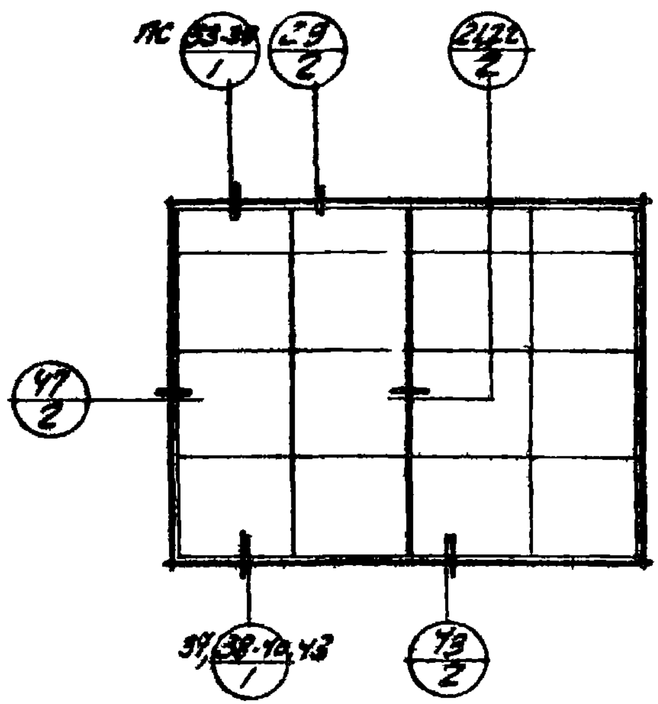
ДВОЙНЫЕ РАЗДЕЛЬНЫЕ ПЕРЕПЛЕТЫ В ПАНЕЛЬНЫХ СТЕНАХ
