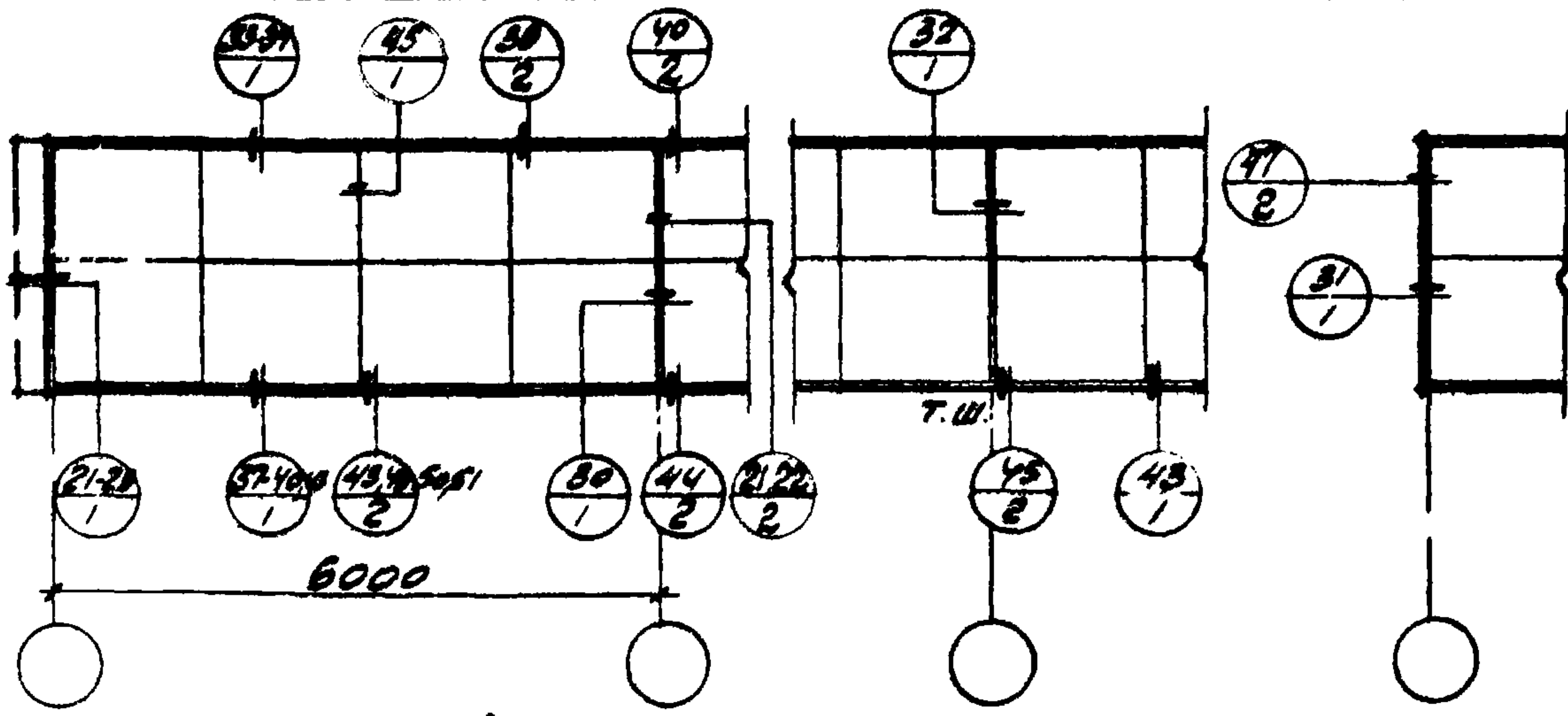
СХЕМА С ДВОЙНЫМИ РАЗДЕЛЬНЫМИ ПЕРЕПЛЕТАМИ
