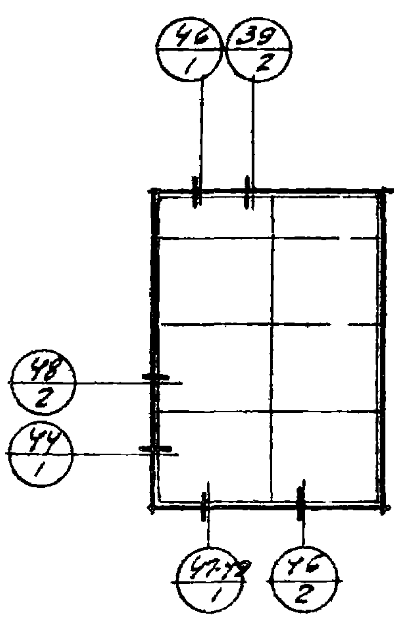
ДВОЙНЫЕ РАЗДЕЛЬНЫЕ ПЕРЕПЛЕТЫ В КИРПИЧНЫХ СТЕНАХ
