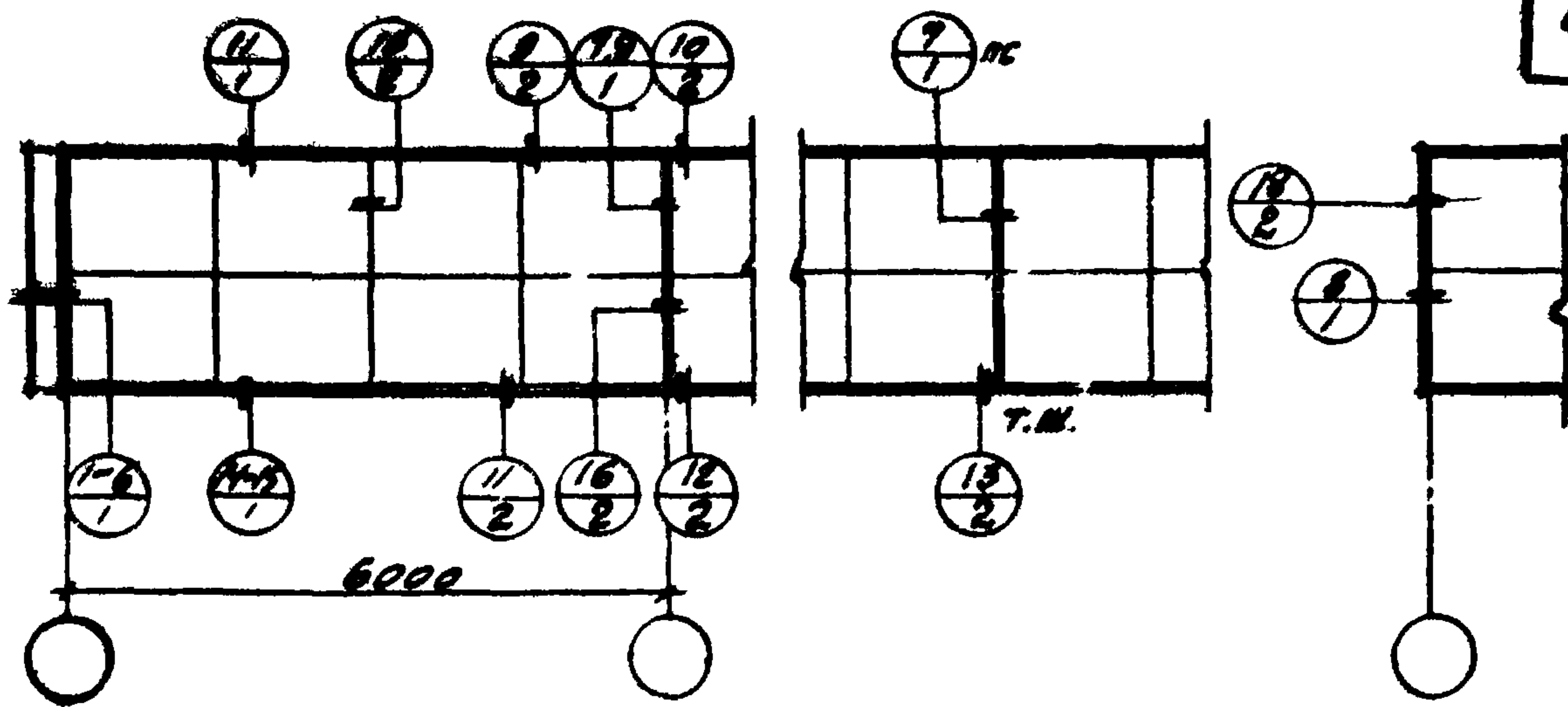
СХЕМА С ОДИНАРНЫМИ ПЕРЕПЛЕТАМИ
