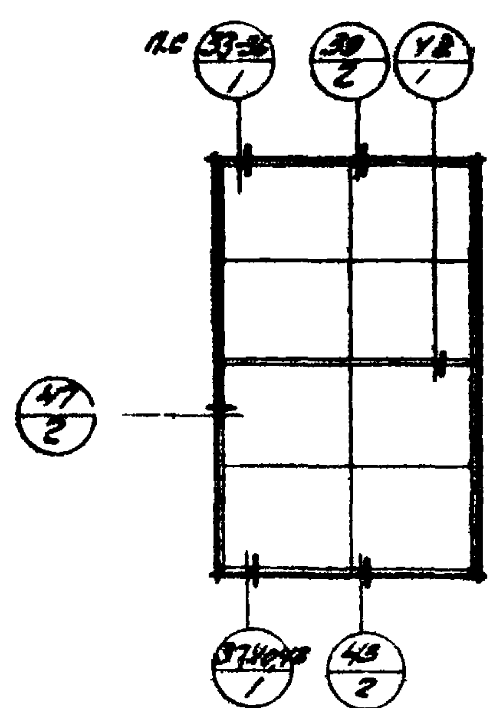
ДВОЙНЫЕ РАЗДЕЛЬНЫЕ ПЕРЕПЛЕТЫ В ПАНЕЛЬНЫХ СТЕНАХ
