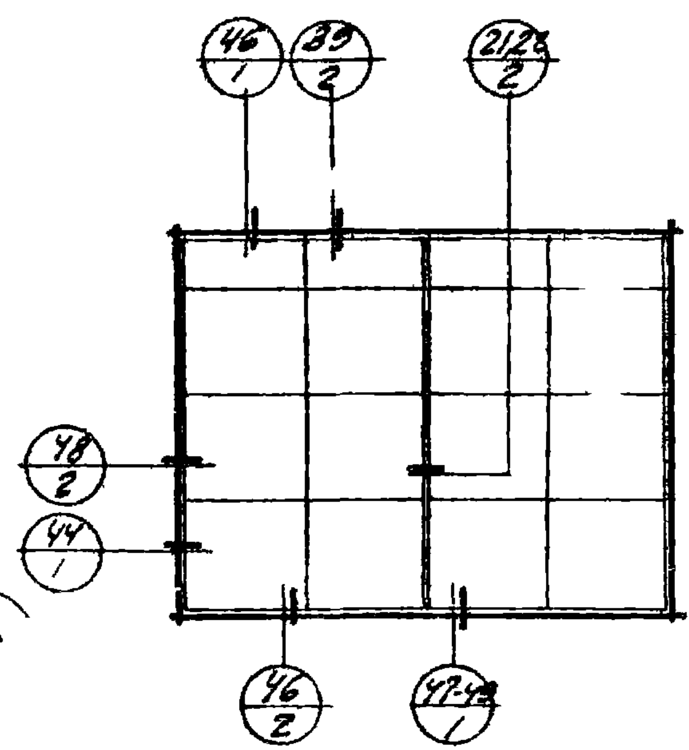
ДВОЙНЫЕ РАЗДЕЛЬНЫЕ ПЕРЕПЛЕТЫ В КИРПИЧНЫХ СТЕНАХ
