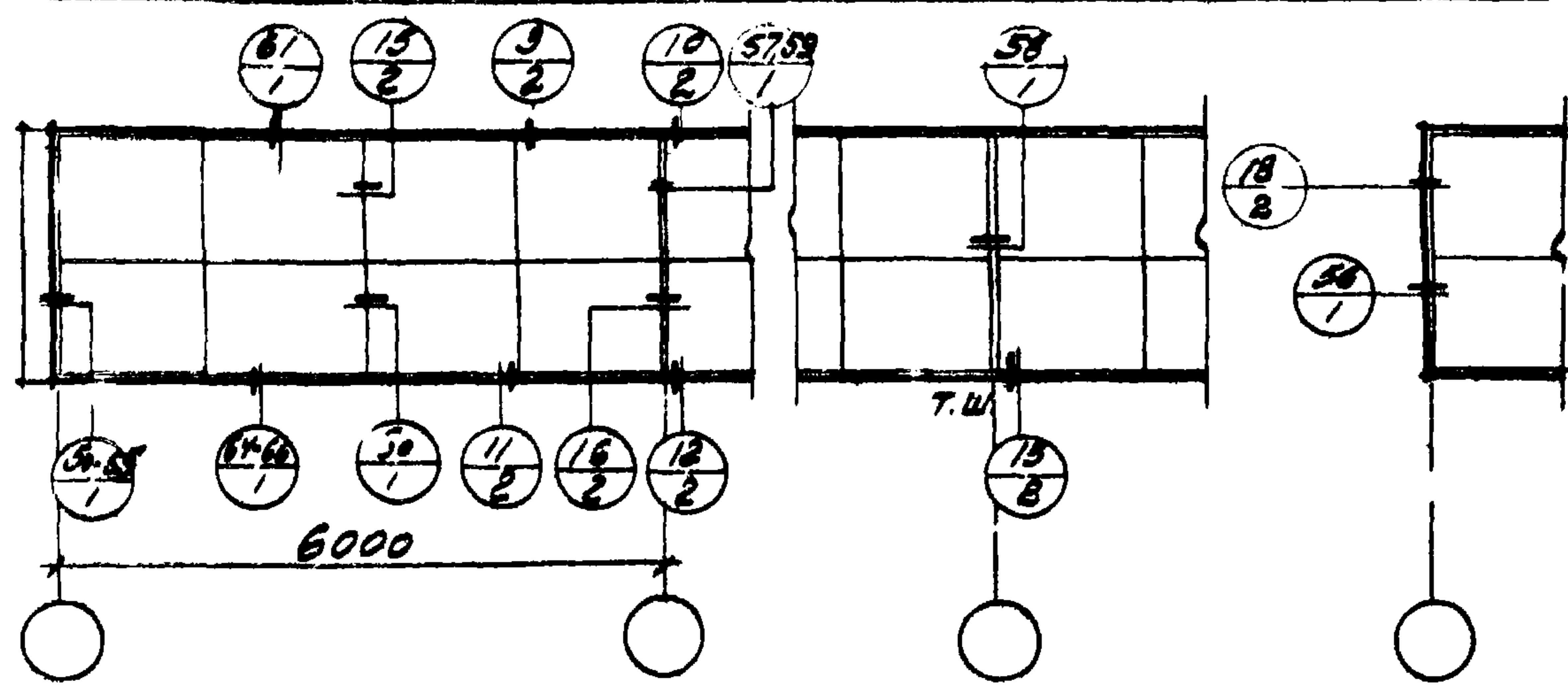
СХЕМА СО СПАРЕННЫМИ ПЕРЕПЛЕТАМИ
