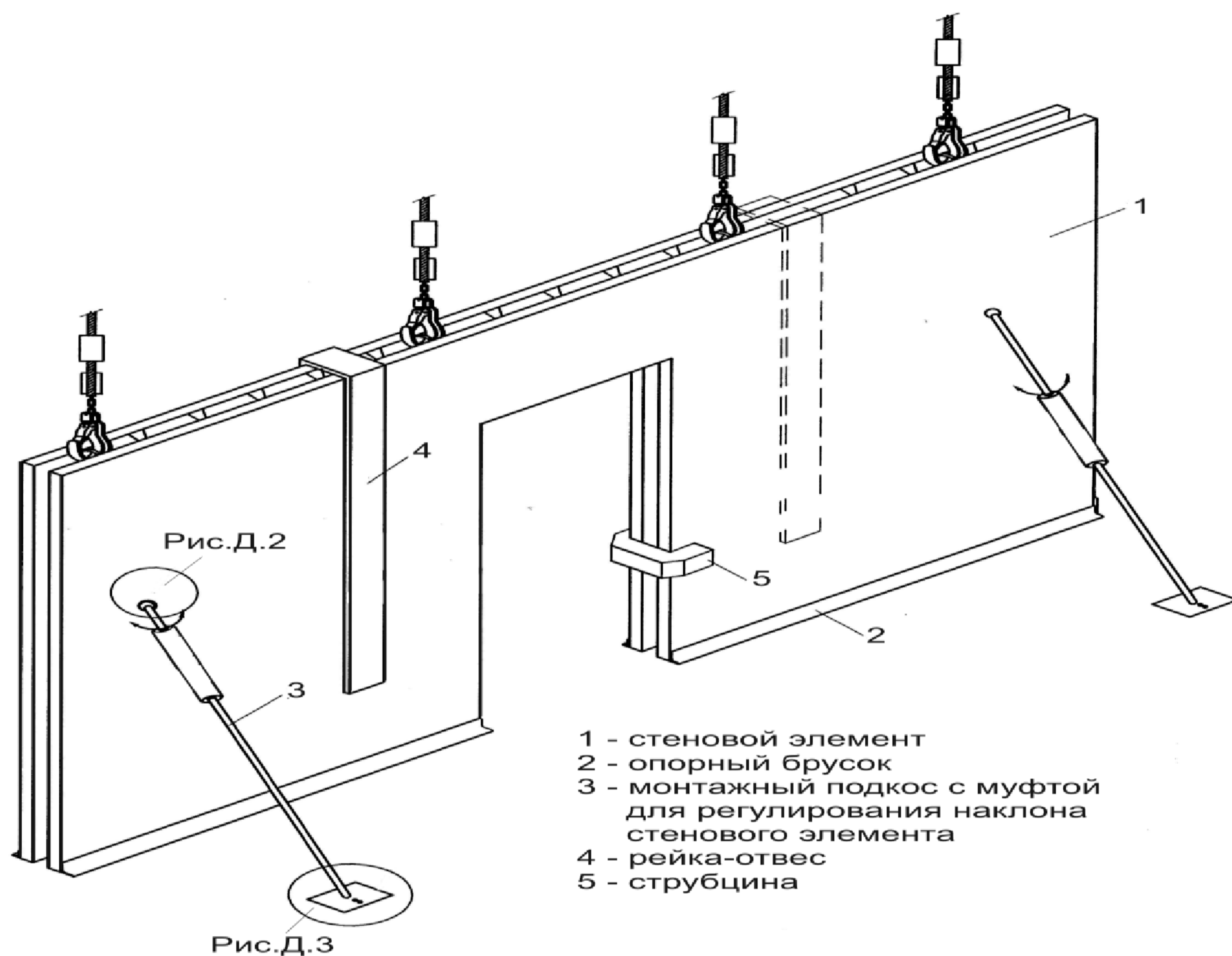
Рисунок Д.5 – Выверка стенового элемента при монтаже
