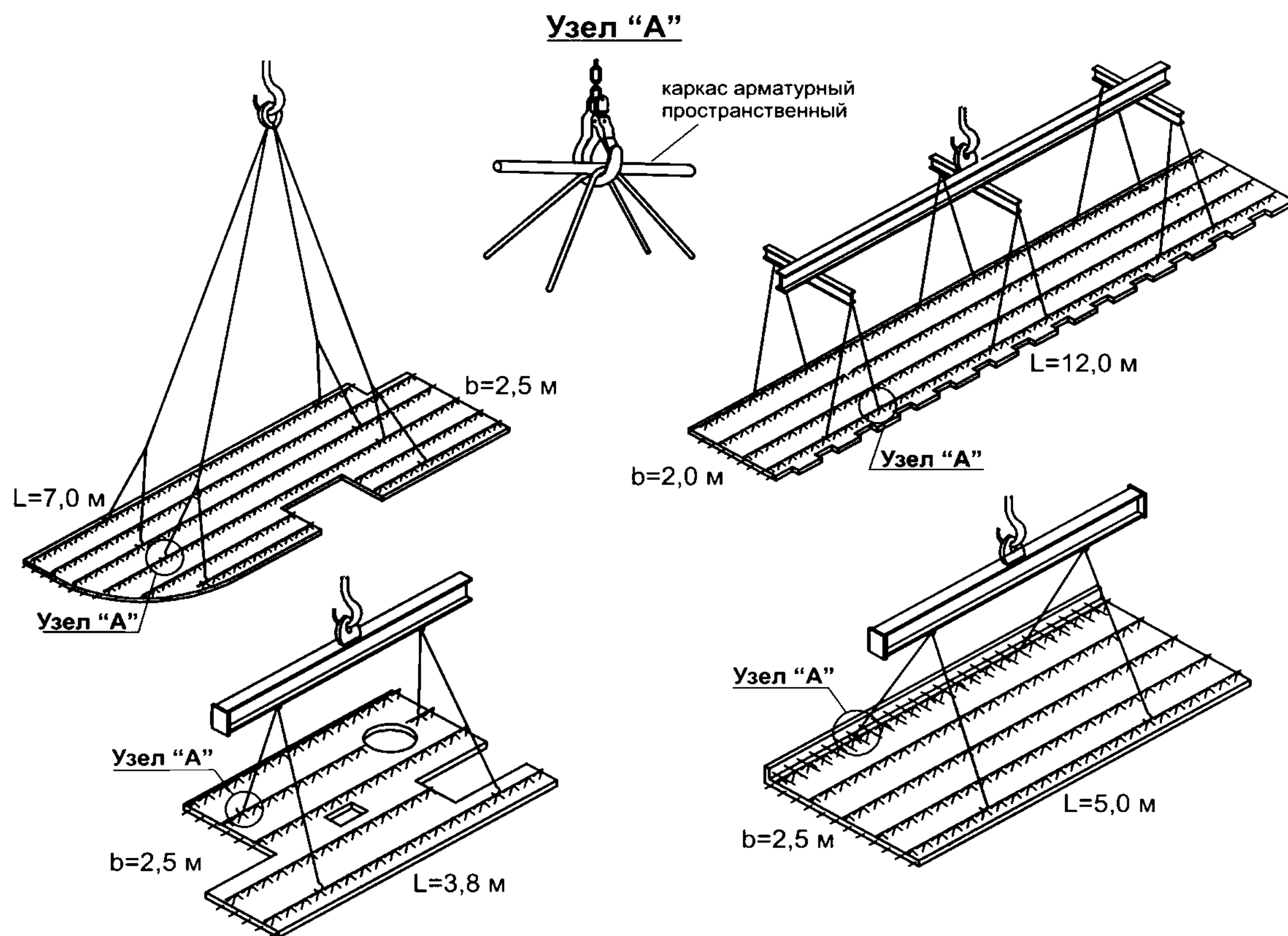
Рисунок Г.1 – Примеры строповок сборных элементов перекрытий
