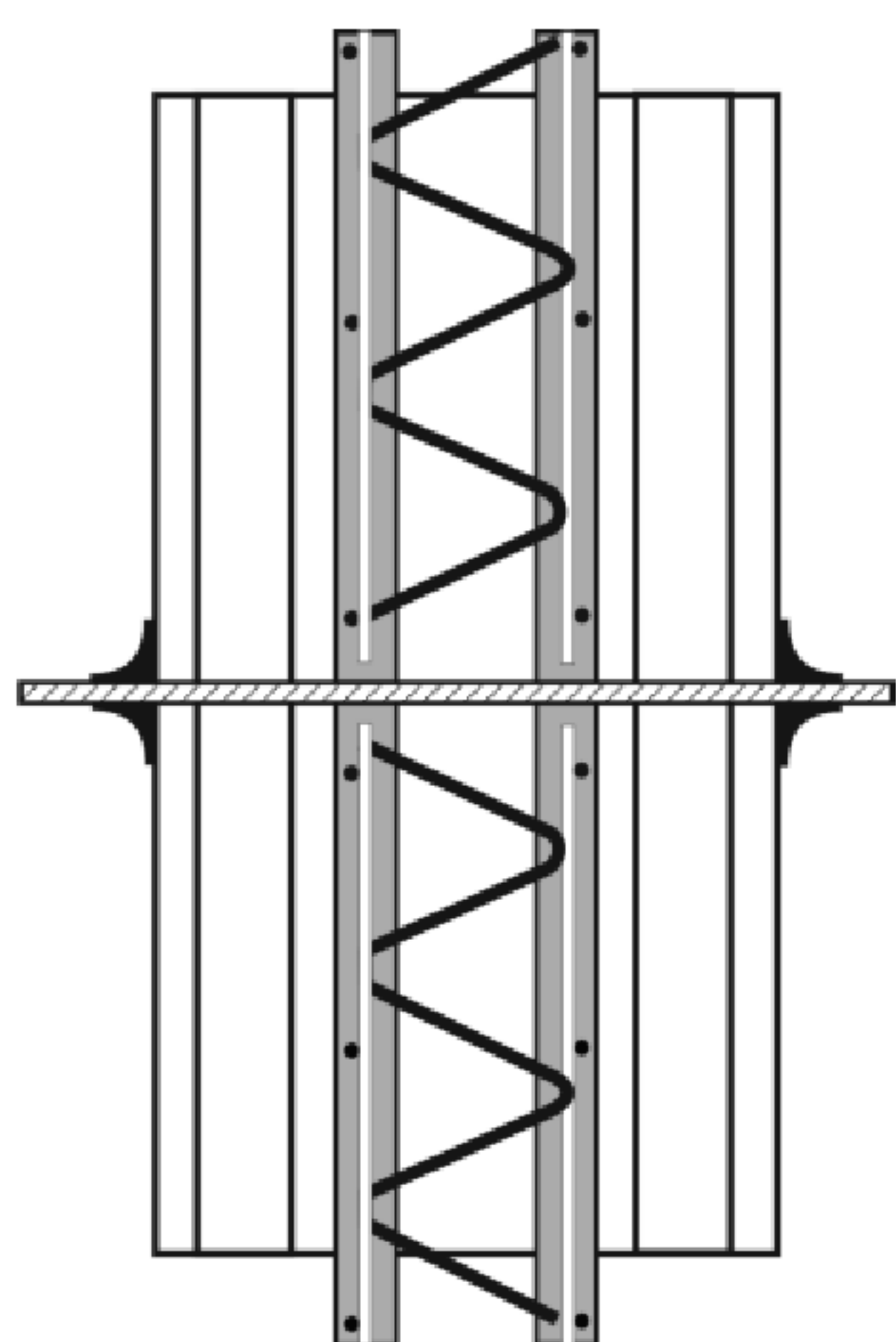
Рисунок Д.4 – Установка стяжек на стыках панелей (вид сверху)
