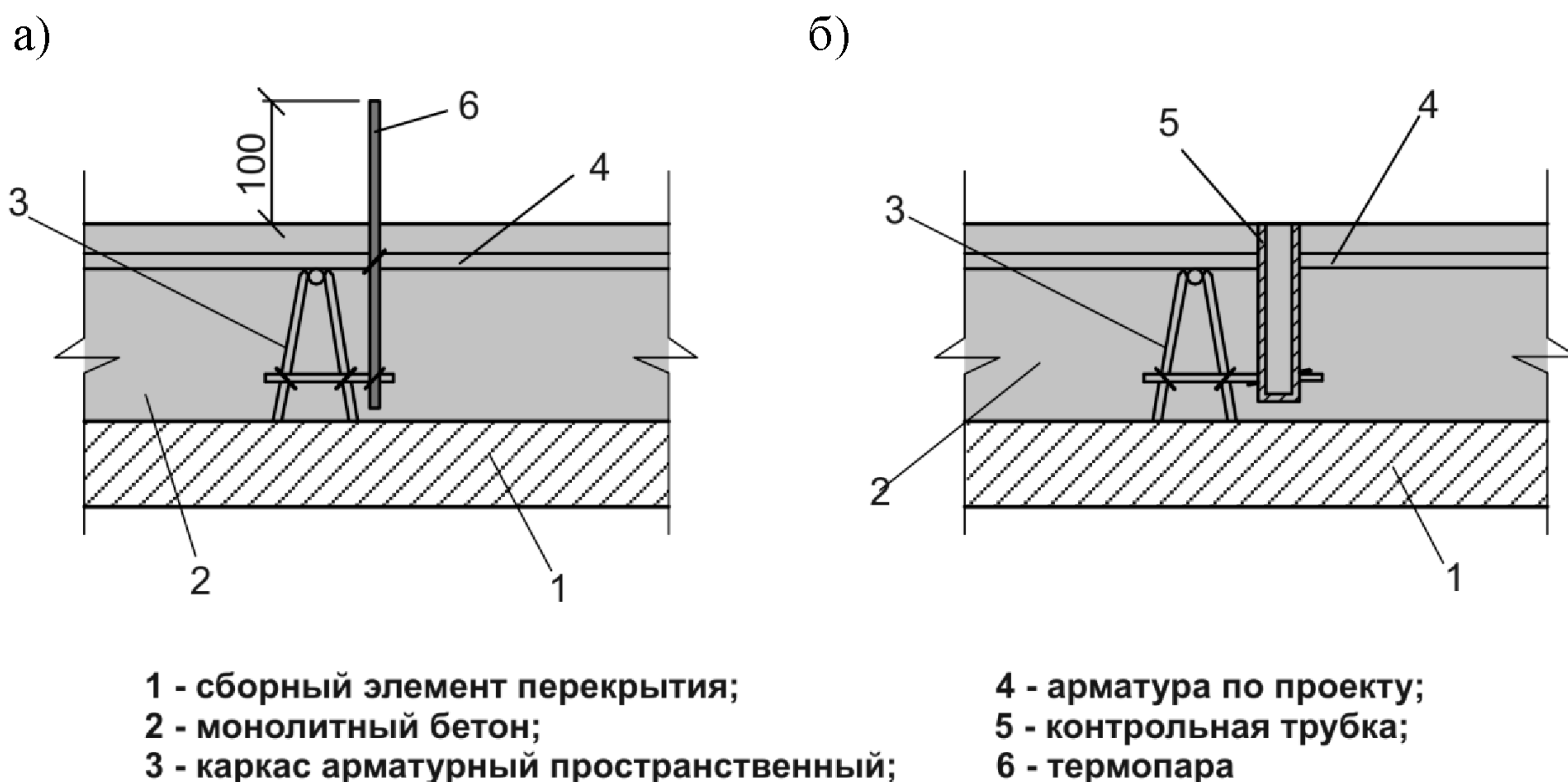
а) схема установки термопар; б) схема установки контрольных трубок
