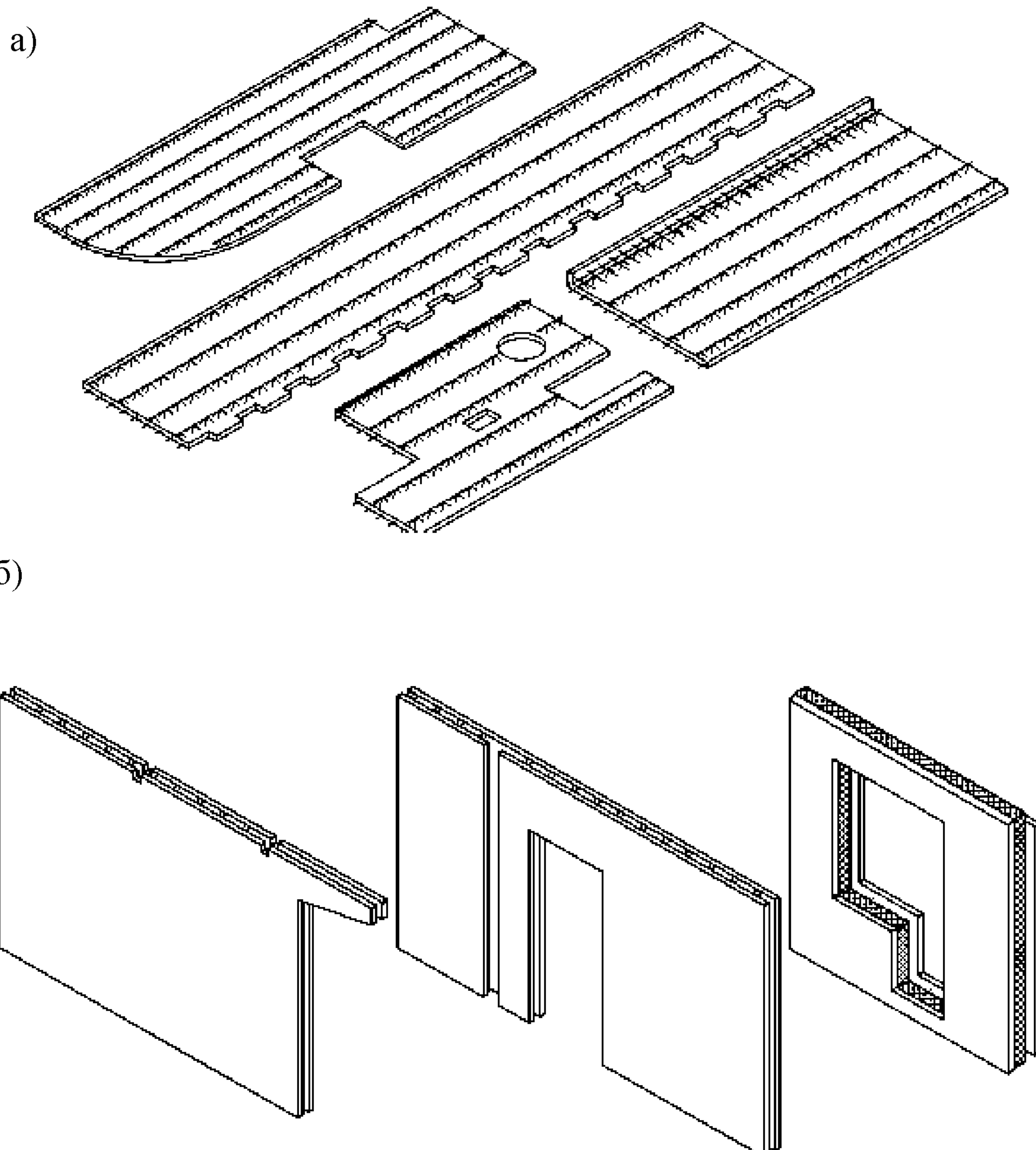
Рисунок 1 – Конструкция сборных железобетонных элементов несъемной опалубки перекрытия а), внутренних и наружных стен б)
