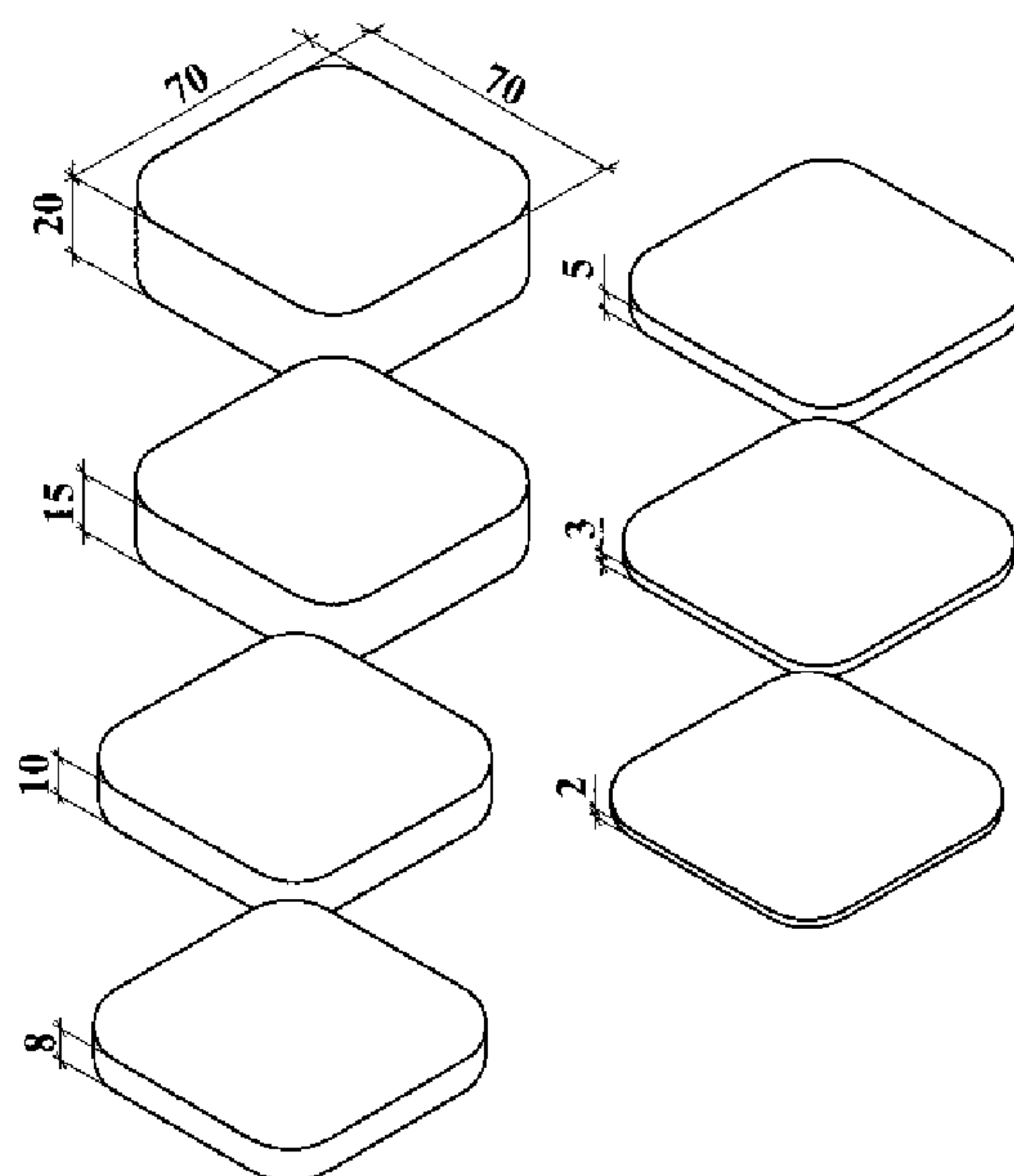
Рисунок 3 – Набор жестких профилей толщиной 2, 3, 5, 8, 10, 15, 20 мм для устройства маяков различной высоты
