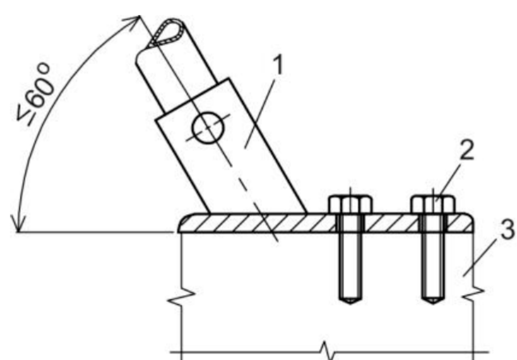
Рисунок Д.3 – Крепление монтажного подкоса стенового элемента к перекрытию
