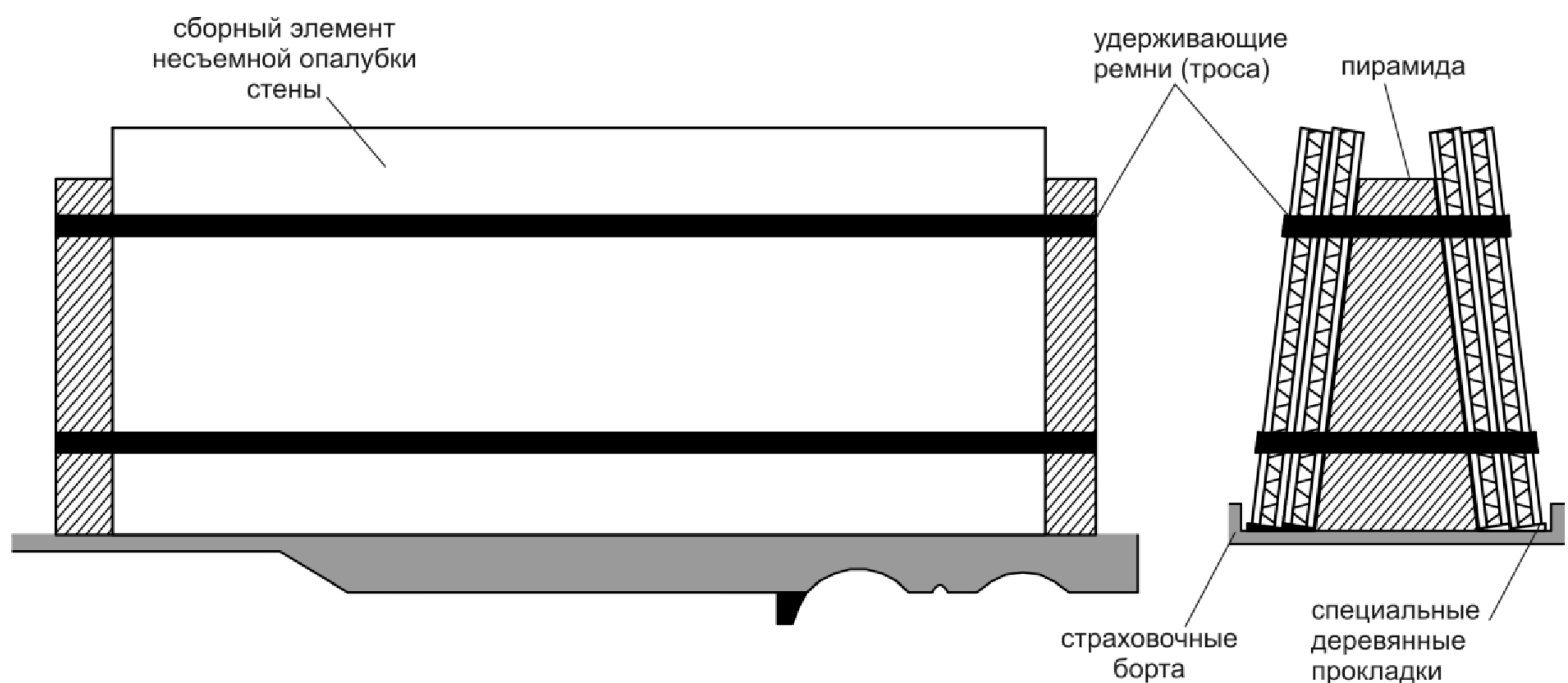
Рисунок А.3 – Схема укладки для перевозки сборных элементов несъемной опалубки стен в вертикальном положении
