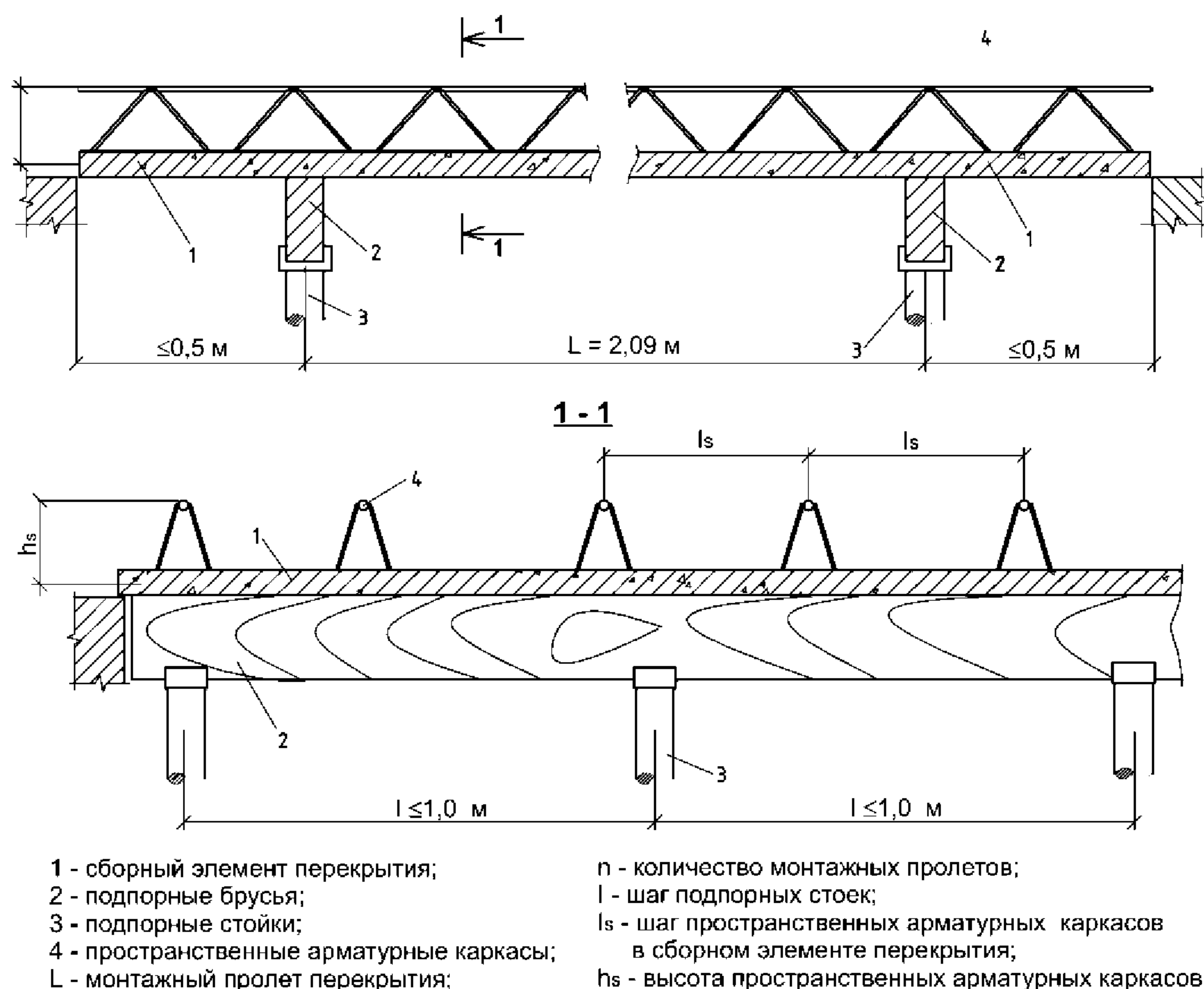
Рисунок 4 – Правила расстановки поддерживающих устройств перекрытий
