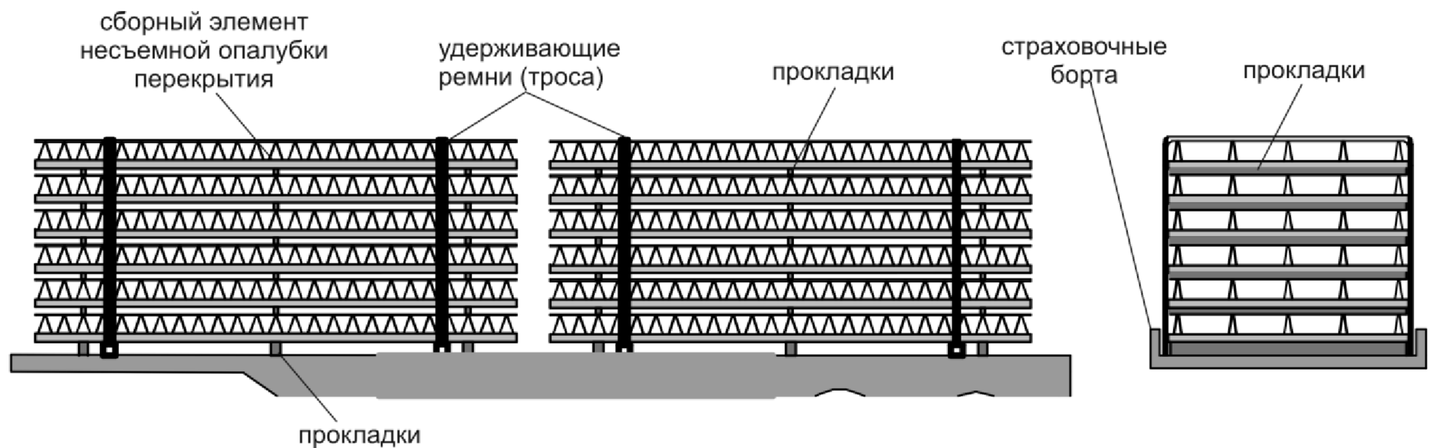
Рисунок А.1 – Схема укладки для перевозки сборных элементов несъемной опалубки перекрытий в горизонтальном положении
