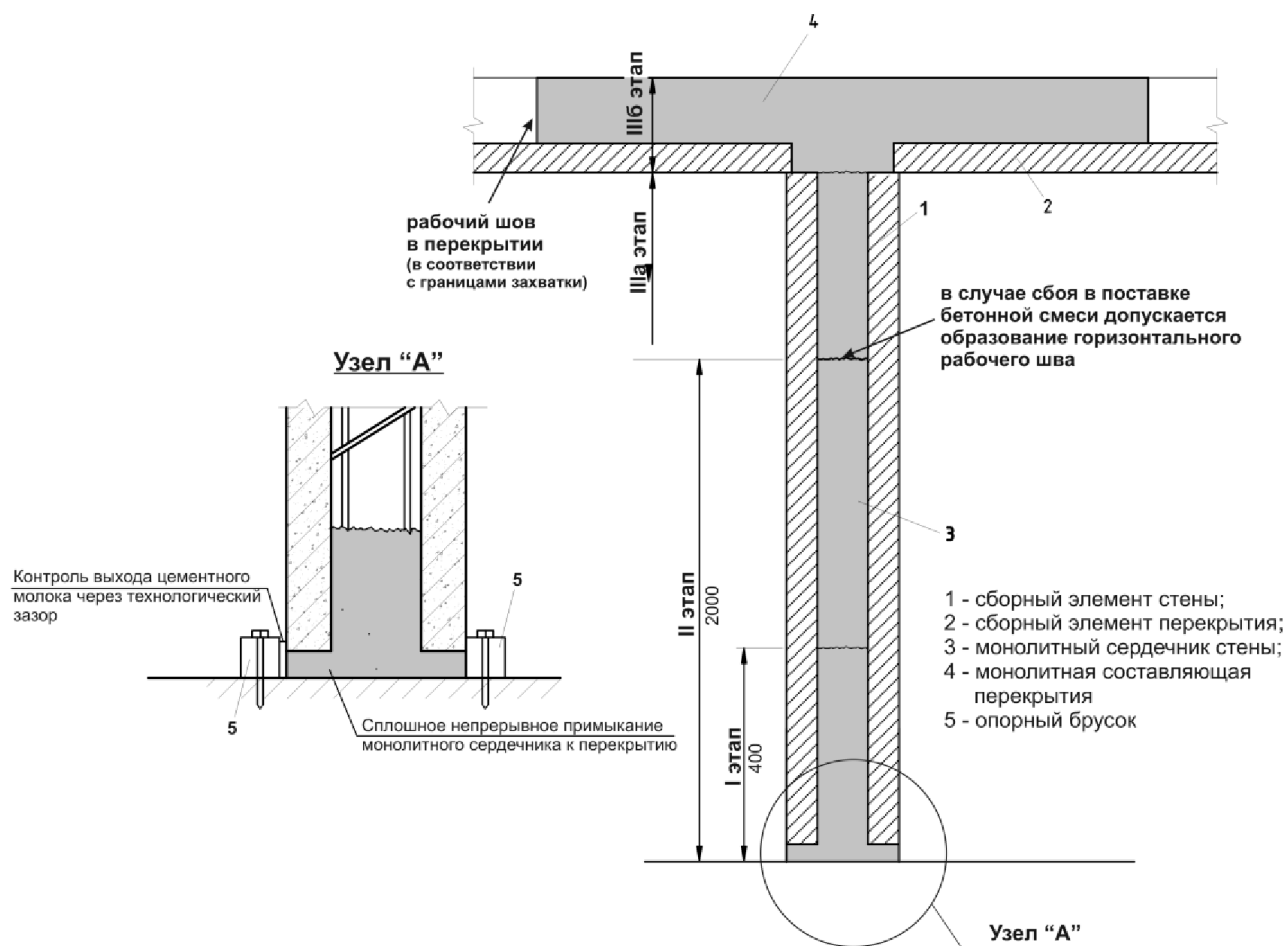
Рисунок 8 – Этапы бетонирования сердечника стены
