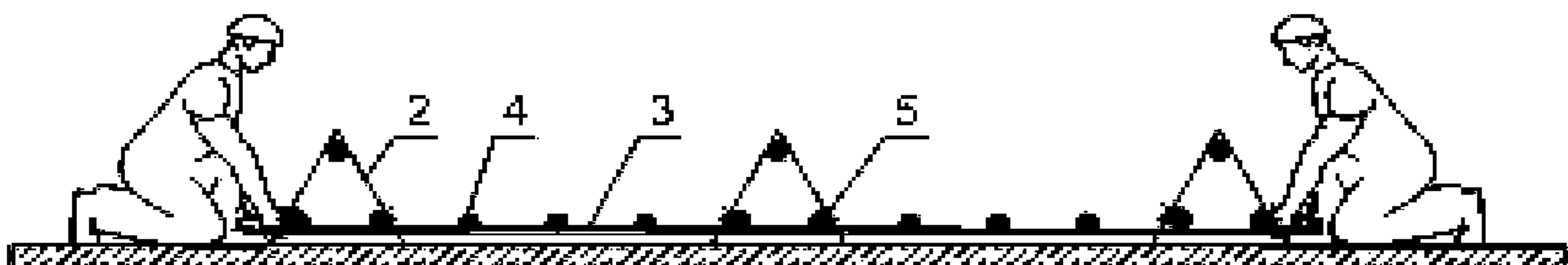
Установка каркасов поддерживающих верхнюю сетку
