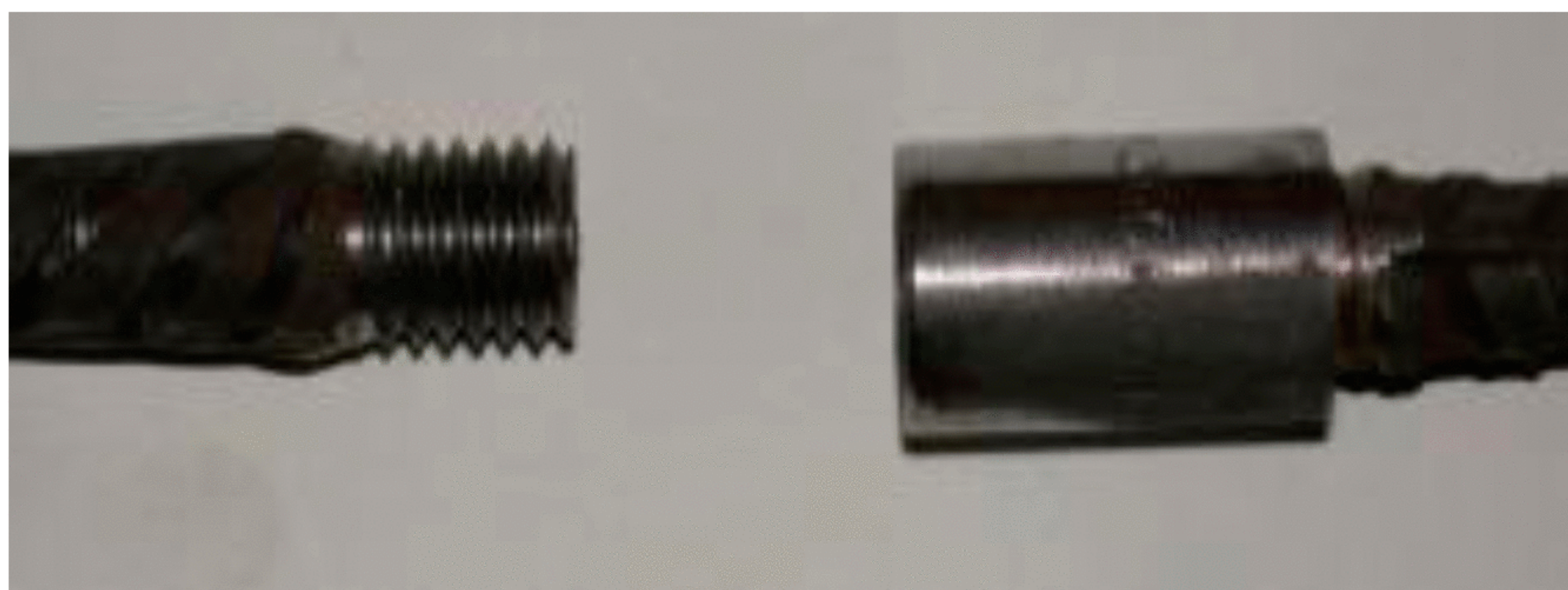
а) - переходное соединение с конической резьбой
