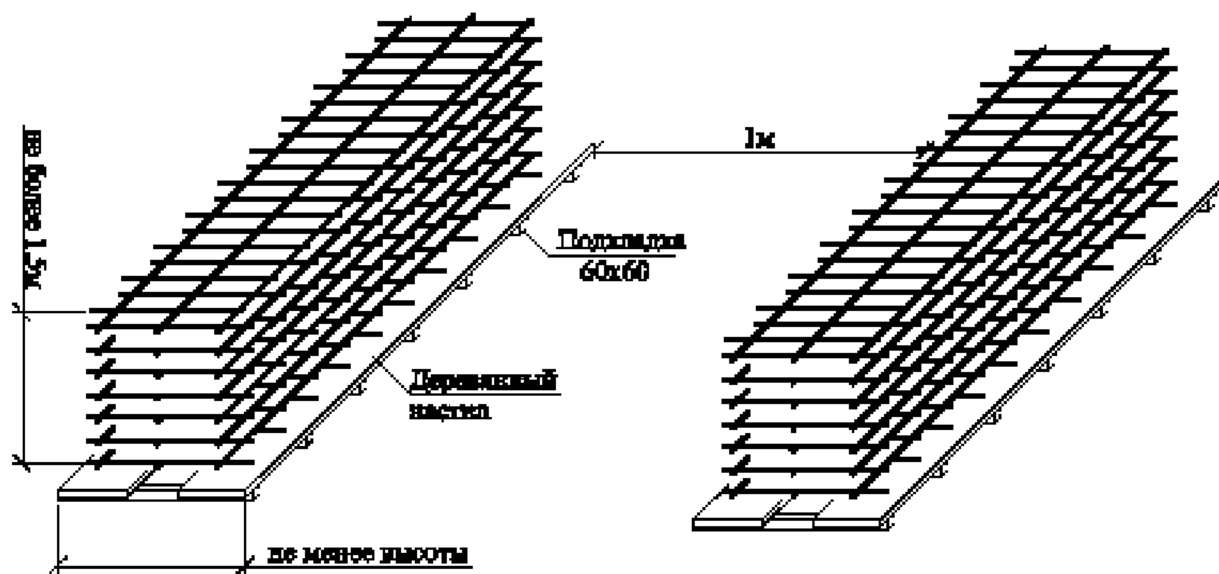
Рисунок Л.1 - Складирование пакета плоских сеток
