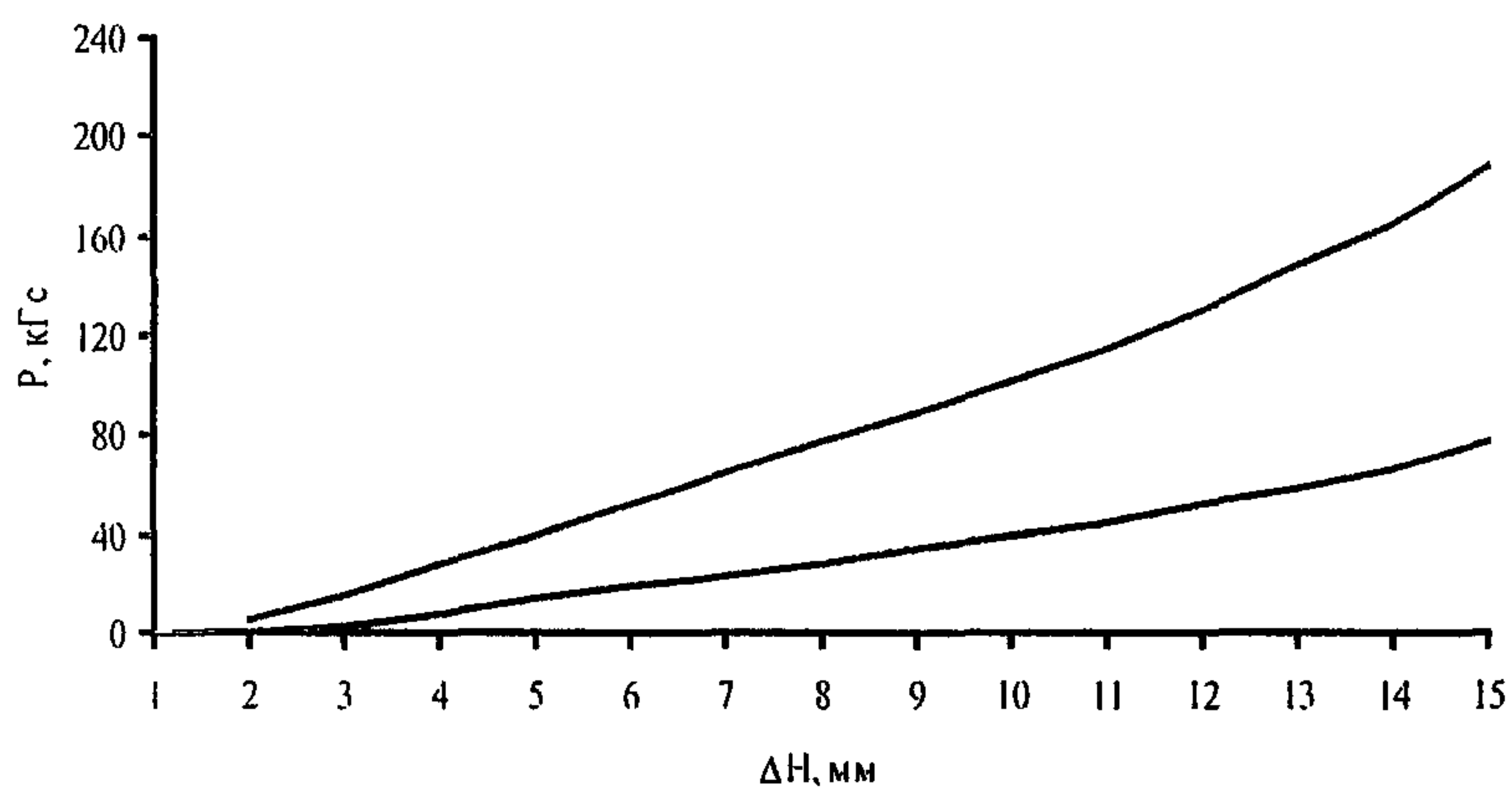
Нормативная диаграмма действительного напряжения сжатия покладки спинки
