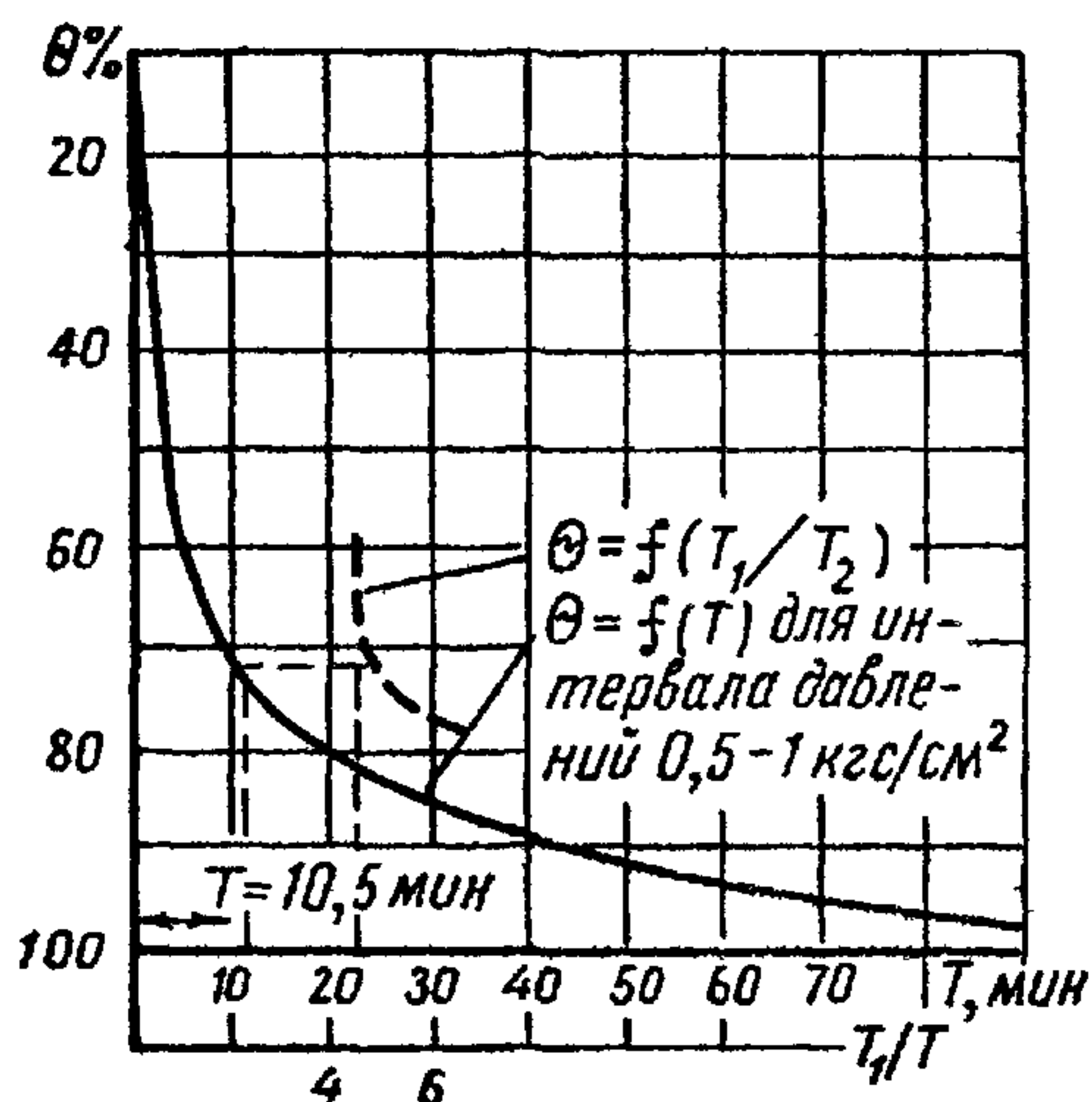
Рис. 15. Кривая консолидации
