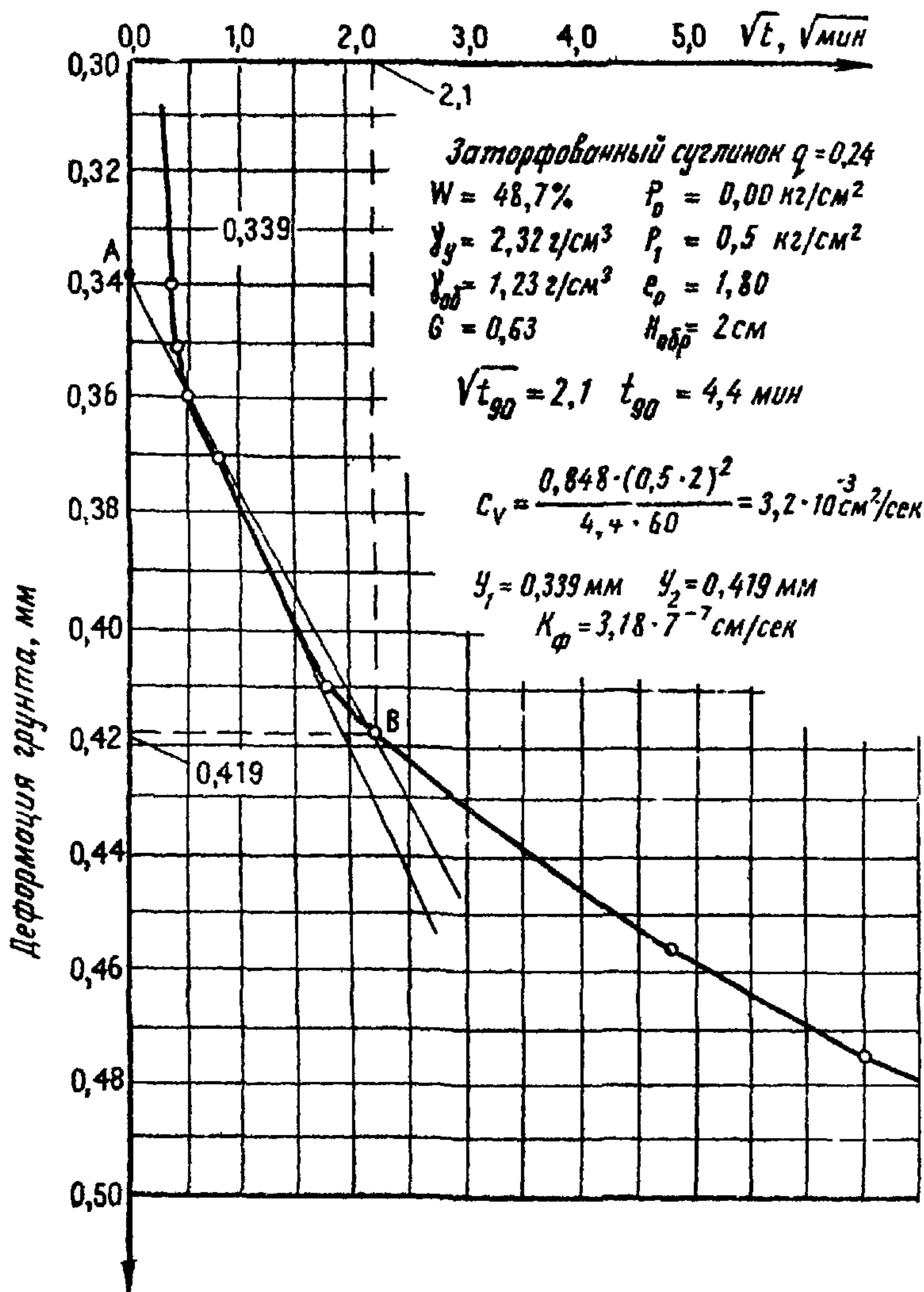
Рис.18. Кривая консолидации к методу определения коэффициента консолидации C_v и коэффициента начальной фильтрации K_{\text{ф}} .
