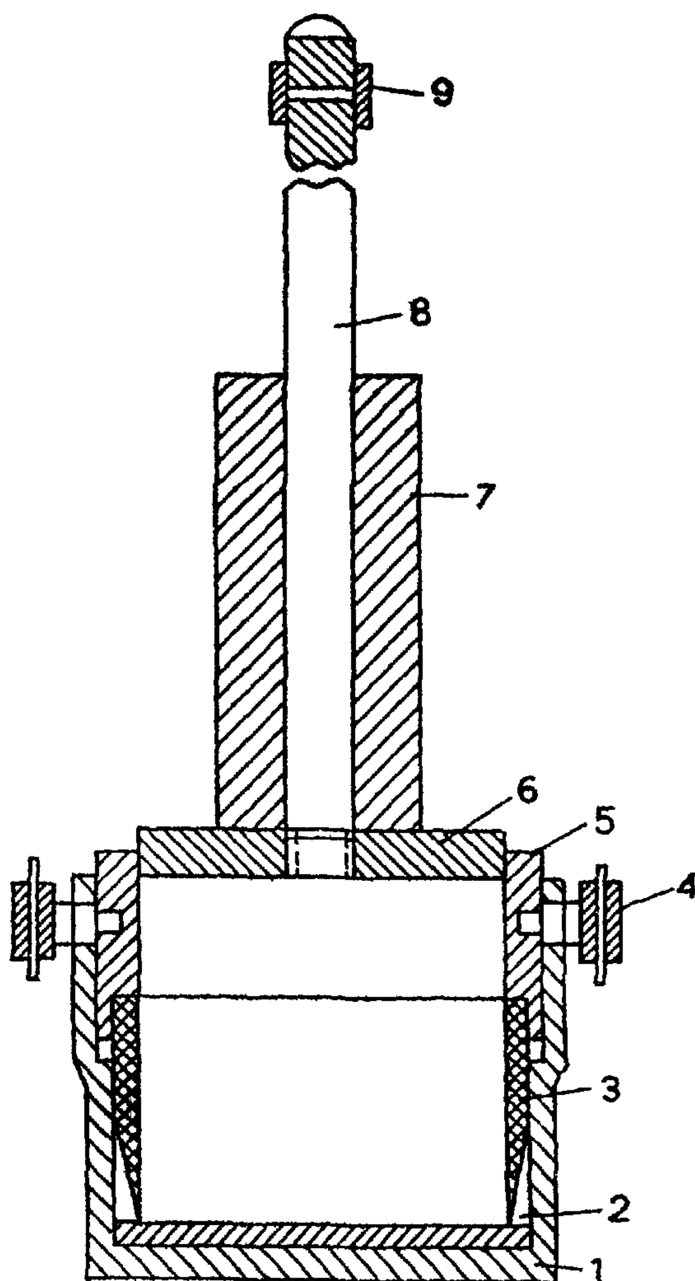
Рис. 8 Прибор ЦНИИС для стандартного уплотнения
