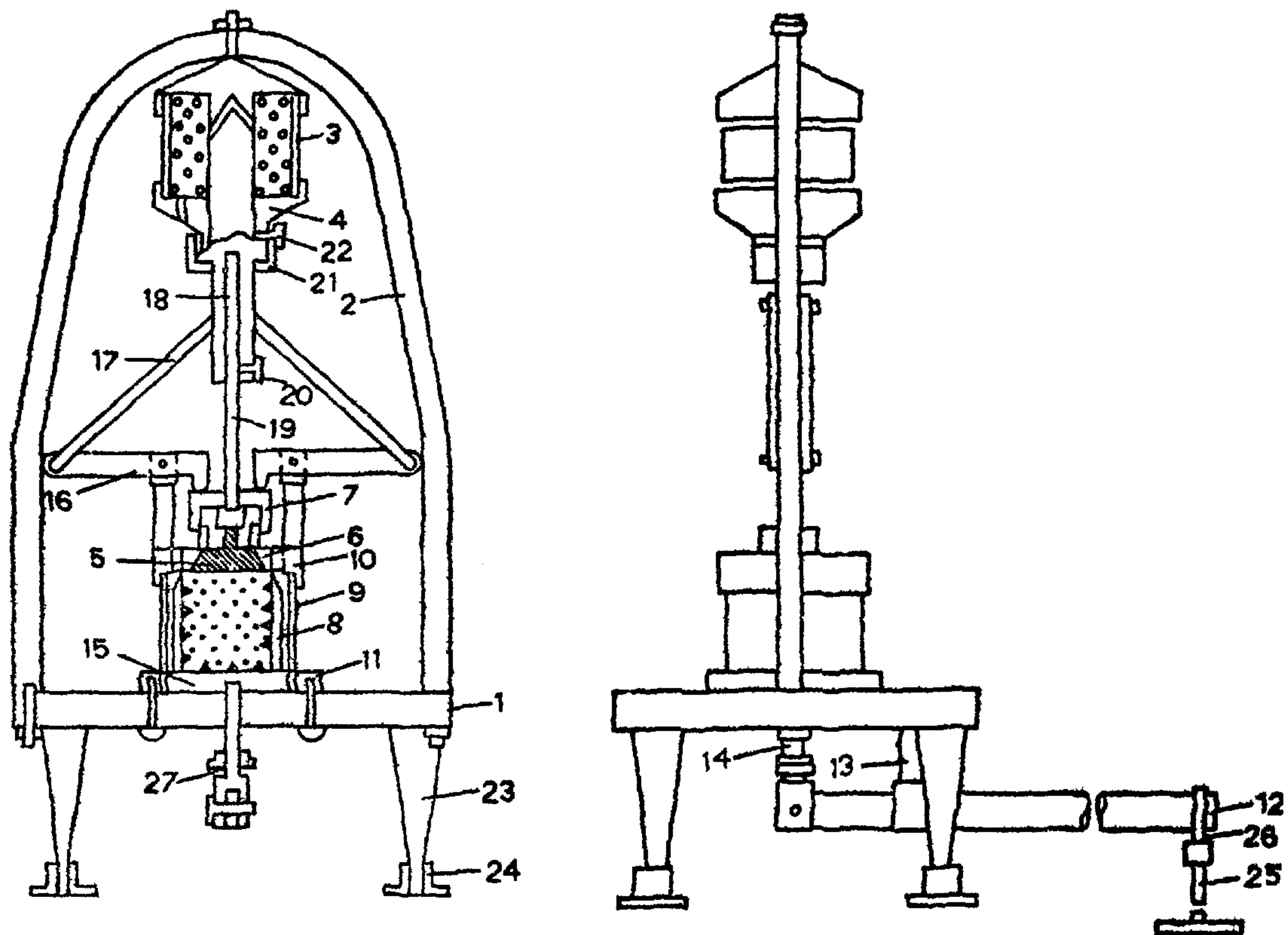
Рис. 16. Прибор (устройство) для измерения липкости почв и грунтов - УИЛ-2
