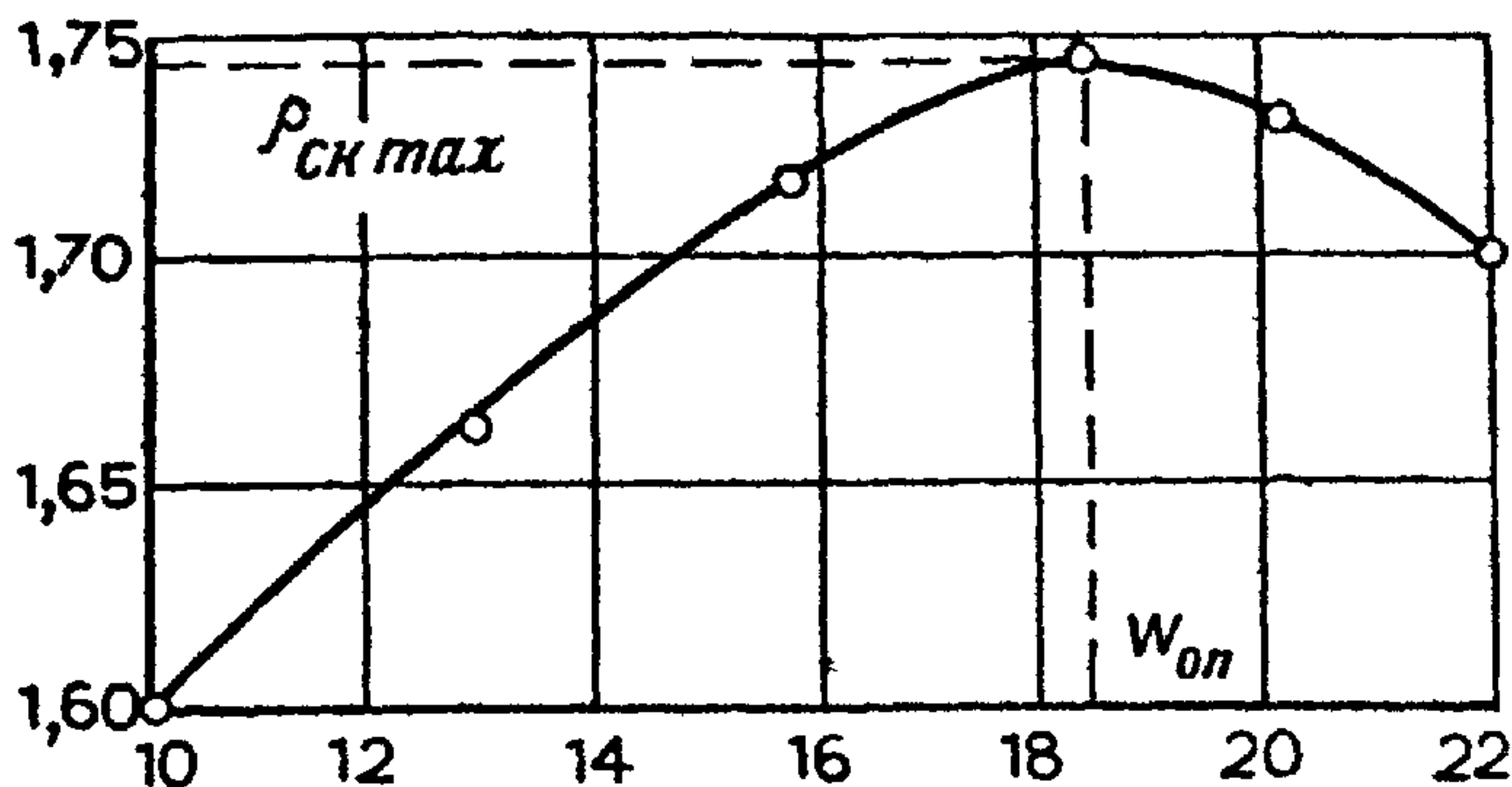
Рис. 9. Кривая стандартного уплотнения
