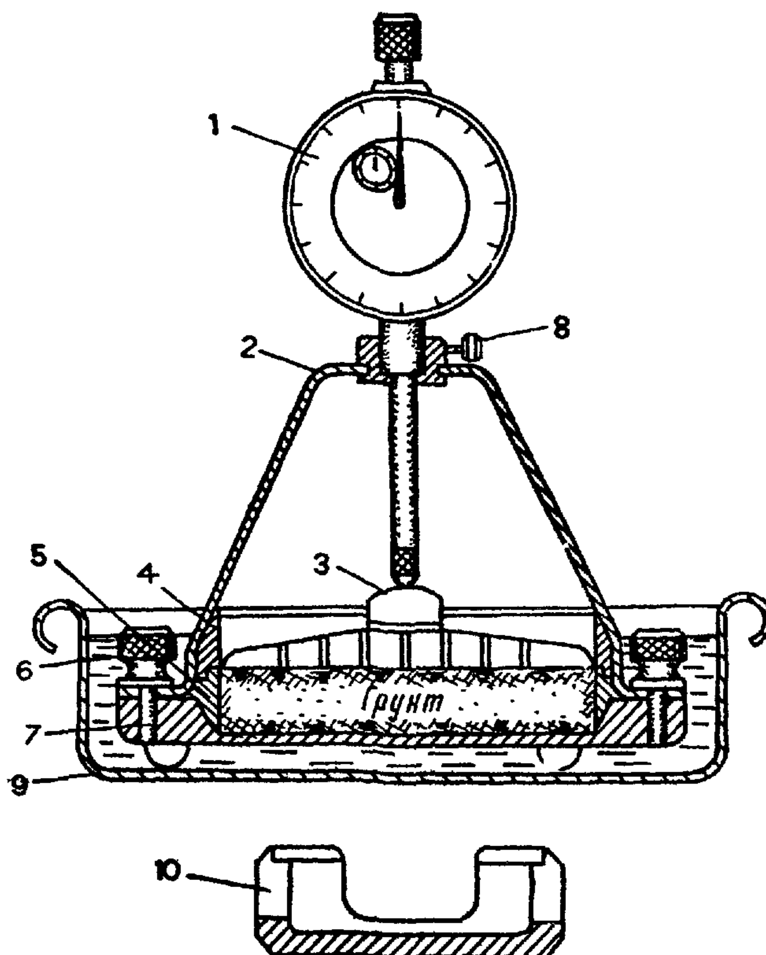
Рис. 11. Прибор для определения набухания грунтов ПНГ
