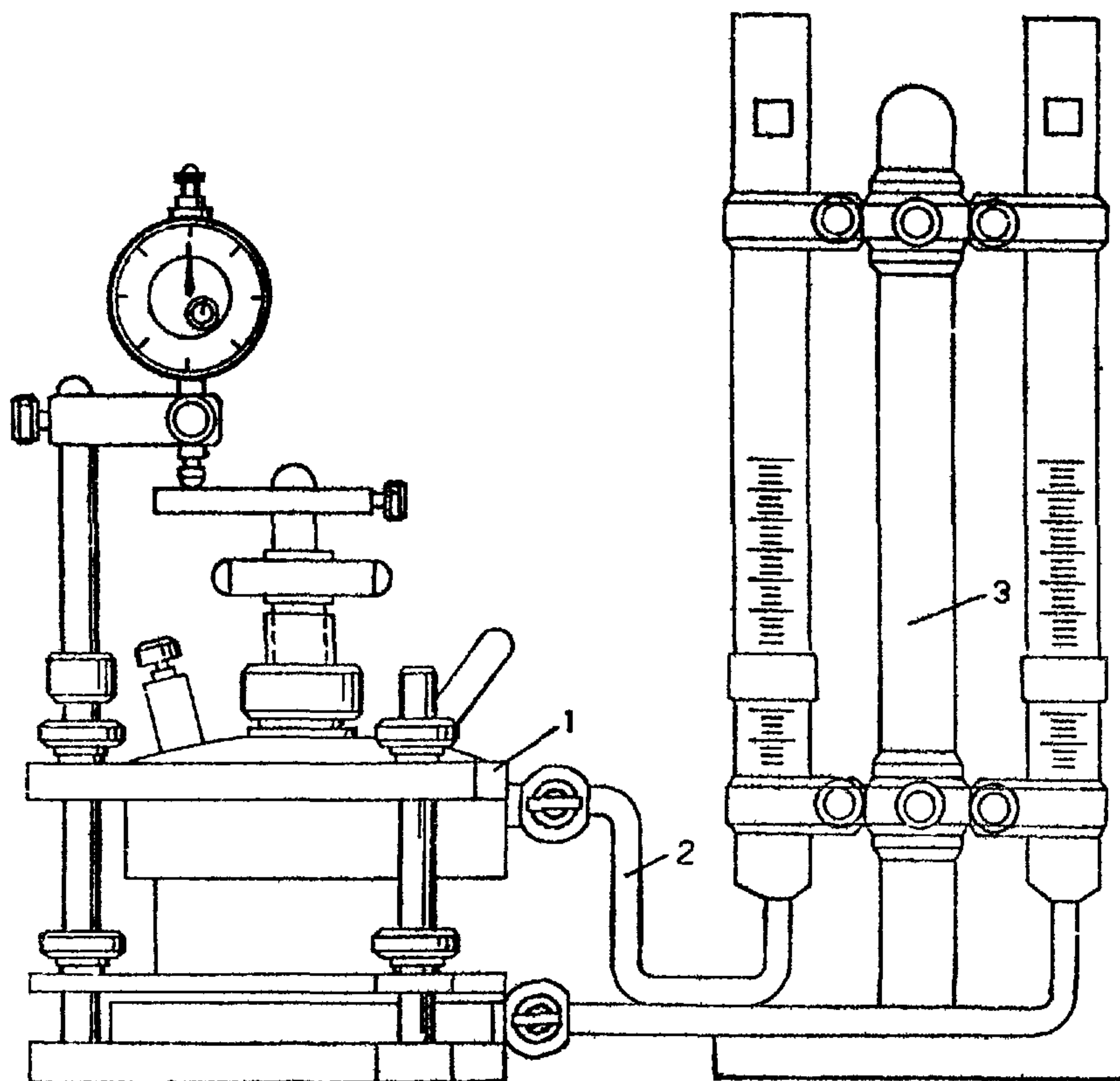
Рис. 14. Фильтрационный прибор Ф-1М 1 - одомер; 2 - подводящие трубки; 3 - пьезометр
