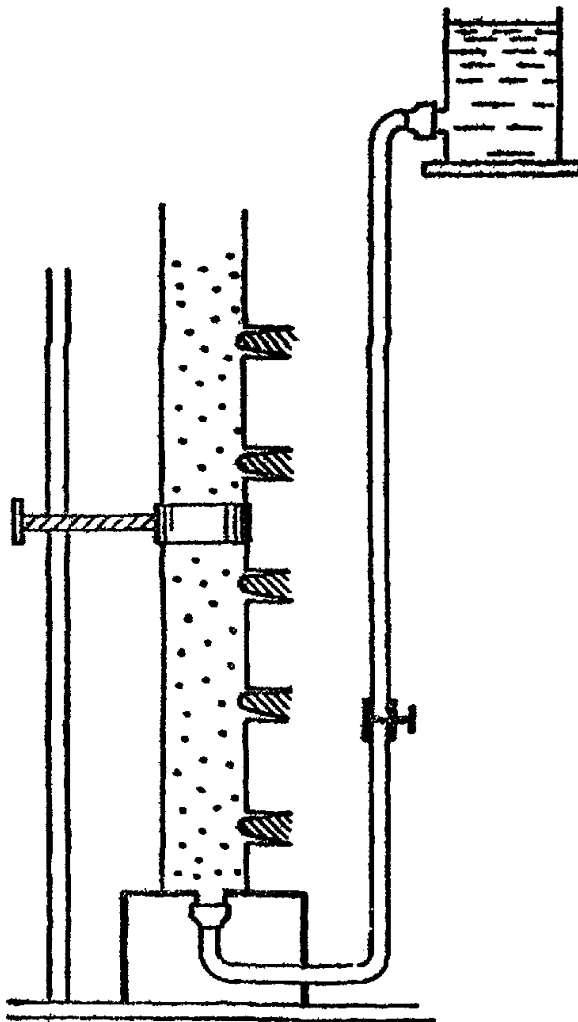
Рис. 12. Прибор для определения максимальной молекулярной влагоемкости песков
