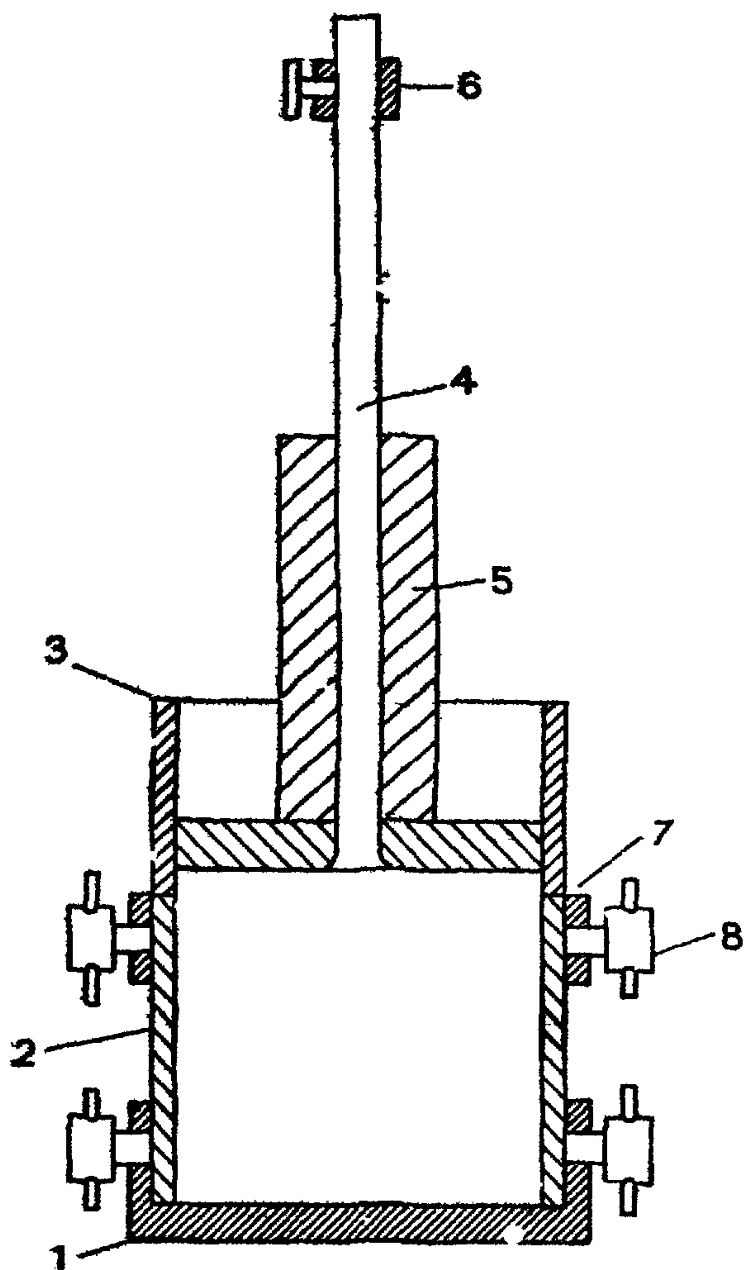
Рис. 7. Прибор СоюздорНИИ для стандартного уплотнения
