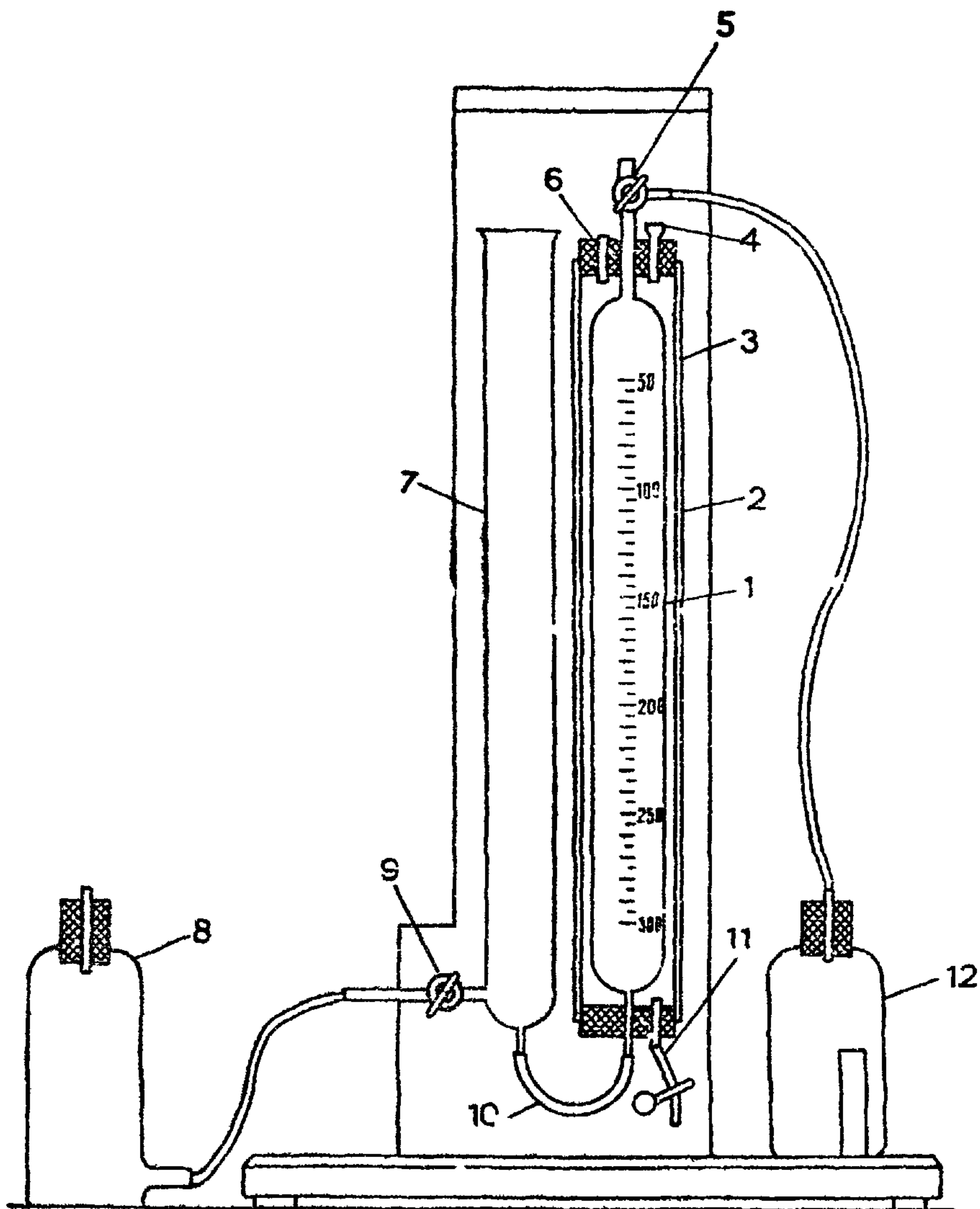
Рис. 5. Кальциметр
