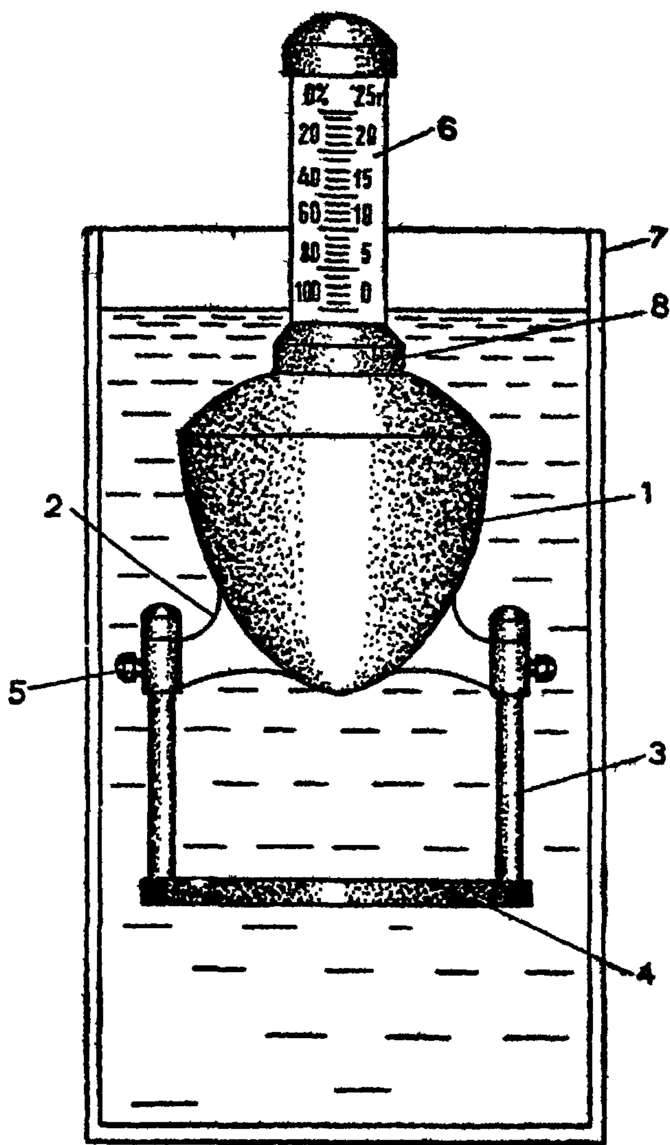
Рис. 10. Прибор ПРГ для определения размокаемости
