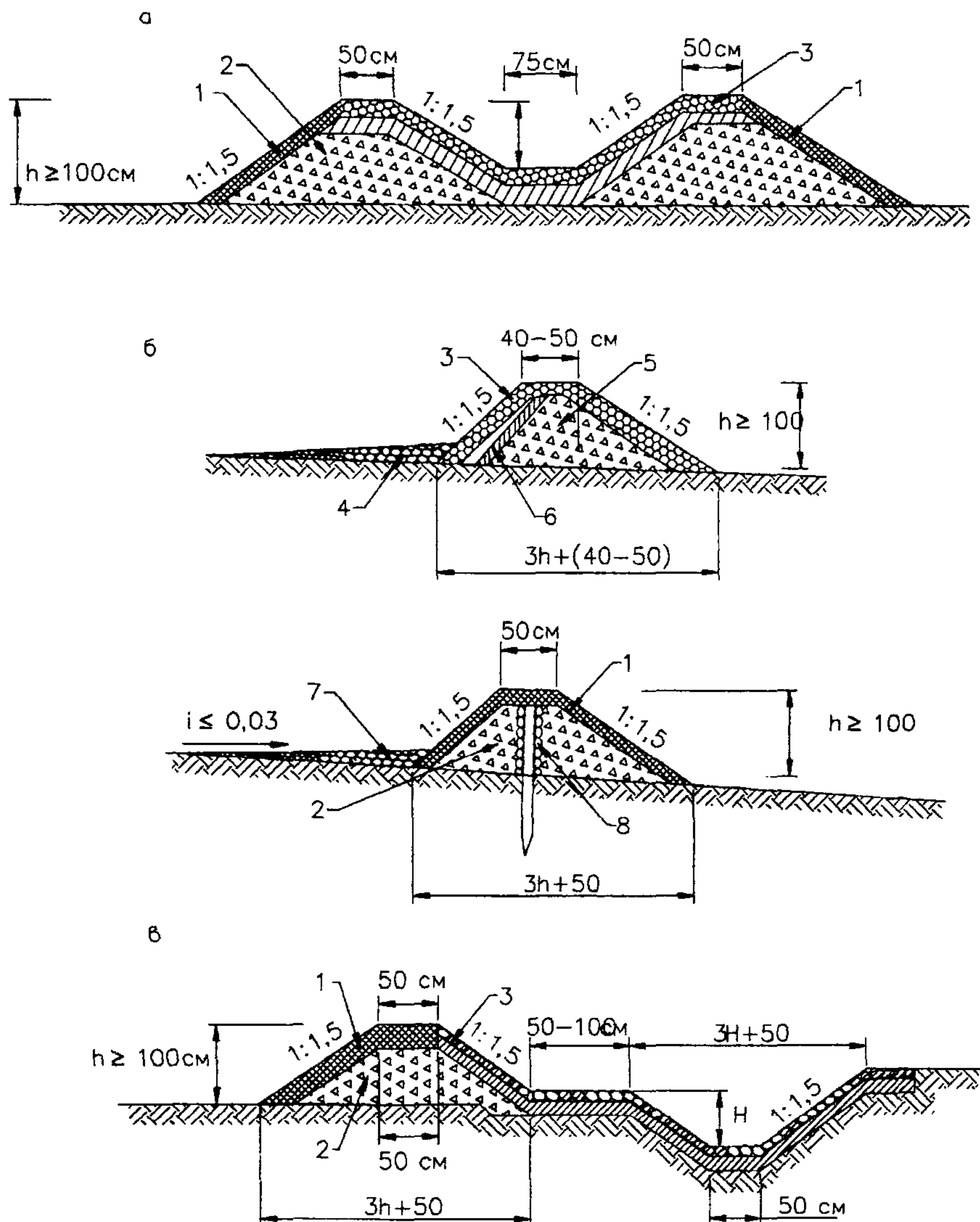
Рисунок 23 Конструкции элементов водоотводных сетей на вечномёрзлых грунтах:
