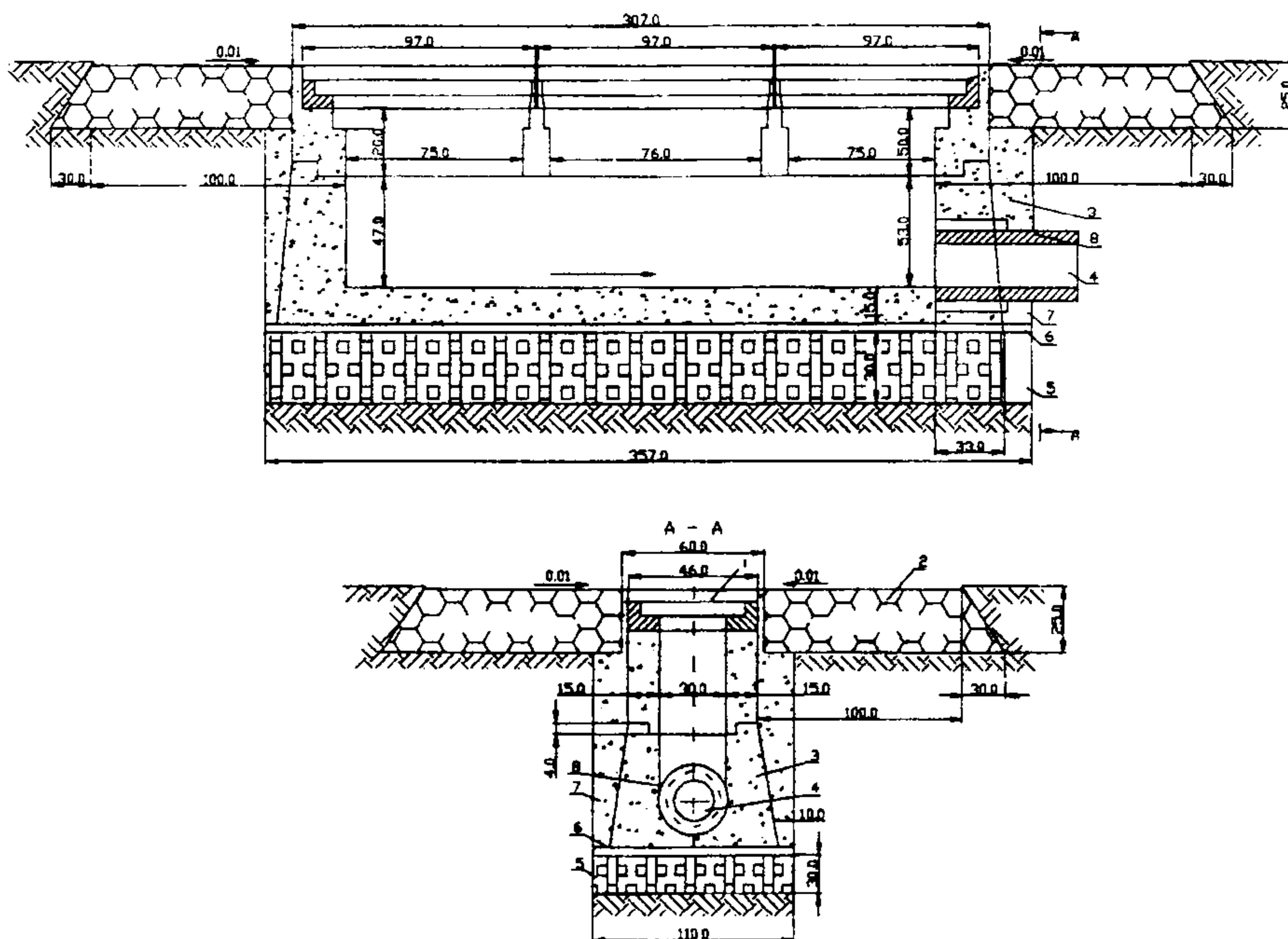
Рисунок 8 Конструкция тальвежного колодца
