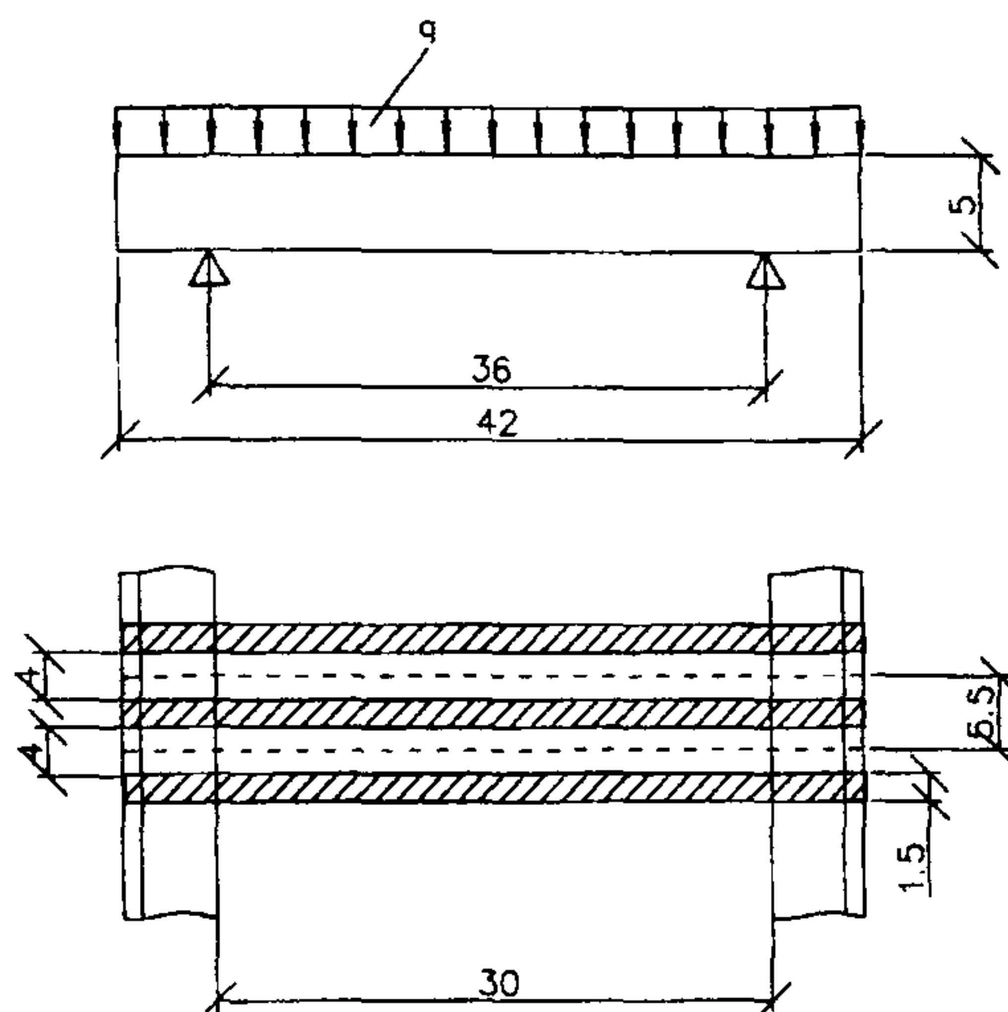
Рисунок Б.2 Расчет металлической решетки дождеприемного колодца.
