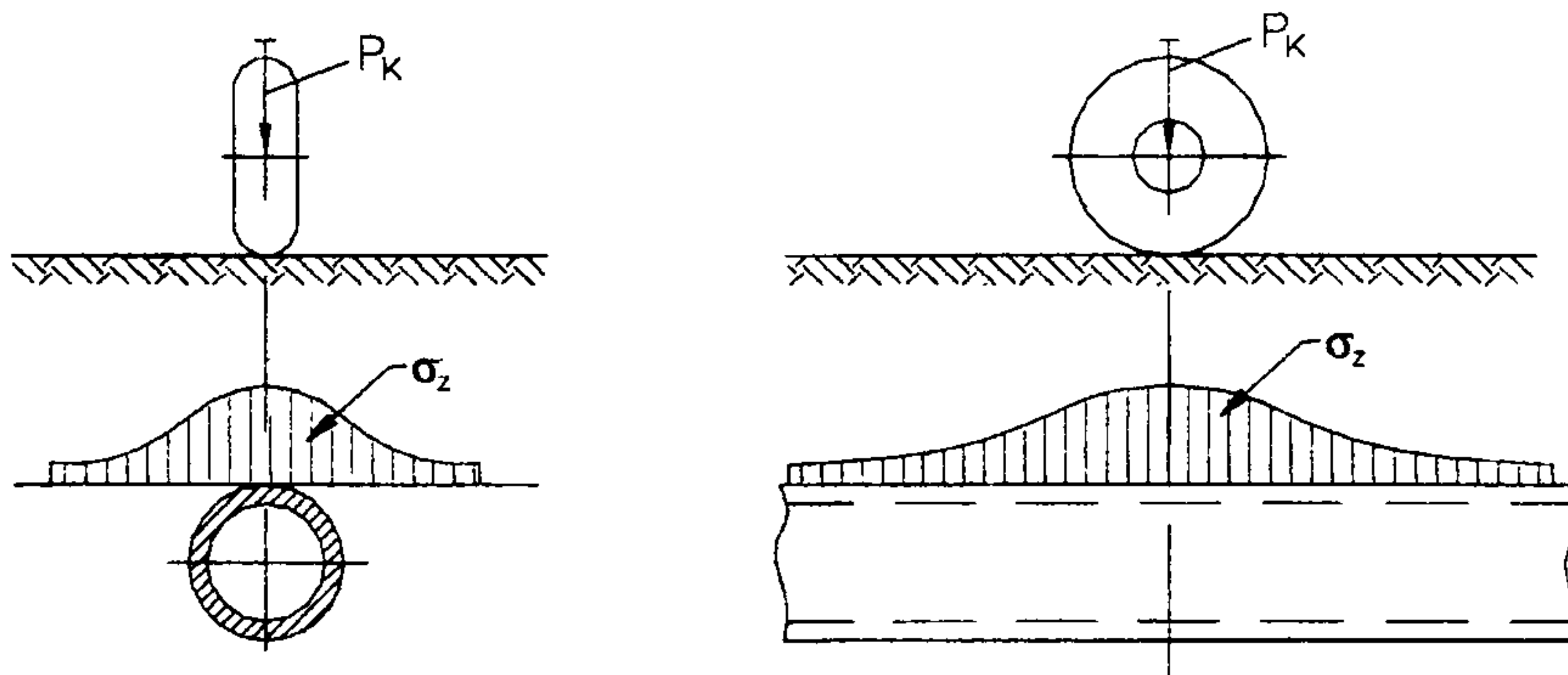
Рисунок 16 Схема к определению давления на трубу
