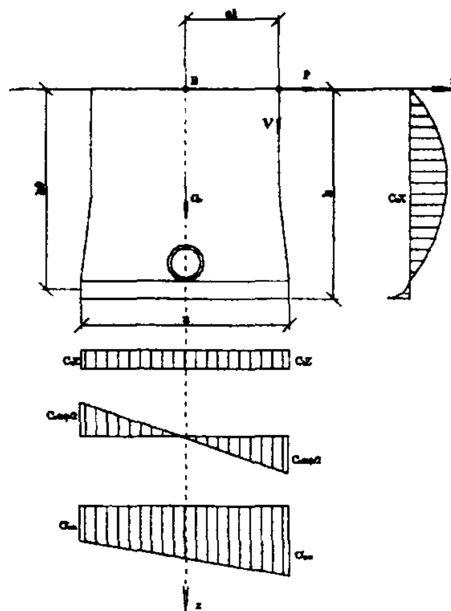
Рисунок 20. Расчет перемещений колодца в вертикальном и горизонтальном
