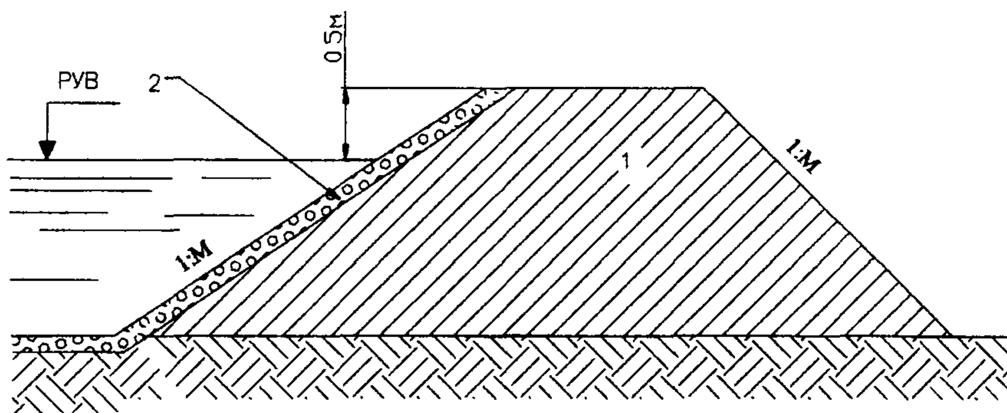
Рисунок 2 Поперечное сечение дамбы 1 – грунт; 2 – крепление откоса; ПУВ – расчетный уровень воды
