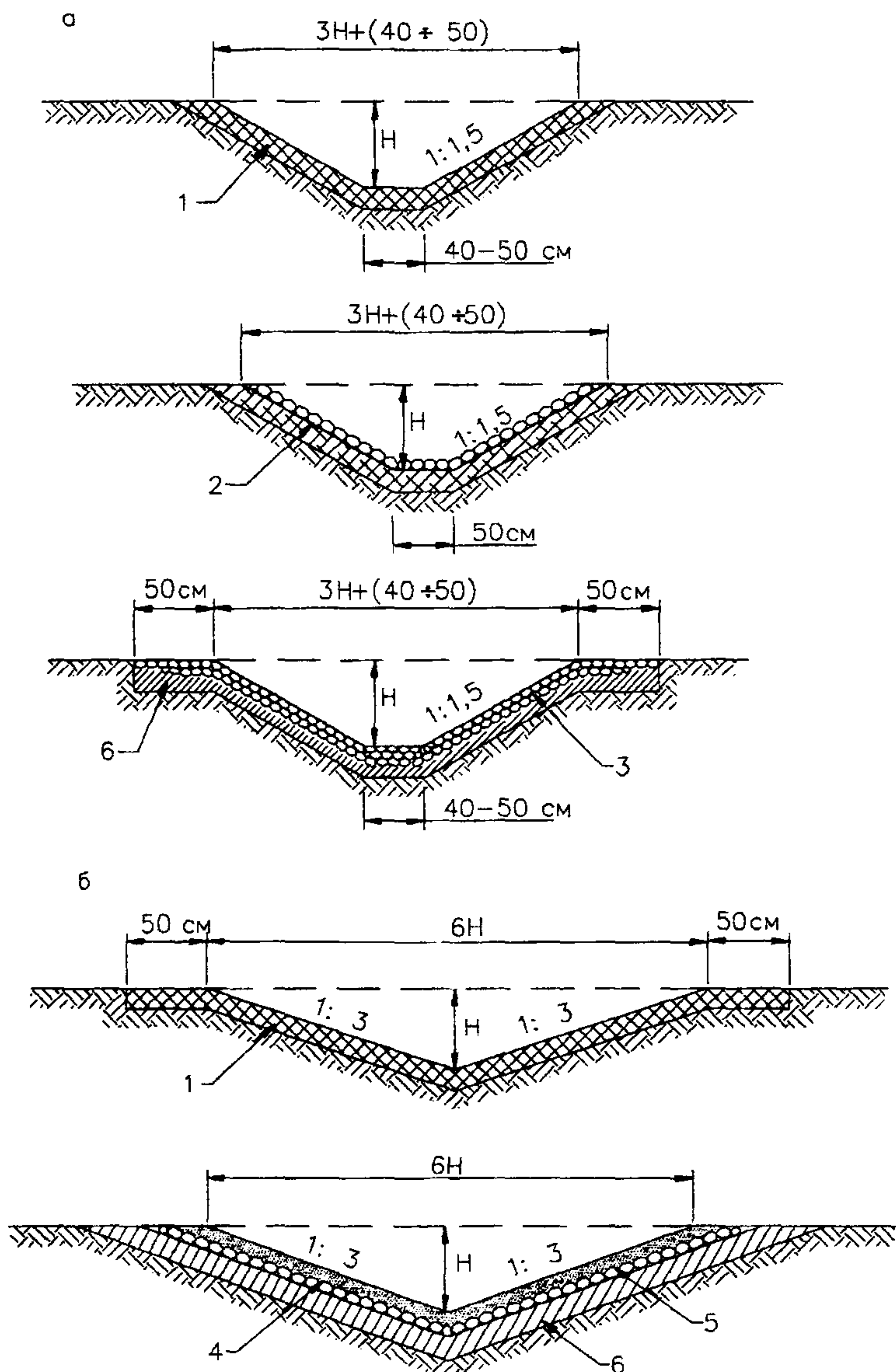
Рисунок 22 Конструкции элементов водоотводных сетей на вечномерзлых грунтах:
