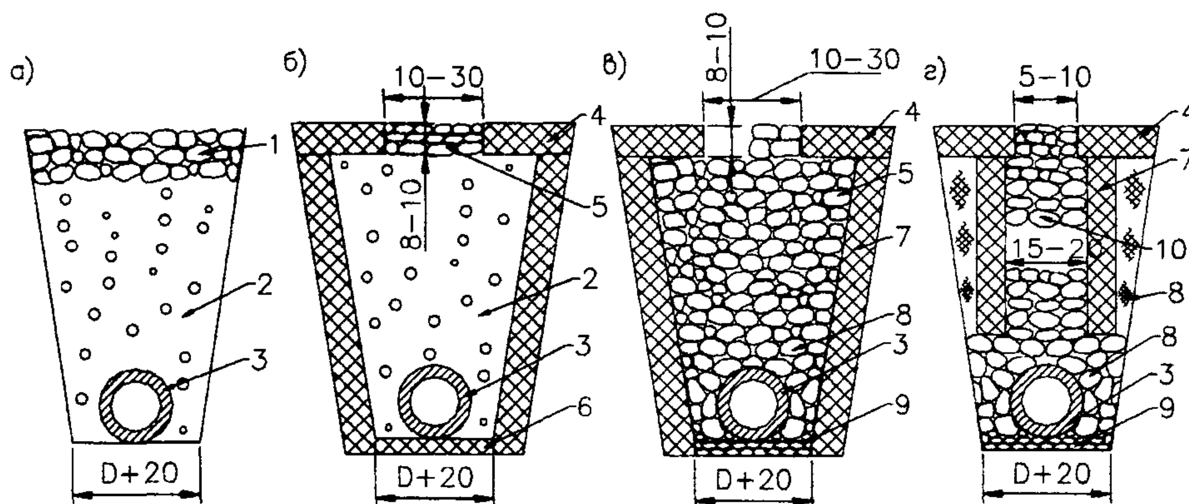
Рисунок 13 Конструкции осушителей:
