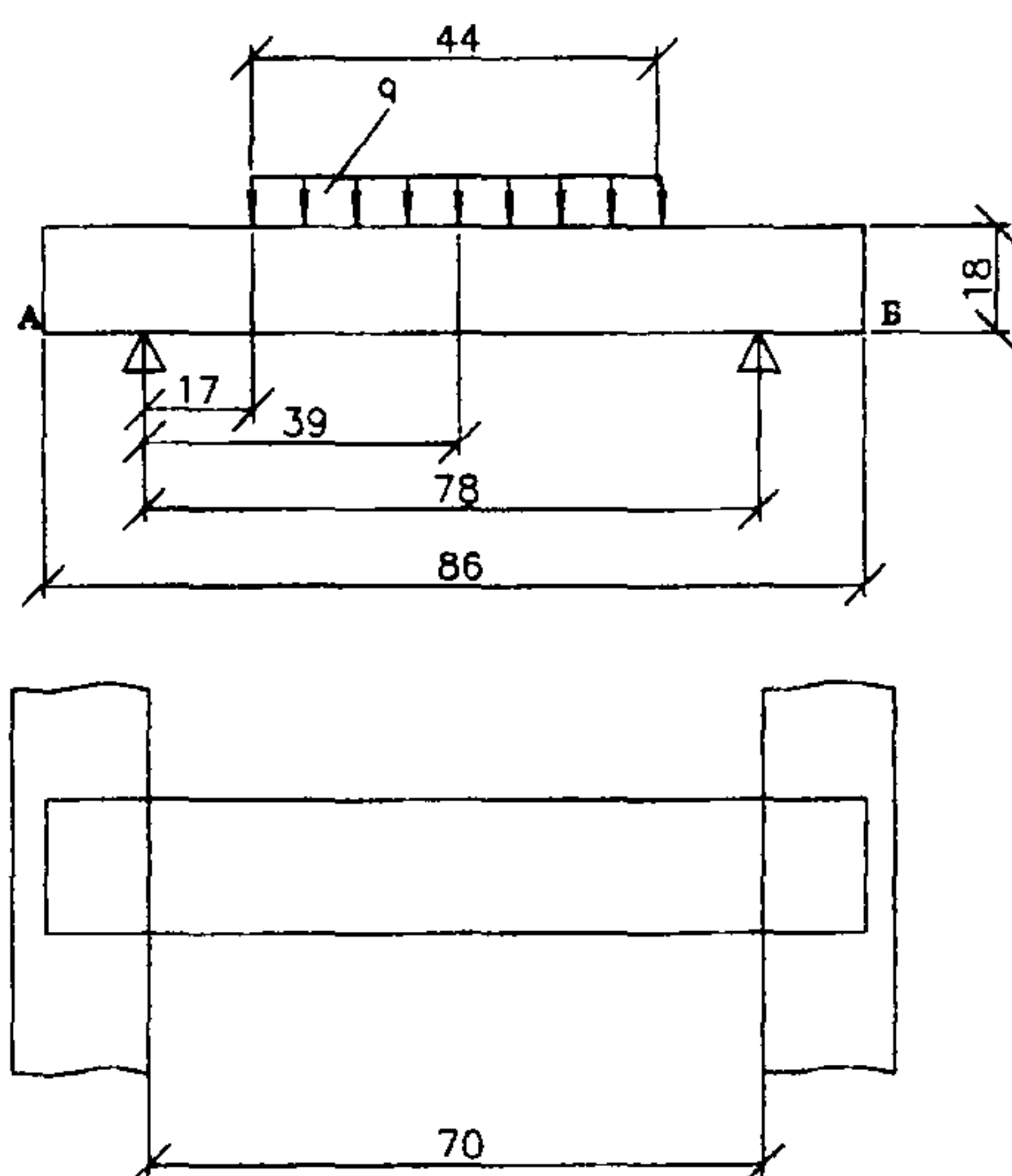
Рисунок Б.3 Расчет балочек крышки смотрового колодца
