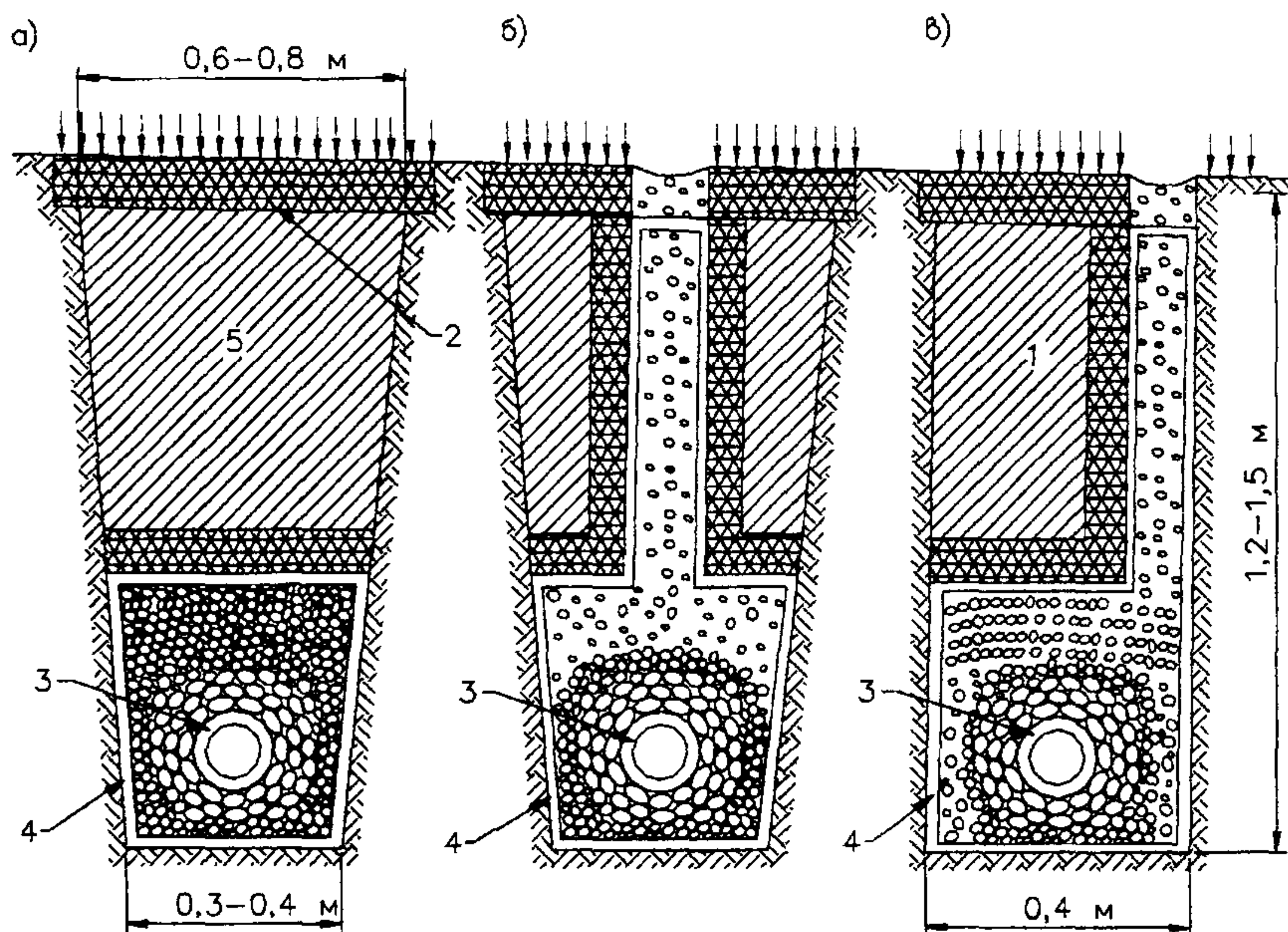
Рисунок 14 Конструкция дрена
