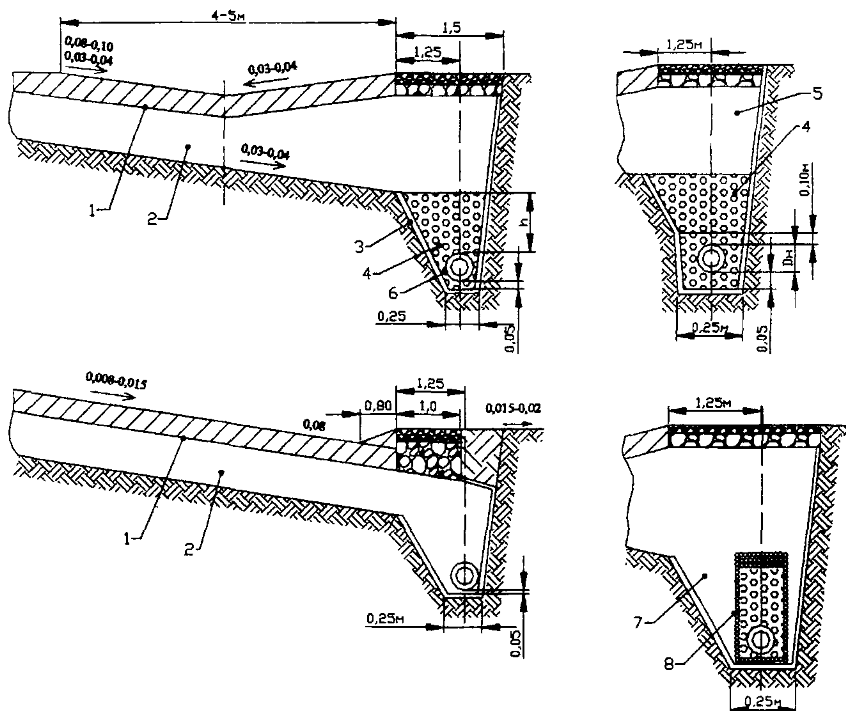
Рисунок 9 Варианты конструкций закомочных дрен
