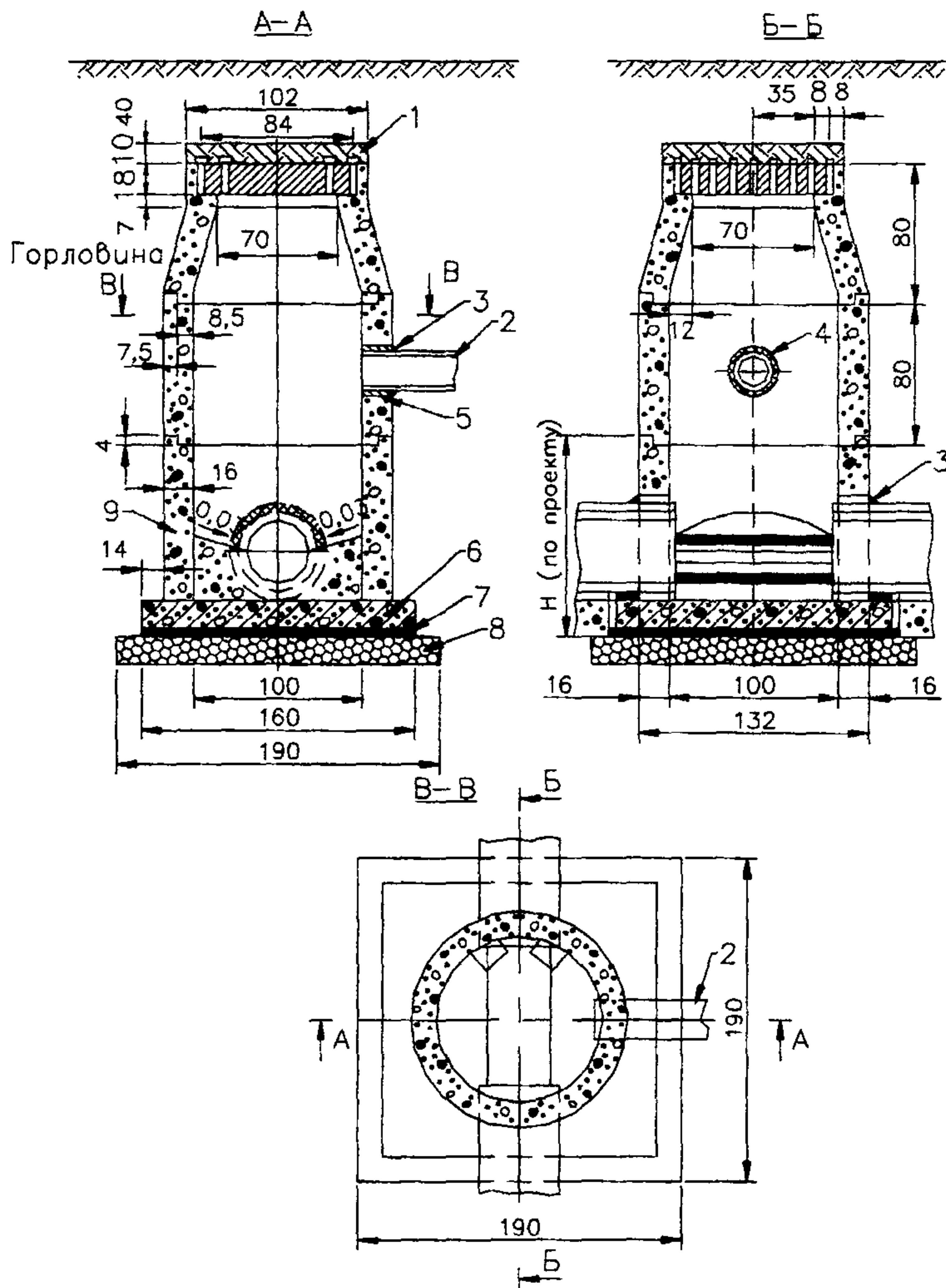
Рисунок 11. Круглый смотровой колодец (сборный из железобетонных звеньев):
