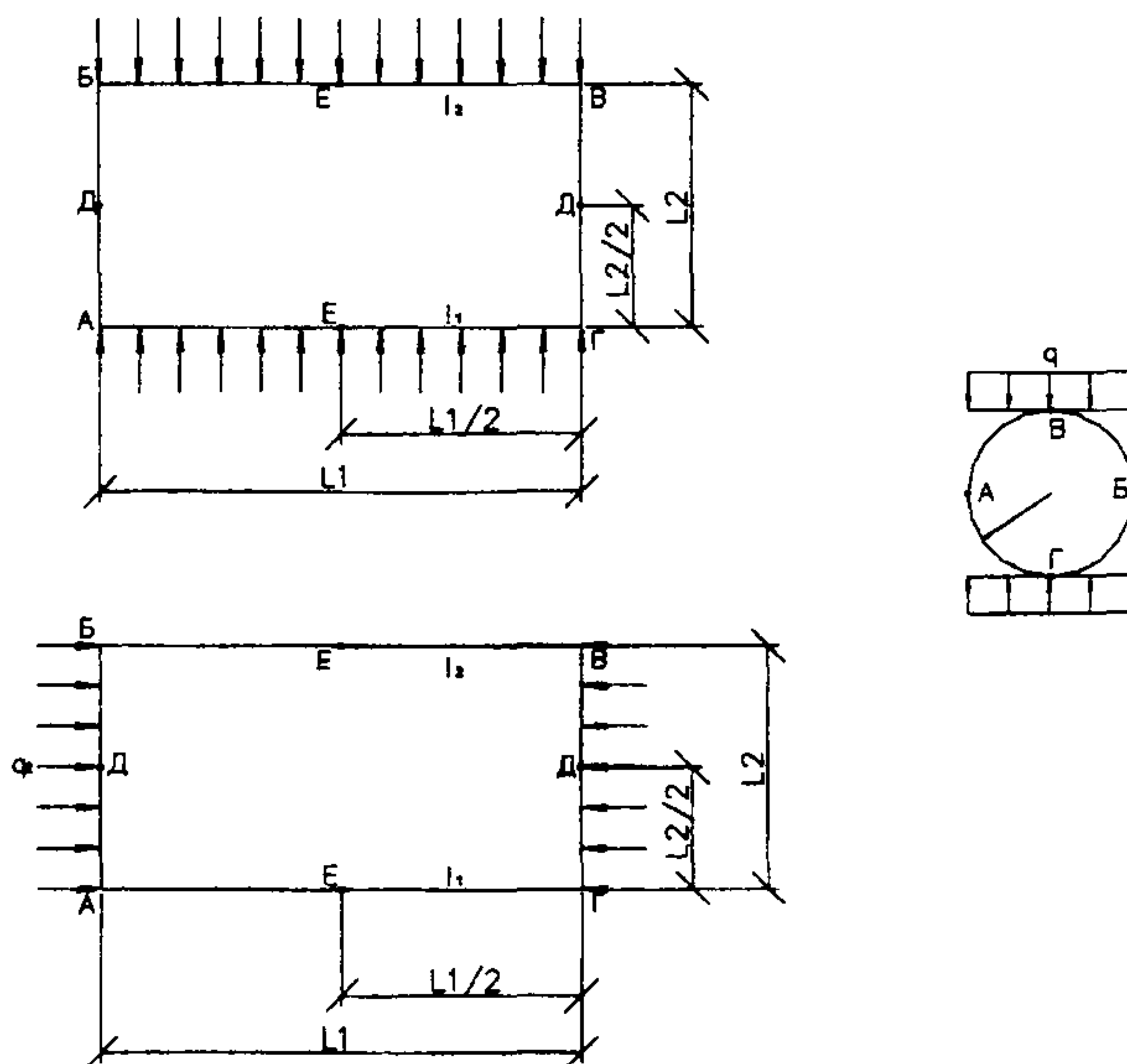
Рисунок 19 Расчет стенок прямоугольных и круглых колодцев:
