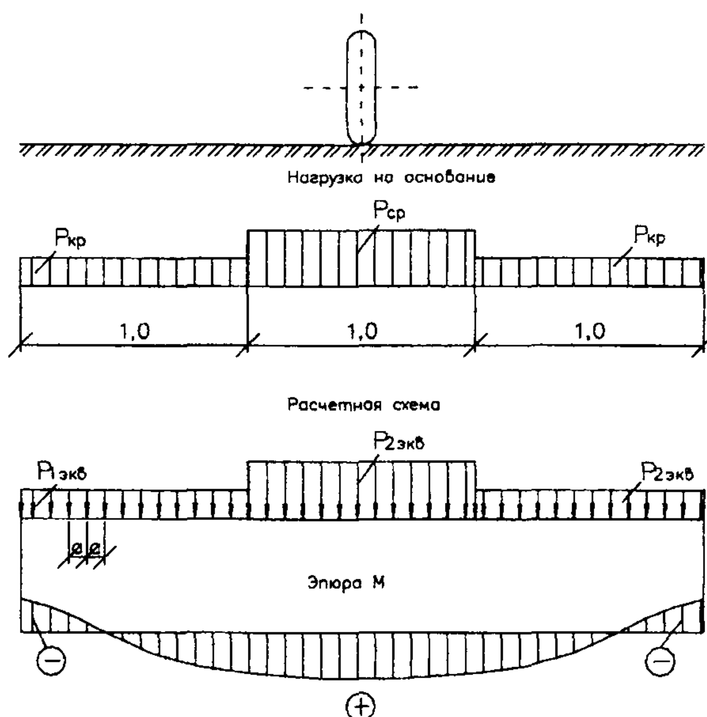
Рисунок 18 Расчет оснований под трубы.
