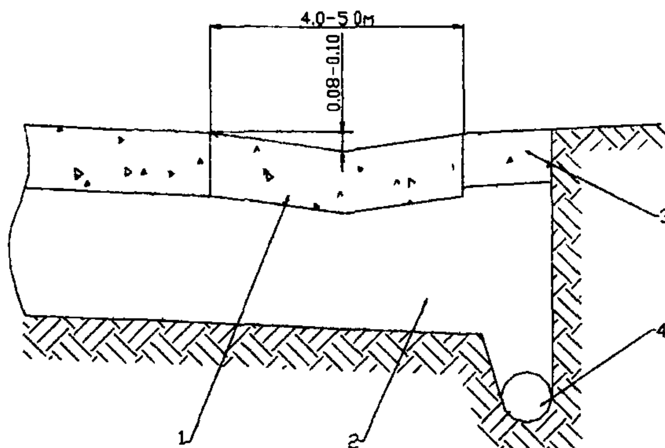
Рисунок 6 Конструкция открытого лотка на ИВПП 1 – покрытие; 2 – основание; 3 – отсостка; 4 – закрочная дрена
