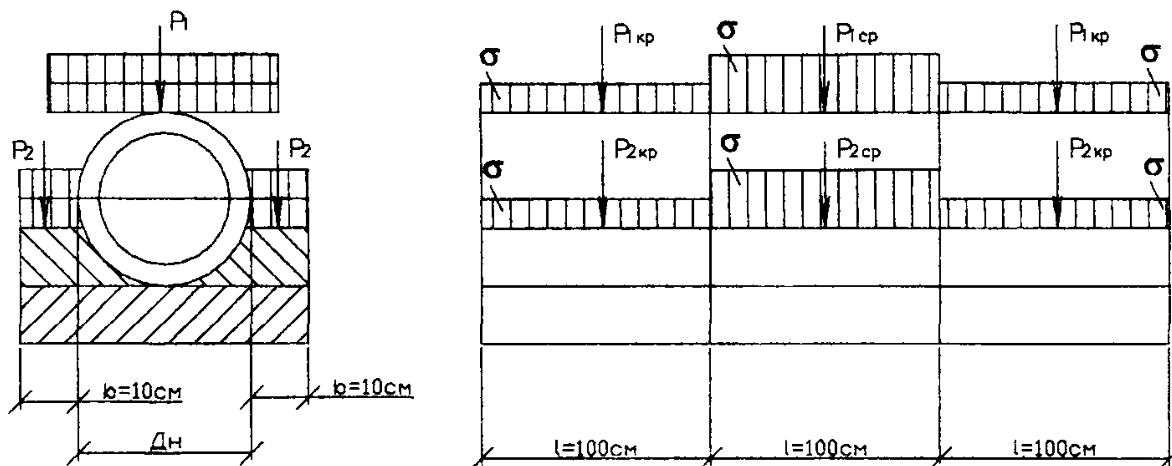
Рисунок 17 Схема нагрузки основания (при передаче нагрузки через три звена труб и выступы оснований)
