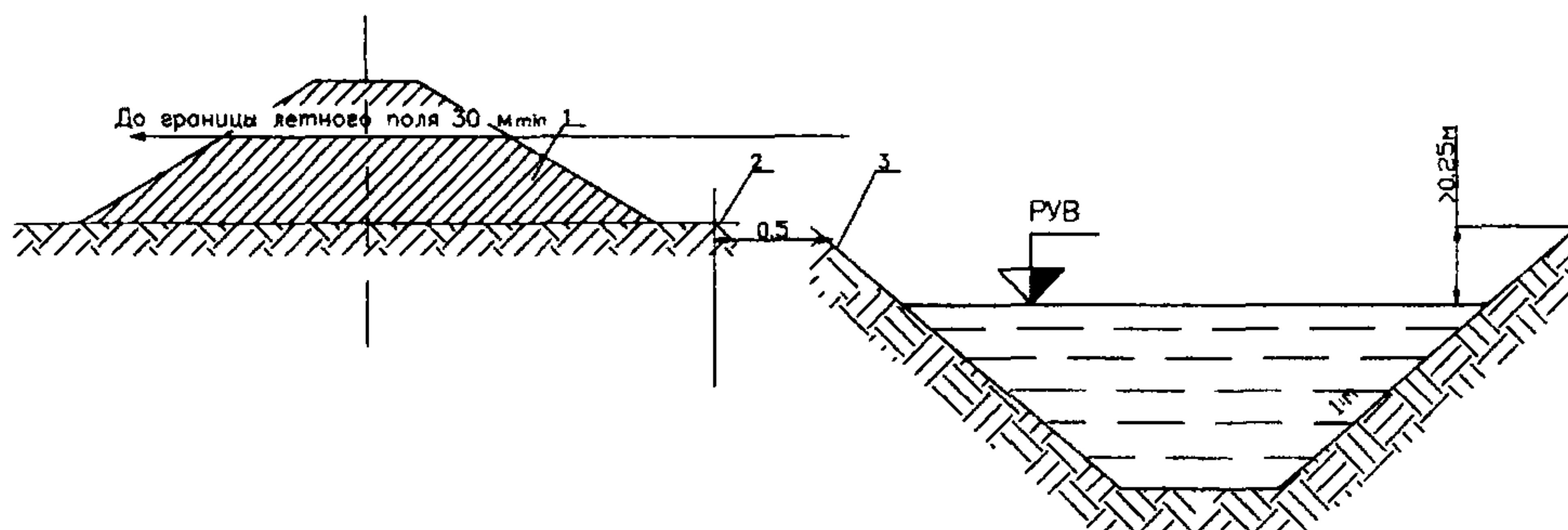
Рисунок 1 Нагорная канава 1 - кавальер; 2 – берма; 3 – бровка; ПУВ – расчетный уровень воды
