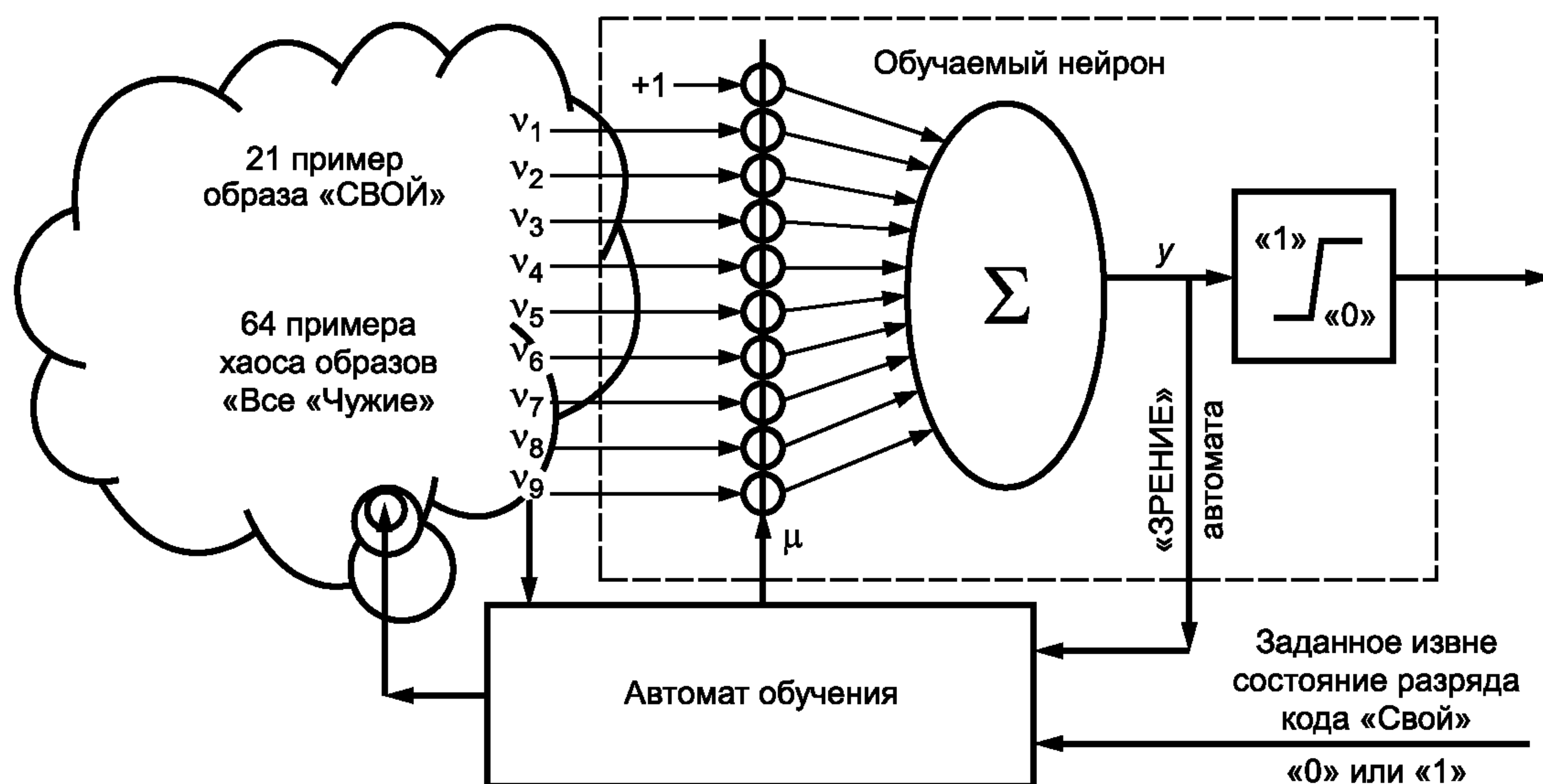
Рисунок 1 — Блок-схема обучения одного искусственного нейрона
