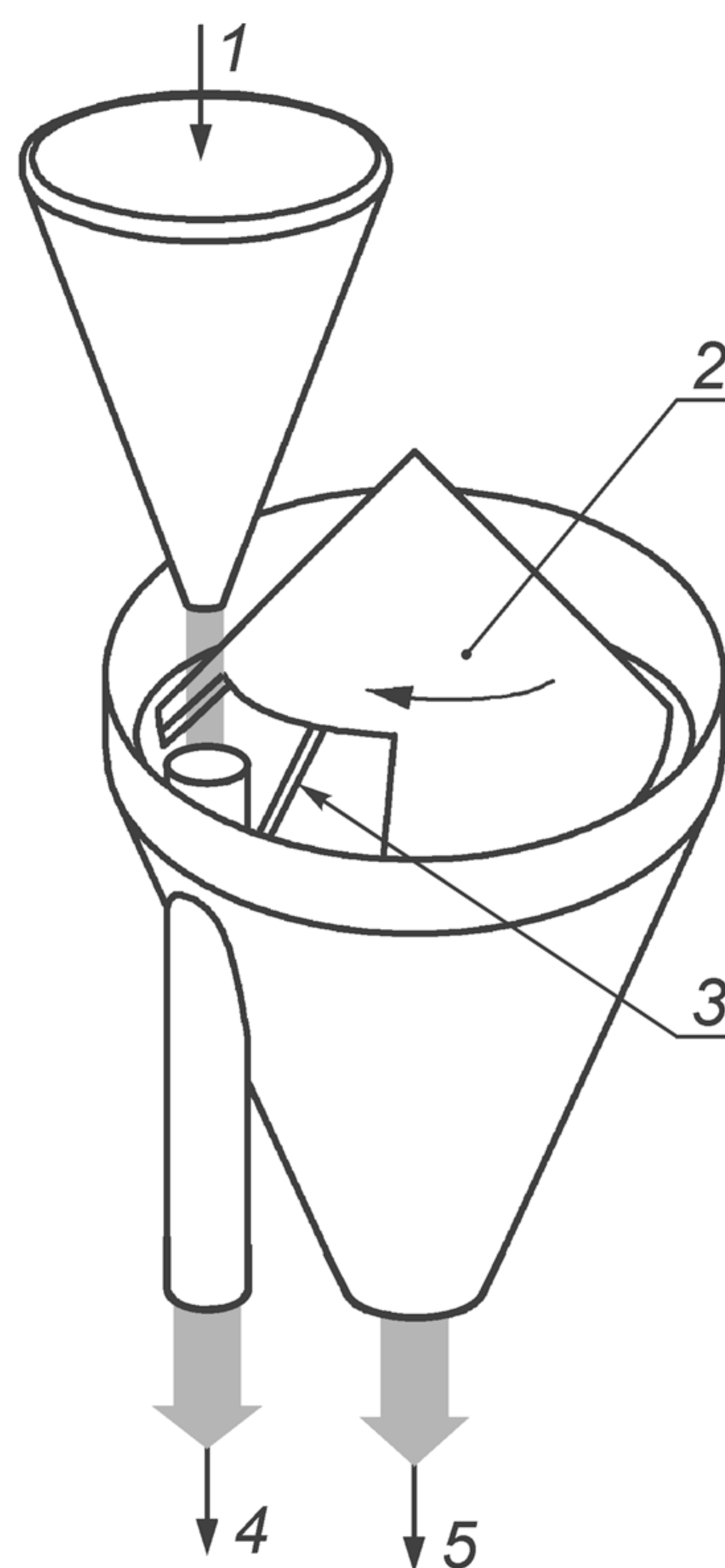
б) Тип с вращающимся конусом
