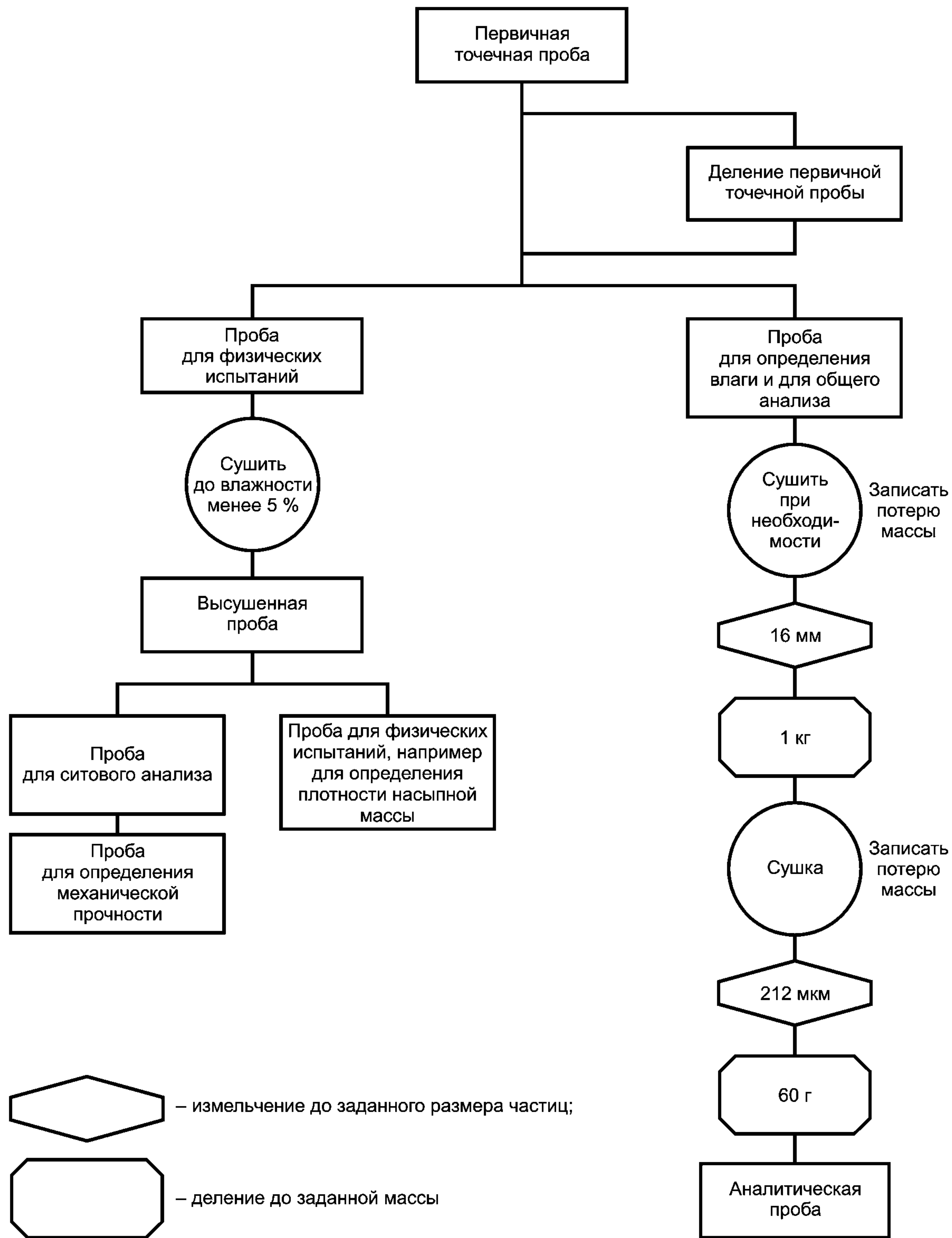
Рисунок 14 — Схема приготовления проб кокса для различных испытаний
