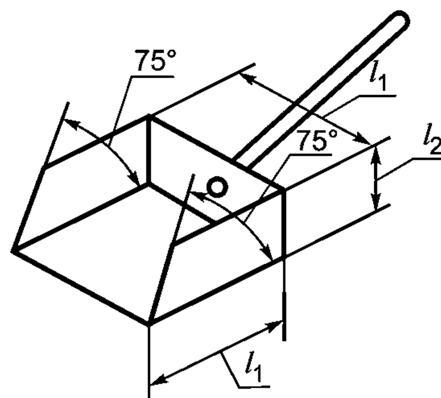
б) Лопата
