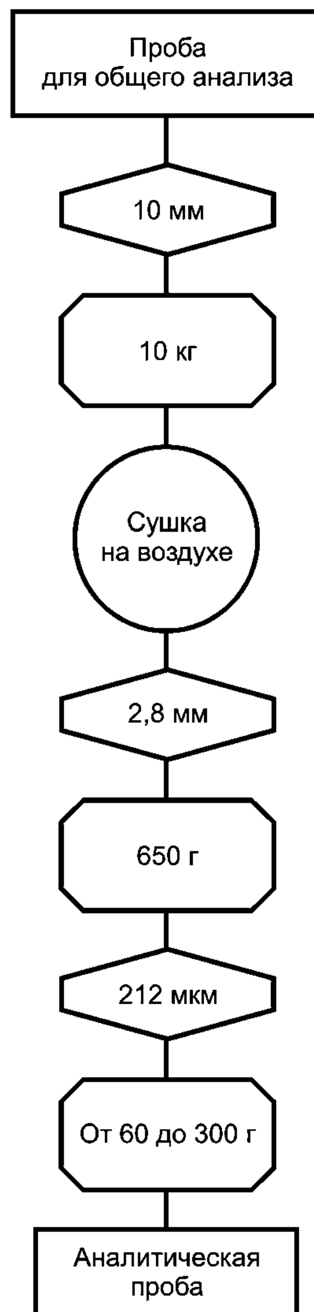
Рисунок 11 — Пример схемы приготовления пробы для общего анализа
