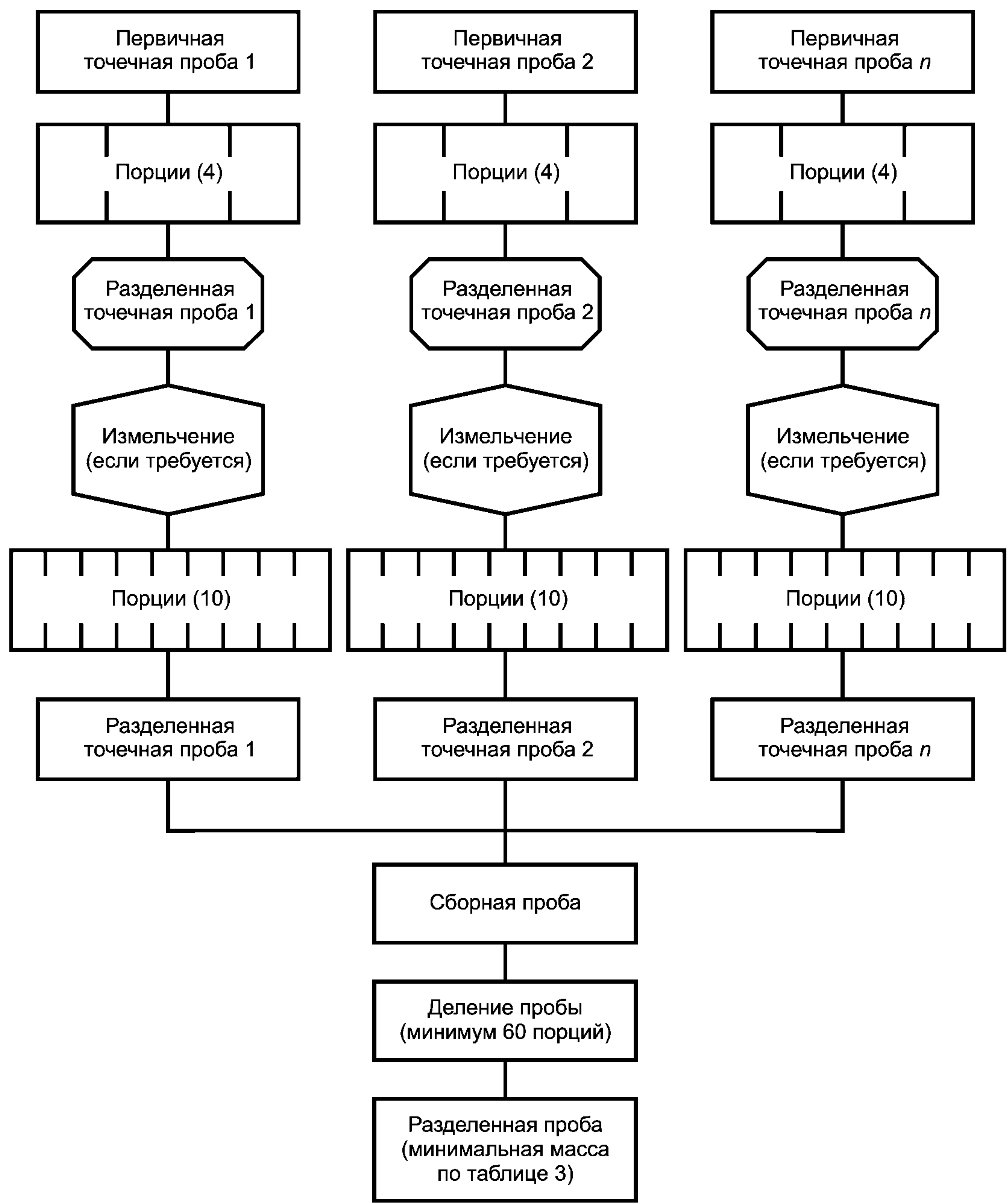
б) Пример двухступенчатого деления отдельных точечных проб
