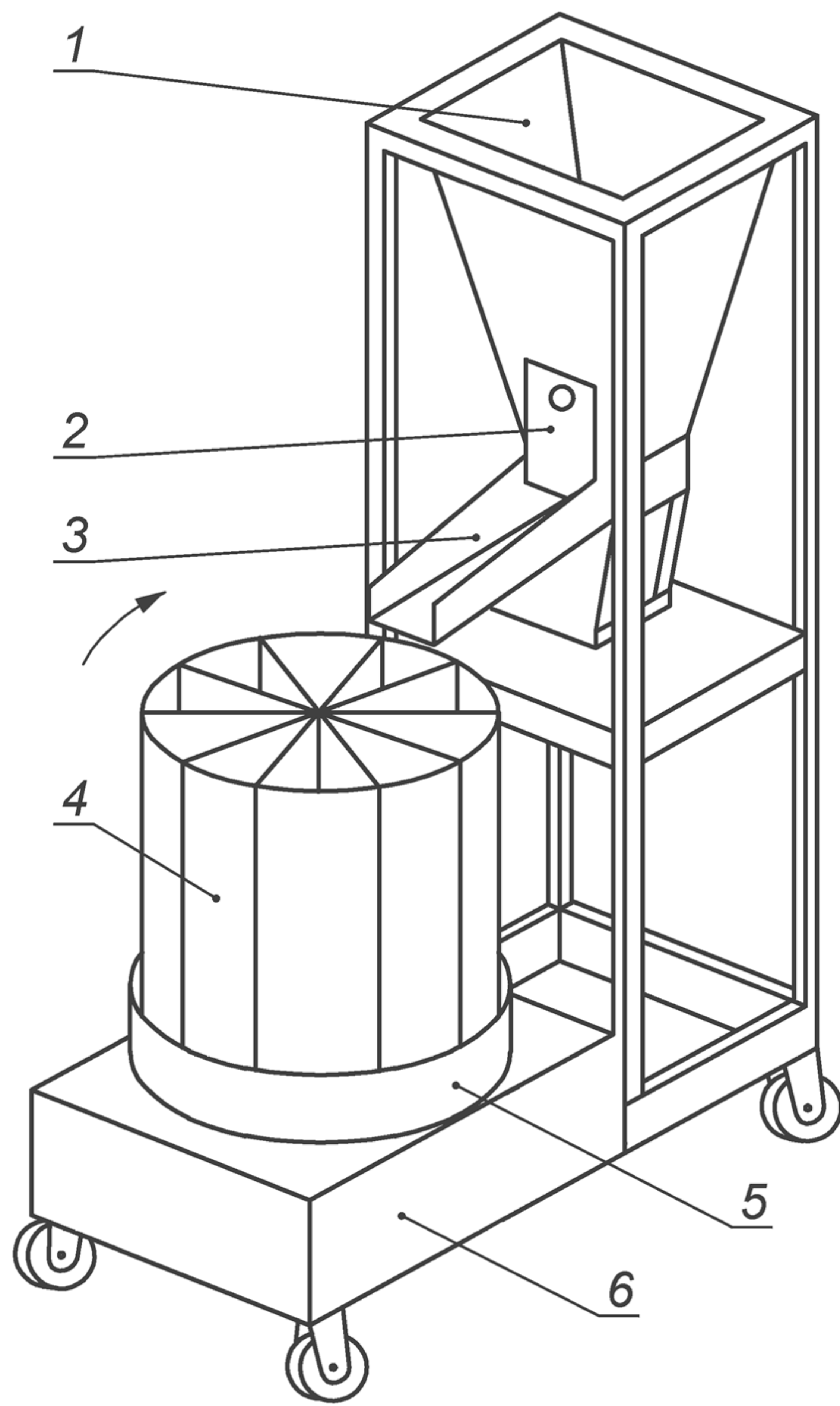
с) Тип с контейнером
