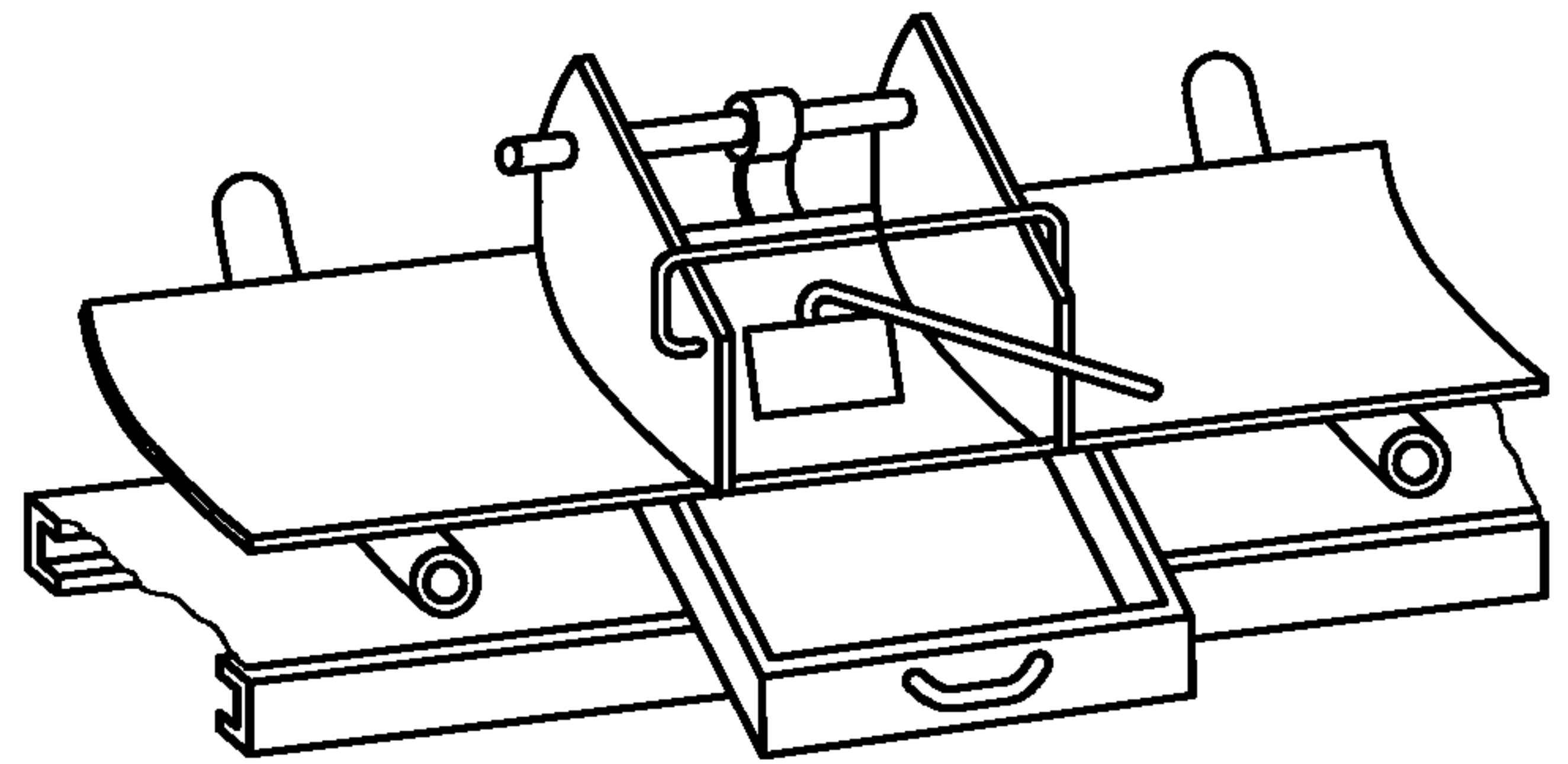
j) Рамка для отбора проб
