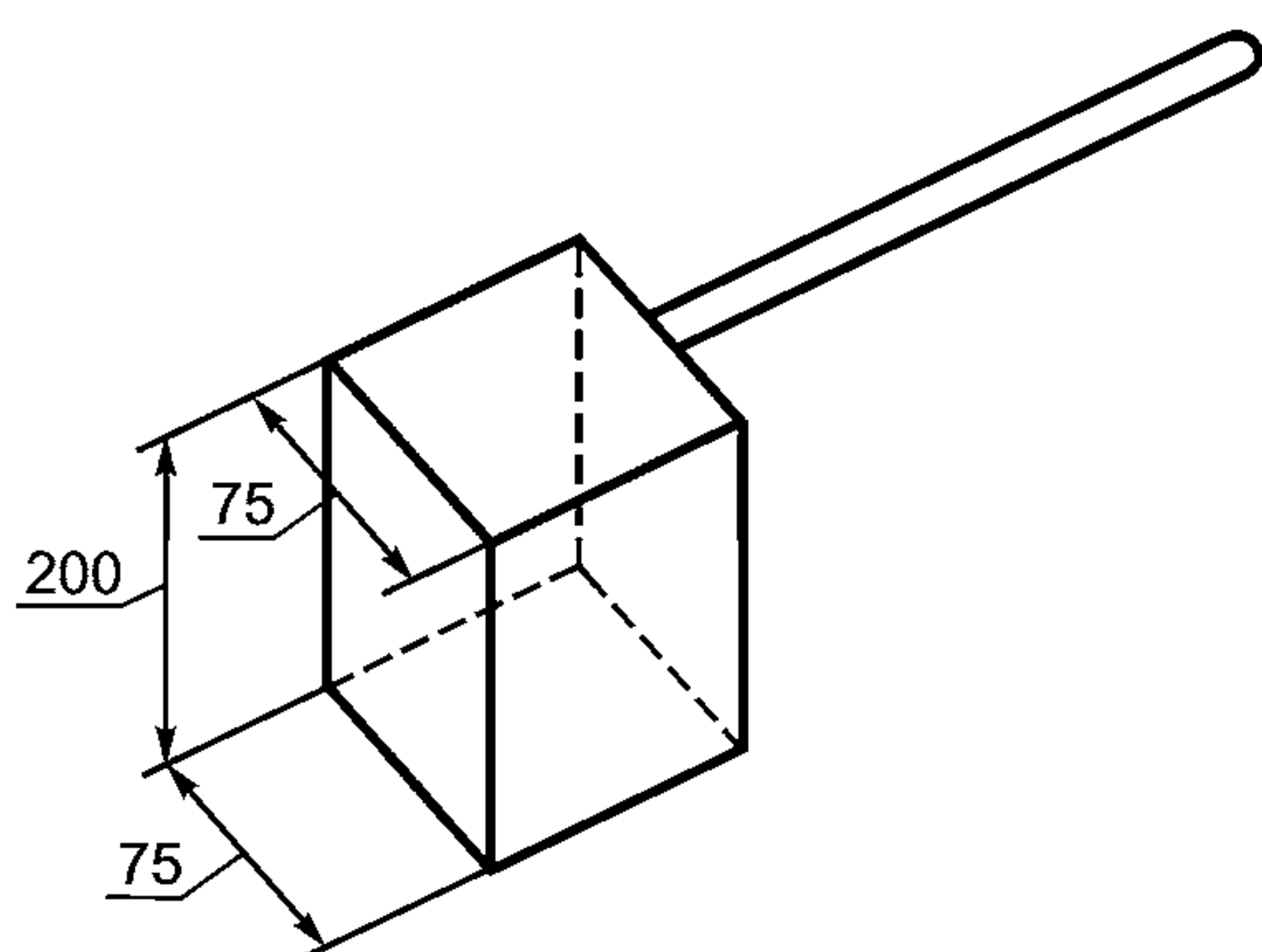
а) Черпак для мелочи размером до 25 мм
