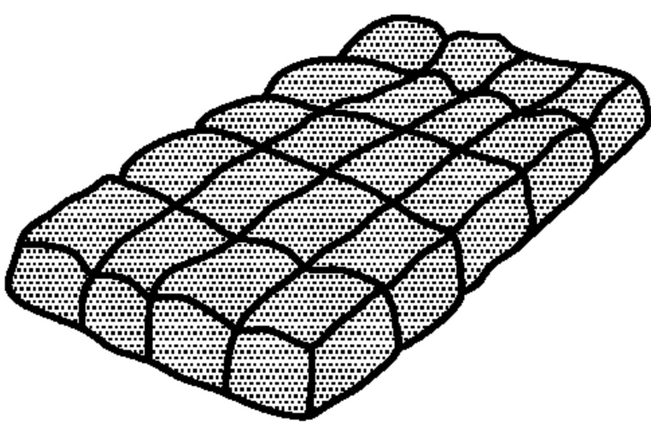
б) Расчерчивают топливо при помощи шаблона на 20 равных частей, например пять равных частей по длине и четыре равные части по ширине
