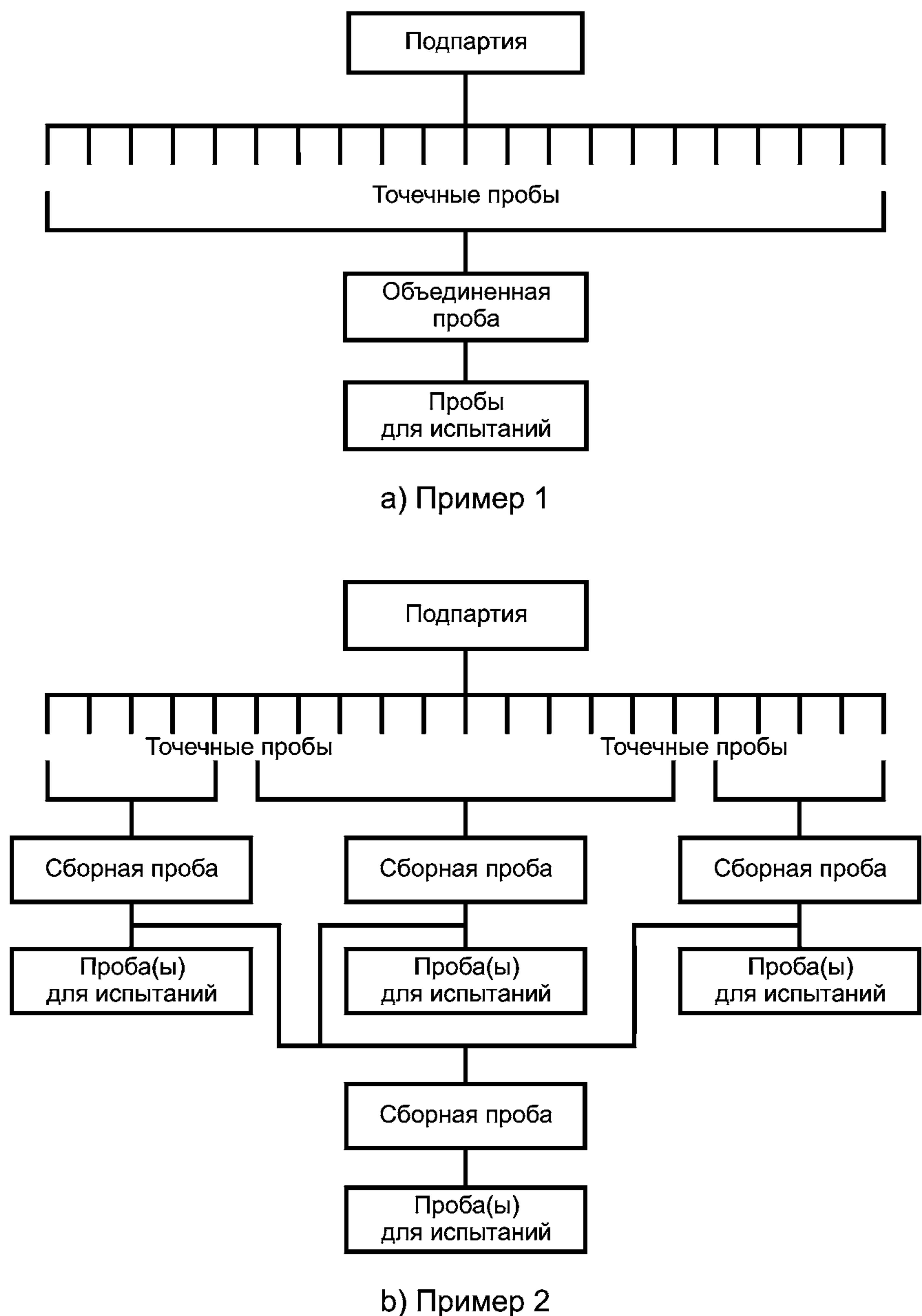
Рисунок 4 — Примеры приготовления проб для испытаний
