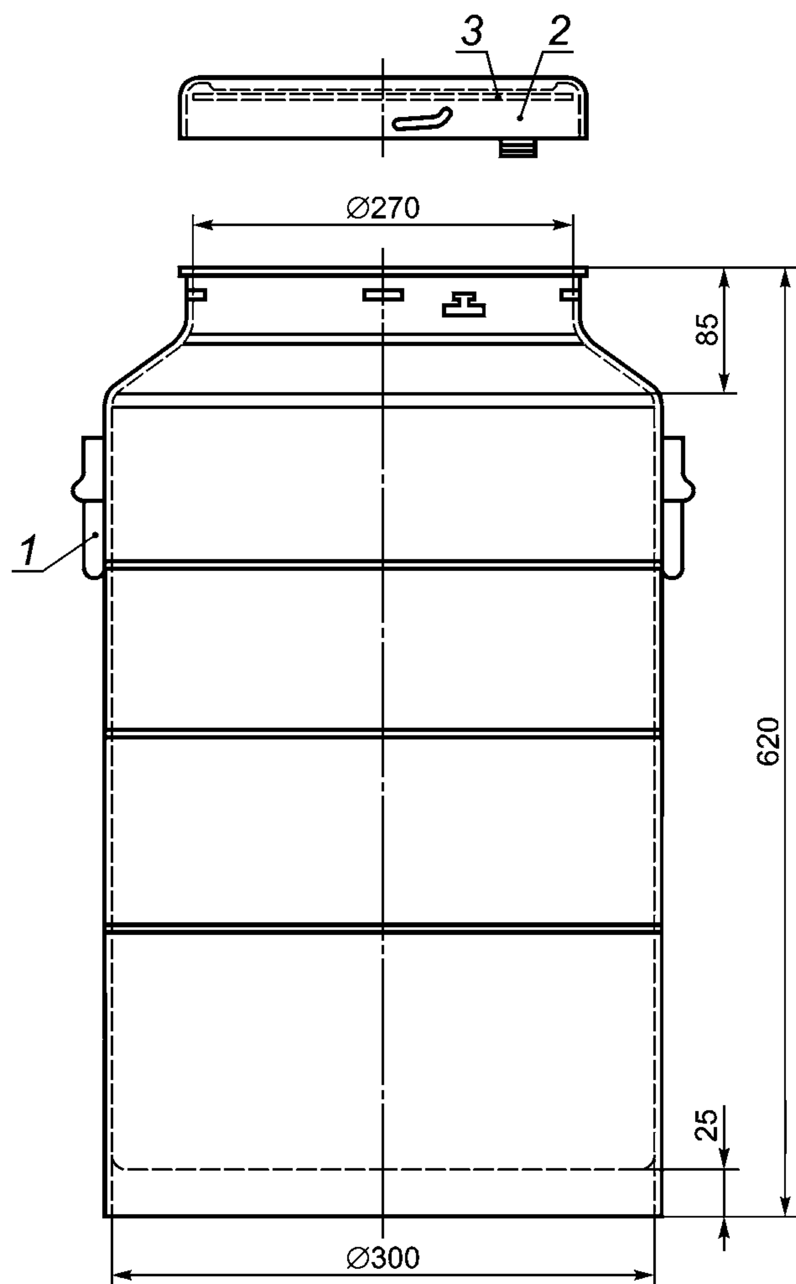
1 — ручка; 2 — крышка; 3 — резиновая прокладка
