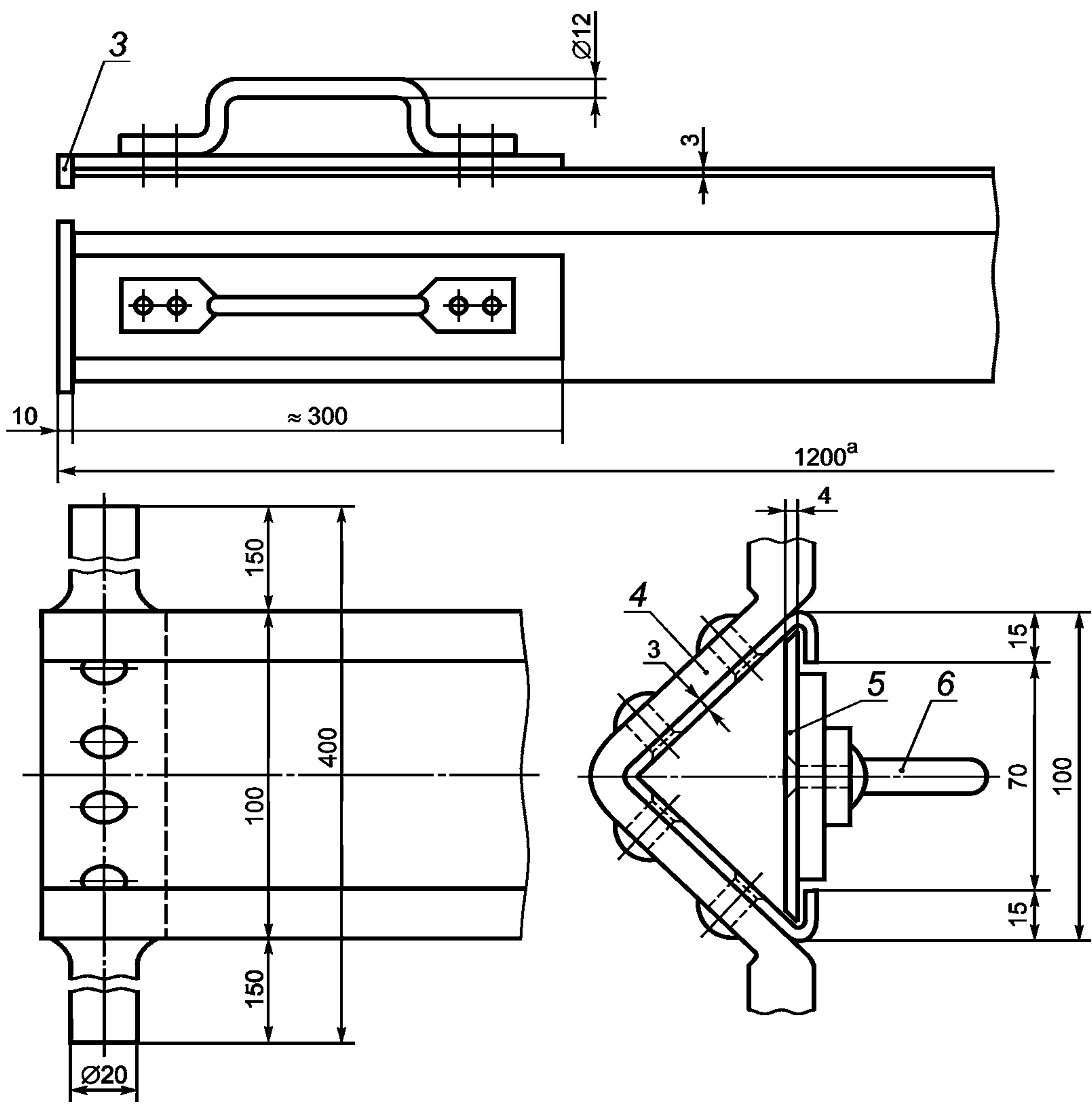
3 — деталь, являющаяся упором; 4 — верхняя опора корпуса зонда; 5 — пластина; 6 — ручка пластины
