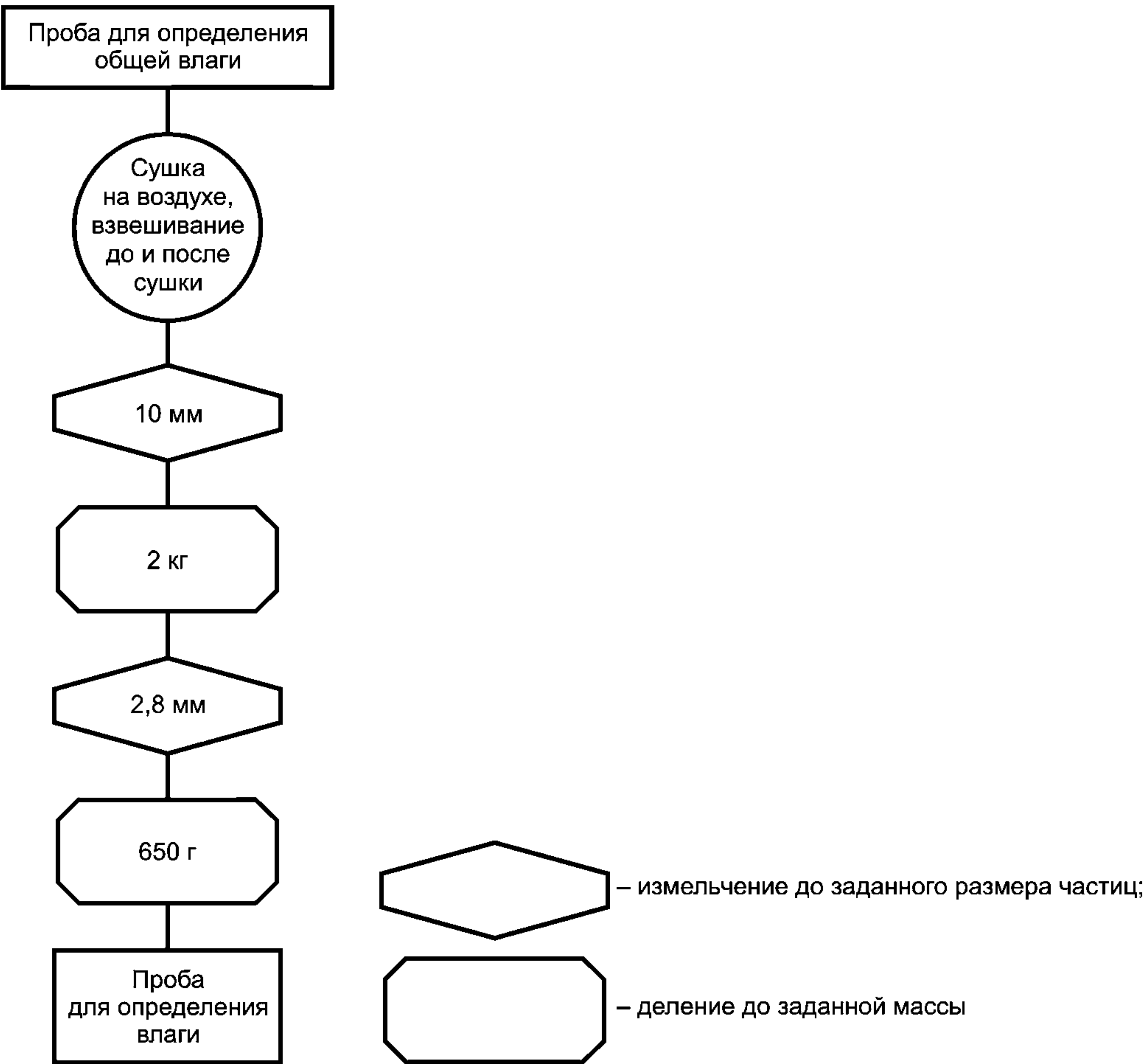
Рисунок 10 — Пример схемы приготовления пробы для двухступенчатого определения содержания общей влаги
