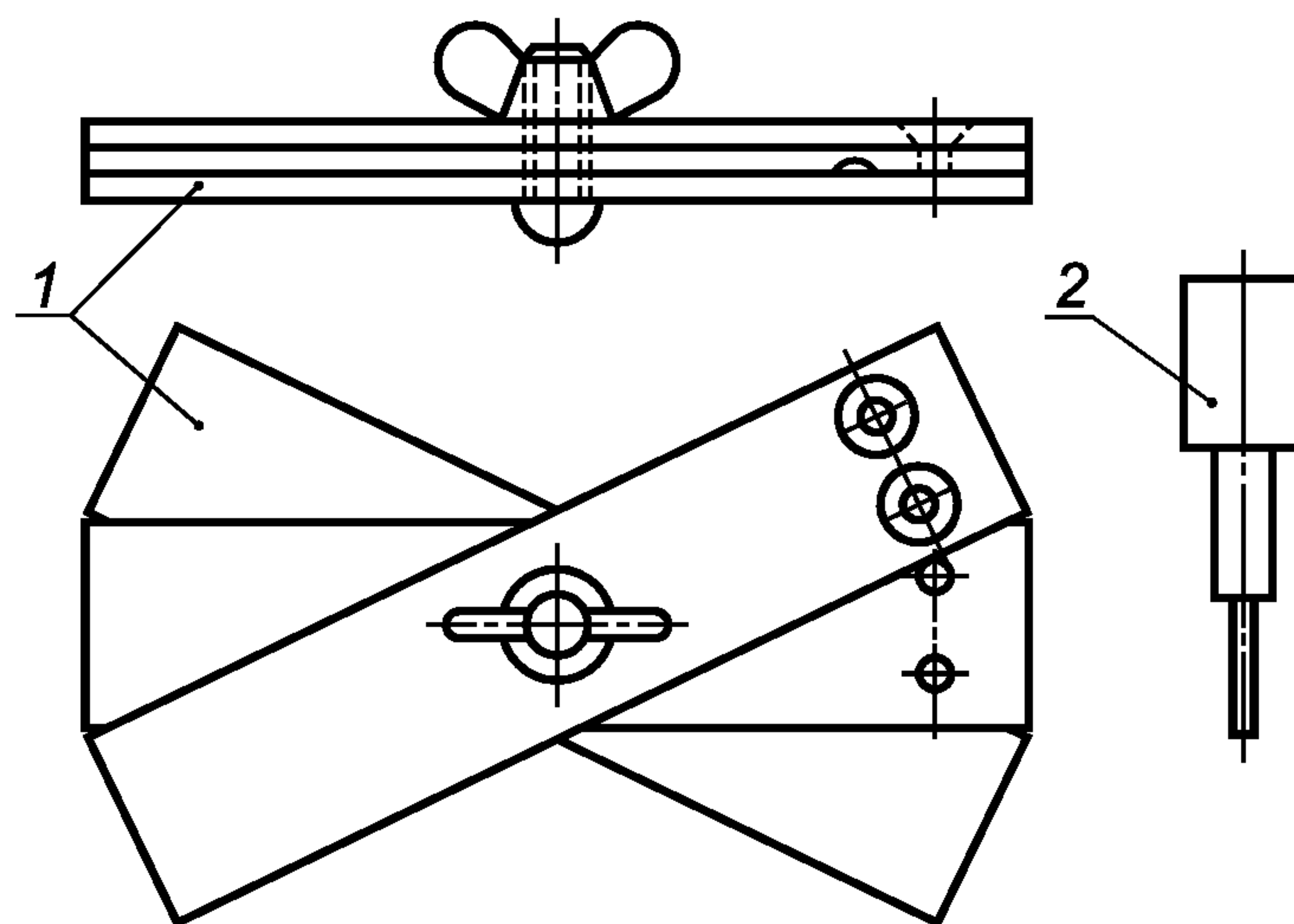
Рисунок 1 — Форма для изготовления образца золы в виде пирамиды
