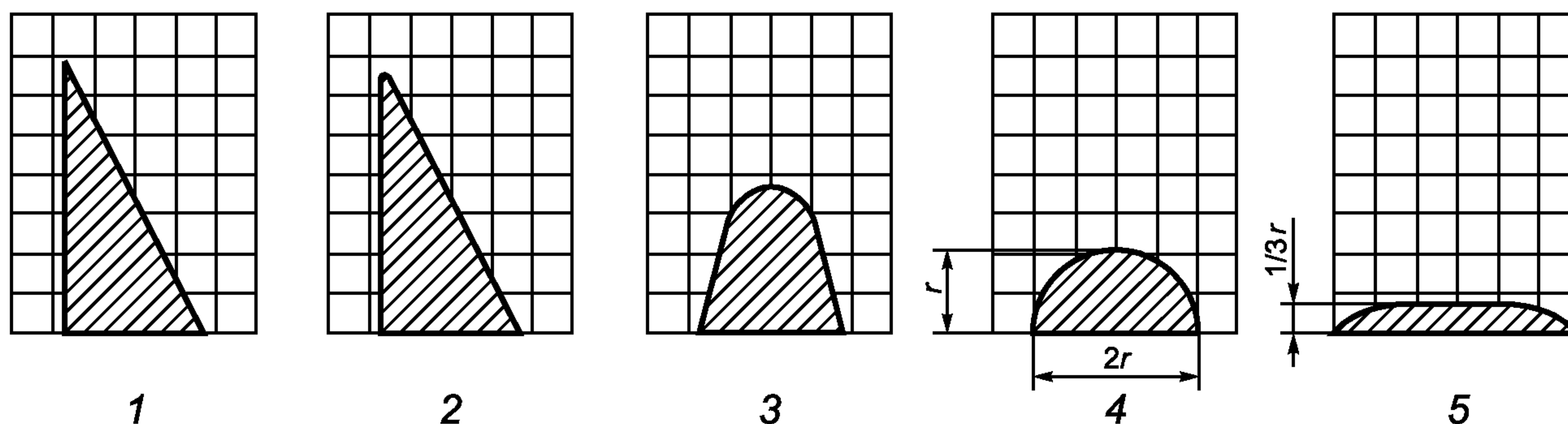
1 — исходный контур; 2 — деформация; 3 — сфера; 4 — полусфера; 5 — растекание
