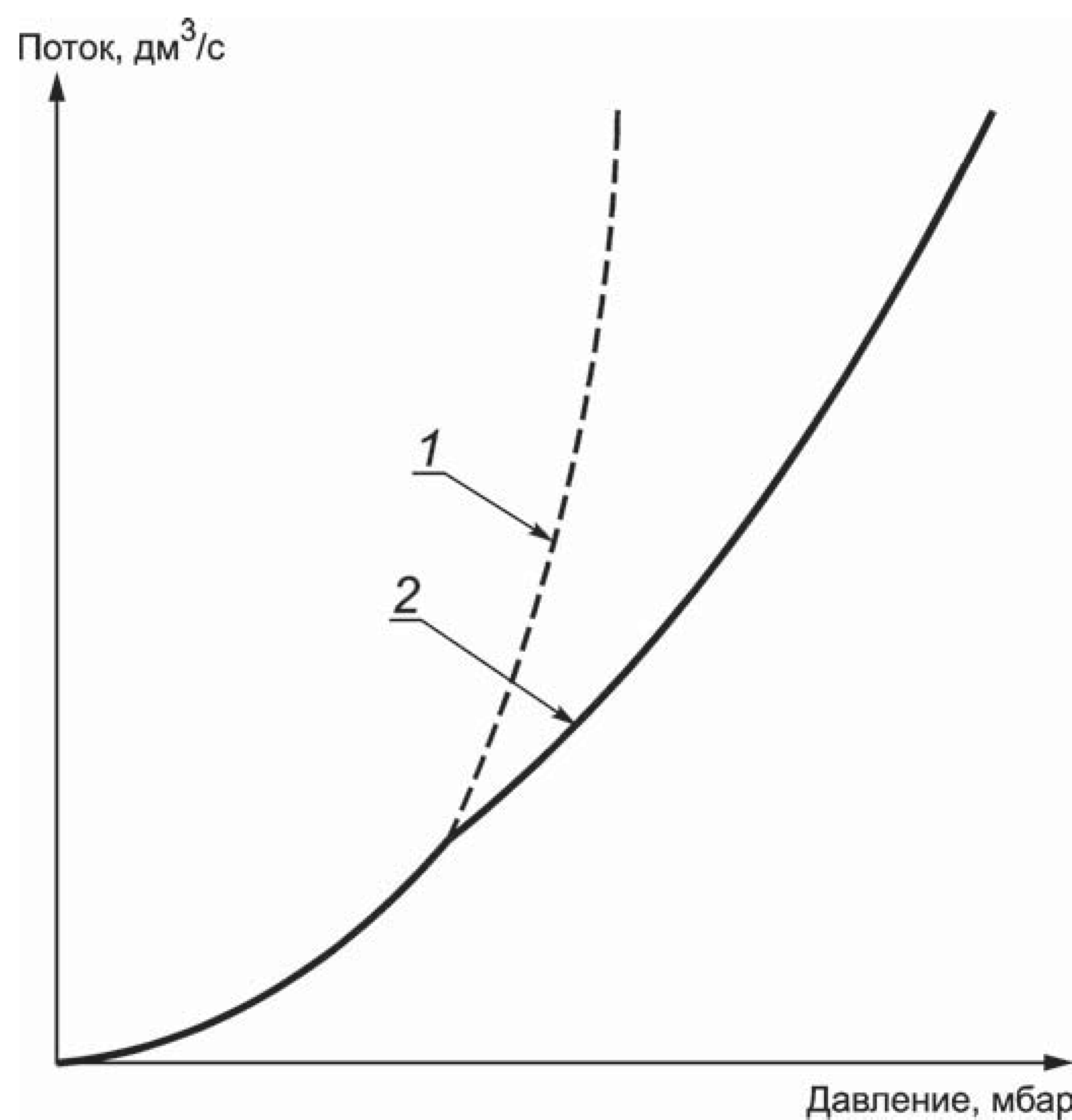
1 — редукционный клапан открыт; 2 — редукционный клапан закрыт
