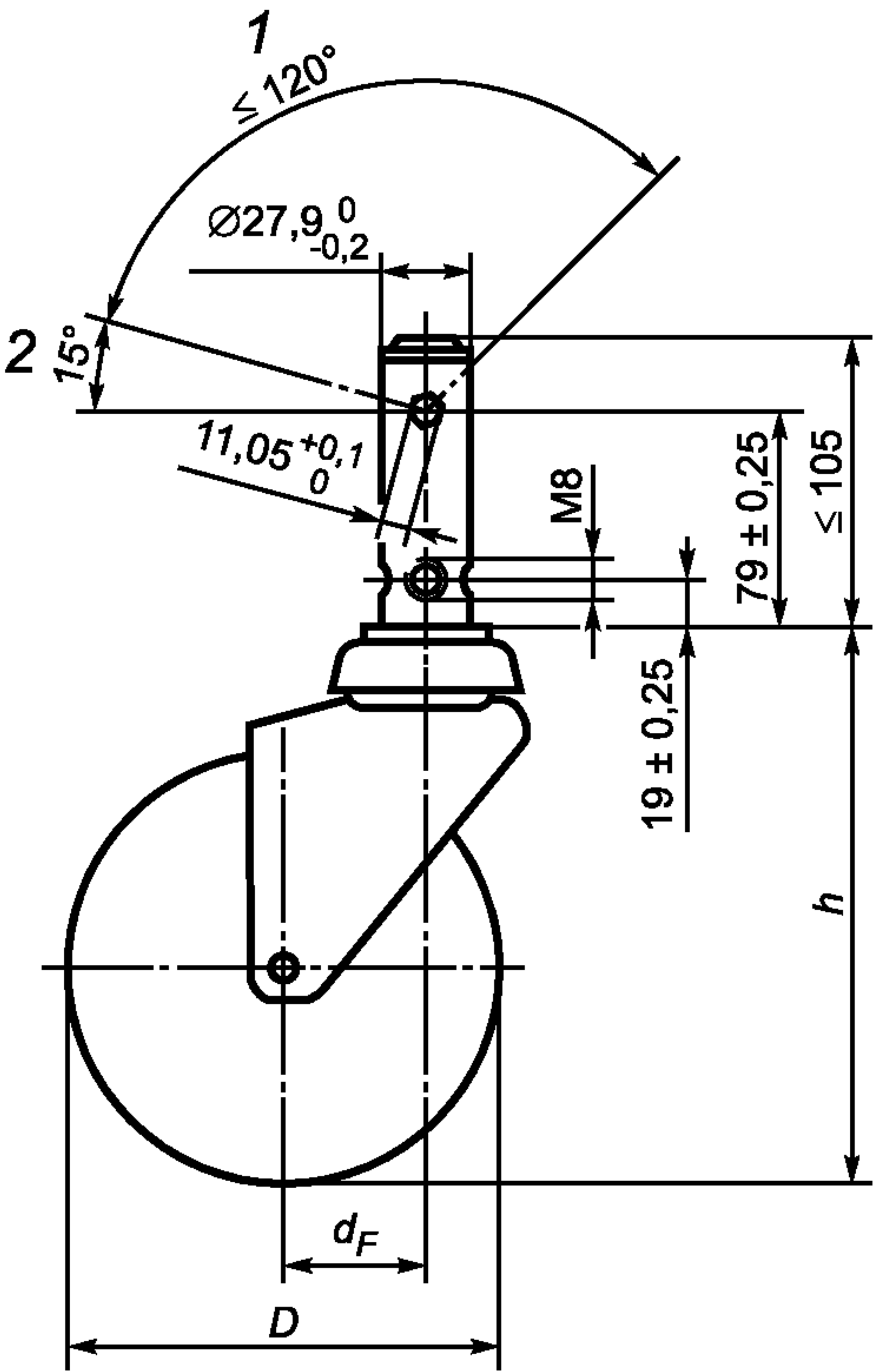
1 — рабочий угол; 2 — разблокированное положение
