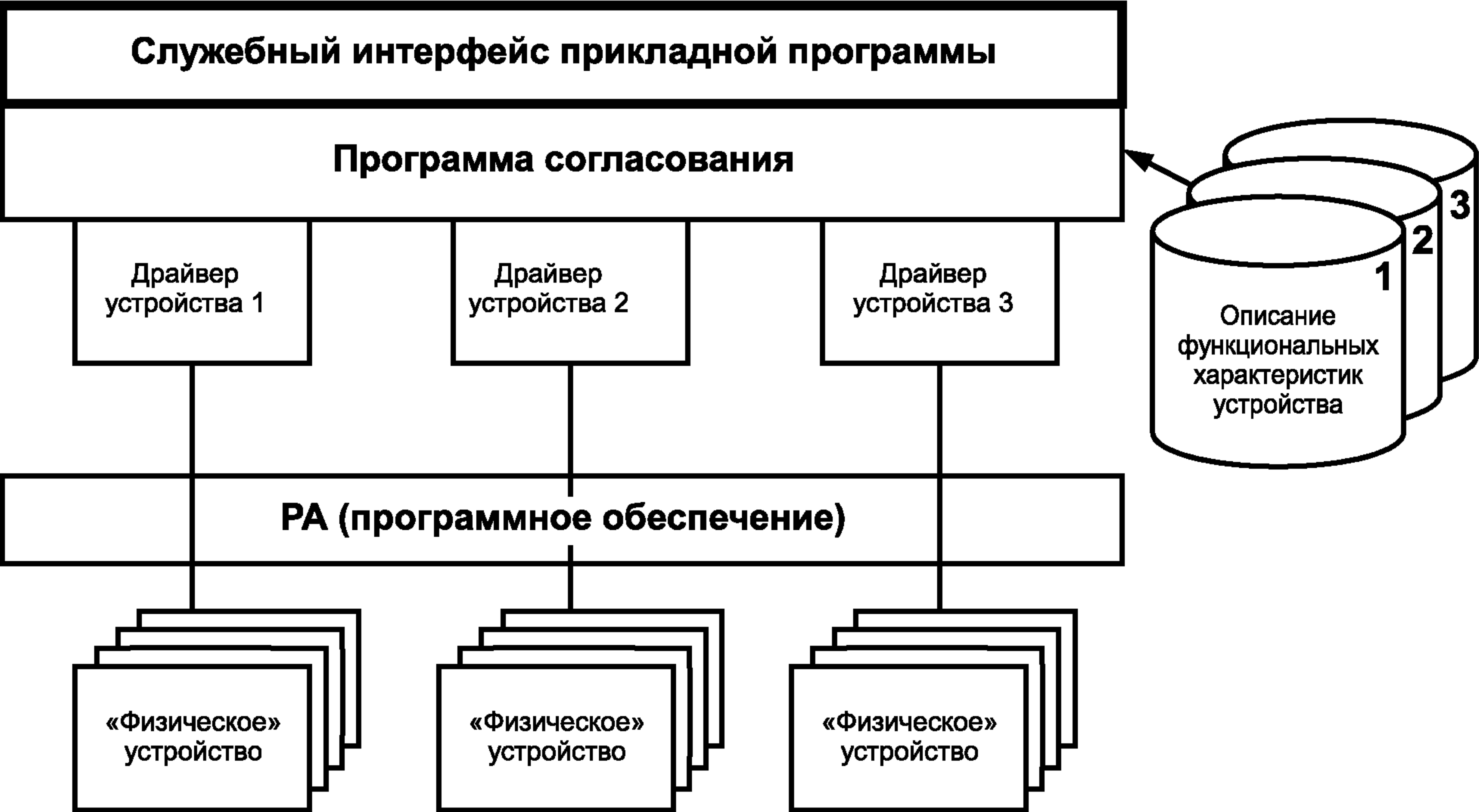
Рисунок 6 — Координатор работы с различными драйверами устройств
