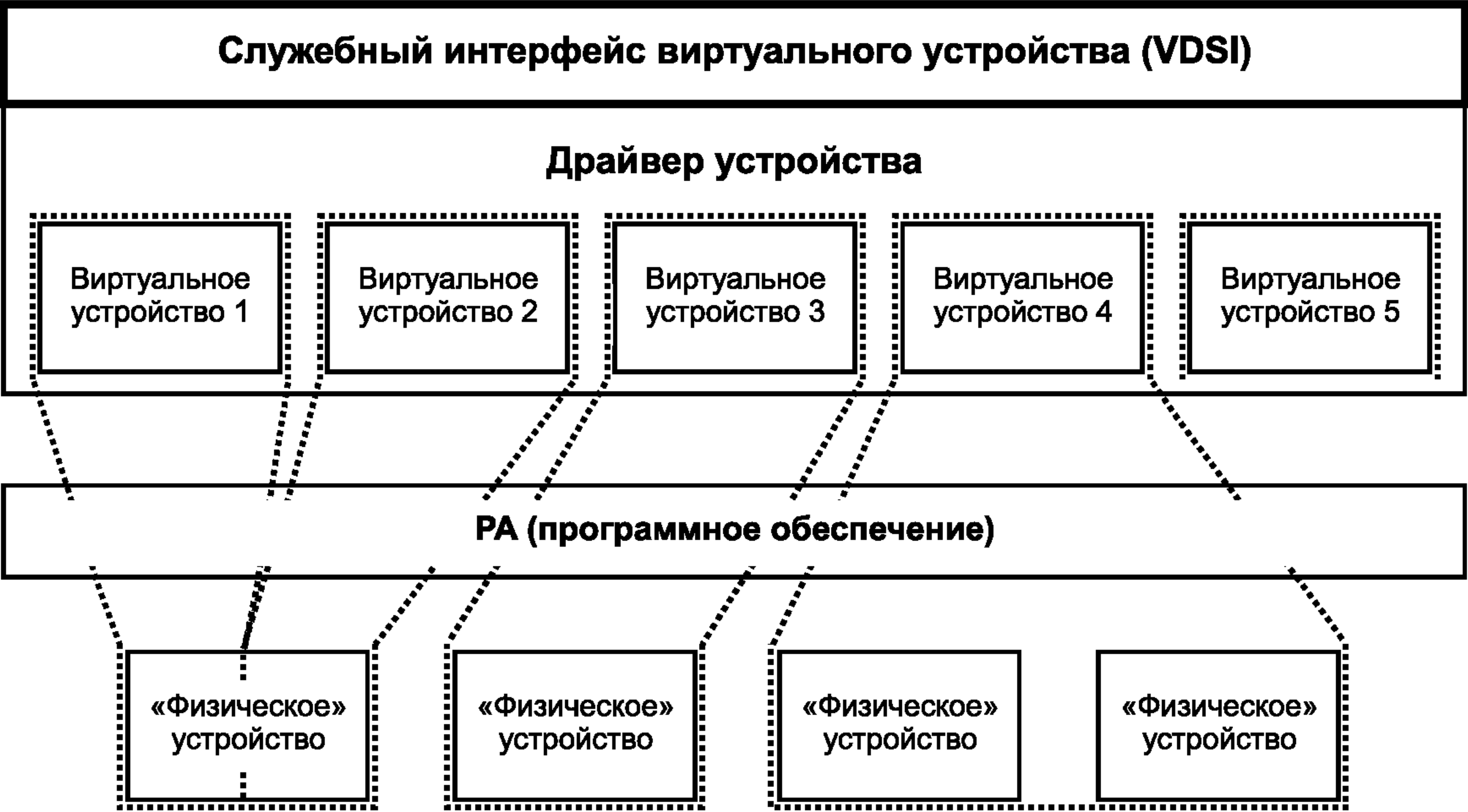
Рисунок 3 — Отображение в памяти виртуальных устройств
