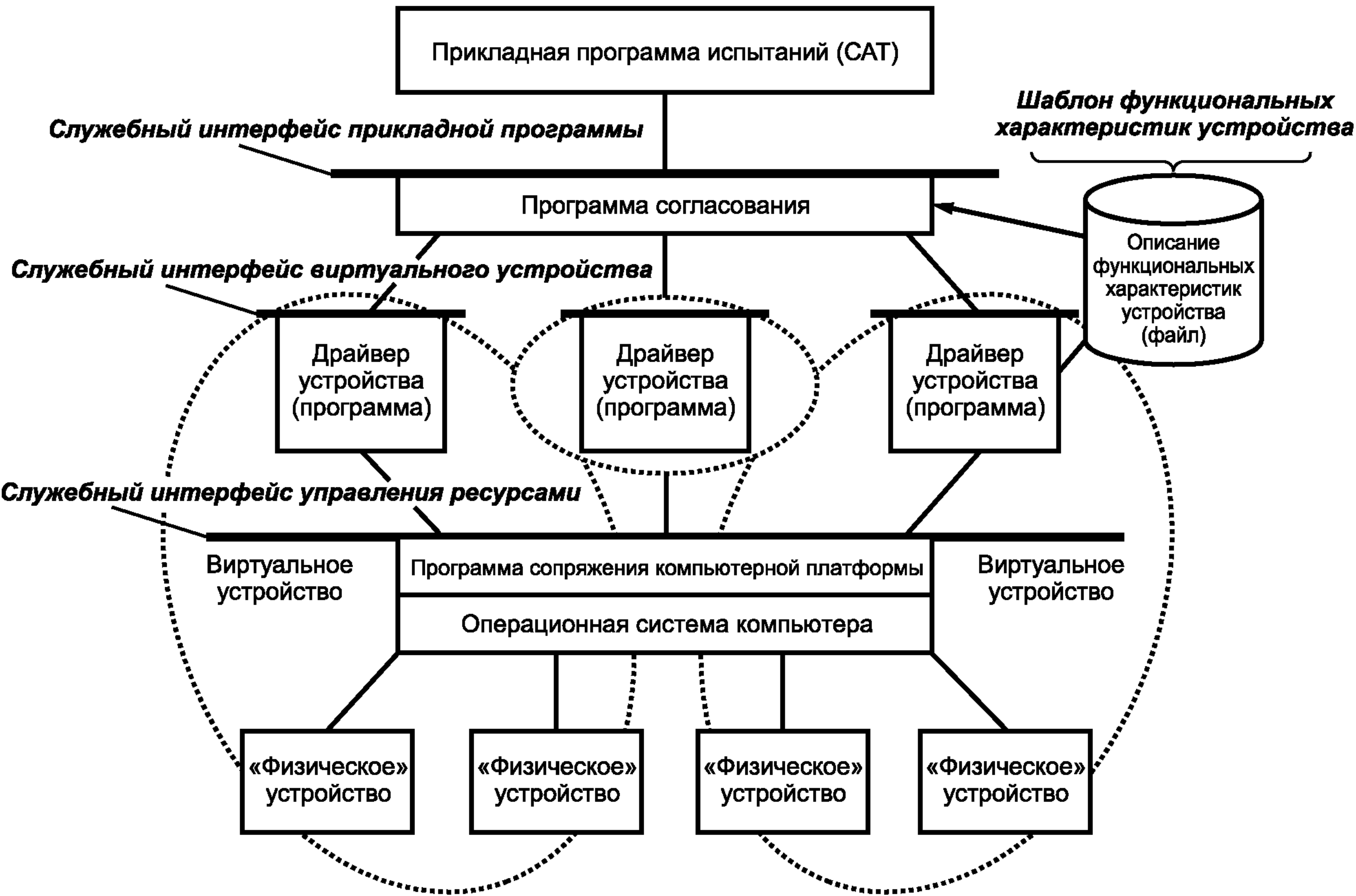
Рисунок 1 — Служебные интерфейсы, определенные в комплексе стандартов ИСО 20242
