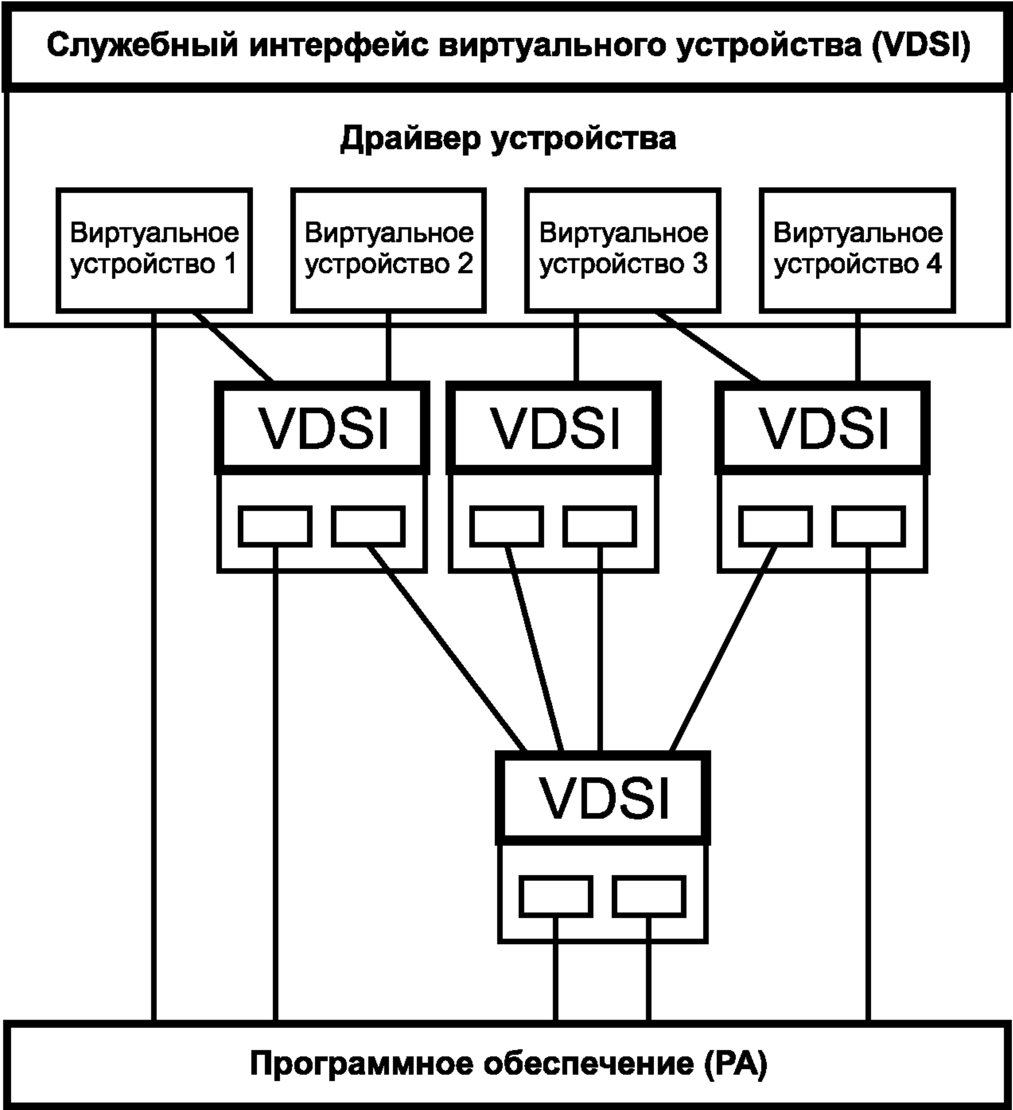
Рисунок С.1 — Пример каскадной структуры драйверов устройства
