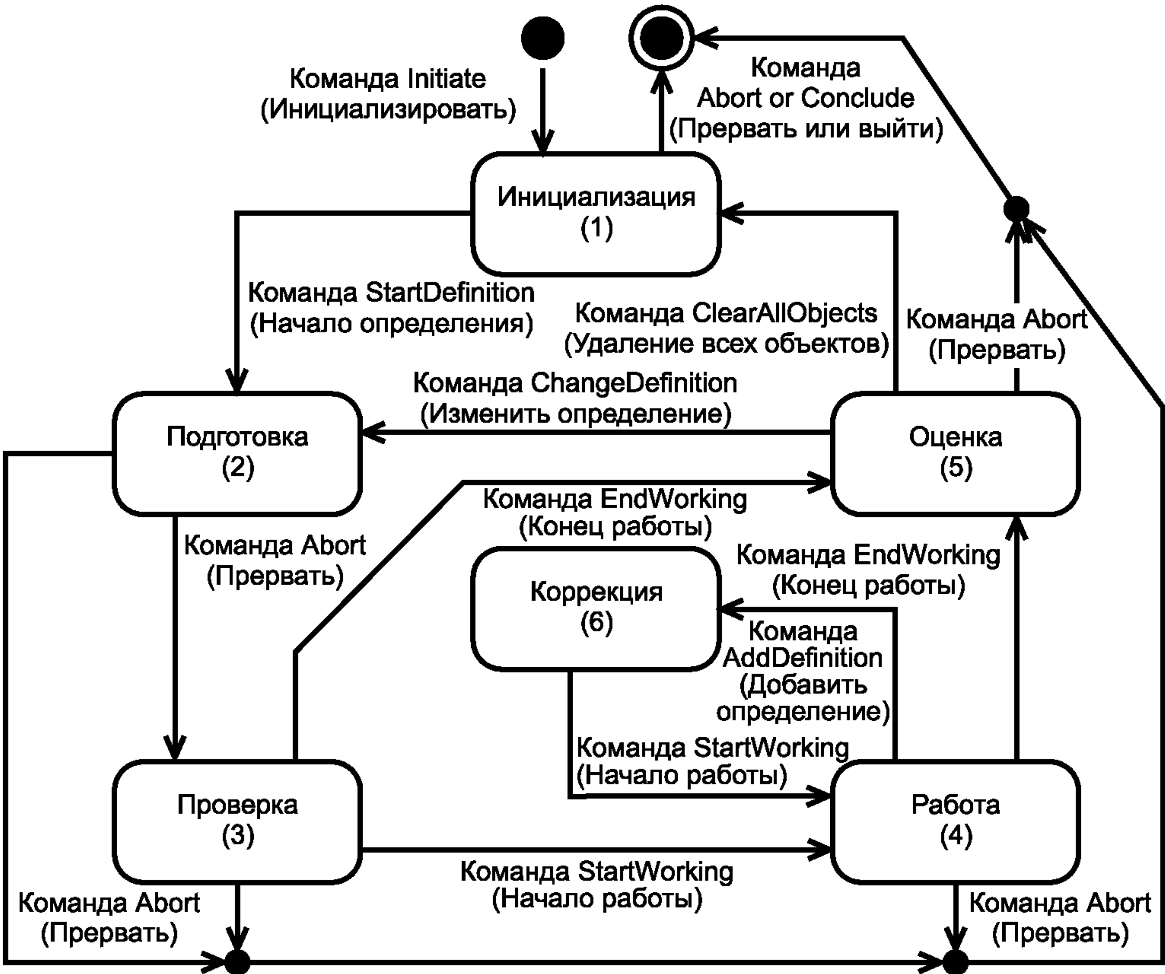
Рисунок В.1 — Различные состояния виртуального устройства
