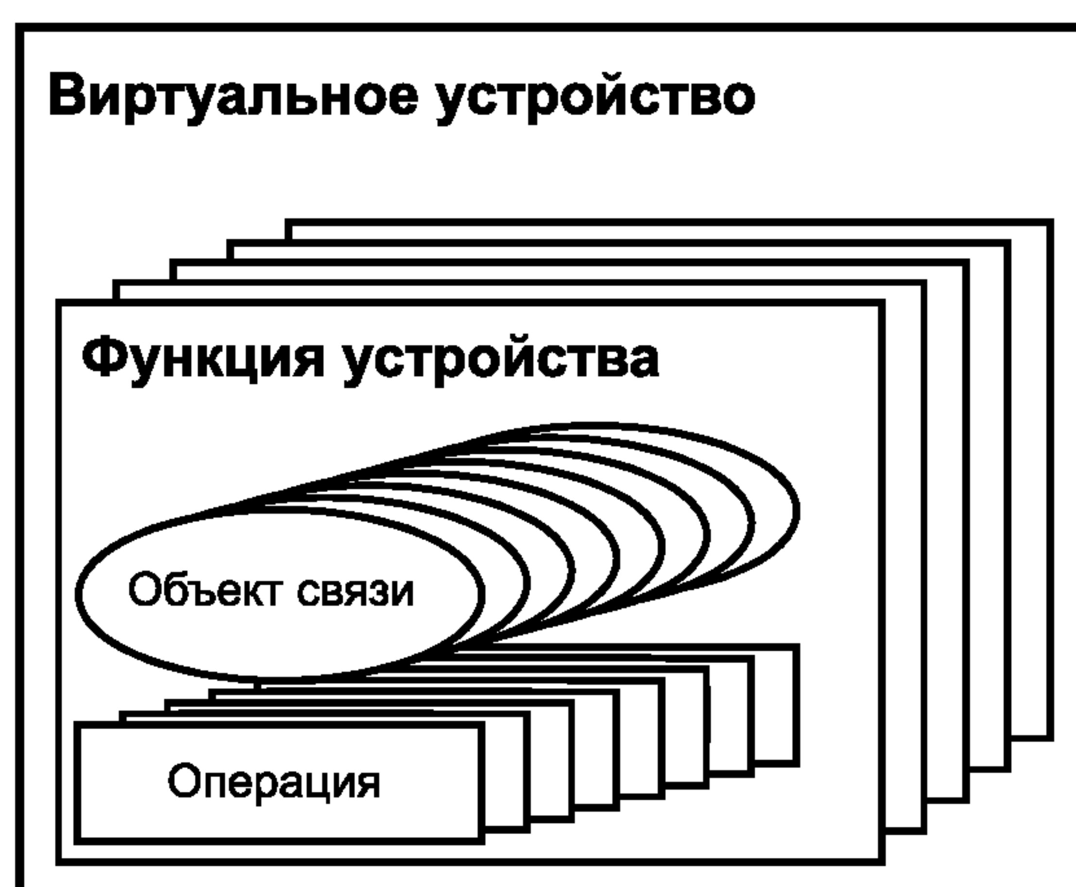
Рисунок 4 — Внутренняя структура виртуальных устройств
