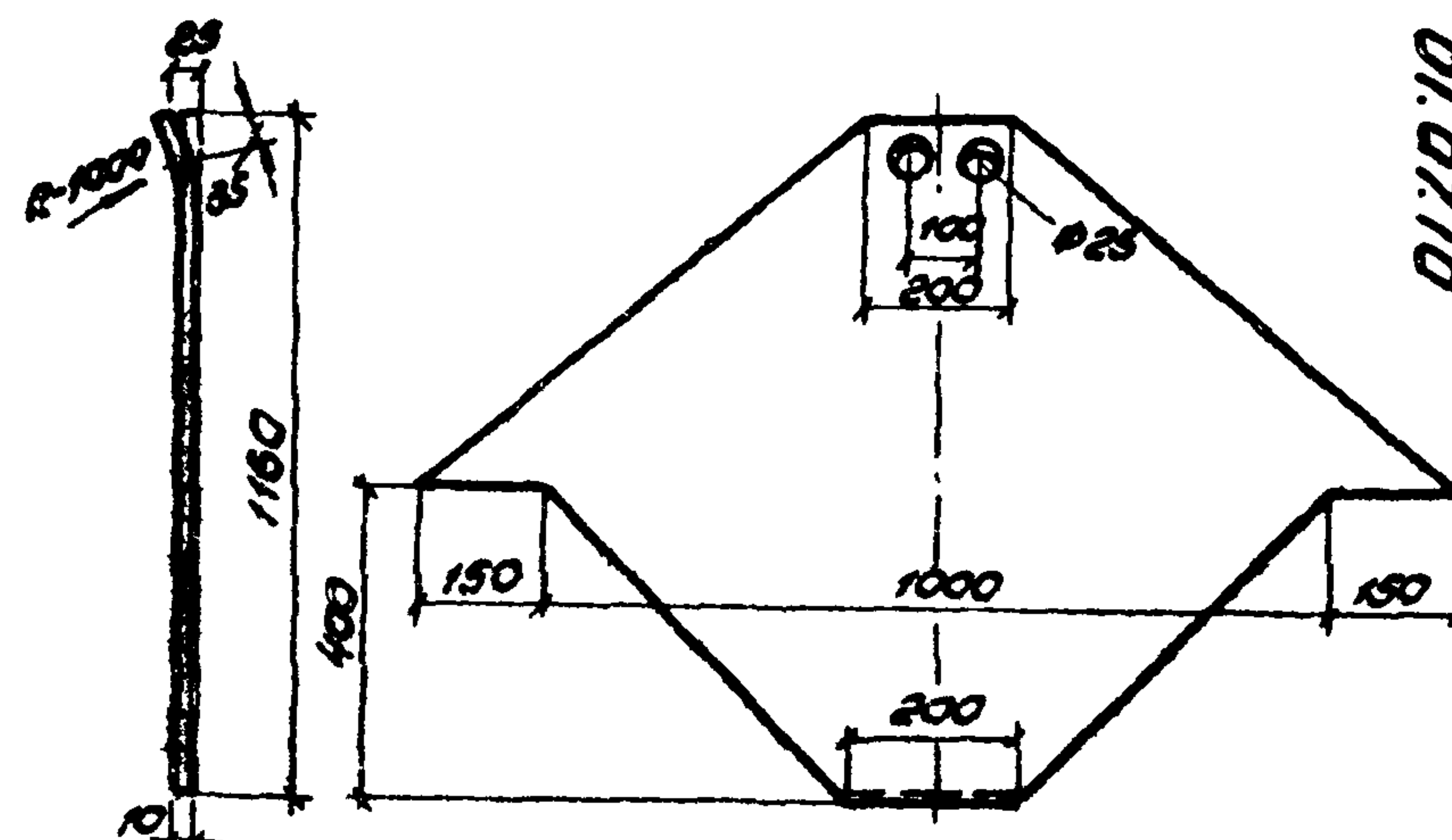
Рис.2 Лобовой лист
