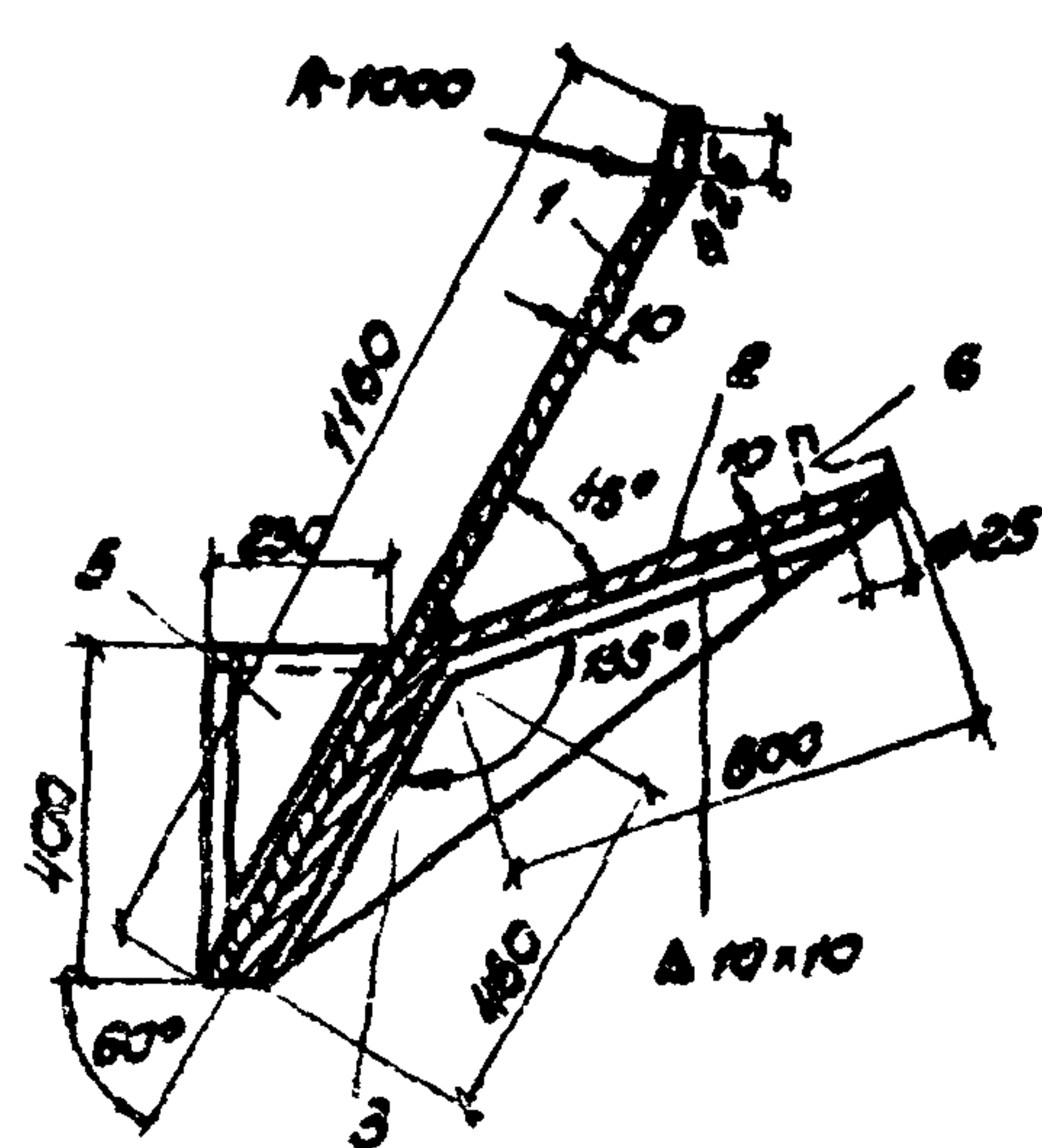
Рис.1 Отвал бульдозе- ра-канавкокопателя.
