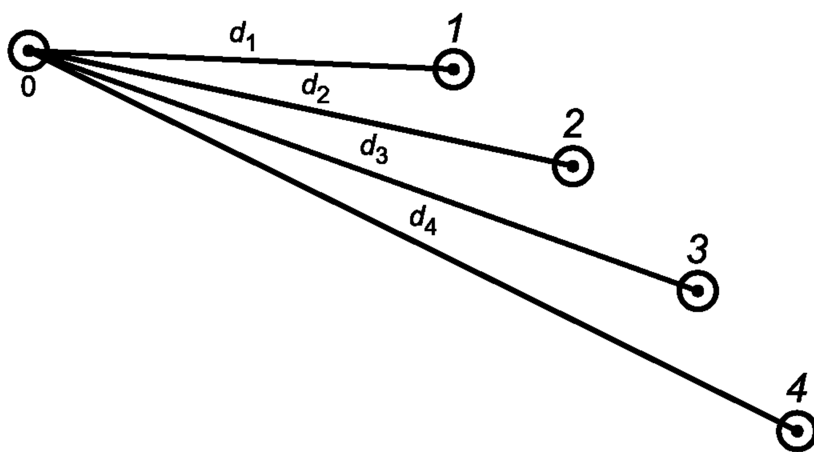
Рисунок 1 — Конфигурация испытательного поля для упрощенной методики испытания
