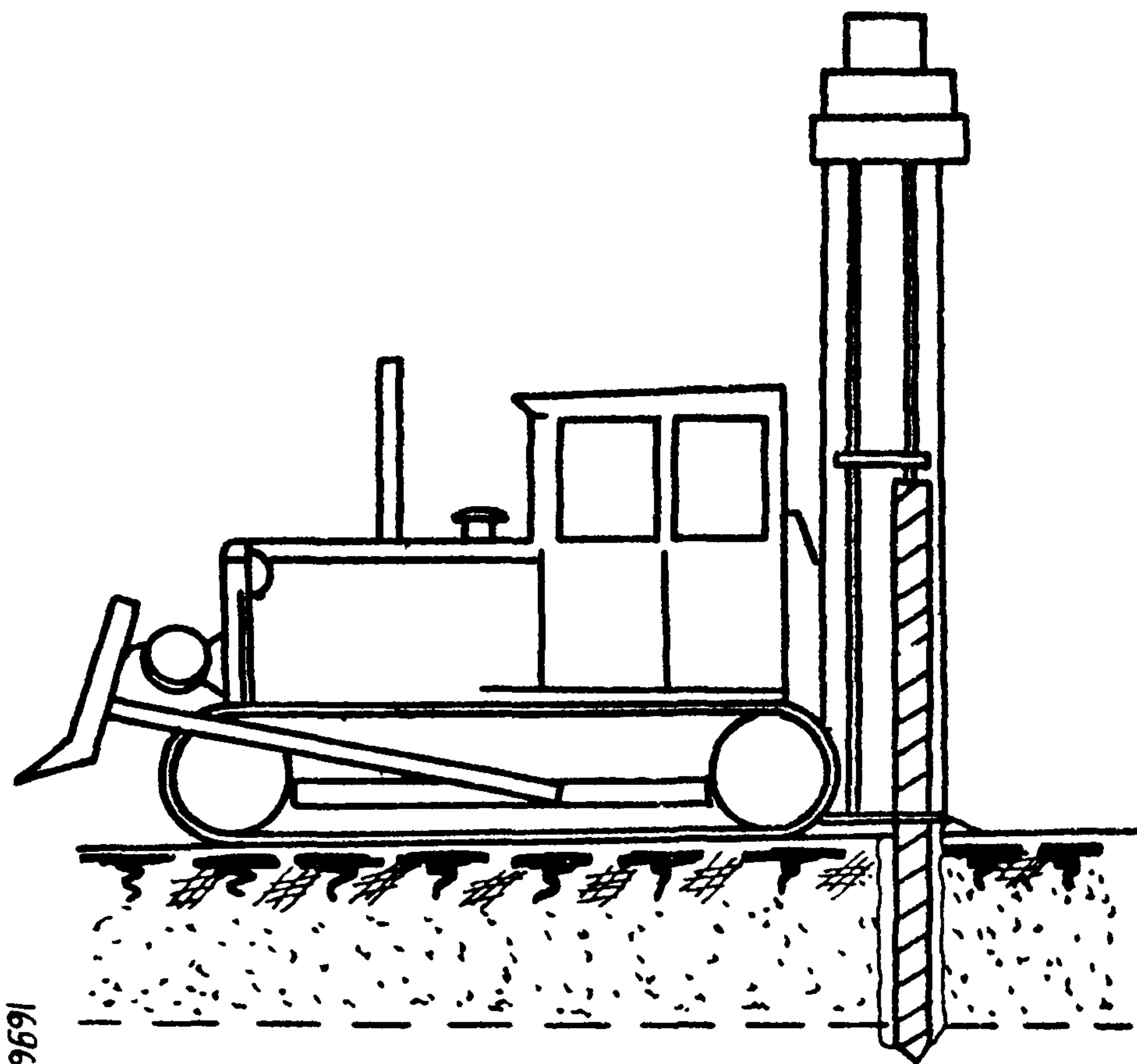
рис. 2 Техническая характеристика буровой установки М-1 на тракторе ДТ-54
