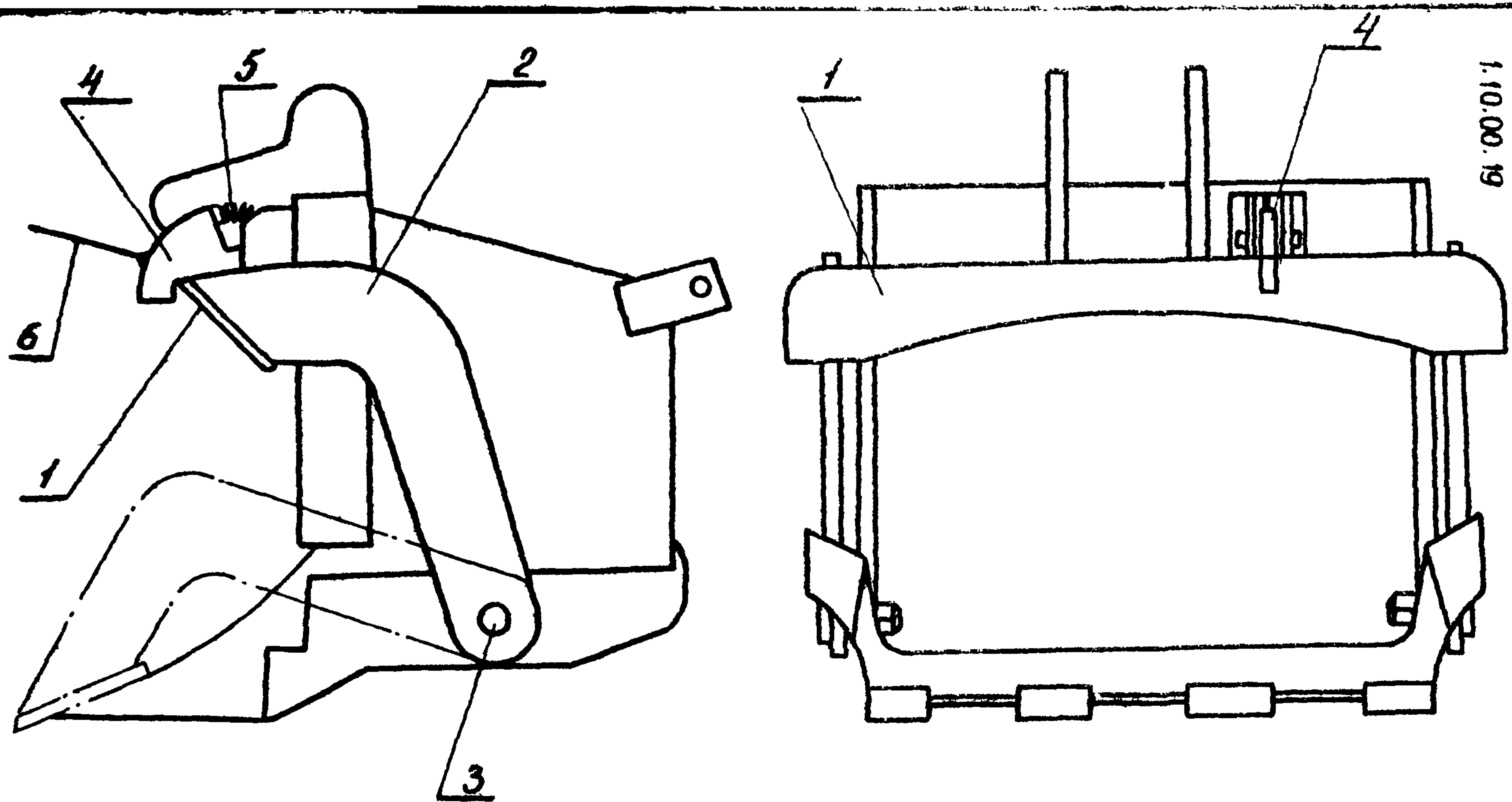
Рис. 5 Струг для зачистки дна траншей экскаватором.
