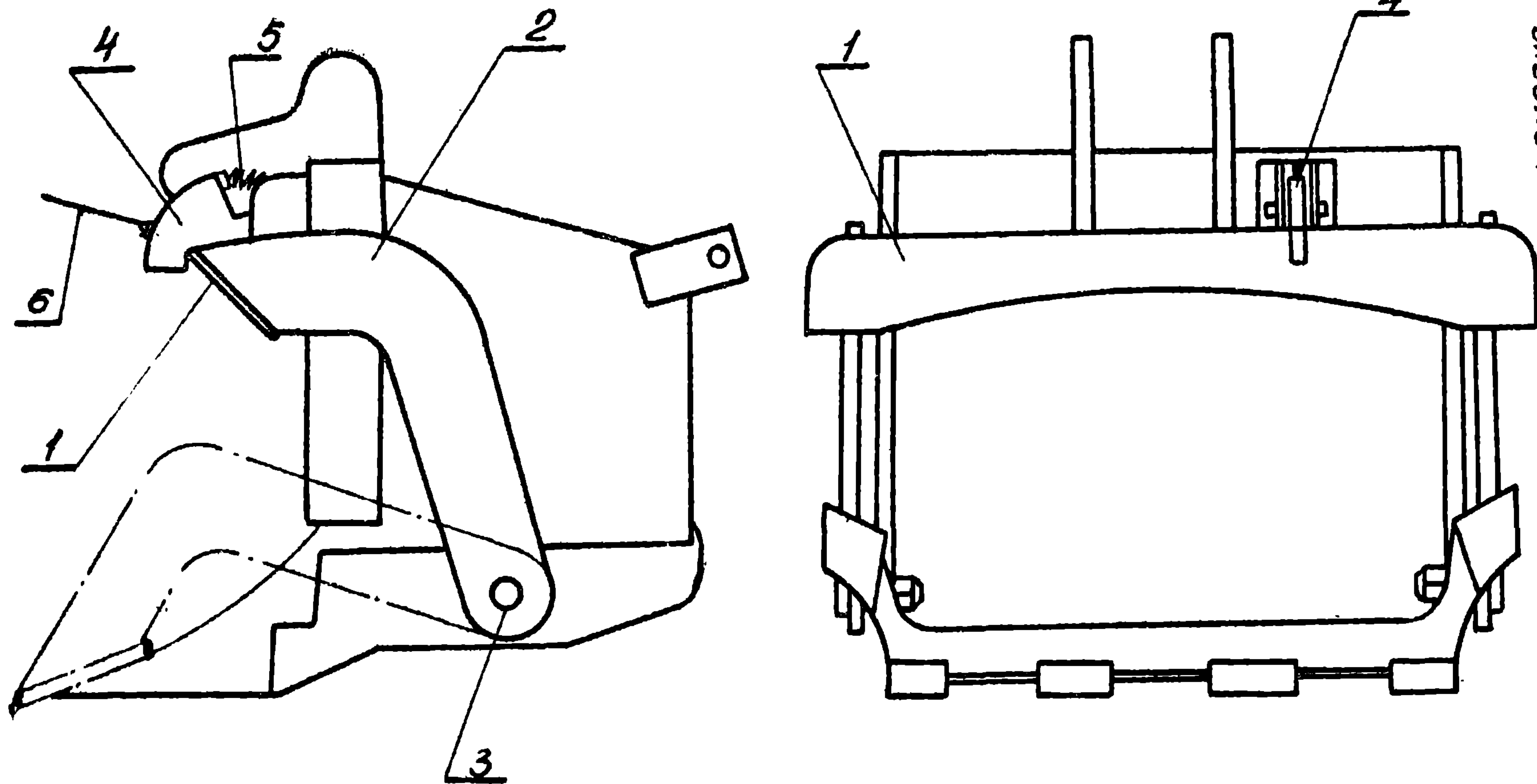
Рис. 4 Струг для зачистки дна траншей экскаватором
