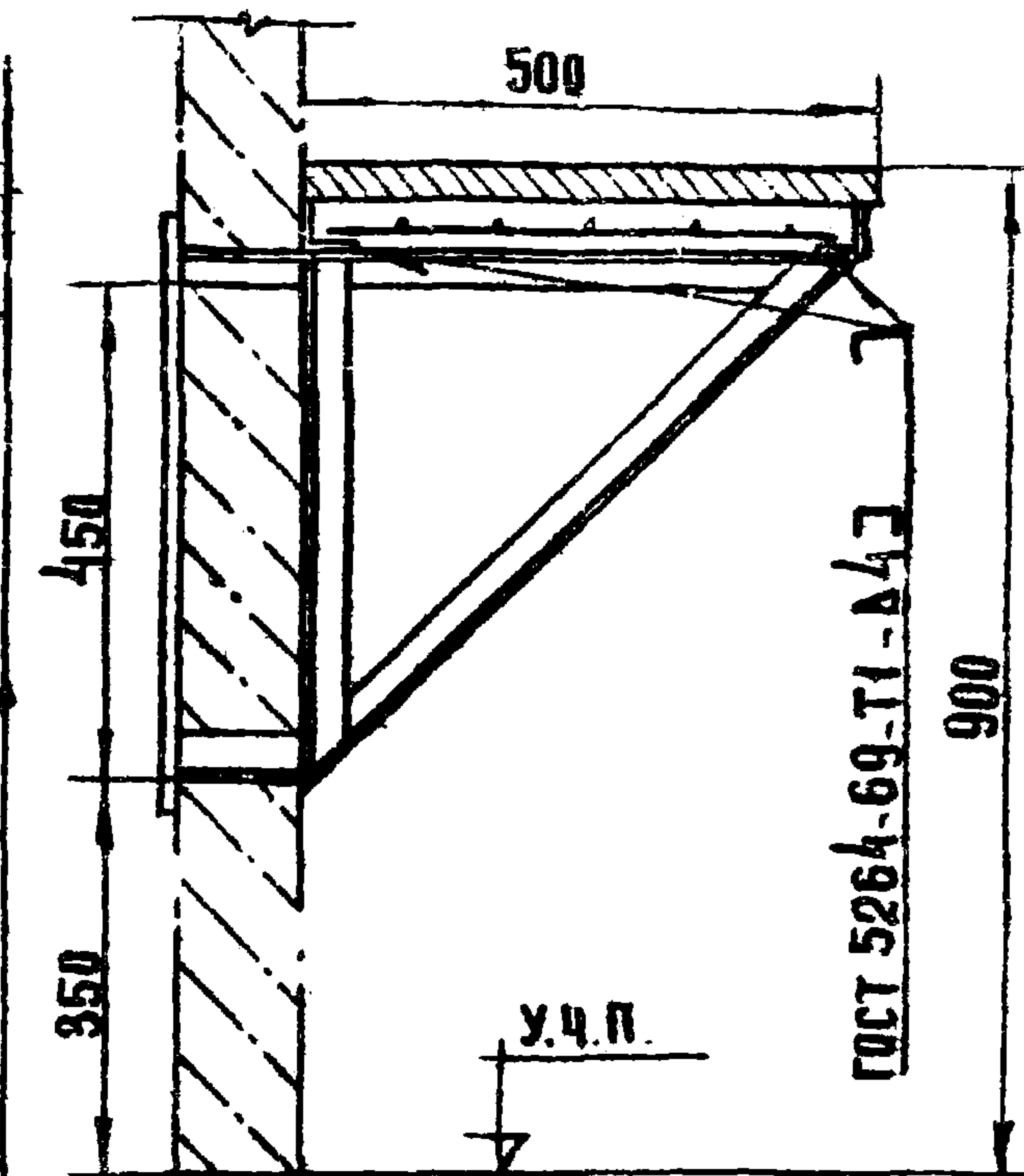
А-А
