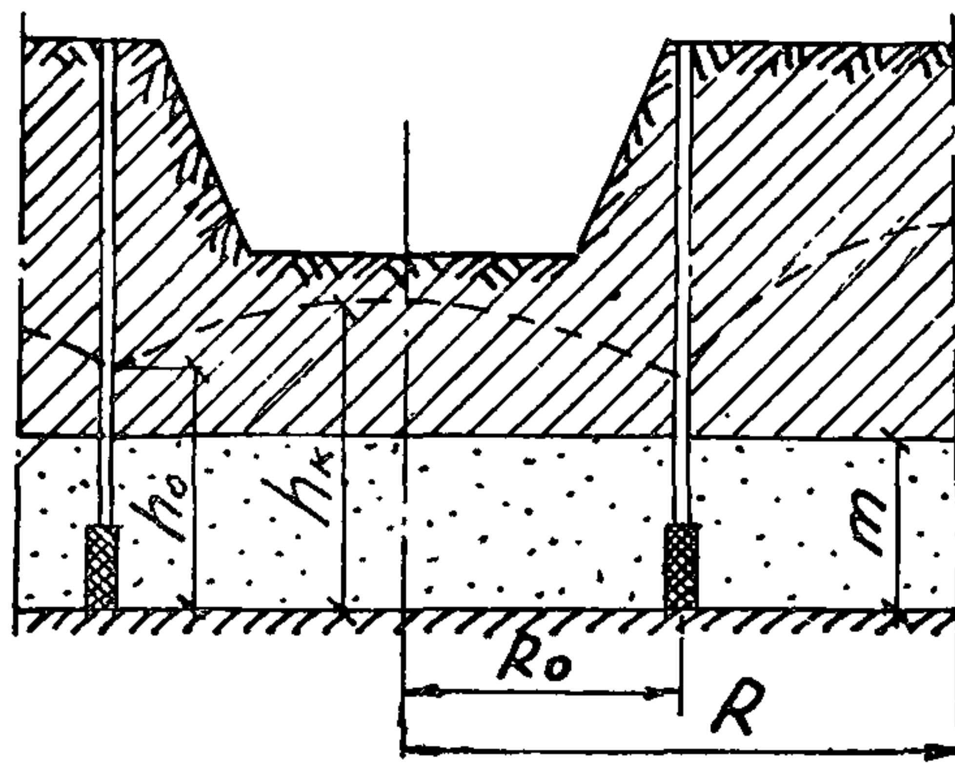
Рис. 2. Схема водопонижения при разработке котлована в условиях напорного водоносного горизонта
