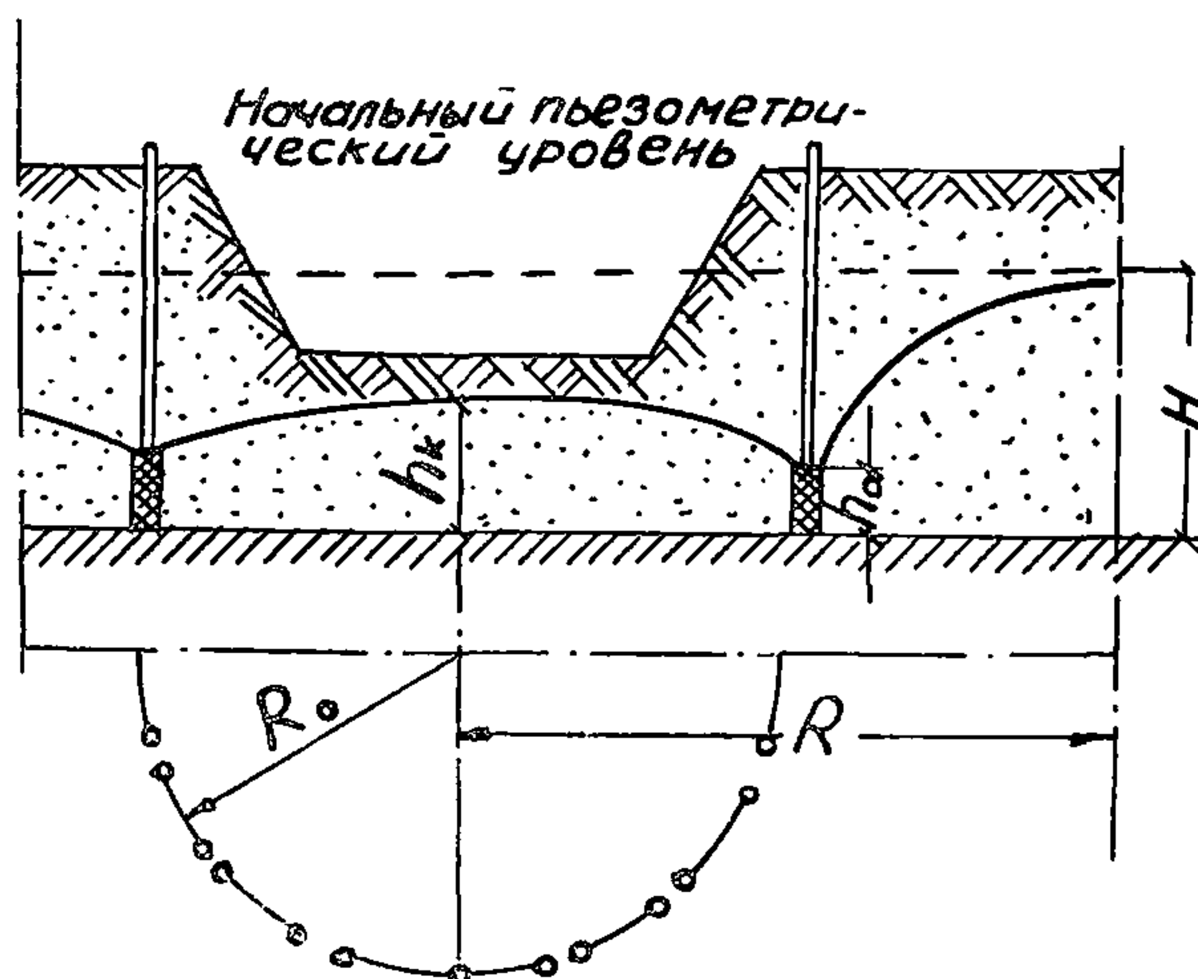
Рис. 1. Схема водопонижения при разработке котлована в безнапорных водах
