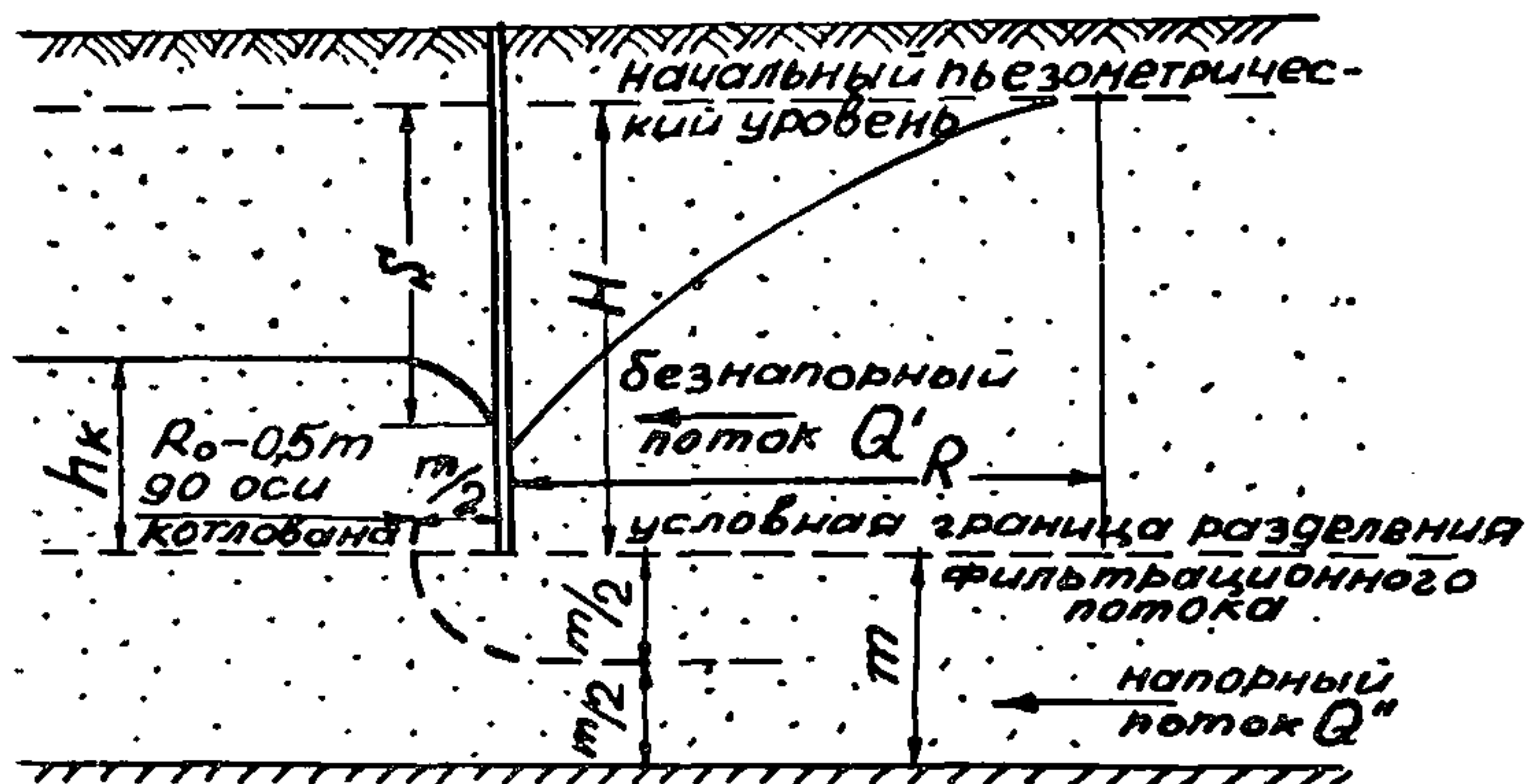
Рис. 3. Расчетная схема водопонижительной установки несовершенного типа
