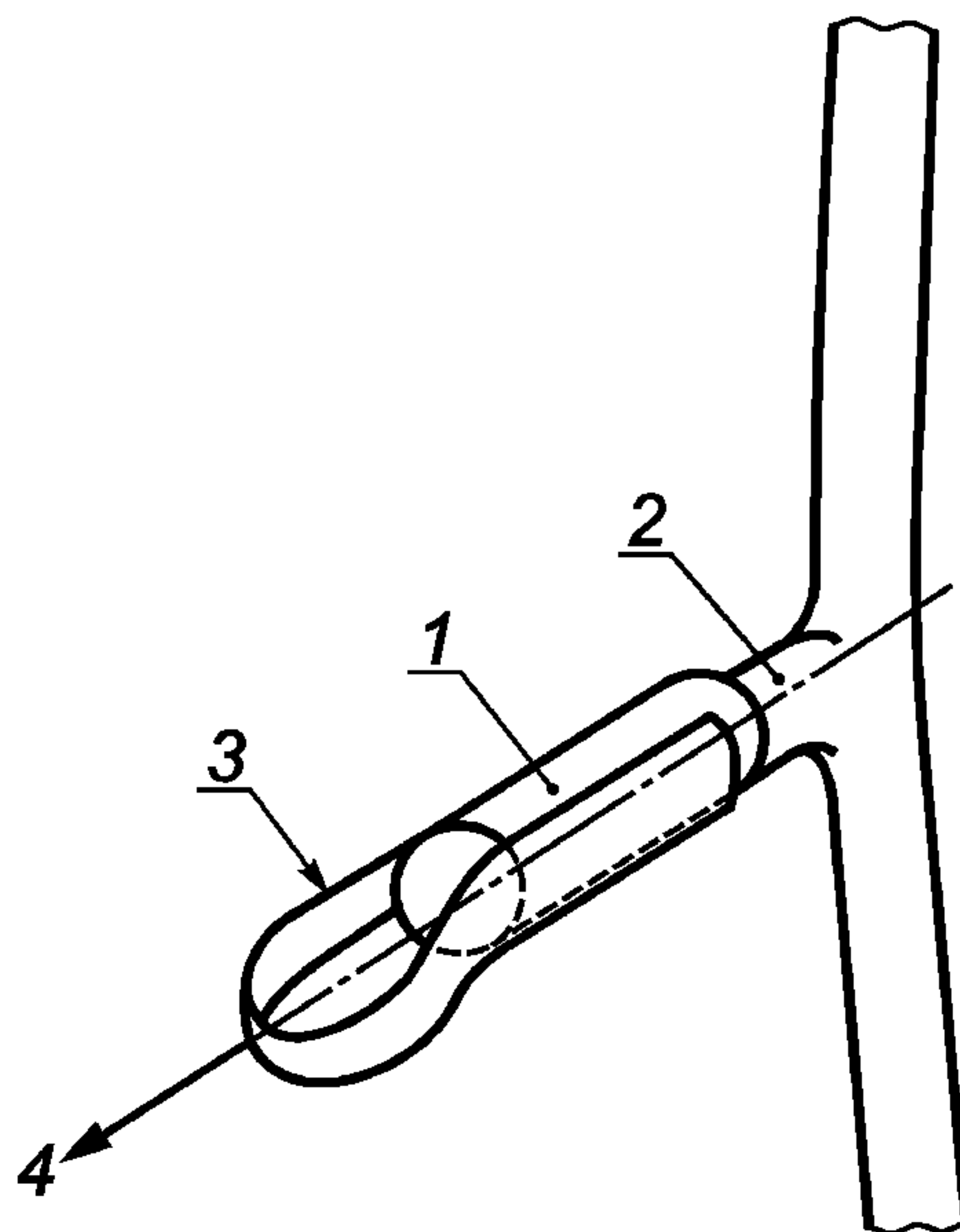
1 — рукоятка; 2 — ручка; 3 — петля из тесьмы; 4 — осевая нагрузка
