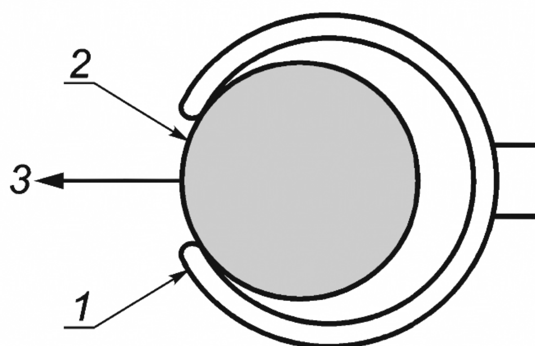
1 — манжета; 2 — цилиндр; 3 — сила растяжения
