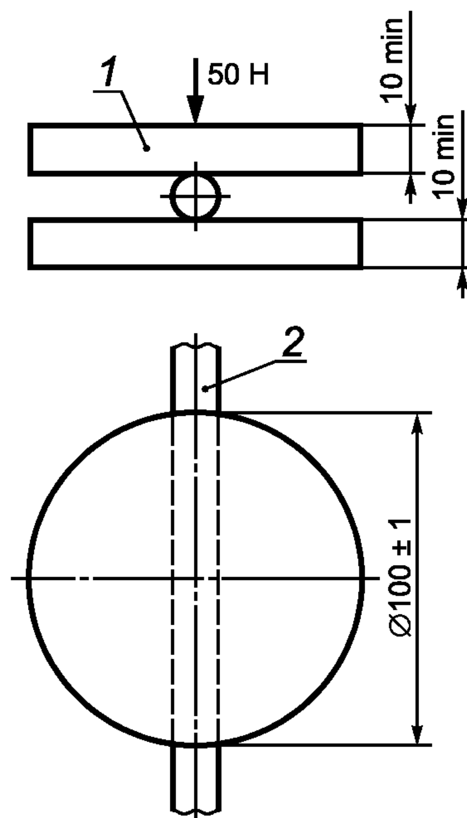
1 — подвижная пластина; 2 — дыхательный шланг
