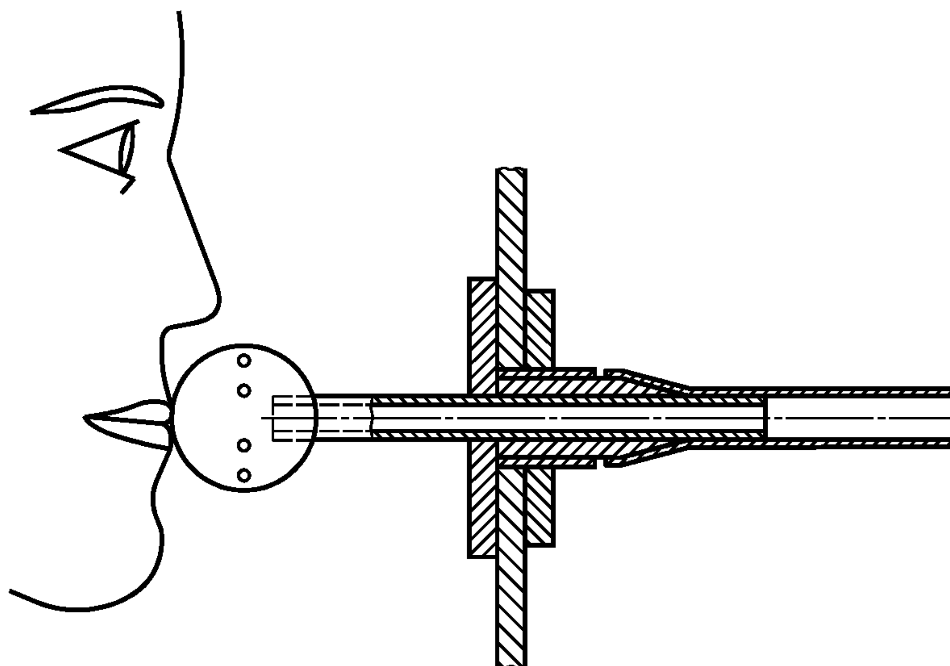
Рисунок 1 — Положение шарового пробоотборника
