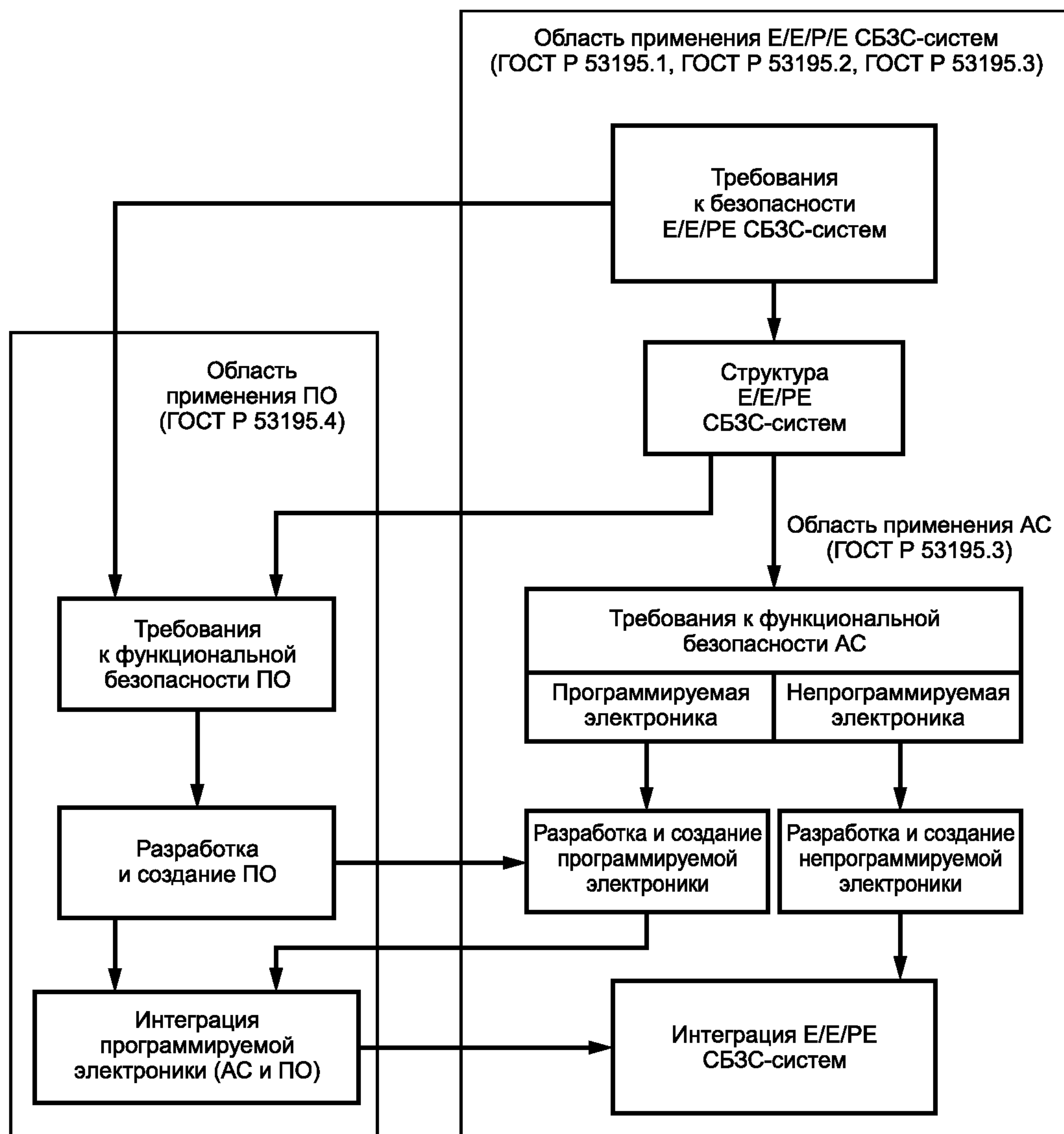
Рисунок 1 — Взаимосвязь областей применения АС и ПО
