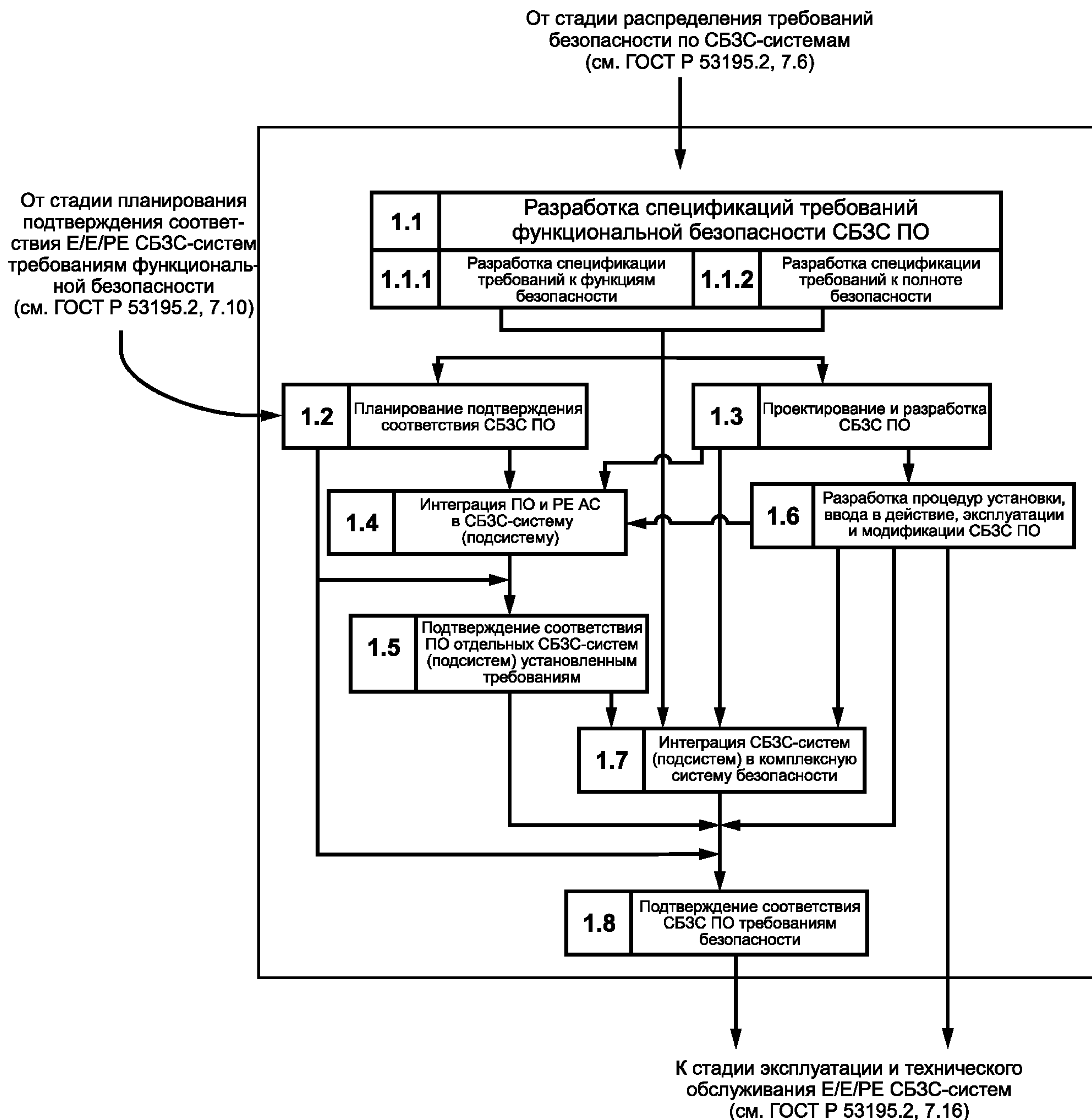
Рисунок 3 — Детализация стадии реализации жизненного цикла СБЗС ПО
