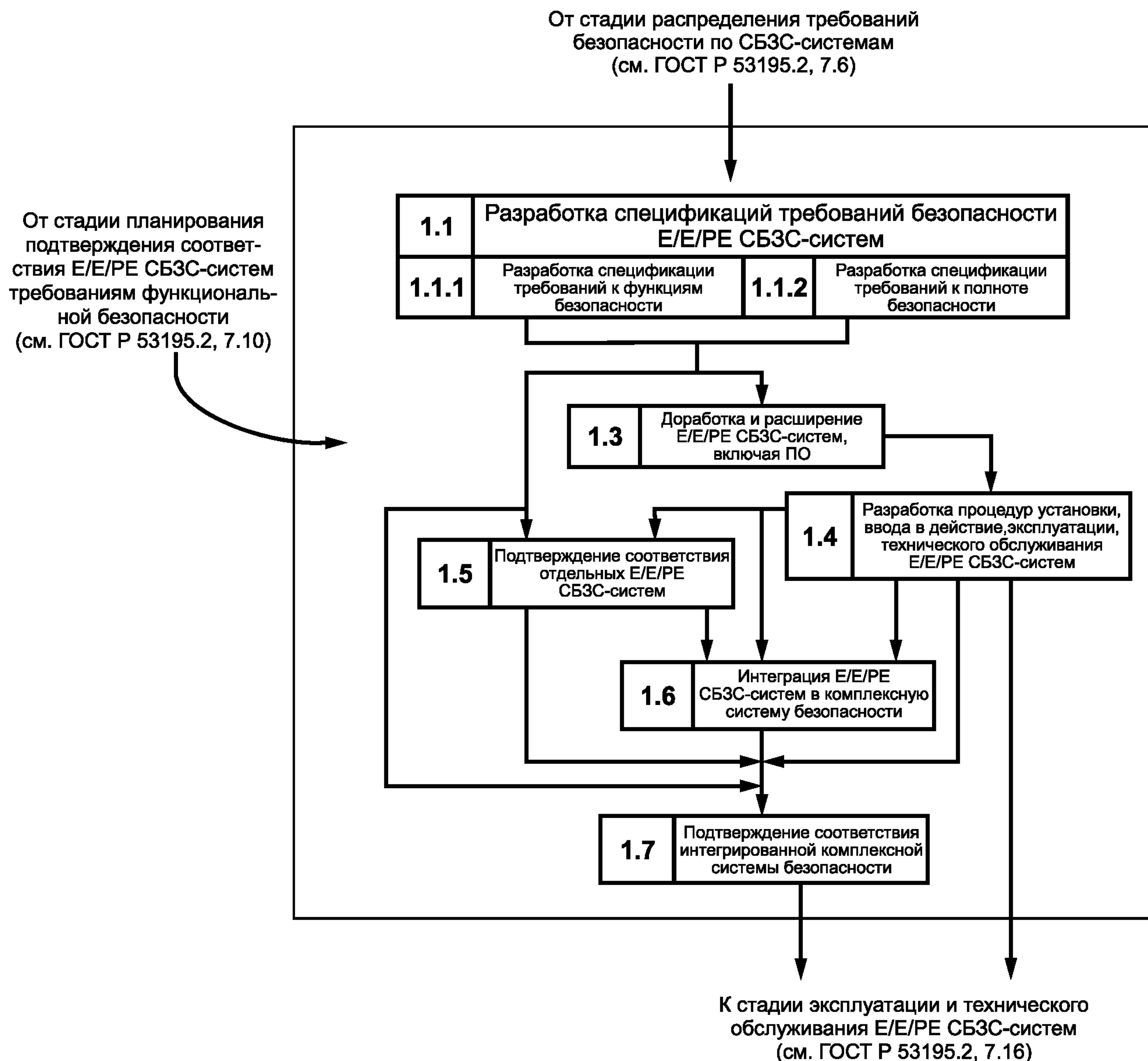
Рисунок 2 — Детализация стадии реализации жизненного цикла Е/Е/РЕ СБЗС-системы
