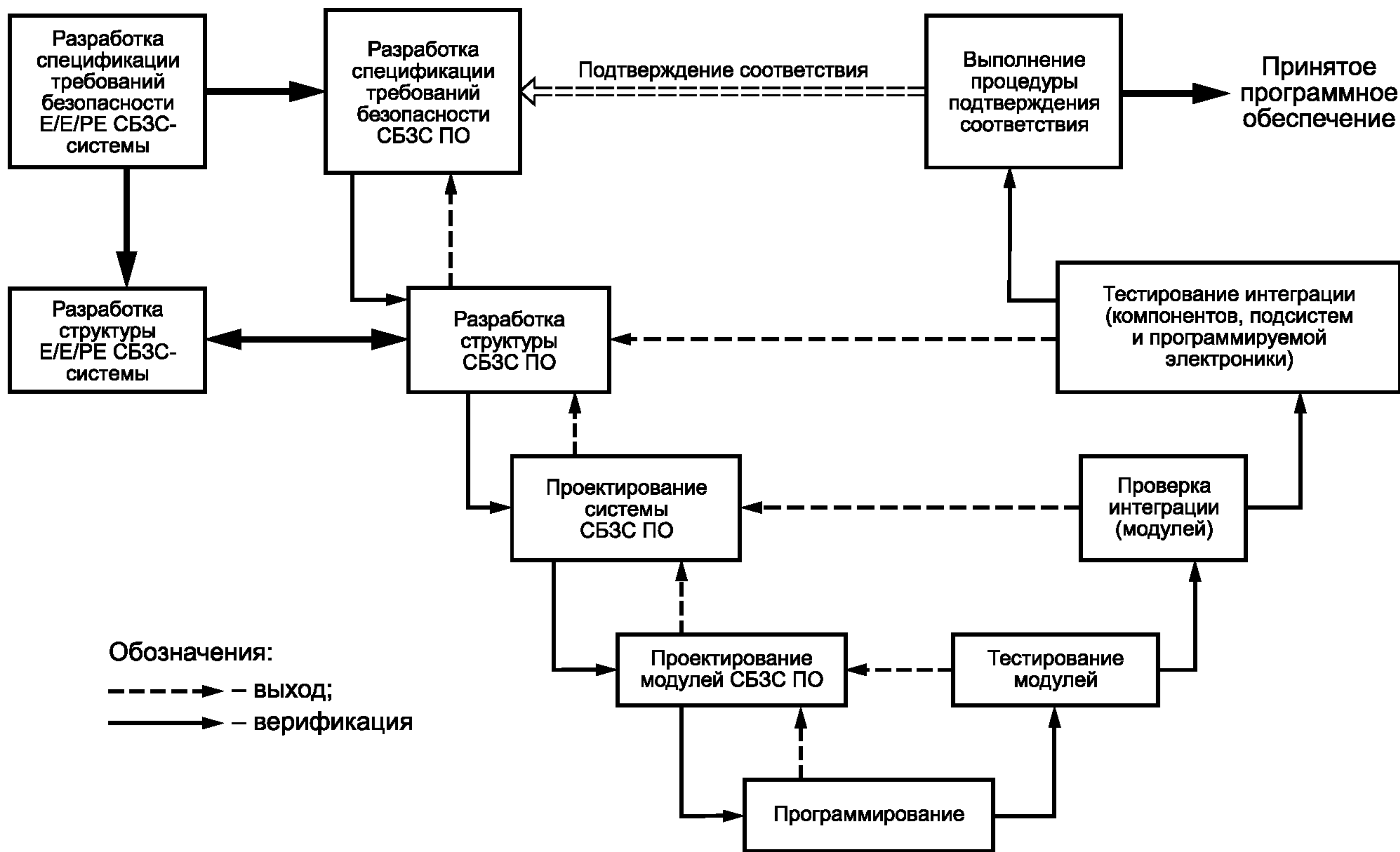
Рисунок 4 — V-модель проектирования и разработки СБЗС ПО
