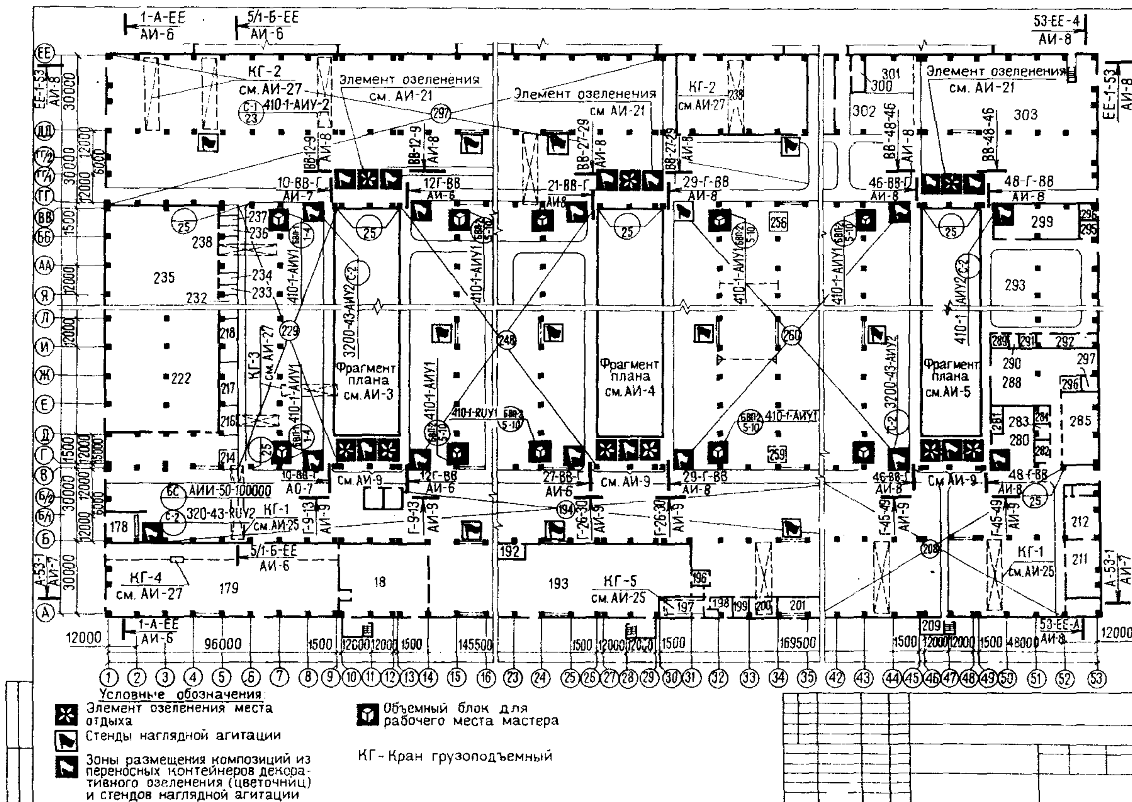
Рис. 35. Пример выполнения рабочего чертежа плана марки АИ
