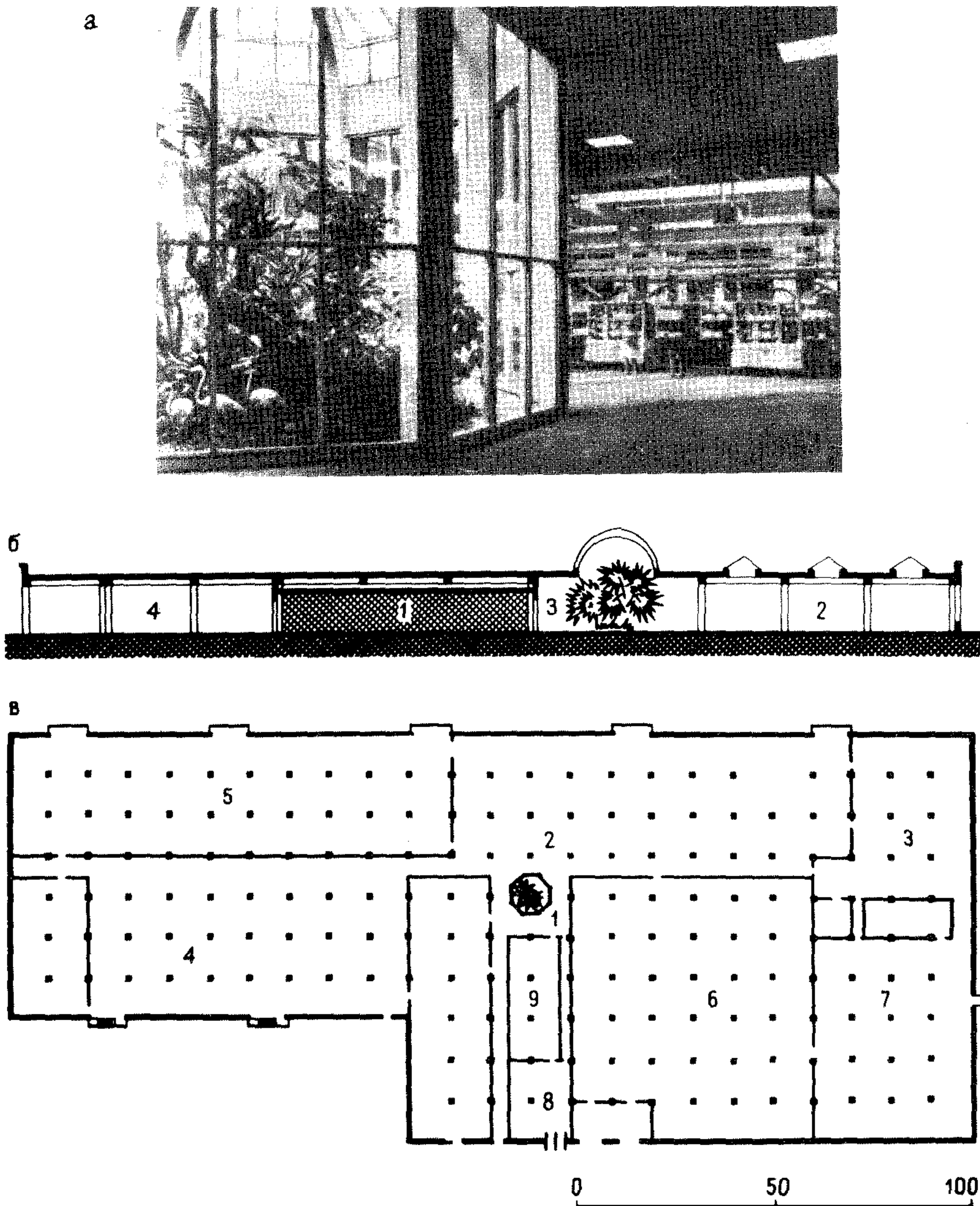
Рис. 30. Пример изолированного размещения озеленения внутри остекленной оранжереи в интерьере производственных помещений фарфорового завода (ФРГ)
